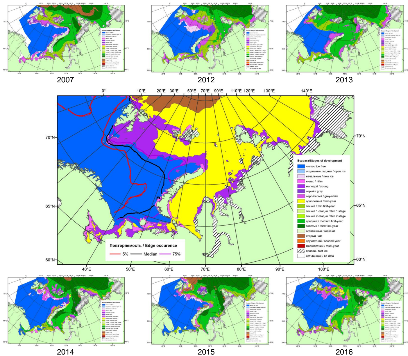
Рисунок 3 – Обзорная ледовая карта акваторий нац. парка «Русская Арктика» и заповедных территорий Таймыра за 14.03.2017 г. и аналогичные периоды 2007-2016 гг. на основе ледового анализа ААНИИ и Национального ледового центра США.
