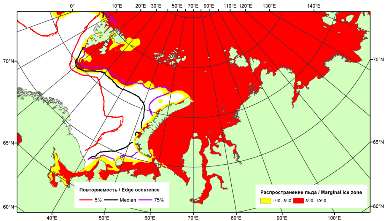
Рисунок 2 – Положение кромки льда (районов безледокольного плавания) и сплошных льдов акваторий нац. парка «Русская Арктика» и заповедных территорий Таймыра за 13.03.2017 г. на основе ледового анализа Национального Ледового Центра США и повторяемость кромки за 11-15.03 за период 1979-2012 гг. по наблюдениям SSMR-SSM/I-SSMIS (алгоритм NASATEAM)
