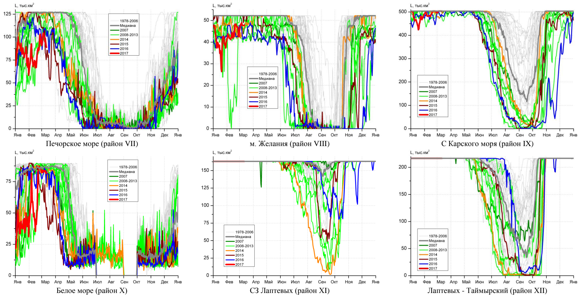
Рисунок 4 – Ежедневные оценки сезонного хода ледовитости для акваторий (рис.7) нац. парка «Русская Арктика» и заповедных территорий Таймыра за период 26.10.1978 – 12.03.2017 по годам на основе расчетов по данным SSMR-SSM/I-SSMIS-AMSR2, алгоритм NASATEAM/BOOTSTRAP.
