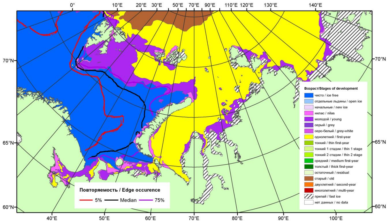
Рисунок 1 – Обзорная ледовая карта акваторий нац. парка «Русская Арктика» и заповедных территорий Таймыра за 14.03.2017 г. на основе ледового анализа ААНИИ (14.03.2017) и повторяемость кромки за 11-15.03 за период 1979-2012 гг. по наблюдениям SSMR-SSM/I-SSMIS (алгоритм NASATEAM).
