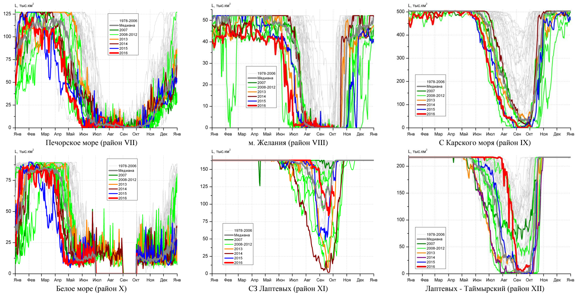
Рисунок 4 – Ежедневные оценки сезонного хода ледовитости для акваторий (рис.7) нац. парка «Русская Арктика» и заповедных территорий Таймыра за период 26.10.1978 – 02.10.2016 по годам на основе расчетов по данным SSMR-SSM/I-SSMIS-AMSR2, алгоритм NASATEAM/BOOTSTRAP.
