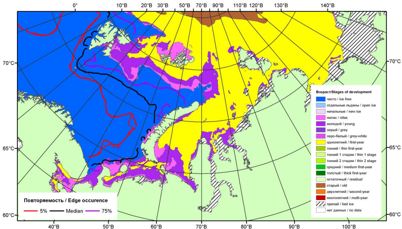
Рисунок 1 – Обзорная ледовая карта акваторий нац. парка «Русская Арктика» и заповедных территорий Таймыра за 02.02.2016 г. на основе ледового анализа ААНИИ (02.02.2016) и повторяемость кромки за 01-05.02 за период 1979-2012 гг. по наблюдениям SSMR-SSM/I-SSMIS (алгоритм NASATEAM).
