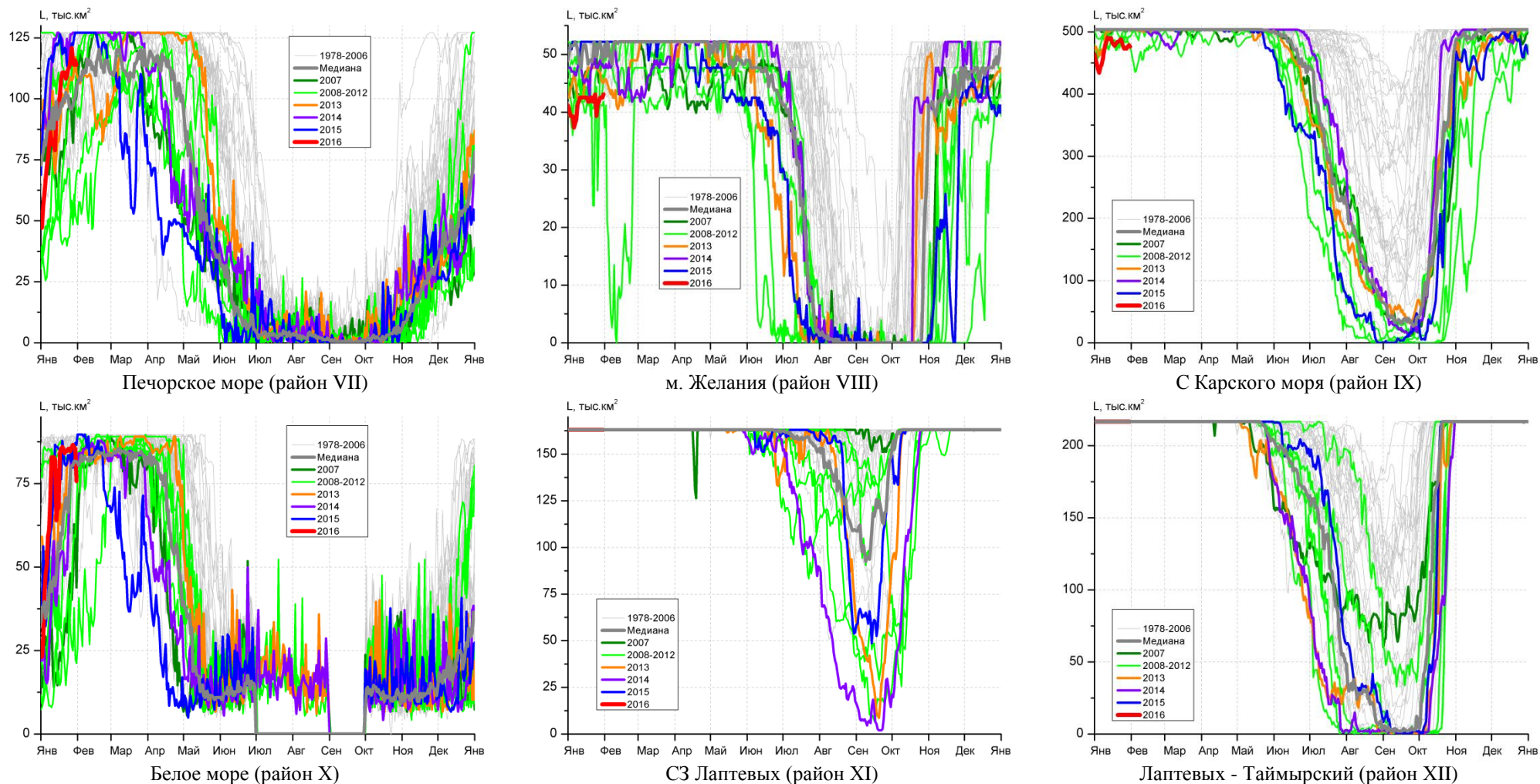
Рисунок 4 – Ежедневные оценки сезонного хода ледовитости для акваторий (рис.7) нац. парка «Русская Арктика» и заповедных территорий Таймыра за период 26.10.1978 – 31.01.2016 по годам на основе расчетов по данным SSMR-SSM/I-SSMIS-AMSR2, алгоритм NASATEAM/BOOTSTRAP.
