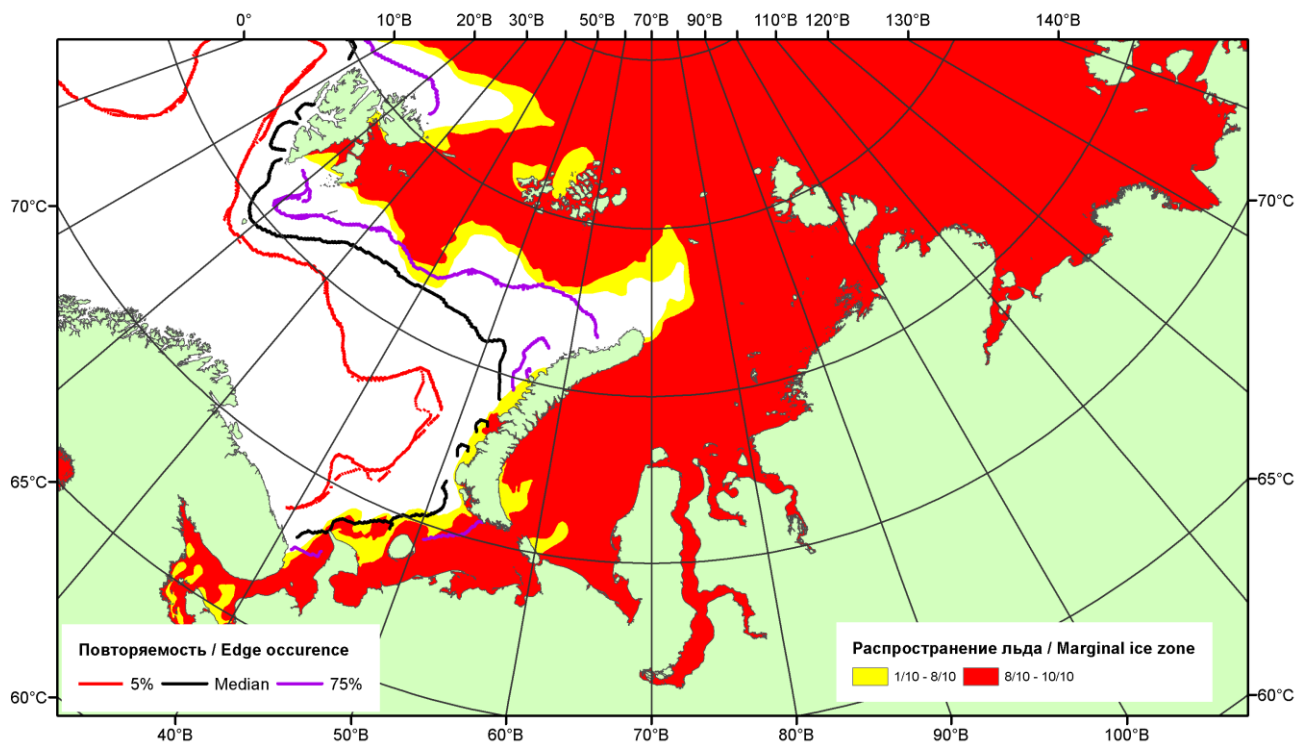
Рисунок 2 – Положение кромки льда (районов безледокольного плавания) и сплошных льдов акваторий нац. парка «Русская Арктика» и заповедных территорий Таймыра за 01.02.2016 г. на основе ледового анализа Национального Ледового Центра США и повторяемость кромки за 01-05.02 за период 1979-2012 гг. по наблюдениям SSMR-SSM/I-SSMIS (алгоритм NASATEAM)
