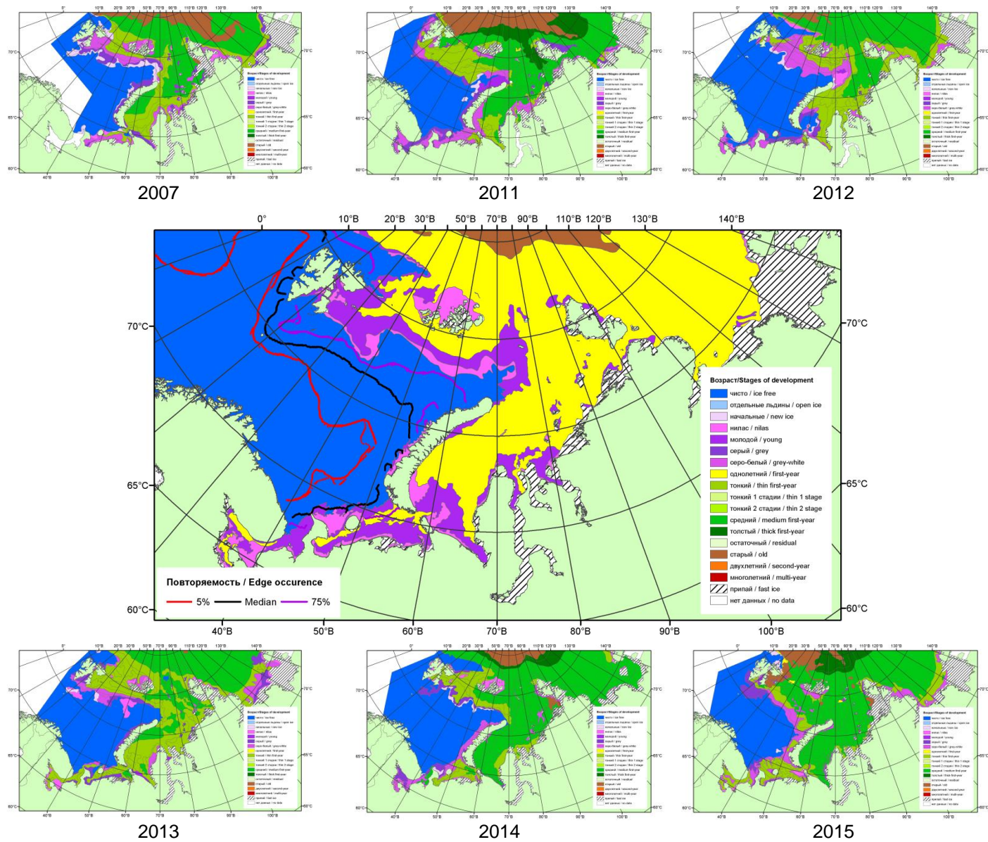
Рисунок 3 – Обзорная ледовая карта акваторий нац. парка «Русская Арктика» и заповедных территорий Таймыра за 02.02.2016 г. и аналогичные периоды 2007-2015 гг. на основе ледового анализа ААНИИ и Национального ледового центра США.
