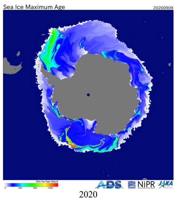
Рисунок 86 – Оценка максимального возраста льда (сутки) на 09.09 за 2018 – 2026 гг. по данным JAXA-NIPR [29]
