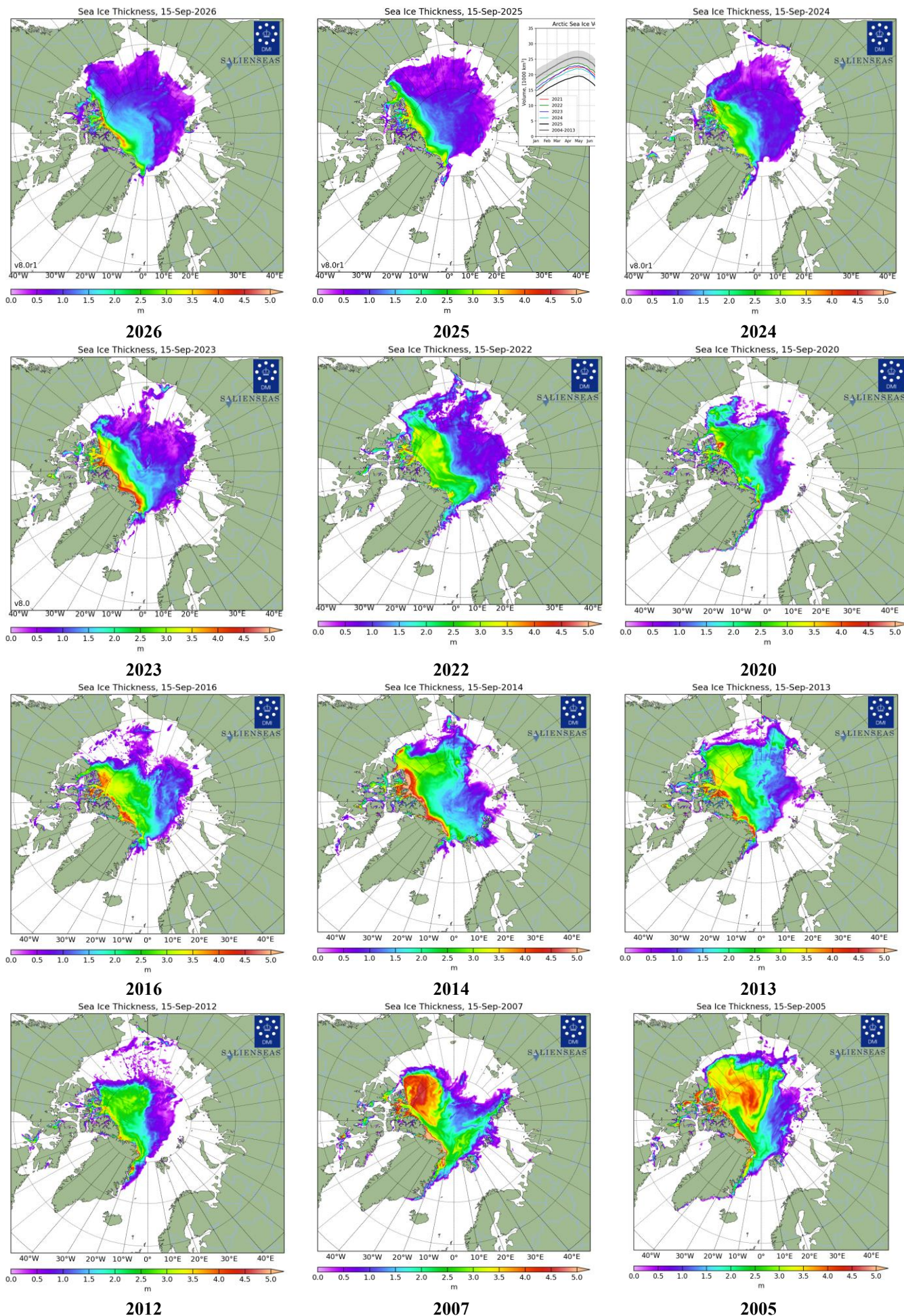
Рисунок 4в – Поля распределения средневзвешенной толщины льда совместной модели морского льда – океана HYCOM/CICE Датского метеорологического института 15.09 за 2005-2026 гг. [22].
