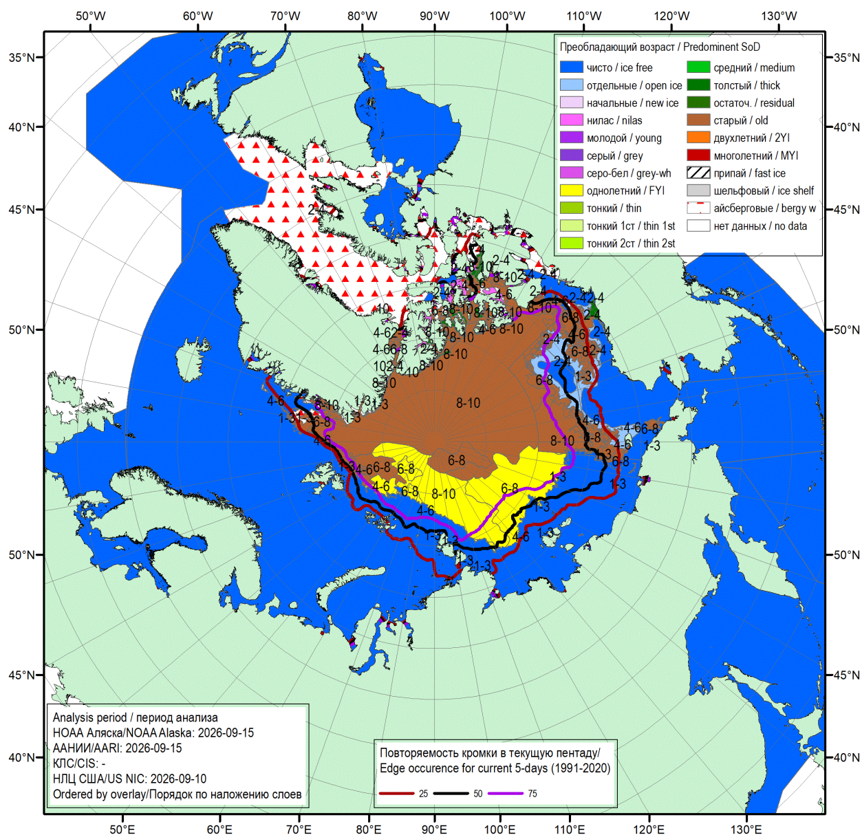
Рисунок 16 – Обзорная ледовая карта СЛО за 10.09.2026 – 15.09.2026 (цветовая раскраска по преобладающему возрасту) на основе ледового анализа NOAA Аляска, ААНИИ и Национального ледового центра США и повторяемость кромки за соответствующий 5-дневный период за 1991-2020 гг. по наблюдениям SSMR-SSM/I-SSMIS (алгоритм NASATEAM) [4, 10, 23, 17].
