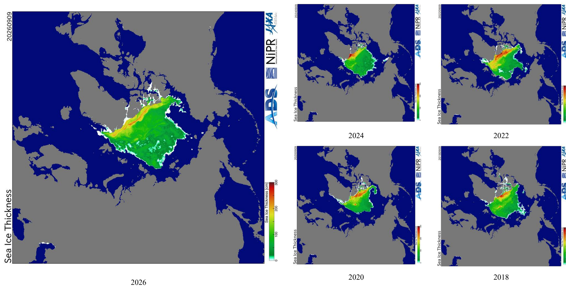
Рисунок 2а - Оценка толщины льда на основе данных пассивного микроволнового зондирования AMSR2 09.09 в 2018 – 2026 гг. [29].
