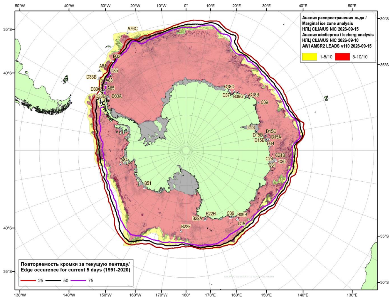
Рисунок 7в – Положение кромки льда и зон разреженных ( <8/10 ) и сплошных ( \geq 8/10 ) льдов Южного океана за 15.09.2026 и расположение крупных айсбергов за 10.09.2026 на основе ледового анализа Национального Ледового Центра США, повторяемость кромки за ближайшую пентаду за период 1991-2020 гг. по наблюдениям SSMR-SSM/I-SSMIS (алгоритм NASATEAM), совмещенное с положением разрежений на основе данных ИСЗ AMSR2 за 15.09.2026 (AWI-JAXA, v110) [10, 17, 24]
