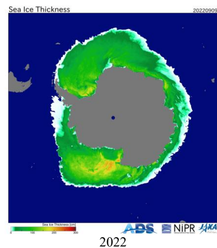
Рисунок 8а - Оценка толщины льда на основе данных пассивного микроволнового зондирования AMSR2 09.09 в 2018 – 2026 гг. [29].
