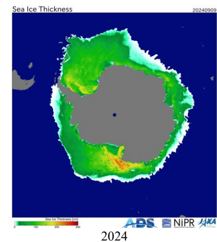
Рисунок 8а - Оценка толщины льда на основе данных пассивного микроволнового зондирования AMSR2 09.09 в 2018 – 2026 гг. [29].
