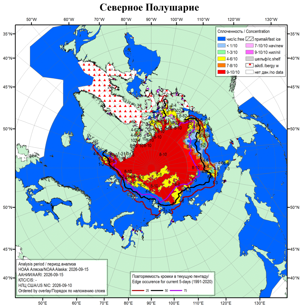
Рисунок 1а – Обзорная ледовая карта СЛО за 10.09.2026 – 15.09.2026 (цветовая раскраска по общей сплоченности) на основе ледового анализа НОАА Аляска, ААНИИ и Национального ледового центра США и повторяемость кромки за соответствующий 5-дневный период за 1991-2020 гг. по наблюдениям SSMR-SSM/I-SSMIS (алгоритм NASATEAM) [4, 10, 23, 17].
