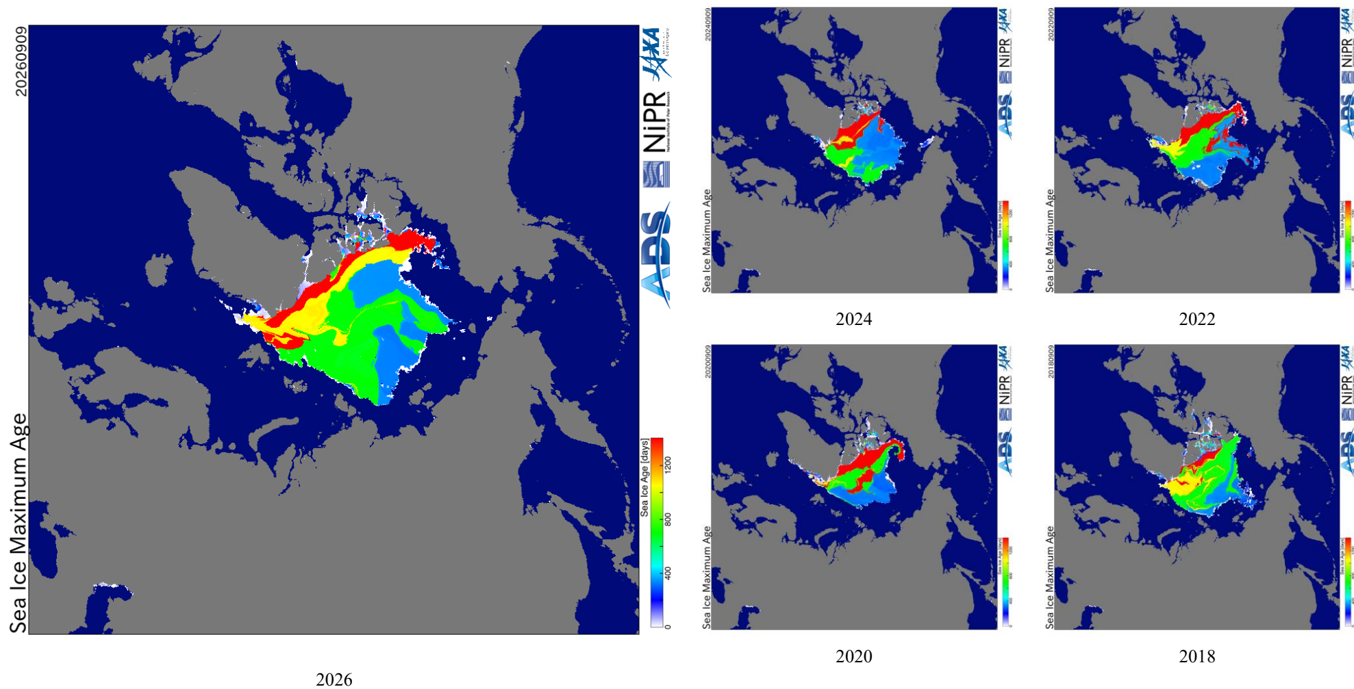
Рисунок 46 – Оценка максимального возраста льда (сутки) на 09.09 за 2018 – 2026 гг. по данным JAXA-NIPR [29]
