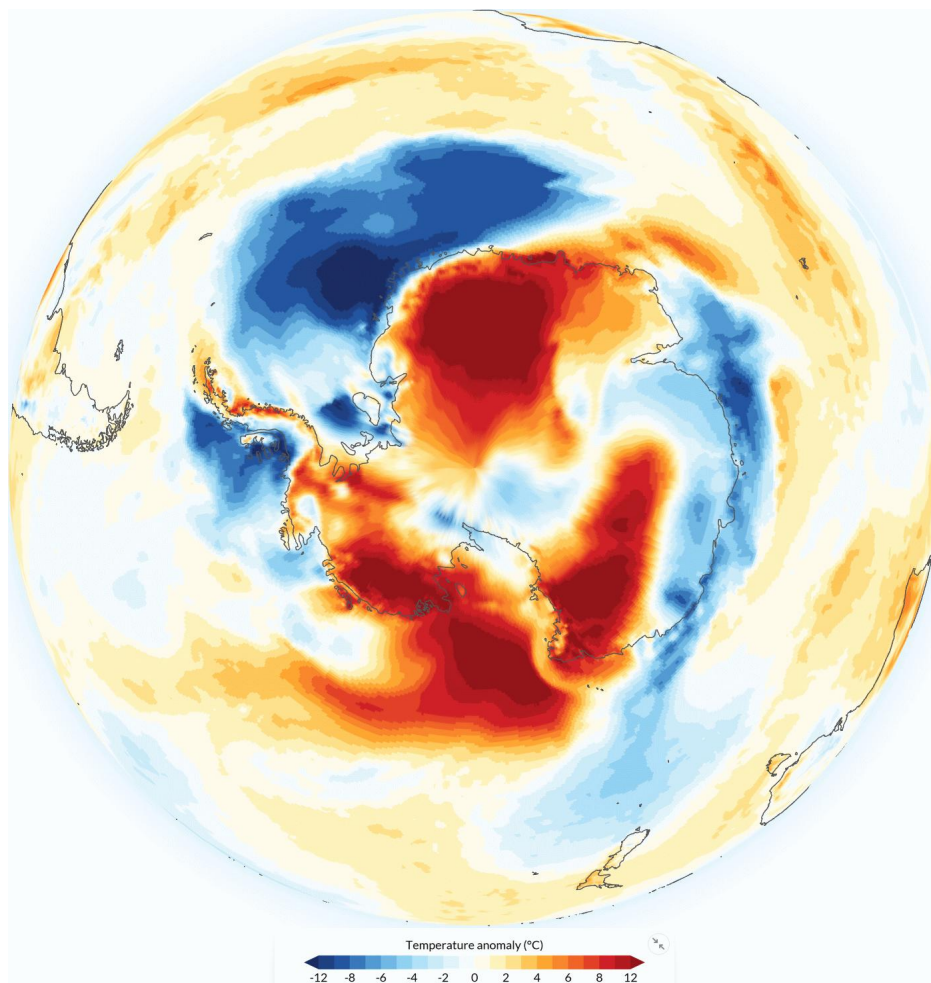
Рисунок 5а – Аномалия приземной температуры воздуха (2м) и температуры поверхности моря на 14.09.2026 г. относительно периода 1991-2020 гг. - The Copernicus Climate Change Service (C3S) , implemented by the European Centre for Medium-Range Weather Forecasts (ECMWF) on behalf of the European Commission is part of the European Union's space programme
