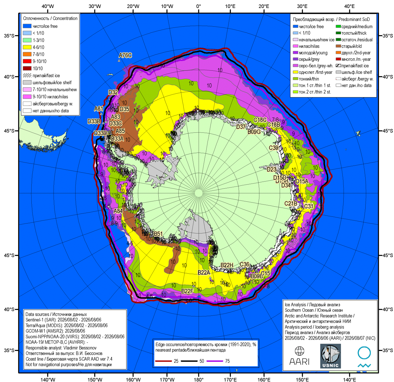
Рисунок 76 – Ледовая карта Южного океана (цветовая окраска по возрасту) и расположение крупных айсбергов на основе ледового анализа за 06.08.2026 в рамках проекта совместного ледового картирования Южного океана ААНИИ, НЛЦ США и НМИ и повторяемость кромки за ближайшую пентаду за период 1991-2020 гг. по наблюдениям SSMR-SSM/I-SSMIS (алгоритм NASATEAM) [5, 10, 17, 21].
