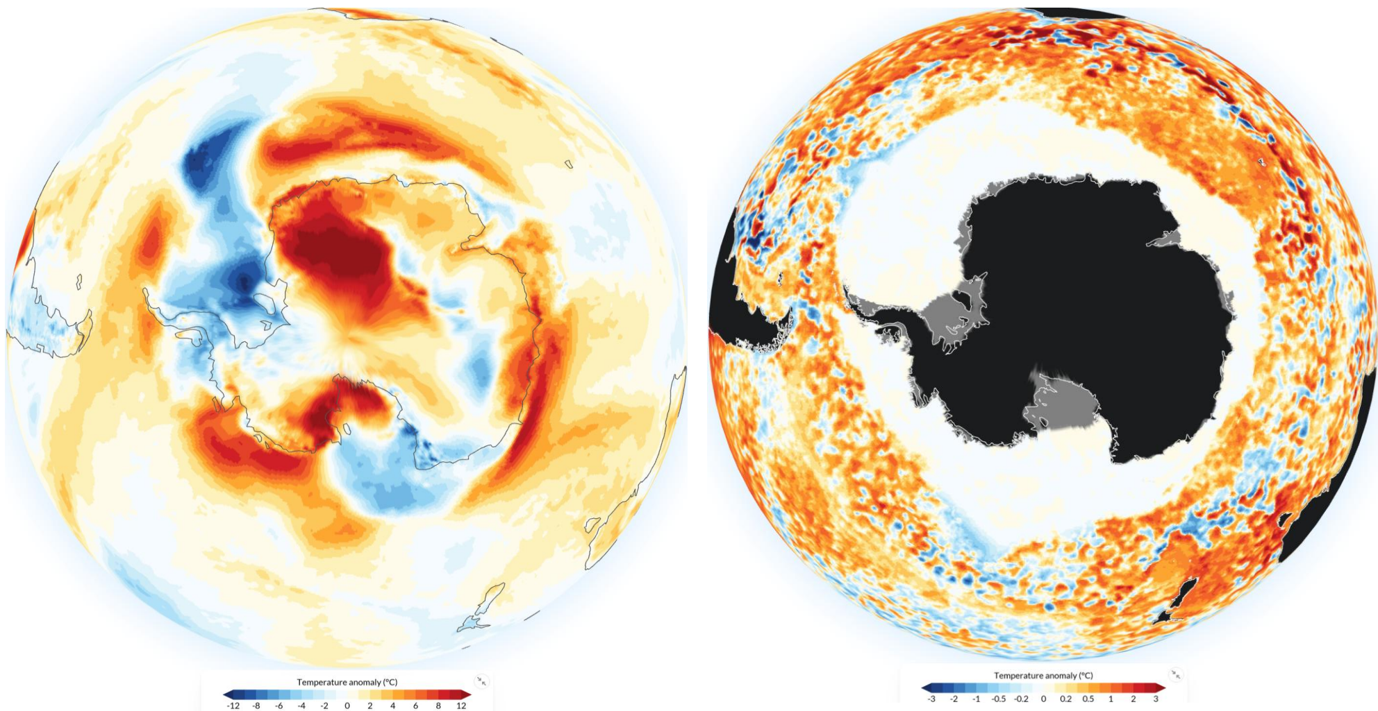
Рисунок 9 – Аномалия приземной температуры воздуха (2м) на 16.08.2026 г. относительно периода 1991-2020 гг. - The Copernicus Climate Change Service (C3S) , implemented by the European Centre for Medium-Range Weather Forecasts (ECMWF) on behalf of the European Commission is part of the European Union's space programme.
