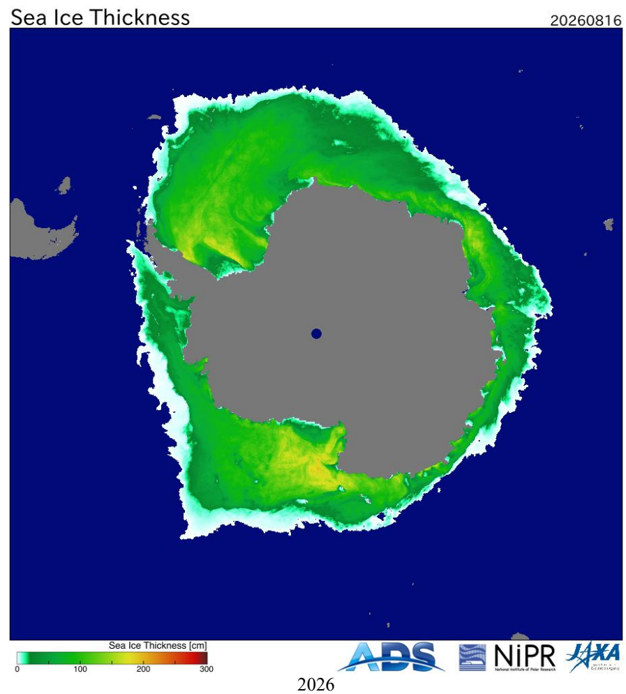
Рисунок 8а - Оценка толщины льда на основе данных пассивного микроволнового зондирования AMSR2 16.08 в 2018 – 2026 гг. [29].
