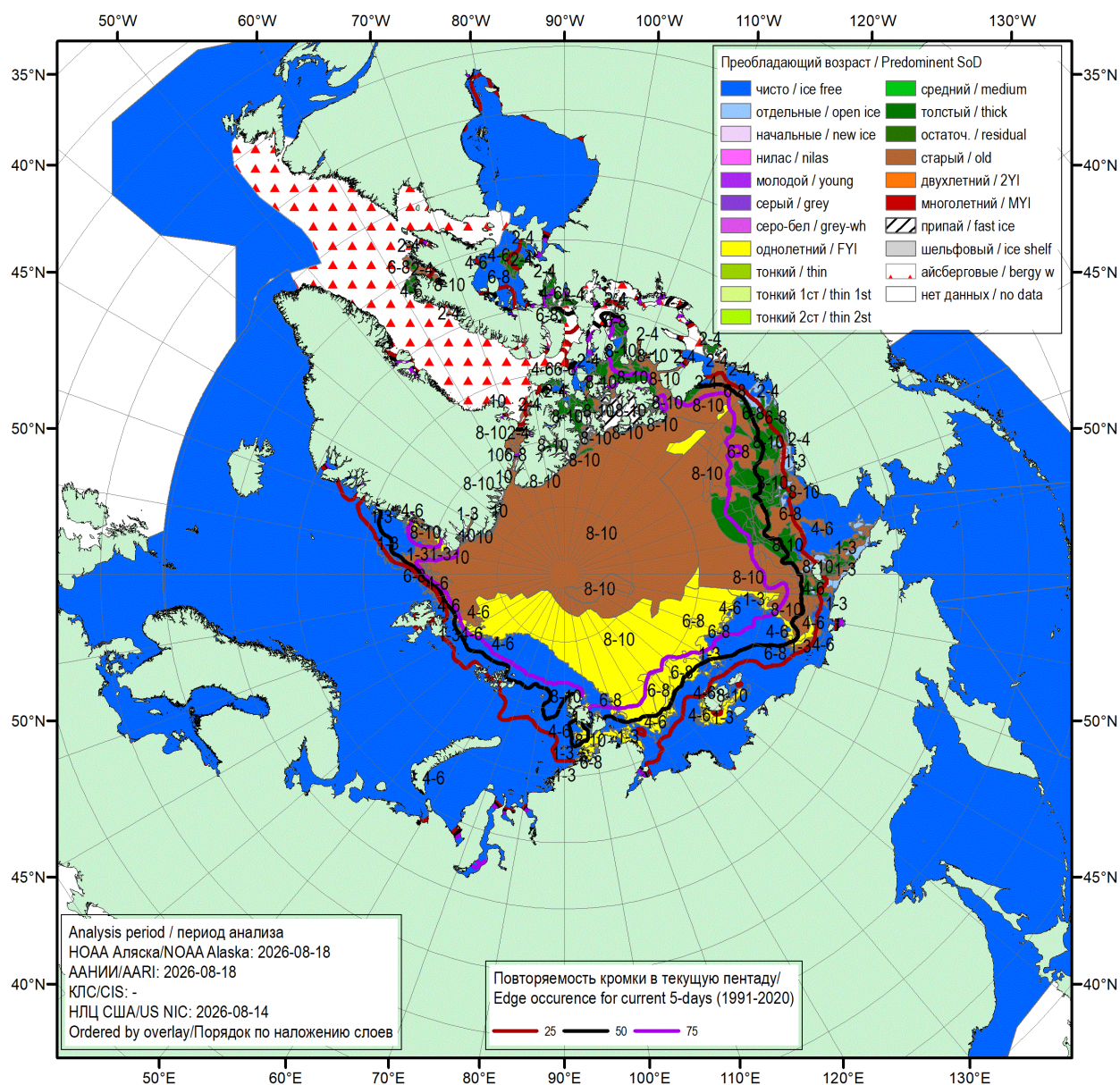
Рисунок 16 – Обзорная ледовая карта СЛО за 14.08.2026 – 18.08.2026 (цветовая раскраска по преобладающему возрасту) на основе ледового анализа NOAA Аляска, ААНИИ и Национального ледового центра США и повторяемость кромки за соответствующий 5-дневный период за 1991-2020 гг. по наблюдениям SSMR-SSM/I-SSMIS (алгоритм NASATEAM) [4, 10, 23, 17].
