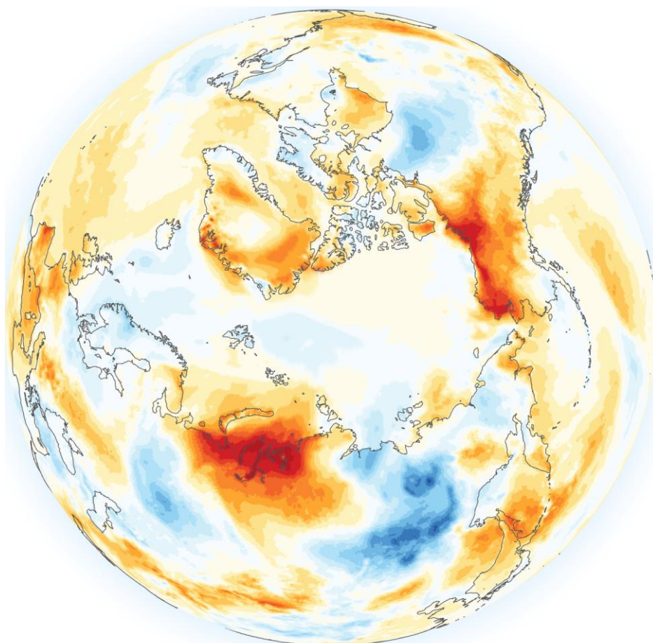
Рисунок 5а – Аномалия приземной температуры воздуха (2м) и температуры поверхности моря на 16.08.2026 г. относительно периода 1991-2020 гг. - The Copernicus Climate Change Service (C3S) , implemented by the European Centre for Medium-Range Weather Forecasts (ECMWF) on behalf of the European Commission is part of the European Union's space programme
