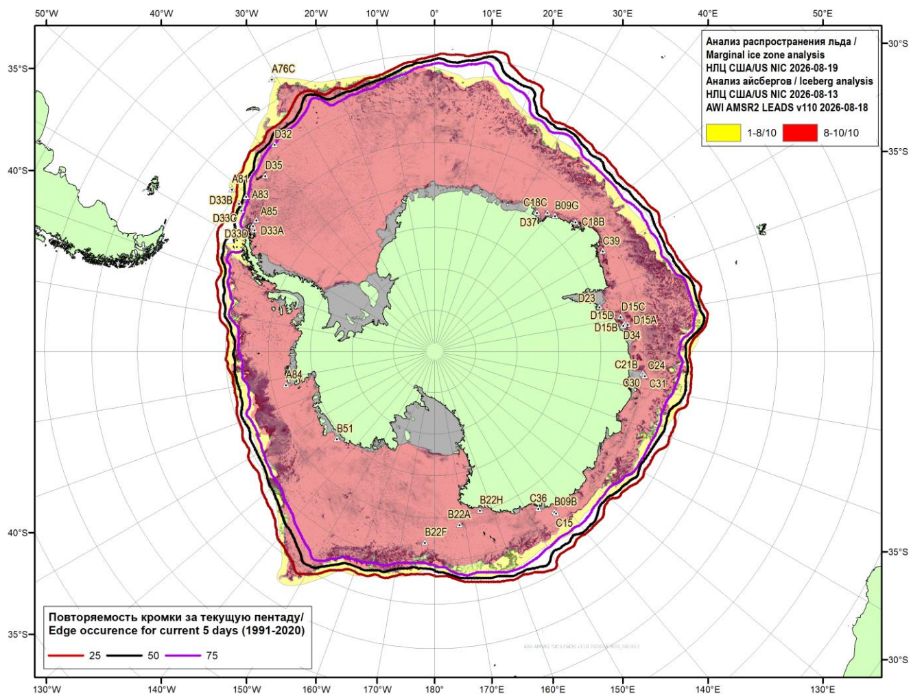
Рисунок 7в – Положение кромки льда и зон разреженных ( <8/10 ) и сплоченных ( \geq 8/10 ) льдов Южного океана за 19.08.2026 и расположение крупных айсбергов за 13.08.2026 на основе ледового анализа Национального Ледового Центра США, повторяемость кромки за ближайшую пентаду за период 1991-2020 гг. по наблюдениям SSMR-SSM/I-SSMIS (алгоритм NASATEAM), совмещенное с положением разрежений на основе данных ИСЗ AMSR2 за 18.08.2026 (AWI-JAXA, v110) [10, 17, 24]
