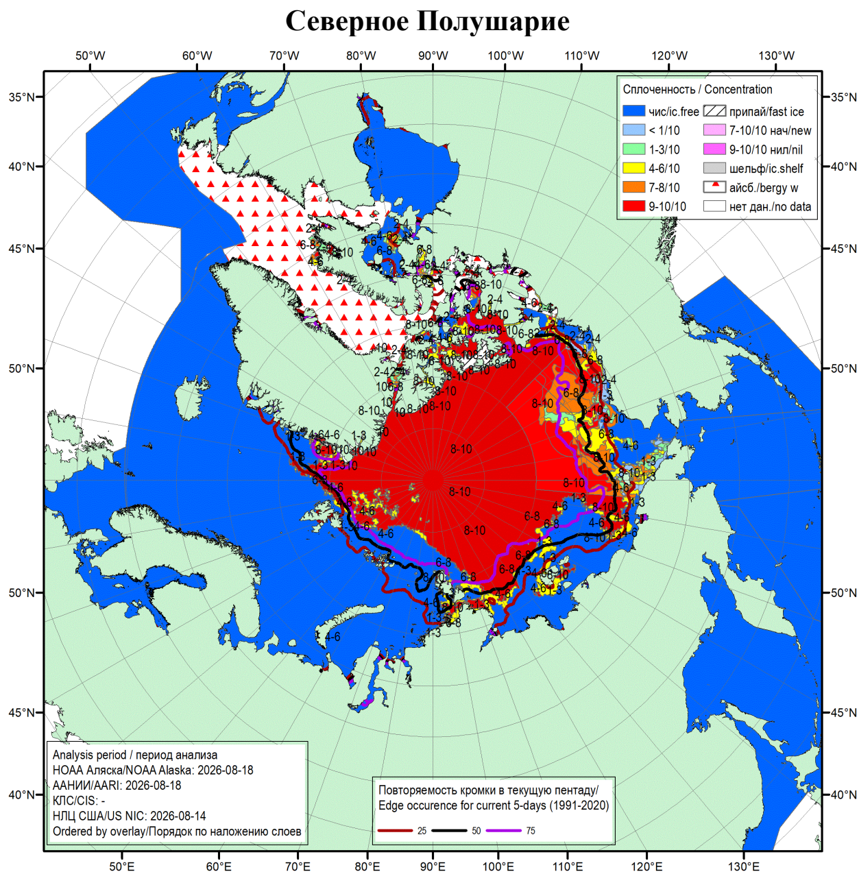
Рисунок 1а – Обзорная ледовая карта СЛО за 14.08.2026 – 18.08.2026 (цветовая раскраска по общей сплоченности) на основе ледового анализа НОАА Аляска, ААНИИ и Национального ледового центра США и повторяемость кромки за соответствующий 5-дневный период за 1991-2020 гг. по наблюдениям SSMR-SSM/I-SSMIS (алгоритм NASATEAM) [4, 10, 23, 17].
