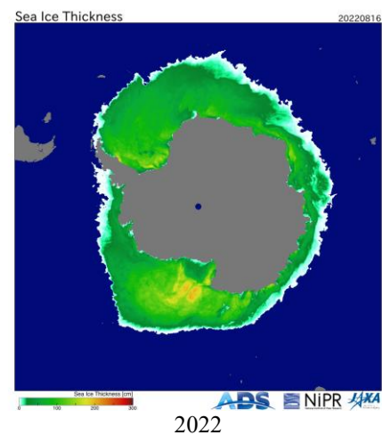
Рисунок 8а - Оценка толщины льда на основе данных пассивного микроволнового зондирования AMSR2 16.08 в 2018 – 2026 гг. [29].
