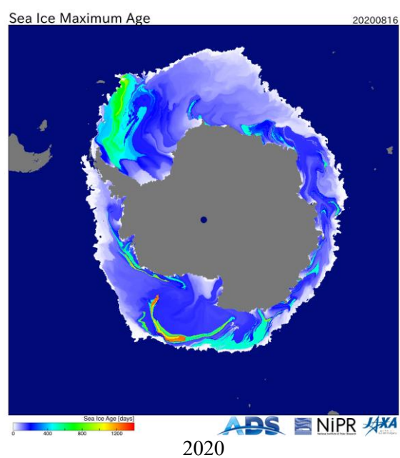
Рисунок 86 – Оценка максимального возраста льда (сутки) на 16.08 за 2018 – 2026 гг. по данным JAXA-NIPR [29]
