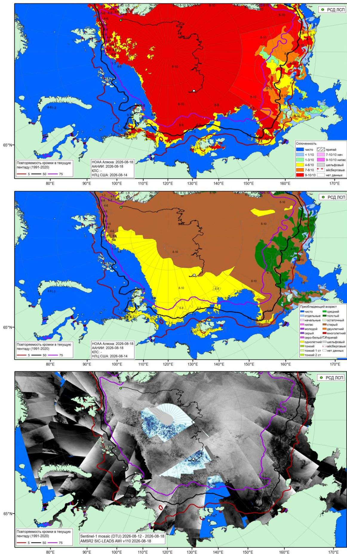
Рисунок 3 - Обзорная ледовая карта МП за 14.08-18.08.2026 г., мозаика радиолокационных снимком ИСЗ Sentinel-1AC за 12.08-18.08.2026 (DTU) с оценкой положения полыней за 18.08.2026 г. по данным AMSR2 (AWI-JAXA), повторяемость крошки за соответствующий 5-дневный период 1991-2020 гг. по наблюдениям SSMR-SSM/I-SSMIS (алгоритм NASATEAM) и положение РСН СП-42 на 19.08.2026 0600МСК [27, 28, 17].
