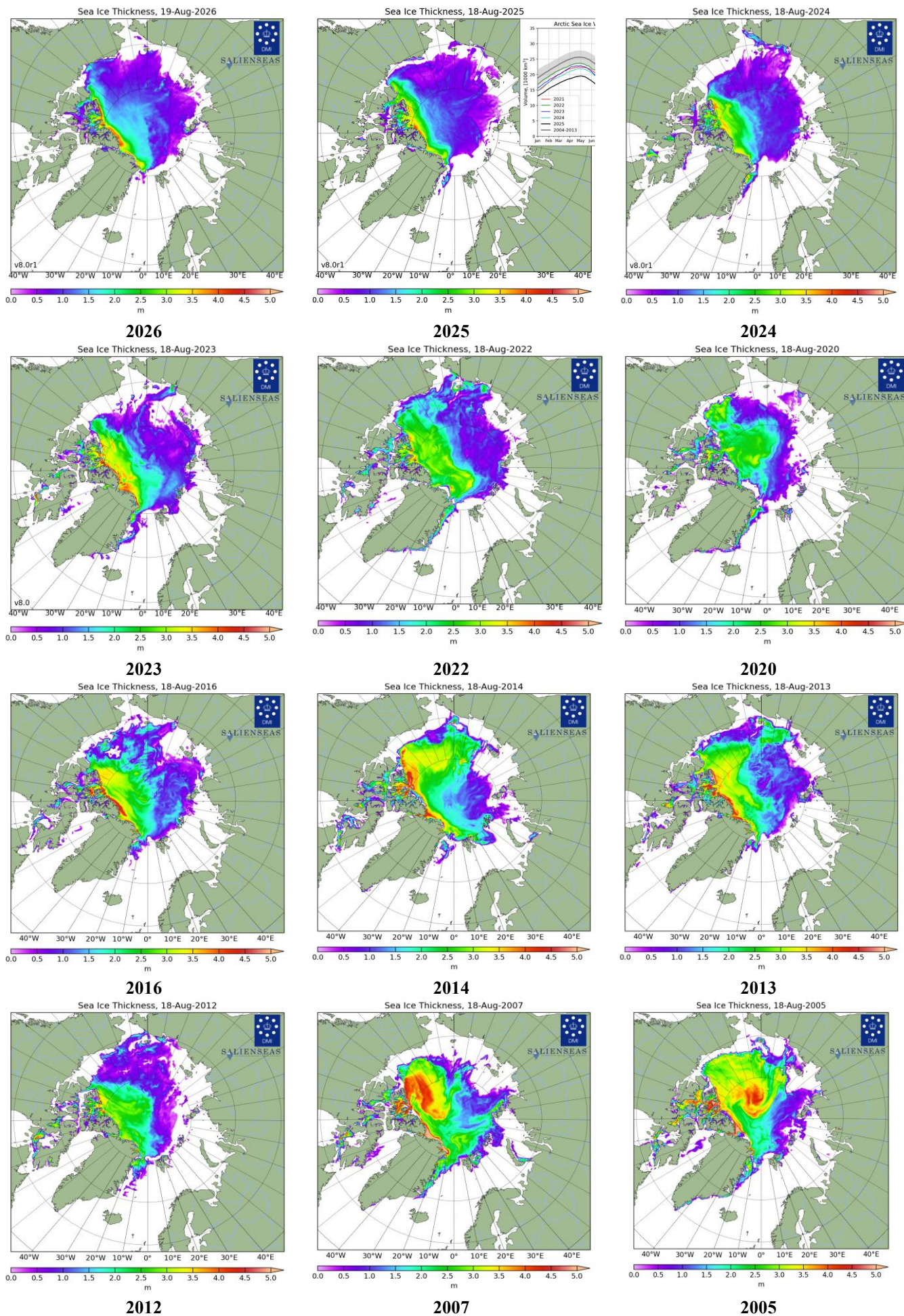
Рисунок 4в – Поля распределения средневзвешенной толщины льда совместной модели морского льда – океана HYCOM/CICE Датского метеорологического института 18-19.08 за 2005-2026 гг. [22].
