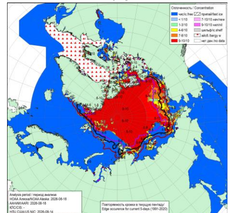
Рисунок 4а – Ледовые условия за 14.08 - 18.08.2026. и аналогичные периоды 2007-2025 гг. на основе ледового анализа ААНИИ, НИЦ Планета, Канадской ледовой службы, Национального ледового центра США и НОАА Аляска [4, 10, 12, 23, 17].
