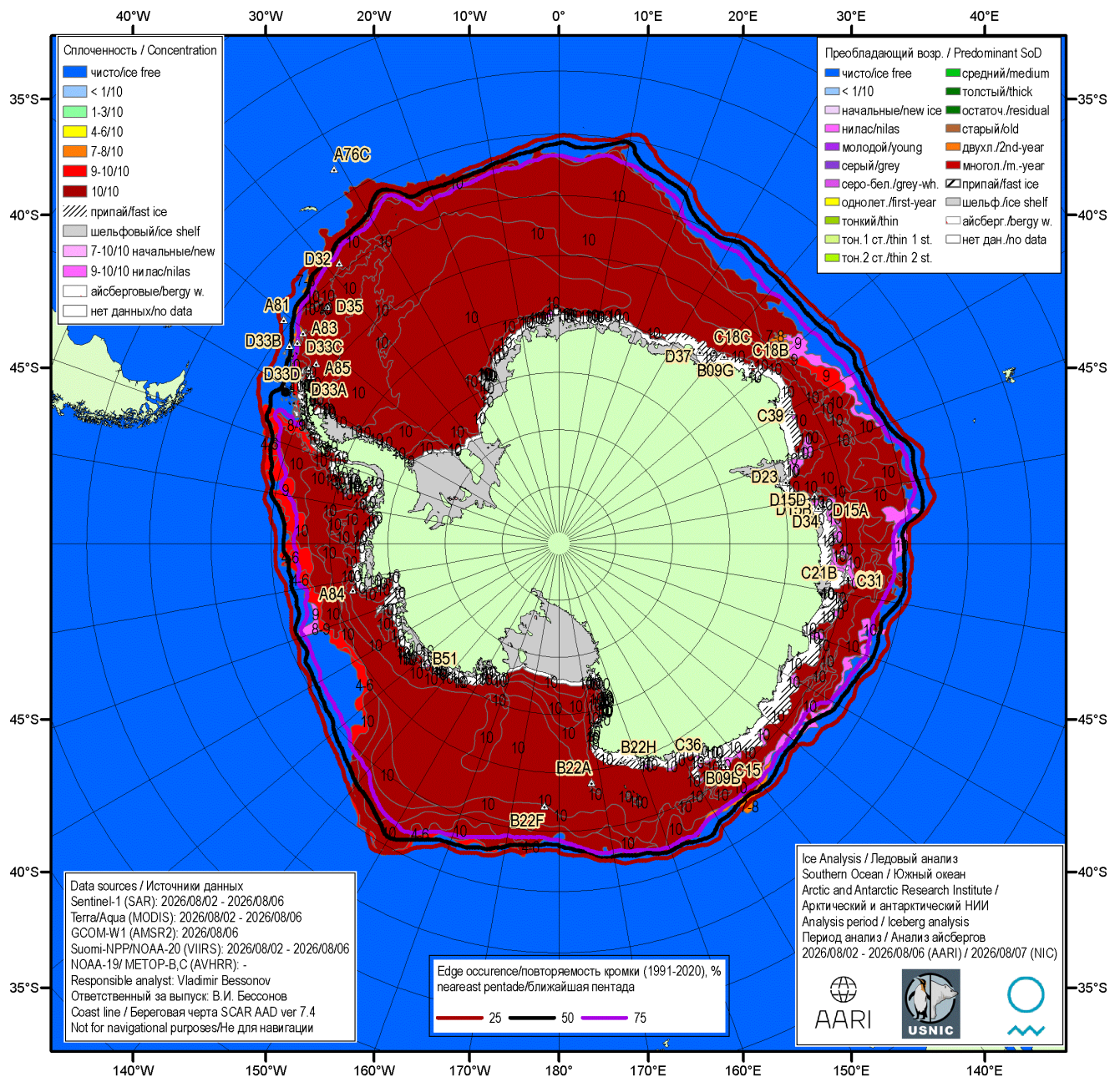
Рисунок 7а – Ледовая карта Южного океана (цветовая окраска по общей сплоченности) и расположение крупных айсбергов на основе ледового анализа за 06.08.2026 в рамках проекта совместного ледового картирования Южного океана ААНИИ, НЛЦ США и НМИ и повторяемость кромки за ближайшую пентаду за период 1991-2020 гг. по наблюдениям SSMR-SSM/I-SSMIS (алгоритм NASATEAM) [5, 10, 17, 21]
