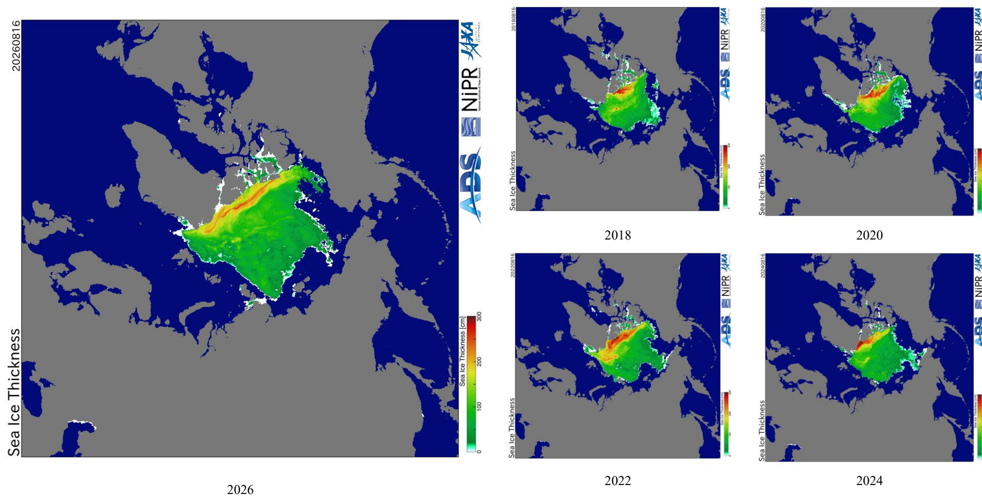
Рисунок 2а - Оценка толщины льда на основе данных пассивного микроволнового зондирования AMSR2 16.08 в 2018 – 2026 гг. [29].
