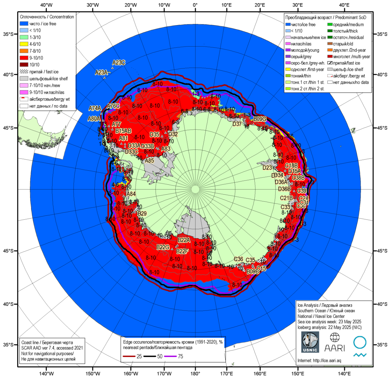
Рисунок 5а – Ледовая карта Южного океана (цветовая окраска по общей сплоченности) и расположение крупных айсбергов на основе ледового анализа за 23.05.2025 в рамках проекта совместного ледового картирования Южного океана ААНИИ, НЛЦ США и НМИ и повторяемость кромки за ближайшую пентаду за период 1991-2020 гг. по наблюдениям SSMR-SSM/I-SSMIS (алгоритм NASATEAM) [5, 10, 17, 21]
