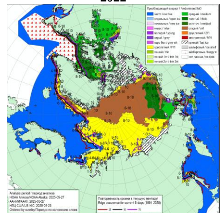
Рисунок 1ж – Ледовые условия за 23.05 - 27.05.2025. и аналогичные периоды 2007-2024 гг. на основе ледового анализа ААНИИ, НИЦ Планета, Канадской ледовой службы, Национального ледового центра США и НОАА Аляска [4, 10, 12, 23, 17]..
