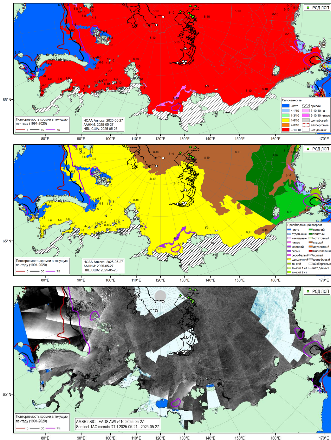
Рисунок 1д – Обзорная ледовая карта СМП за 27.05.2025 г. на основе ледового анализа НОАА Аляска, ААНИИ, мозаика радиолокационных снимком ИСЗ Sentinel-1AC за 21.05-27.05.2025 (DTU), положение крупных полыней по данным AMSR2 за 27.05.2025 (AWI v110), повторяемость кромки за соответствующий 5-дневный период 1991-2020 гг. по наблюдениям SSMR-SSM/I-SSMIS (алгоритм NASATEAM) и положение РСН СП-42 на 08МСК 28.05.2025 [27, 28, 17].
