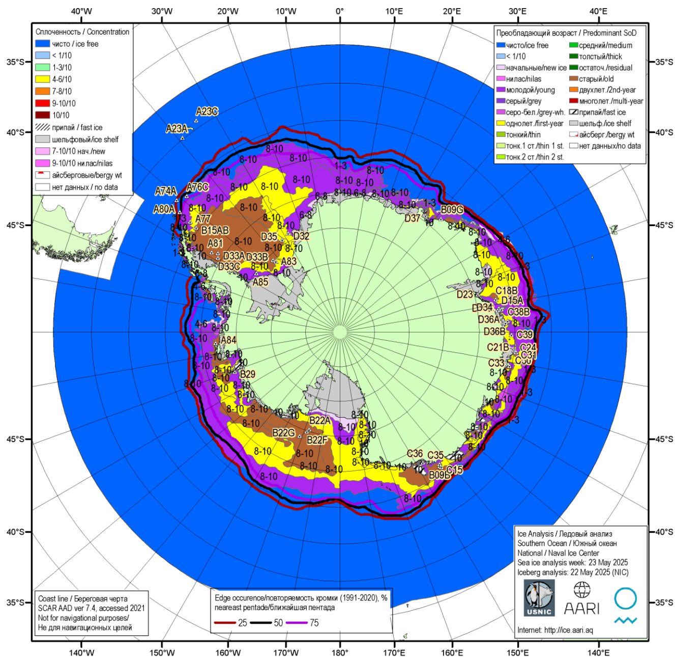
Рисунок 56 – Ледовая карта Южного океана (цветовая окраска по возрасту) и расположение крупных айсбергов на основе ледового анализа за 23.05.2025 в рамках проекта совместного ледового картирования Южного океана ААНИИ, НЛЦ США и НМИ и повторяемость кромки за ближайшую пентаду за период 1991-2020 гг. по наблюдениям SSMR-SSM/I-SSMIS (алгоритм NASATEAM) [5, 10, 17, 21].
