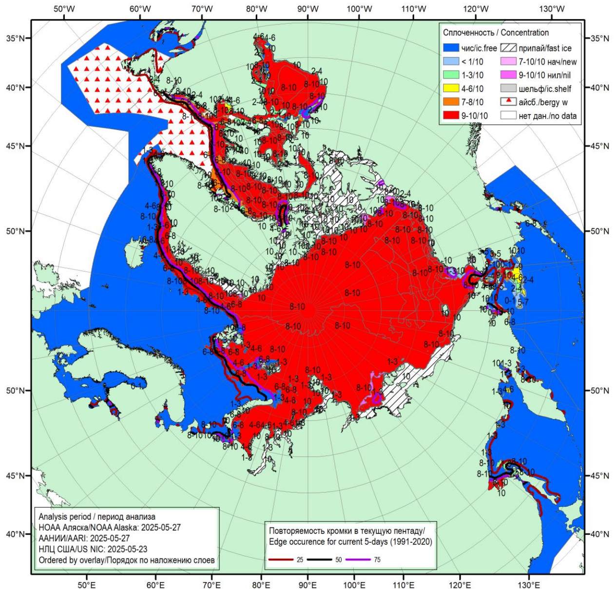
Рисунок 1а – Обзорная ледовая карта СЛО за 23.05.2025 – 27.05.2025 (цветовая раскраска по общей сплоченности) на основе ледового анализа НОАА Аляска, ААНИИ и Национального ледового центра США и повторяемость кромки за соответствующий 5-дневный период за 1991-2020 гг. по наблюдениям SSMR-SSM/I-SSMIS (алгоритм NASATEAM) [4, 10, 23, 17].
