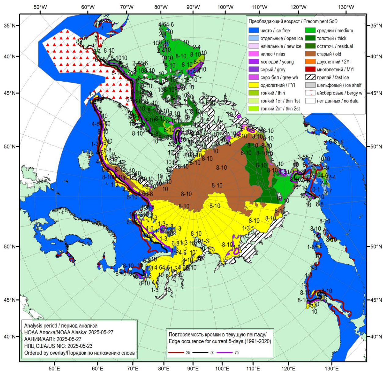
Рисунок 16 – Обзорная ледовая карта СЛО за 23.05.2025 – 27.05.2025 (цветовая раскраска по преобладающему возрасту) на основе ледового анализа NOAA Аляска, ААНИИ и Национального ледового центра США и повторяемость кромки за соответствующий 5-дневный период за 1991-2020 гг. по наблюдениям SSMR-SSM/I-SSMIS (алгоритм NASATEAM) [4, 10, 23, 17].
