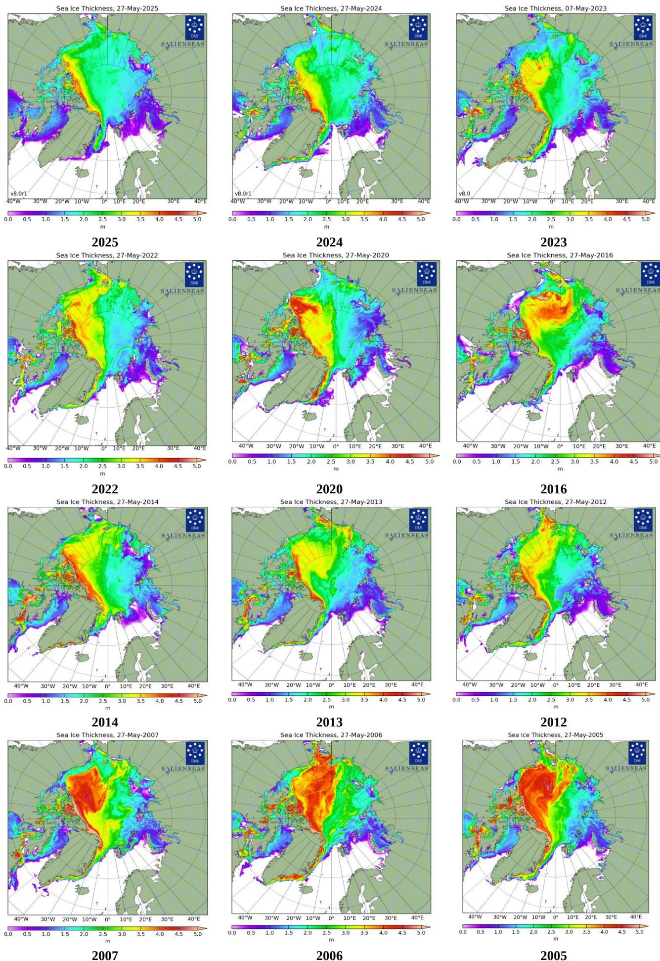
Рисунок 26 – Поля распределения средневзвешенной толщины льда совместной модели морского льда – океана HYCOM/CICE Датского метеорологического института 27.05 за 2005-2025 гг. [22].
