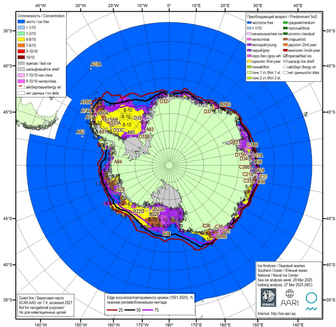
Рисунок 56 – Ледовая карта Южного океана (цветовая окраска по возрасту) и расположение крупных айсбергов на основе ледового анализа за 28.03.2025 в рамках проекта совместного ледового картирования Южного океана ААНИИ, НЛЦ США и НМИ и повторяемость кромки за 26-31.03 за период 1991-2020 гг. по наблюдениям SSMR-SSM/I-SSMIS (алгоритм NASATEAM)
