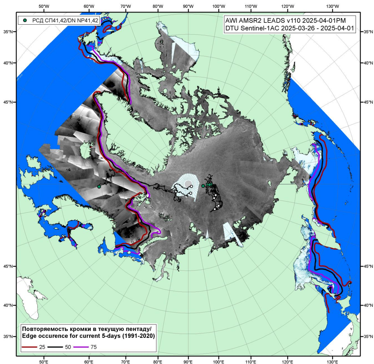
Рисунок 1г – Мозаика радиолокационных снимком ИСЗ Sentinel-1AC за 26.03-01.04.2025 г (DTU), положение разрежений на основе данных ИСЗ AMSR2 2025-04-01PM (AWI, v110), повторяемость кромки за соответствующий 5-дневный промежуток 1991-2020 гг. по наблюдениям SSMR-SSM/I-SSMIS (алгоритм NASATEAM) и положение РСН СП-42 на 02.04.2025 г. 08:00МСК.
