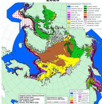
Рисунок 2а – Ледовые условия за 27.03 - 01.04.2025. и аналогичные периоды 2007-2024 гг. на основе ледового анализа ААНИИ, НИЦ Планета, Канадской ледовой службы, Национального ледового центра США и НОАА Аляска.
