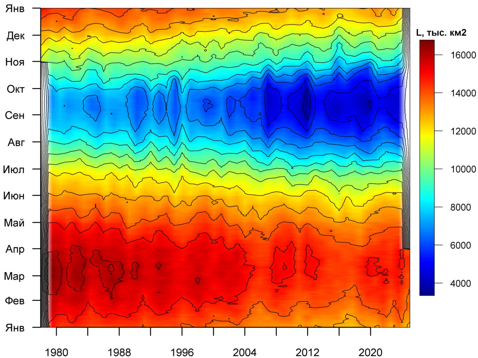
Рисунок 36 – Ежедневные оценки сезонных изменений ледовитости для Северной Полярной Области за период 26.10.1978 – 31.03.2025 на основе расчетов по данным SSMR-SSM/I-SSMIS, алгоритм NASATEAM.
