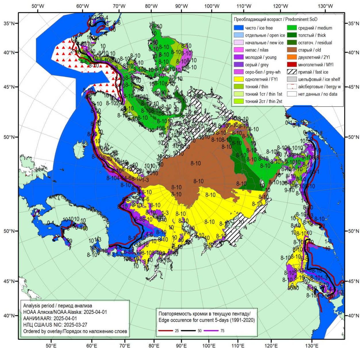
Рисунок 16 – Обзорная ледовая карта СЛО за 27.03.2025 – 01.04.2025 (цветовая раскраска по преобладающему возрасту) на основе ледового анализа NOAA Аляска (01.04.2025), ААНИИ (01.04.2025), Национального ледового центра США (27.03.2025) и повторяемость кромки за 01-05.04 за период 1991-2020 гг. по наблюдениям SSMR-SSM/I-SSMIS (алгоритм NASATEAM).
