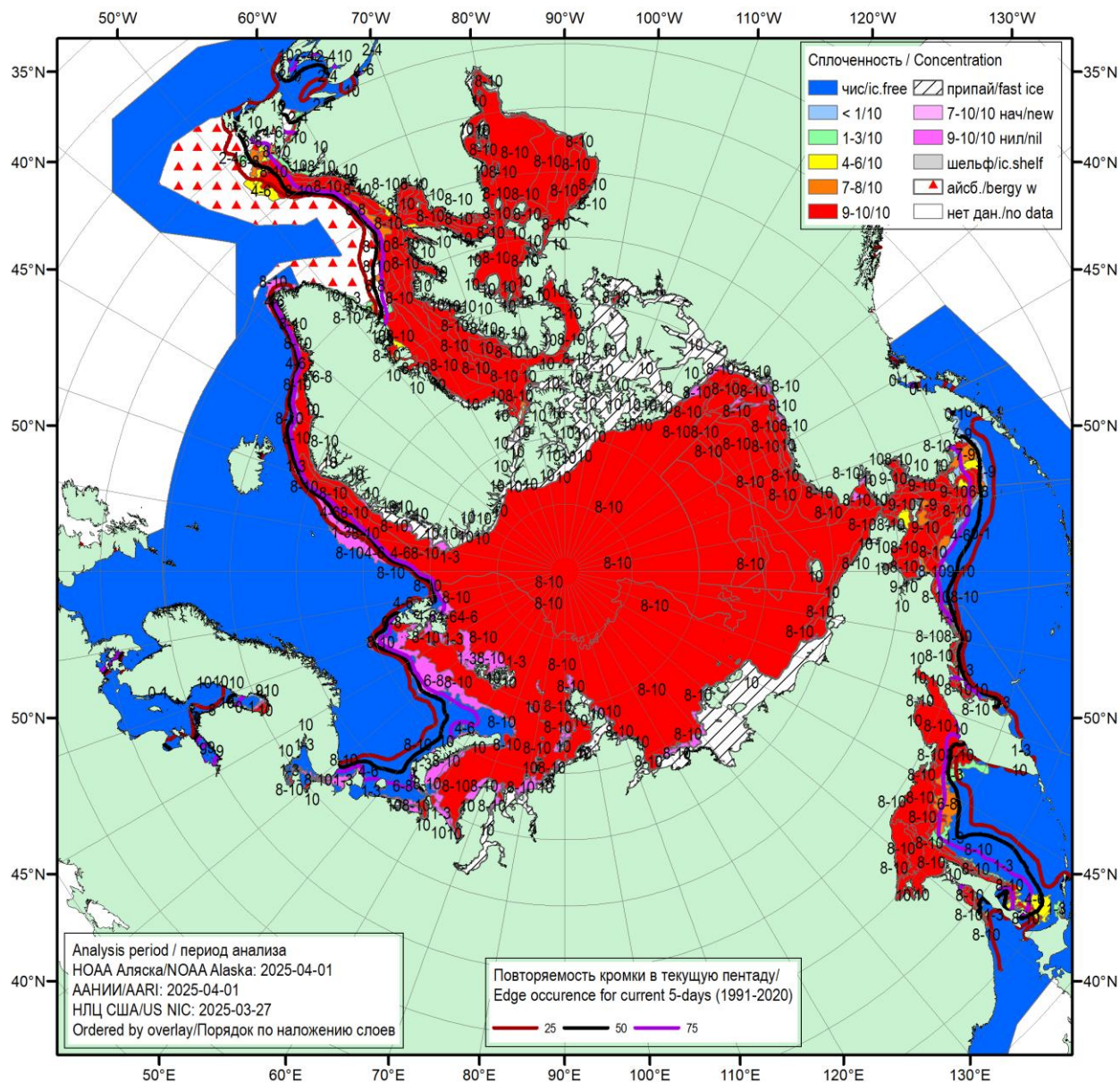
Рисунок 1а – Обзорная ледовая карта СЛО за 27.03.2025 – 01.04.2025 (цветовая раскраска по общей сплоченности) на основе ледового анализа NOAA Аляска (01.04.2025), ААНИИ (01.04.2025), Национального ледового центра США (27.03.2025) и повторяемость кромки за 01-05.04 за период 1991-2020 гг. по наблюдениям SSMR-SSM/I-SSMIS (алгоритм NASATEAM).
