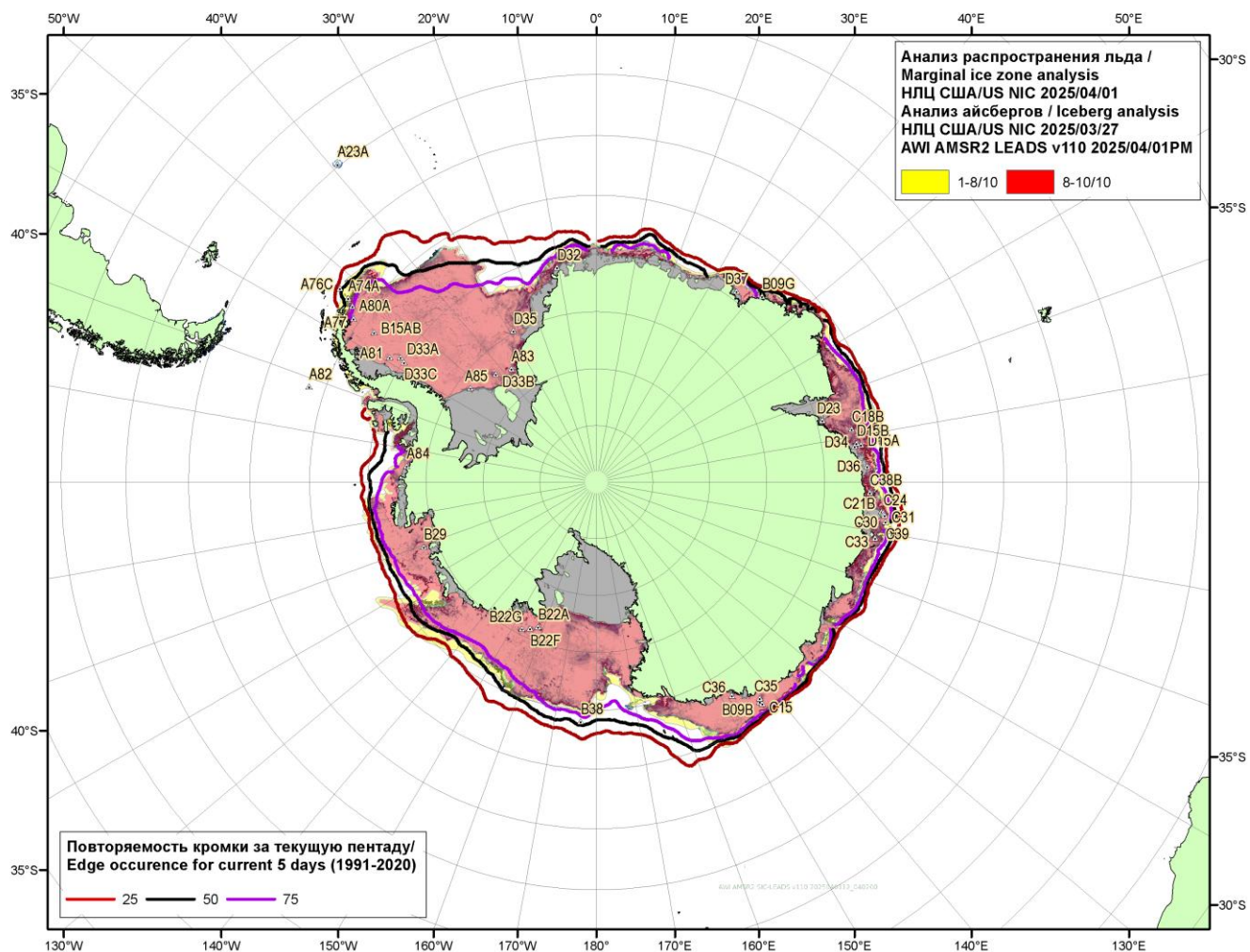
Рисунок 5в – Положение кромки льда и зон разреженных ( <8/10 ) и сплоченных ( \geq 8/10 ) льдов Южного океана за 01.04.2025 г. и расположение крупных айсбергов за 28.03.2025 на основе ледового анализа Национального Ледового Центра США, повторяемость кромки за 26-31.03 за период 1991-2020 гг. по наблюдениям SSMR-SSM/I-SSMIS (алгоритм NASATEAM), совмещенное с положением разрежений на основе данных ИСЗ AMSR2 за 01.04.2025 (AWI, v110).
