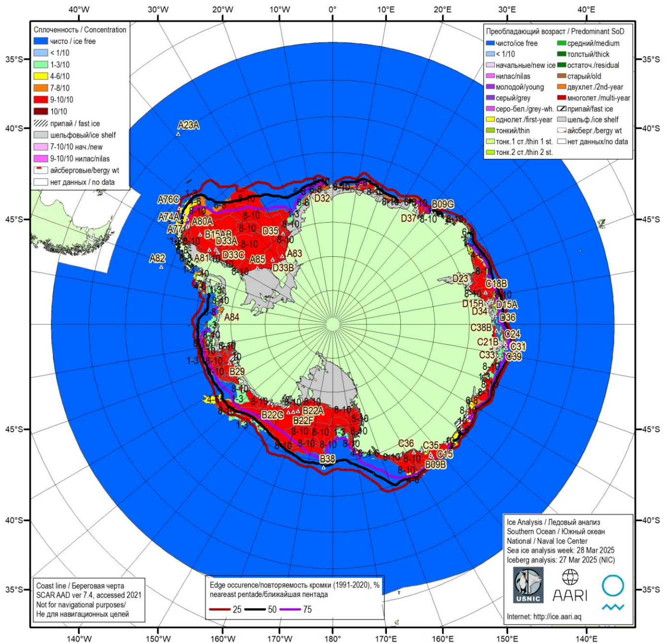
Рисунок 5а – Ледовая карта Южного океана (цветовая окраска по общей сплоченности) и расположение крупных айсбергов на основе ледового анализа за 28.03.2025 в рамках проекта совместного ледового картирования Южного океана ААНИИ, НЛЦ США и НМИ и повторяемость кромки за 26-31.03 за период 1991-2020 гг. по наблюдениям SSMR-SSM/I-SSMIS (алгоритм NASATEAM)
