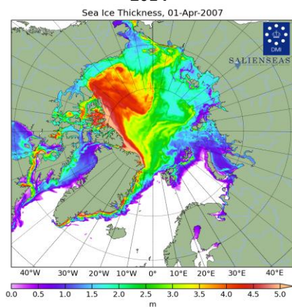
Рисунок 26 – Поля распределения средневзвешенной толщины льда совместной модели морского льда – океана HYCOM/CICE Датского метеорологического института 01.04 за 2005-2025 гг.
