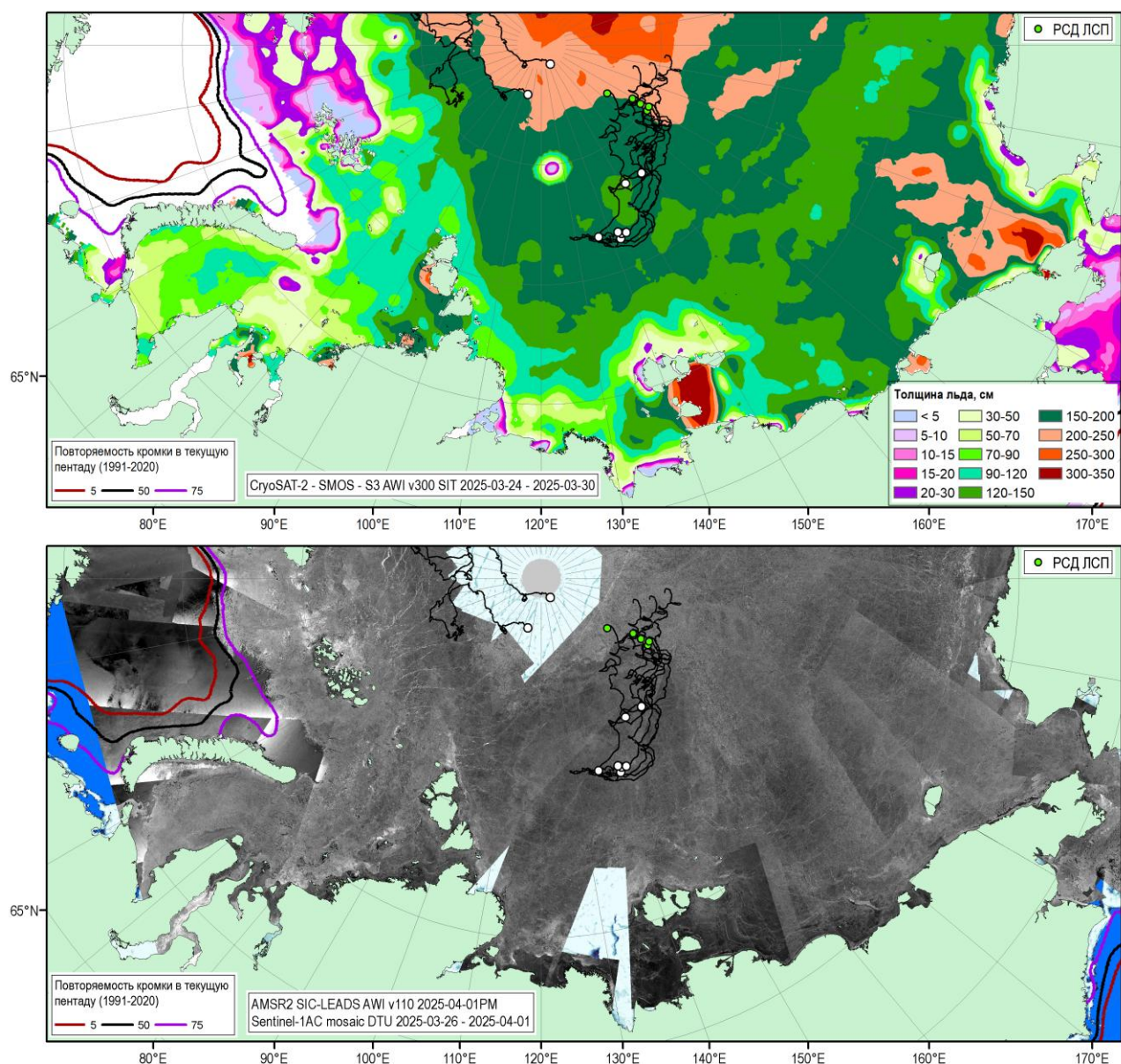
Рисунок 1е - Оценка толщины льда на акватории СМП на основе данных ИСЗ CryoSat-2-SMOS-S3 за 24.03.2025-30.03.2025 (AWI, ver.300), мозаика радиолокационных снимком ИСЗ Sentinel-1AC за 26.03-1.04.2025 (DTU), оценка положения полыней на основе данных AMSR2 (AWI v110) за 01.04.2025, повторяемость кромки за соответствующие 5-дневные промежутки 1991-2020 гг. по наблюдениям SSMR-SSM/I-SSMIS (алгоритм NASATEAM) и положение РСН СП-42 на 07МСК 02.04.2025
