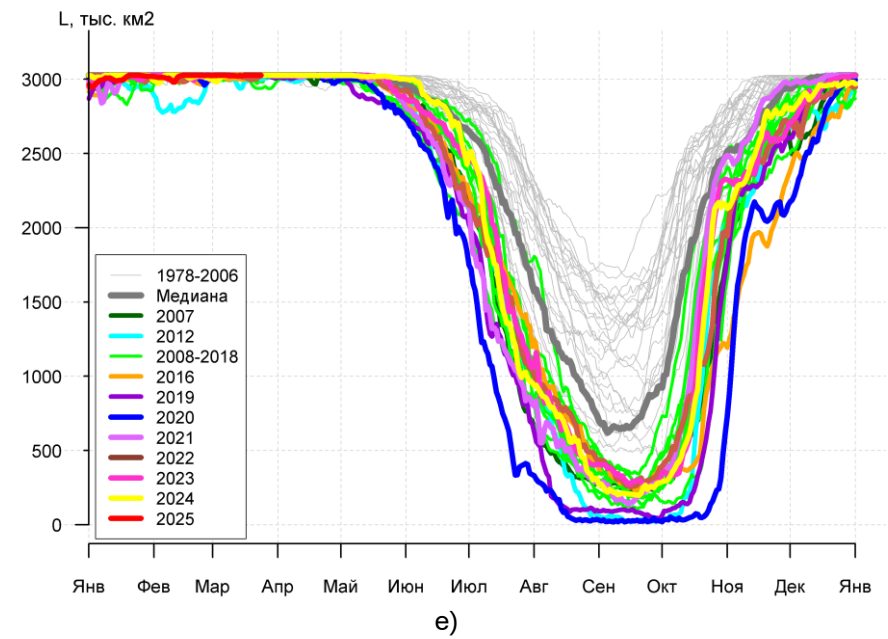
Рисунок 3а – Ежедневные оценки сезонного хода ледовитости для Северной Полярной Области и трех меридиональных секторов, СЛО и морей СМП за период 26.10.1978 – 25.03.2025 по годам на основе расчетов по данным SSMR-SSM/I-SSMIS, алгоритмы NASATEAM: а) Северная полярная область, б) сектор 45°W-95°E (Гренландское – Карское моря), в) сектор 95°E-170°W (моря Лаптевых – Чукотское и Берингово, Охотское), г) сектор 170°W-45°W (море Бофорта и Канадская Арктика), д) Северный Ледовитый океан, е) Северный морской путь (Карское - Чукотское моря).
