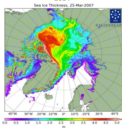
Рисунок 26 – Поля распределения средневзвешенной толщины льда совместной модели морского льда – океана HYCOM/CICE Датского метеорологического института 25.03 за 2005-2025 гг.
