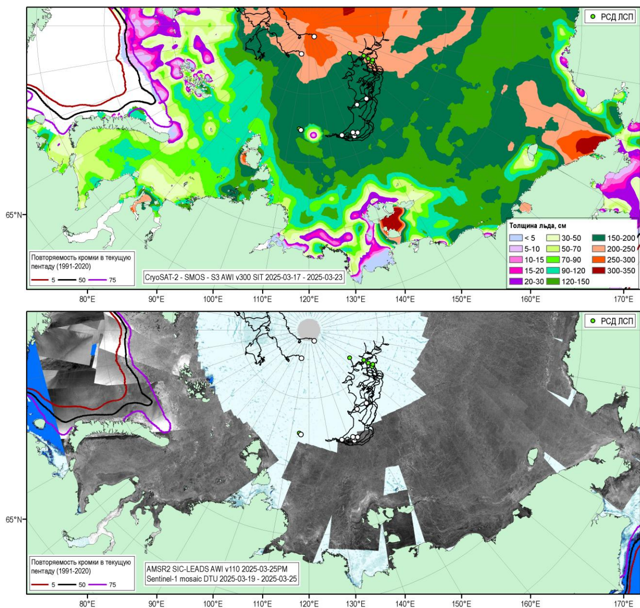
Рисунок 1е - Оценка толщины льда на акватории СМП на основе данных ИСЗ CryoSat-2-SMOS-S3 за 17.03.2025-23.03.2025 (AWI, ver.300), мозаика радиолокационных снимков ИСЗ Sentinel-1A за 19-25.03.2025 (DTU), оценка положения полыней на основе данных AMSR2 (AWI v110) за 25.03.2025, повторяемость кромки за соответствующие 5-дневные промежутки 1991-2020 гг. по наблюдениям SSMR-SSM/I-SSMIS (алгоритм NASATEAM) и положение РСН СП-42 на 07МСК 26.03.2025
