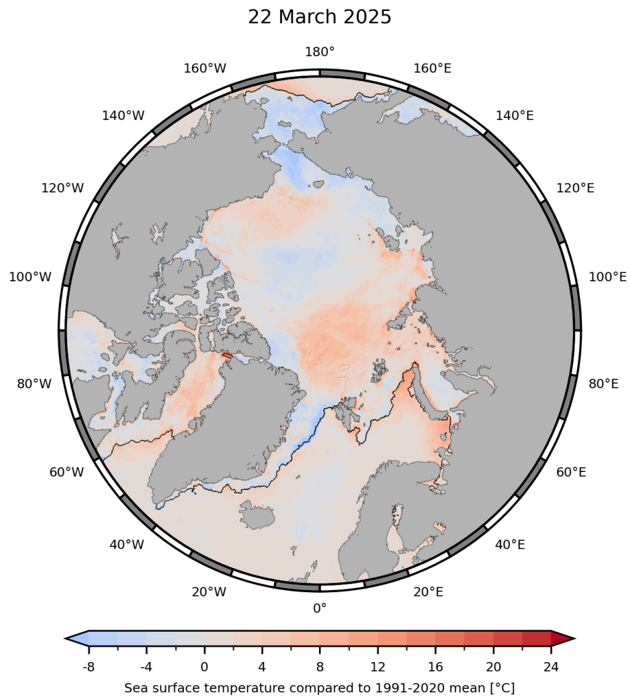
Рисунок 2в – Аномалия температуры поверхности морского льда и океана (к периоду 1991-2020 гг.) Датского метеорологического института за 20-22.03.2025 гг. ( http://polarportal.dk/en/sea-ice-and-icebergs/sea-ice-temperature/#c8099 )
