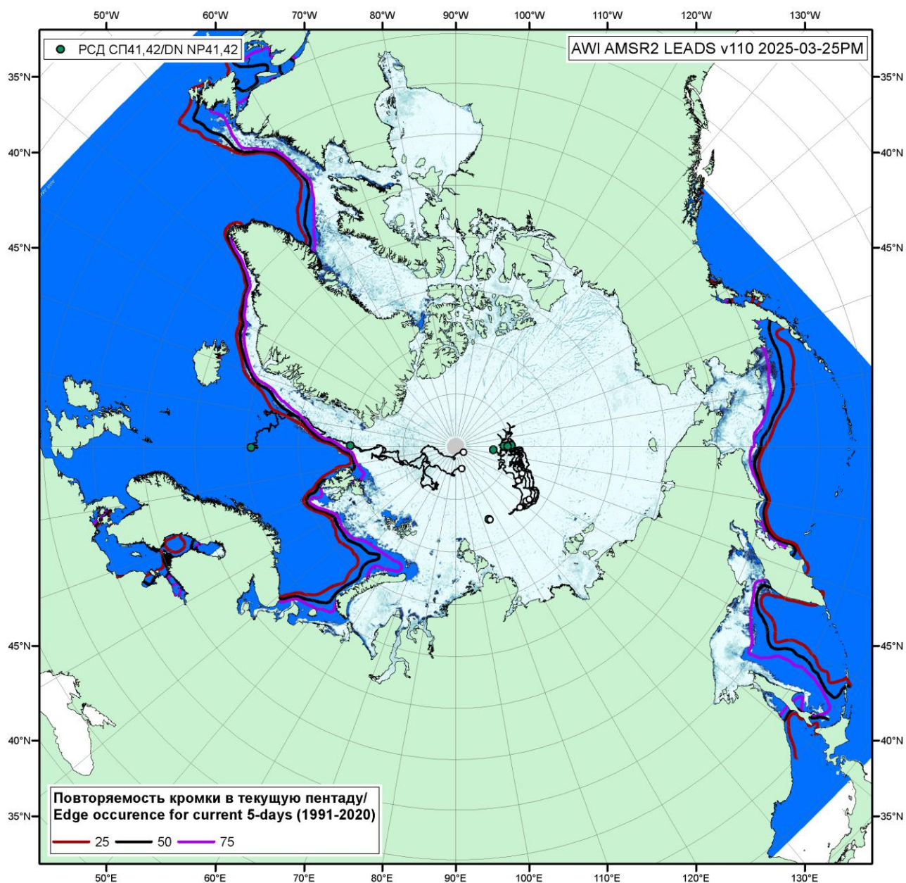
Рисунок 1г – Положение разрежений на основе данных ИСЗ AMSR2 2025-03-25PM (AWI, v110), повторяемость кромки за соответствующий 5-дневный промежуток 1991-2020 гг. по наблюдениям SSMR-SSM/I-SSMIS (алгоритм NASATEAM) и положение РЧН СП-42 на 26.03.2025 г. 08:00МСК.
