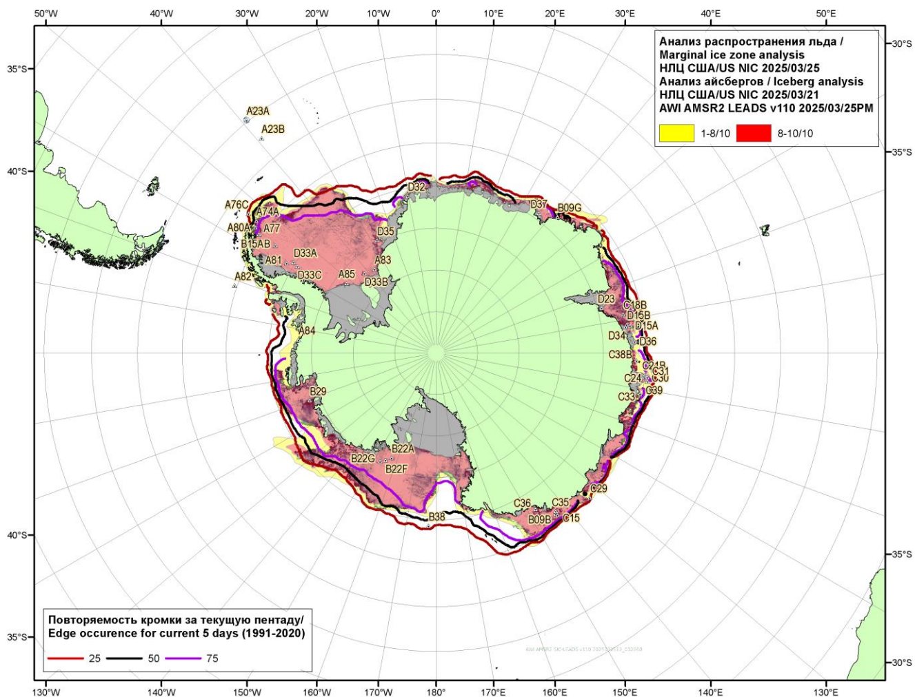
Рисунок 5в – Положение кромки льда и зон разреженных ( <8/10 ) и сплоченных ( \geq 8/10 ) льдов Южного океана за 25.03.2025 г. и расположение крупных айсбергов за 21.03.2025 на основе ледового анализа Национального Ледового Центра США, повторяемость кромки за 21-25.03 за период 1991-2020 гг. по наблюдениям SSMR-SSM/I-SSMIS (алгоритм NASATEAM), совмещенное с положением разрежений на основе данных ИСЗ AMSR2 за 25.03.2025 (AWI, v110).
