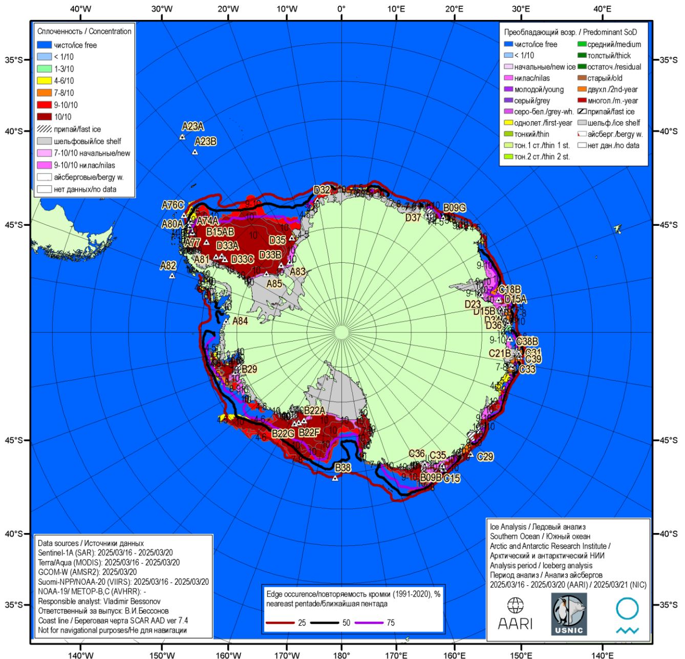
Рисунок 5а – Ледовая карта Южного океана (цветовая окраска по общей сплоченности) и расположение крупных айсбергов на основе ледового анализа за 20.03.2025 в рамках проекта совместного ледового картирования Южного океана ААНИИ, НЛЦ США и НМИ и повторяемость кромки за 16-20.03 за период 1991-2020 гг. по наблюдениям SSMR-SSM/I-SSMIS (алгоритм NASATEAM)
