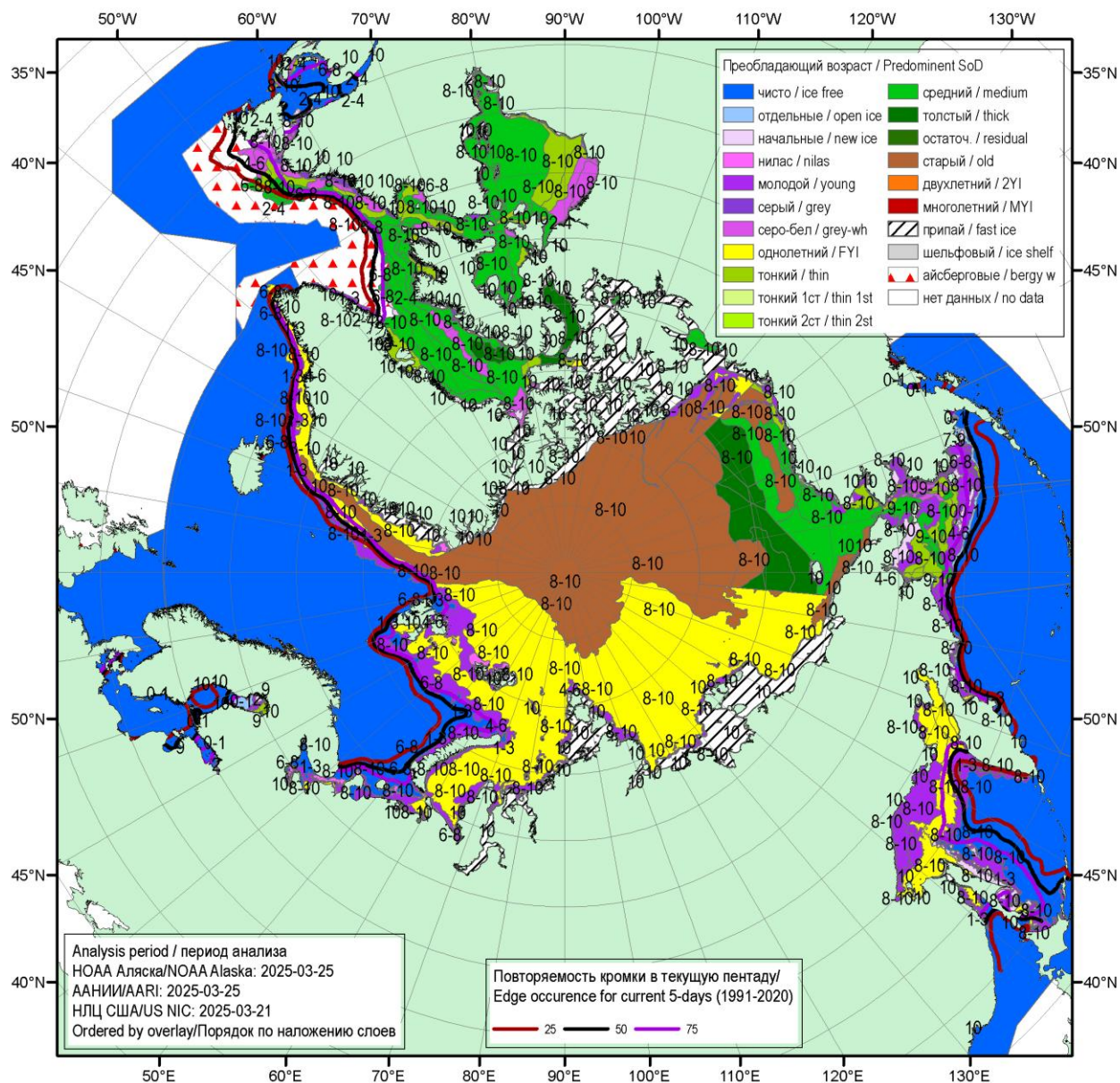
Рисунок 16 – Обзорная ледовая карта СЛО за 21.03.2025 – 25.03.2025 (цветовая раскраска по преобладающему возрасту) на основе ледового анализа НОАА Аляска (25.03.2025), ААНИИ (25.03.2025), Национального ледового центра США (21.03.2025) и повторяемость кромки за 21-25.03 за период 1991-2020 гг. по наблюдениям SSMR-SSM/I-SSMIS (алгоритм NASATEAM).
