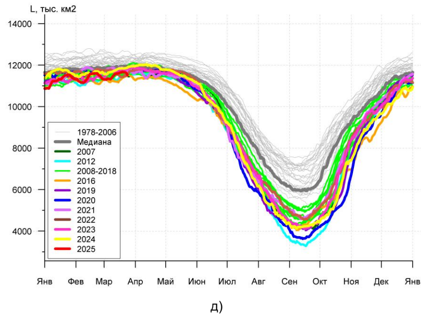
Рисунок 3а – Ежедневные оценки сезонного хода ледовитости для Северной Полярной Области и трех меридиональных секторов, СЛО и морей СМП за период 26.10.1978 – 25.03.2025 по годам на основе расчетов по данным SSMR-SSM/I-SSMIS, алгоритмы NASATEAM: а) Северная полярная область, б) сектор 45°W-95°E (Гренландское – Карское моря), в) сектор 95°E-170°W (моря Лаптевых – Чукотское и Берингово, Охотское), г) сектор 170°W-45°W (море Бофорта и Канадская Арктика), д) Северный Ледовитый океан, е) Северный морской путь (Карское - Чукотское моря).
