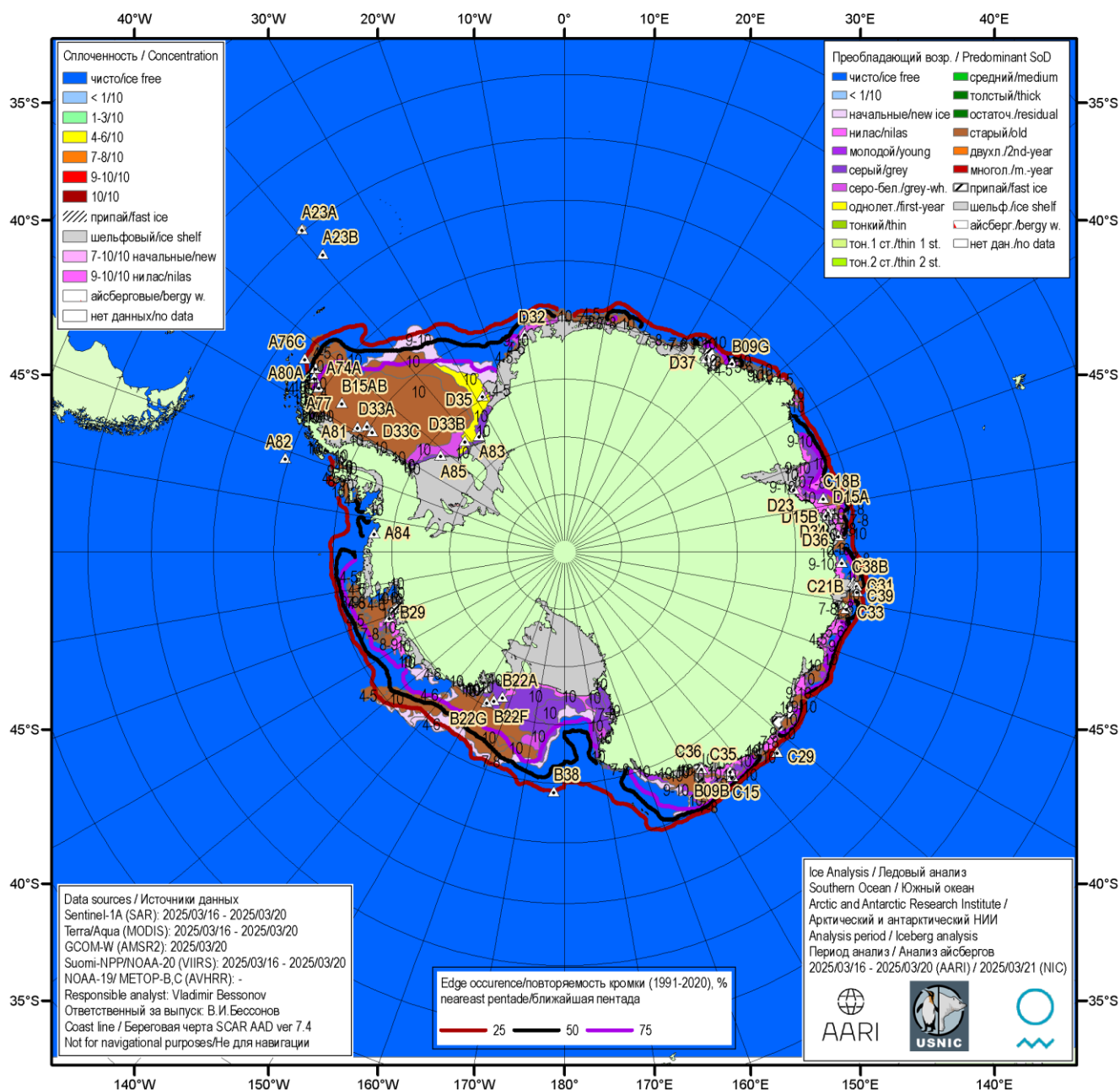
Рисунок 56 – Ледовая карта Южного океана (цветовая окраска по возрасту) и расположение крупных айсбергов на основе ледового анализа за 20.03.2025 в рамках проекта совместного ледового картирования Южного океана ААНИИ, НЛЦ США и НМИ и повторяемость кромки за 16-20.03 за период 1991-2020 гг. по наблюдениям SSMR-SSM/I-SSMIS (алгоритм NASATEAM)
