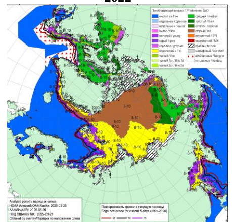
Рисунок 2а – Ледовые условия за 21.03 - 25.03.2025. и аналогичные периоды 2007-2024 гг. на основе ледового анализа ААНИИ, НИЦ Планета, Канадской ледовой службы, Национального ледового центра США и НОАА Аляска.
