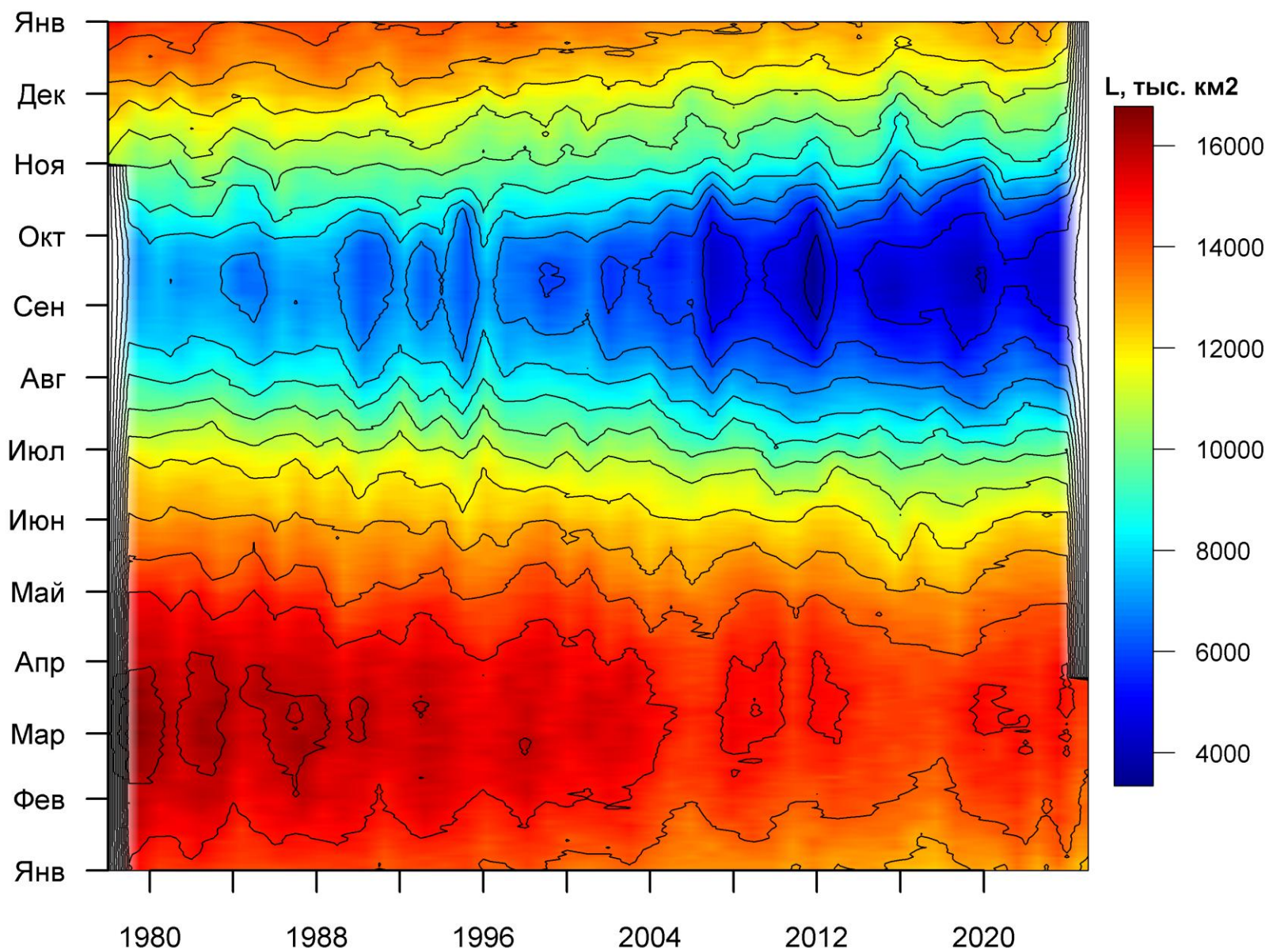
Рисунок 36 – Ежедневные оценки сезонных изменений ледовитости для Северной Полярной Области за период 26.10.1978 – 25.03.2025 на основе расчетов по данным SSMR-SSM/I-SSMIS, алгоритм NASATEAM.
