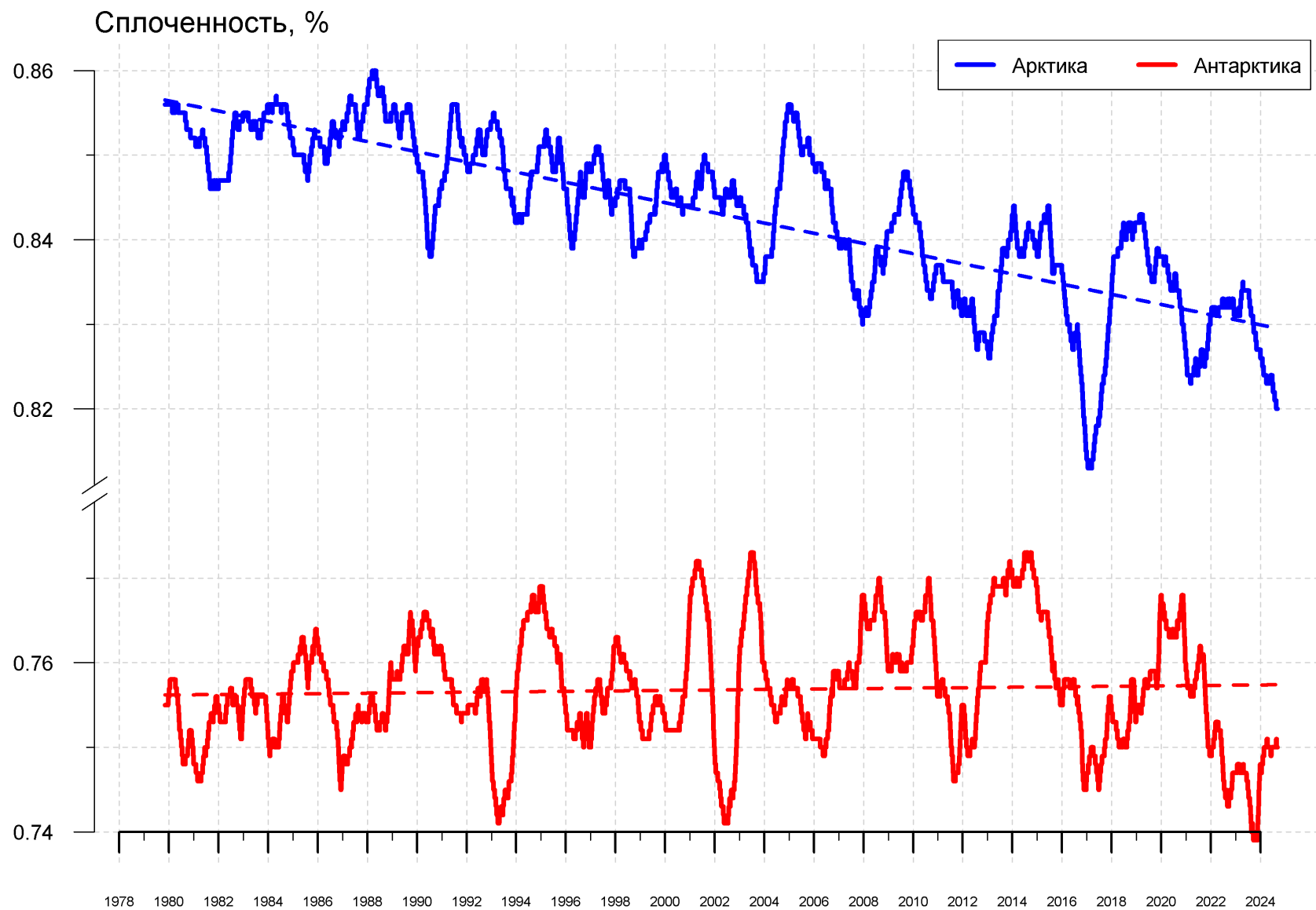
Рисунок 11 – Ежедневные сглаженные окном 365 суток значения средней общей сплоченности Арктики и Антарктики с 07.11.1978 по 09.09.2024 на основе SSMR-SSM/I-SSMIS
