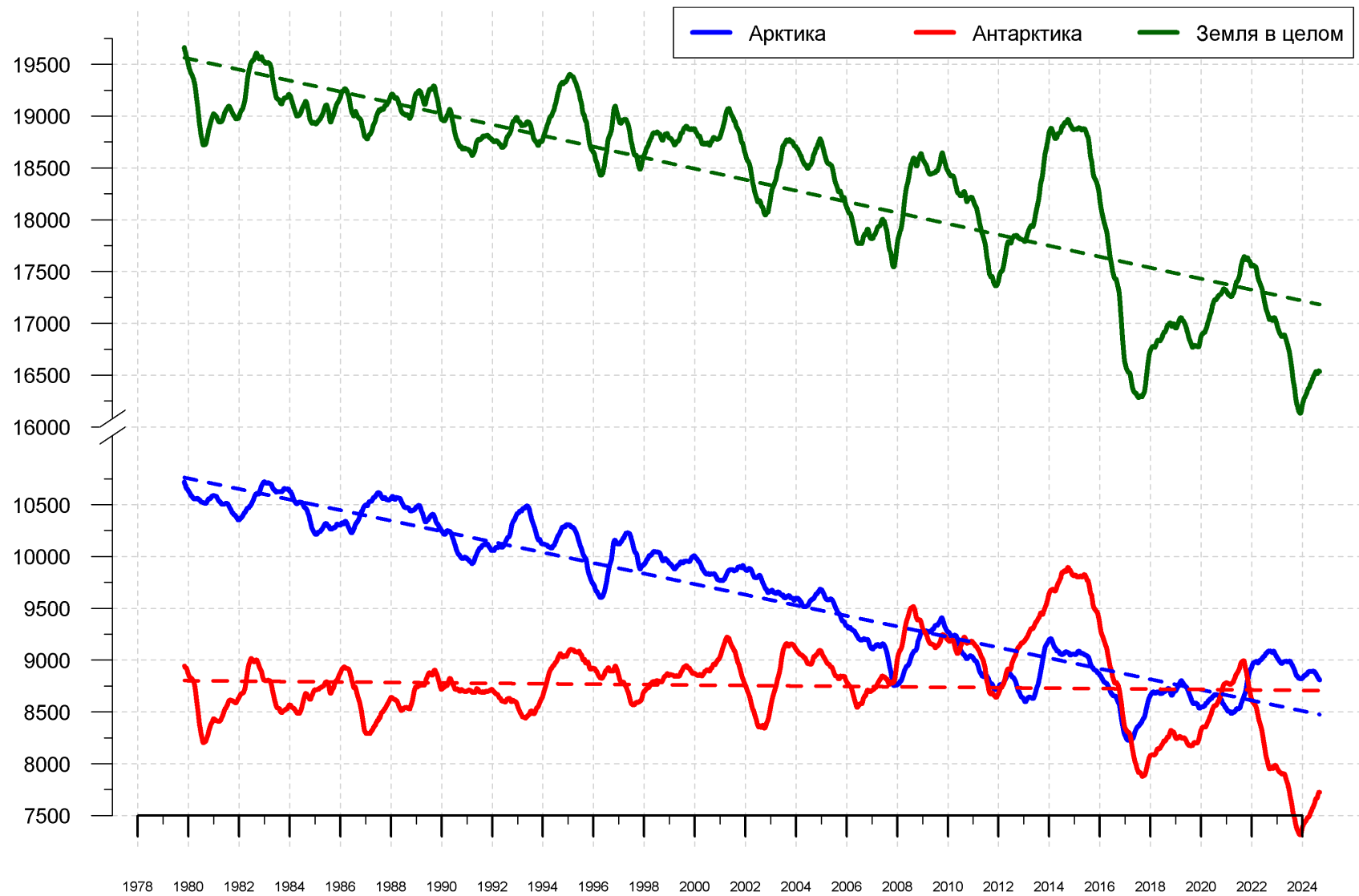
Рисунок 10 – Ежедневные сглаженные окном 365 суток значения приведенной ледовитости (площади морского льда) Арктики, Антарктики и Земли в целом с 25.10.1978 по 09.09.2024 на основе SSMR-SSM/I-SSMIS
