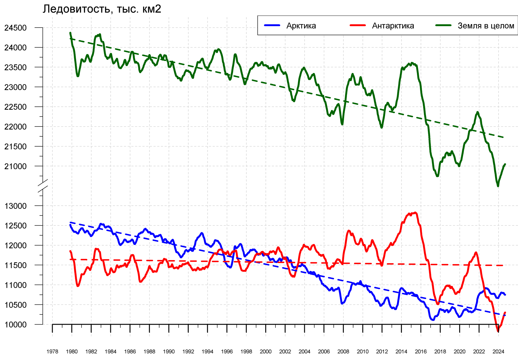
Рисунок 9 – Ежедневные сглаженные окном 365 суток значения ледовитости (площади распространения морского льда) Арктики, Антарктики и Земли в целом с 26.10.1978 по 09.09.2024 на основе SSMR-SSM/I-SSMIS
