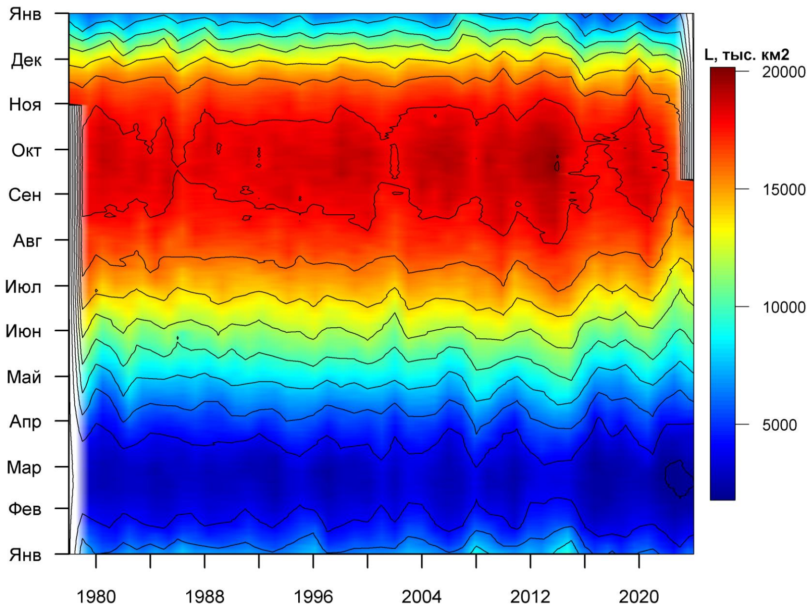
Рисунок 76 – Ежедневные оценки сезонных изменений ледовитости для Южного океана за период 26.10.1978 - 09.09.2024 на основе расчетов по данным SSMR-SSM/I-SSMIS, алгоритм NASATEAM.
