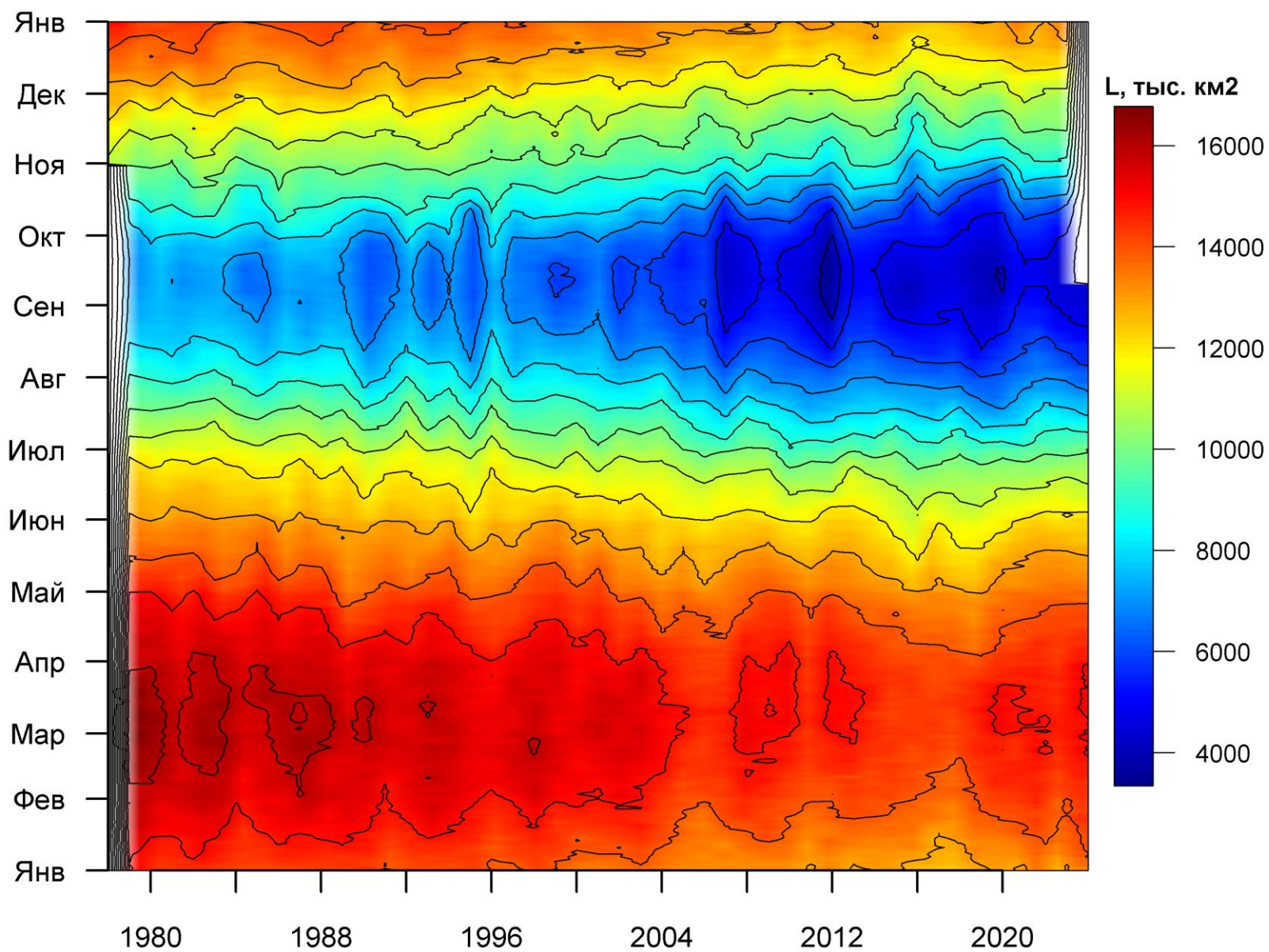
Рисунок 36 – Ежедневные оценки сезонных изменений ледовитости для Северной Полярной Области за период 26.10.1978 – 09.09.2024 на основе расчетов по данным SSMR-SSM/I-SSMIS, алгоритм NASATEAM.
