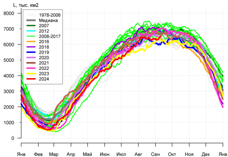
Рисунок 7а – Ежедневные оценки сезонного хода ледовитости Южного Океана и меридиональных секторов за период 26.10.1978 – 09.09.2024 по годам на основе расчетов по данным SSMR-SSM/I-SSMIS, алгоритм NASATEAM: а) Южный Океан, б) Атлантический сектор (60°W-30°E, море Уэдделла), в) Индоокеанский сектор (30°E-150°E, моря Космонавтов, Содружества, Моусона), г) Тихоокеанский сектор (150°E-60°W, моря Росса, Беллинсгаузена)
