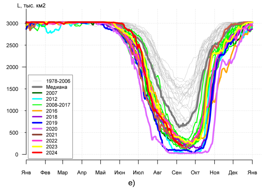
Рисунок 3а – Ежедневные оценки сезонного хода ледовитости для Северной Полярной Области и трех меридиональных секторов за период 26.10.1978 – 09.09.2024 по годам на основе расчетов по данным SSMR-SSM/I-SSMIS, алгоритмы NASATEAM: а) Северная полярная область, б) сектор 45°W-95°E (Гренландское – Карское моря), в) сектор 95°E-170°W (моря Лаптевых – Чукотское и Берингово, Охотское), г) сектор 170°W-45°W (море Бофорта и Канадская Арктика), д) Северный Ледовитый океан, е) Северный морской путь (Карское - Чукотское моря).
