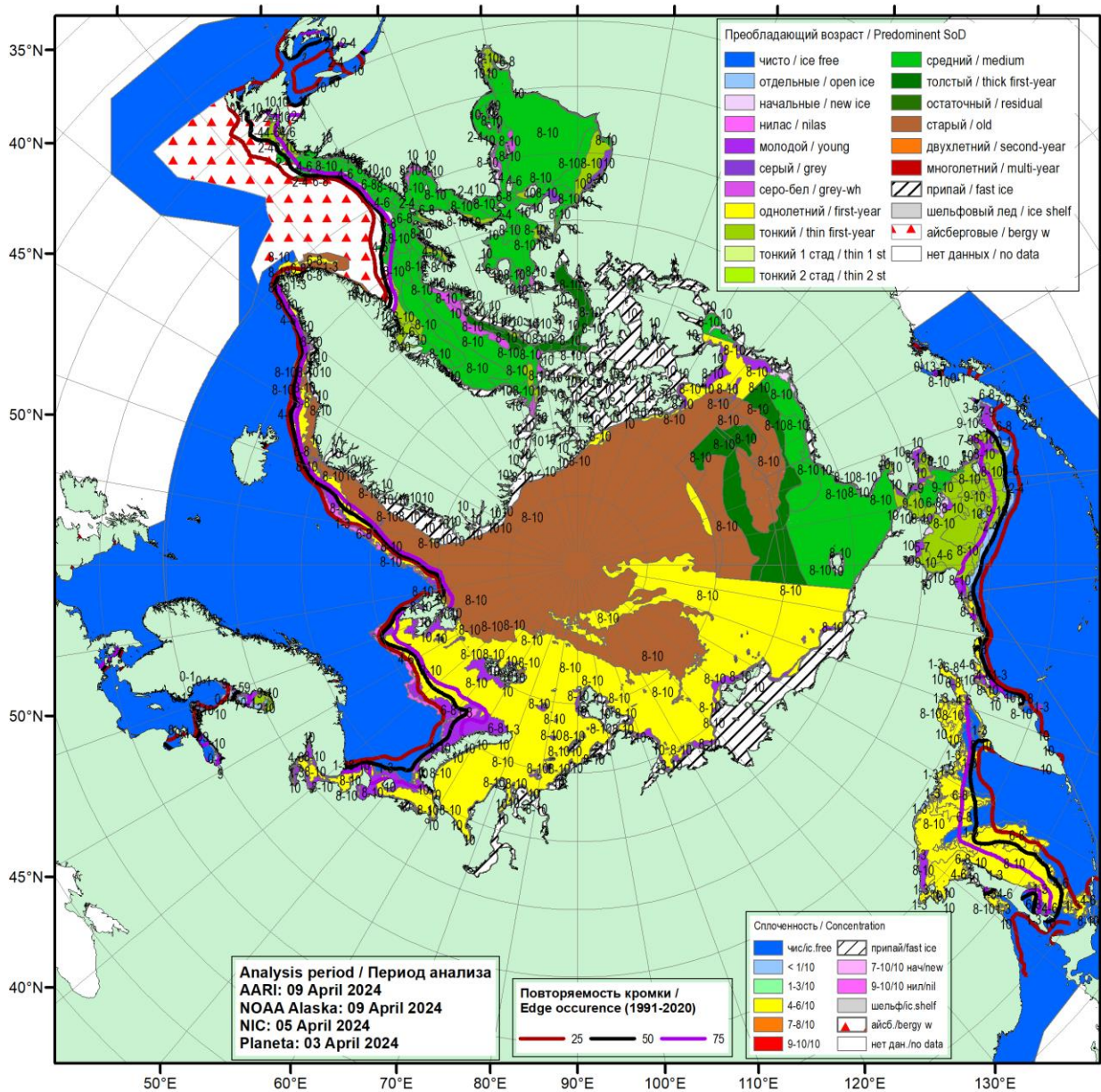
Рисунок 16 – Обзорная ледовая карта СЛО за 03.04 - 09.04.2024 г. (цветовая раскраска по преобладающему возрасту) на основе ледового анализа ААНИИ (09.04), НОАА Аляска (09.04), НИЦ Планета (03.04), Национального ледового центра США (05.04) и повторяемость кромки за 06-10.04 за период 1991-2020гг. по наблюдениям SSMR-SSM/I-SSMIS (алгоритм NASATEAM).
