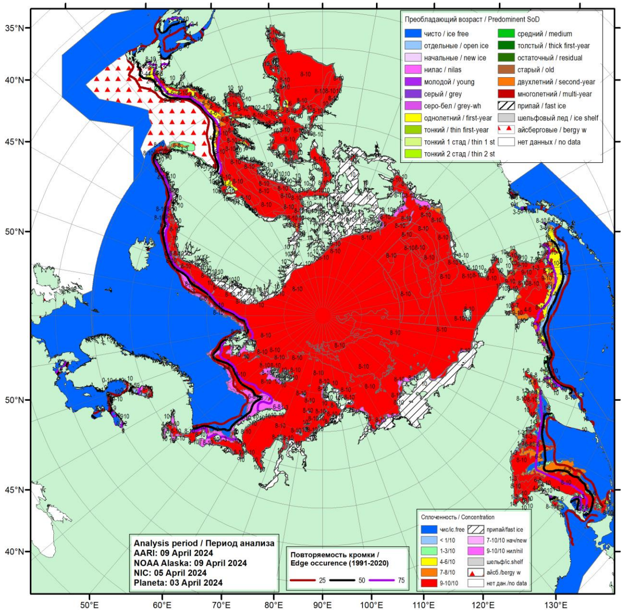
Рисунок 16 – Обзорная ледовая карта СЛО за 03.04 - 09.04.2024 г. (цветовая раскраска по общей сплоченности) на основе ледового анализа ААНИИ (09.04), NOAA Аляска (09.04), НИЦ Планета (03.04), Национального ледового центра США (05.04) и повторяемость кромки за 06-10.04 за период 1991-2020гг. по наблюдениям SSMR-SSM/I-SSMIS (алгоритм NASATEAM).
