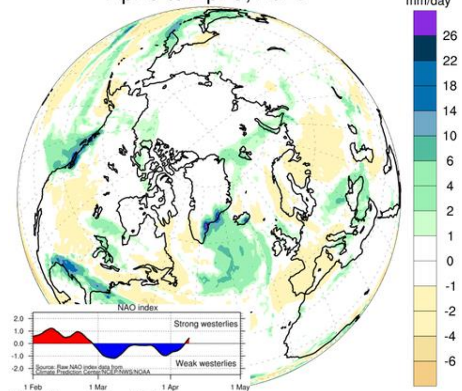
Рисунок 2ж – Аномалии приземной суммы осадков 05.04 – 09.04 в 2023-2024 гг. относительно периода 2004-2013 гг. ( http://polarportal.dk )
