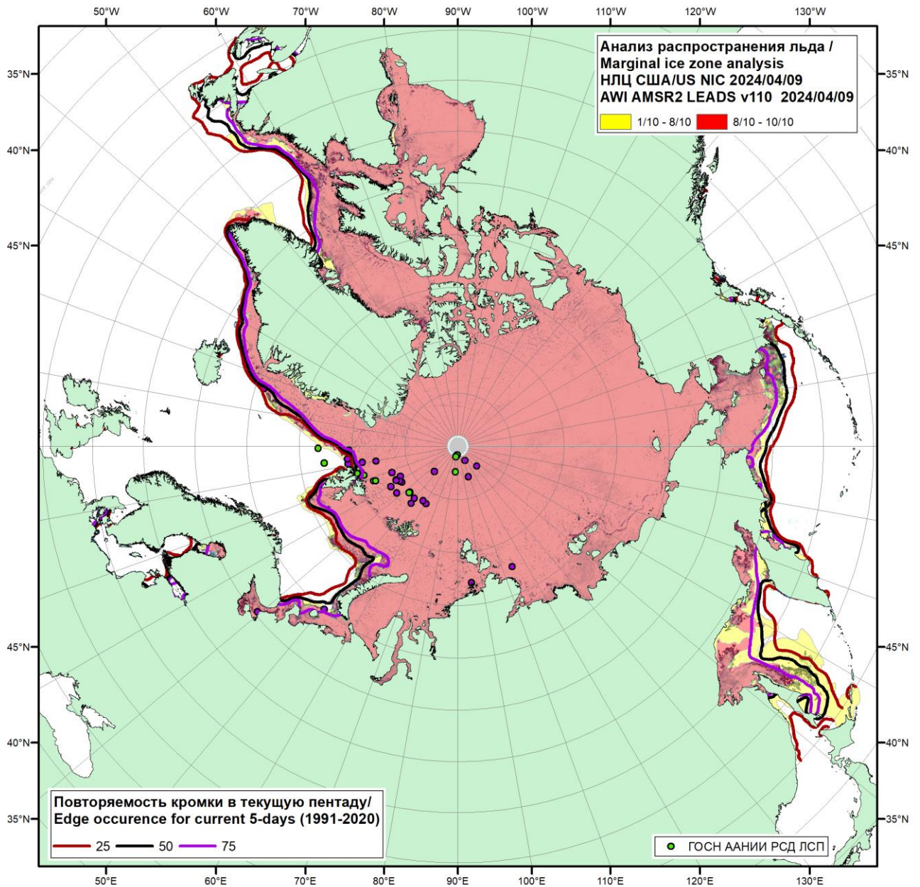
Рисунок 1г – Положение кромки льда и зон разреженных ( <8/10 ) и сплоченных ( \geq 8/10 ) льдов СЛО за 09.04.2024 г. на основе ледового анализа Национального Ледового Центра США и повторяемость кромки за 06-10.04 за период 1991-2020 гг. по наблюдениям SSMR-SSM/I-SSMIS (алгоритм NASATEAM), совмещенное с положением разрежений на основе данных ИСЗ AMSR2 09.04.2024 (AWI, v110) и положение РСД ЛСП на 11.04.2024.
