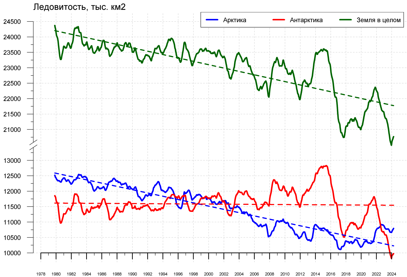
Рисунок 9 – Ежедневные сглаженные окном 365 суток значения ледовитости (площади распространения морского льда) Арктики, Антарктики и Земли в целом с 26.10.1978 по 07.04.2024 на основе SSMR-SSM/I-SSMIS
