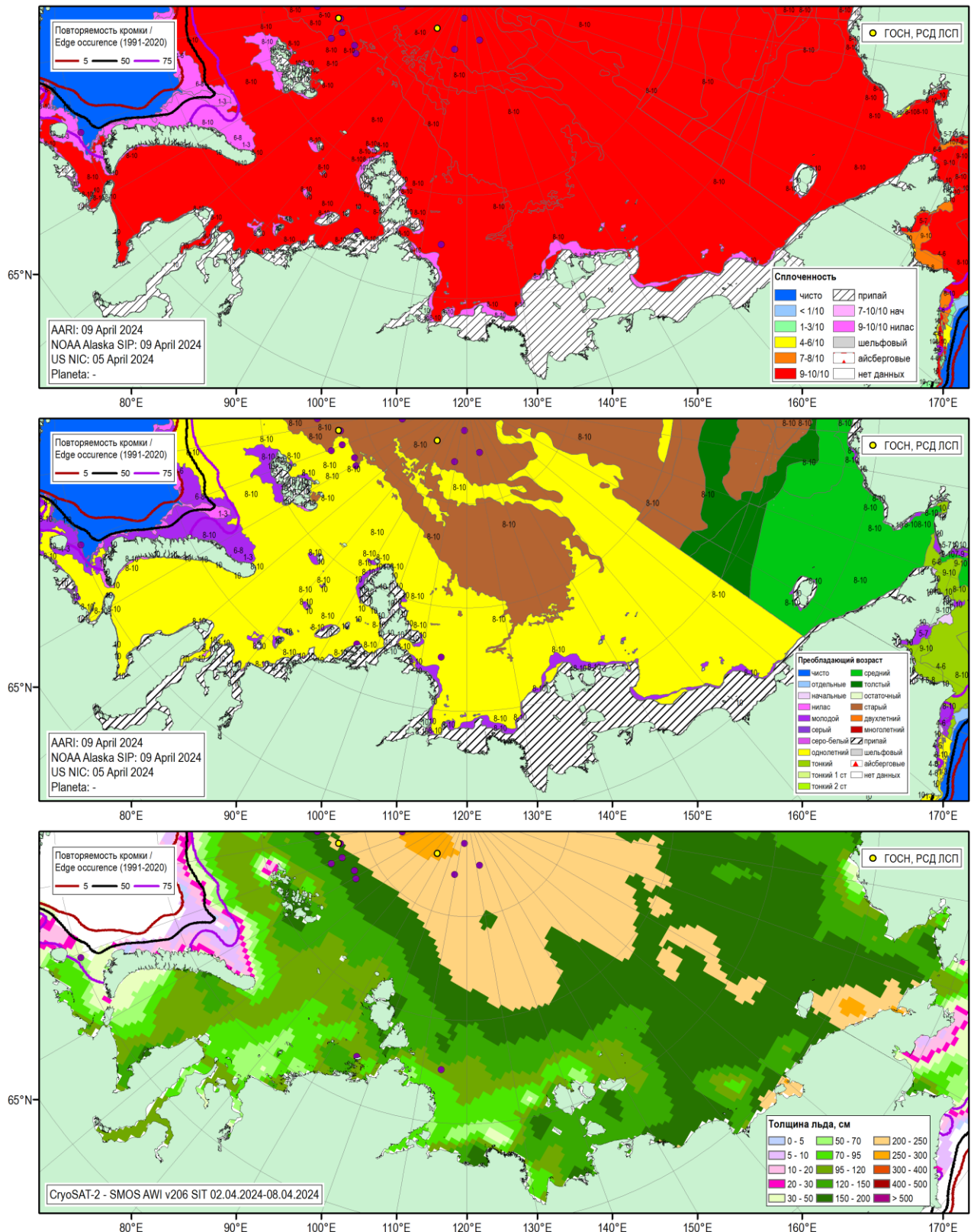
Рисунок 1д – Обзорная ледовая карта СМП за 03.04 - 09.04.2024 г. (цветовая раскраска по общей сплоченности – верх, по преобладающему возрасту - низ) на основе ледового анализа ААНИИ (09.04), NOAA Аляска (09.04), НИЦ Планета (-.-), Национального ледового центра США (05.04) оценка толщин льда по данным CryoSAT-2-SMOS AWI v206 за 02.04-08.04.2024 и повторяемость кромки за 06-10.04 за период 1991-2020гг. по наблюдениям SSMR-SSM/I-SSMIS (алгоритм NASATEAM), положение РСД ЛСП на 11.04.2024.
