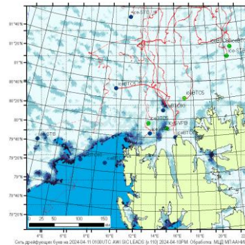
Сеть дрейфующих буев на 2024-04-11 0100UTC AWI SIC LEADS (v.110) 2024-04-10PM Обработка: МЦД МП ААНИИ
