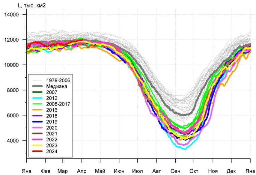
Рисунок 3а – Ежедневные оценки сезонного хода ледовитости для Северной Полярной Области и трех меридиональных секторов за период 26.10.1978 – 31.03.2024 по годам на основе расчетов по данным SSMR-SSM/I-SSMIS, алгоритмы NASATEAM: а) Северная полярная область, б) сектор 45°W-95°E (Гренландское – Карское моря), в) сектор 95°E-170°W (моря Лаптевых – Чукотское и Берингово, Охотское), г) сектор 170°W-45°W (море Бофорта и Канадская Арктика), д) Северный Ледовитый океан, е) Северный морской путь (Карское - Чукотское моря).
