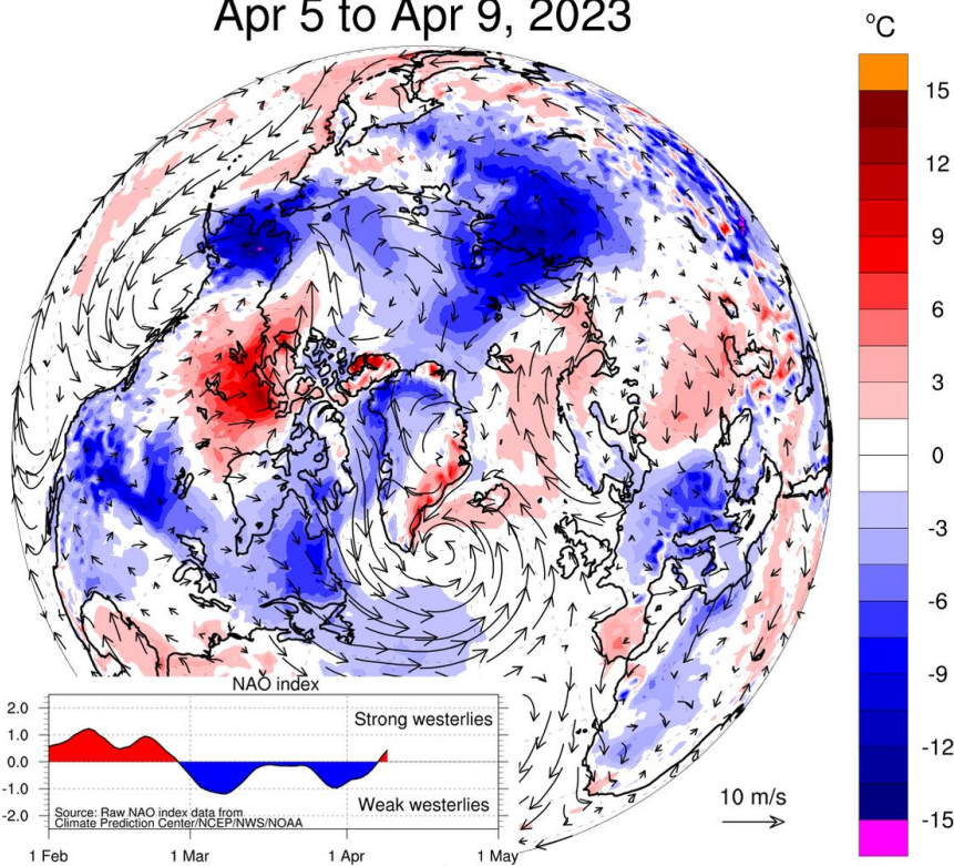
Рисунок 2е – Аномалии приземной температуры воздуха (2м) и осредненные вектора скорости ветра (10 м) за 05.04 – 09.04 в 2023-2024 гг. относительно периода 2004-2013 гг. ( http://polarportal.dk )
