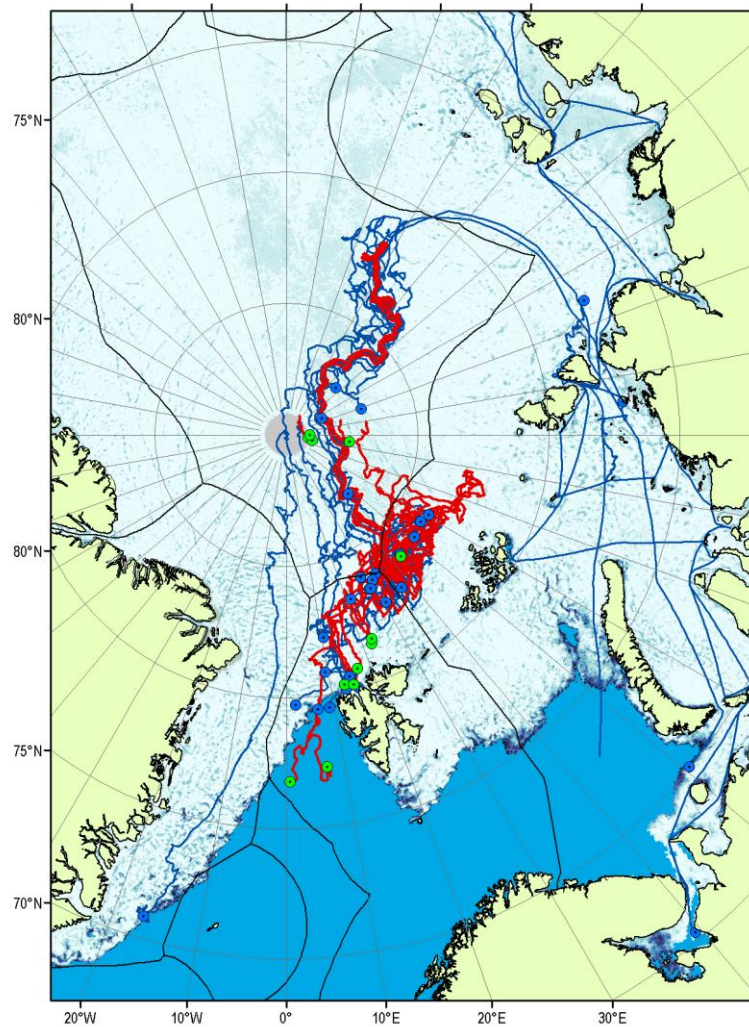
Сеть дрейфующих буев на 2024-04-11 0100UTC. AWI SIC LEADS (v.110) 2024-04-10PM. Обработка: МЦД МП ААНИИ.
