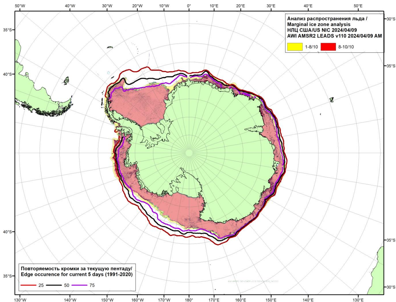
Рисунок 5в – Положение кромки льда и зон разреженных ( <8/10 ) и сплоченных ( \geq 8/10 ) льдов Южного океана за 09.04.2024 г. на основе ледового анализа Национального Ледового Центра США и повторяемость кромки за 06-10.04 за период 1991-2020 гг. по наблюдениям SSMR-SSM/I-SSMIS (алгоритм NASATEAM), совмещенное с положением разрежений на основе данных ИСЗ AMSR2 за 09.04.2024 (AWI, v110).
