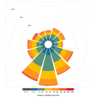
Рисунок 1а – Трек дрейфа ГСН и РСД дрейфующей станции «Северный Полос-41» на 11.04.2024, совмещенные с положением разрежений на основе данных ИСЗ AMSR2 за 10.04.2024 (Leads AWI, v110) и S1A. Красным/зеленым цветом выделены активные буи, синим неактивные буи. Диаграмма скоростей и направлений дрейфа за неделю дана в полярной проекции с осевым меридианом 0°
