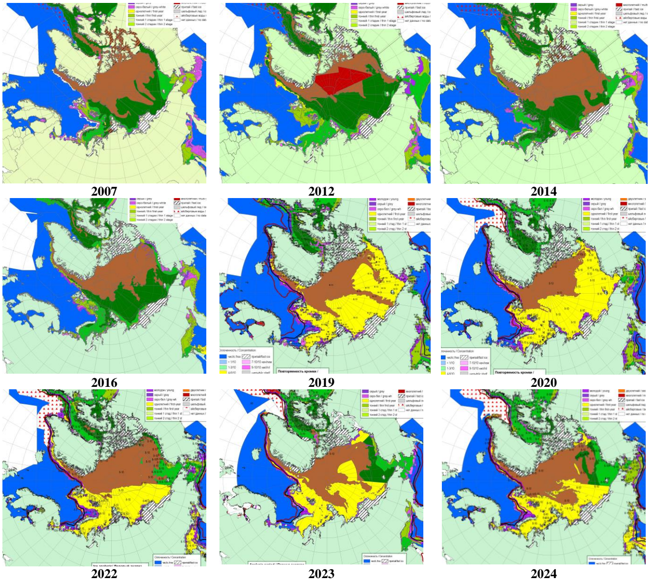
Рисунок 2а – Ледовые условия за 03.04-09.04.2024г. и аналогичные периоды 2007-2023 гг. на основе ледового анализа ААНИИ, НИЦ Планета, Канадской ледовой службы и Национального ледового центра США.
