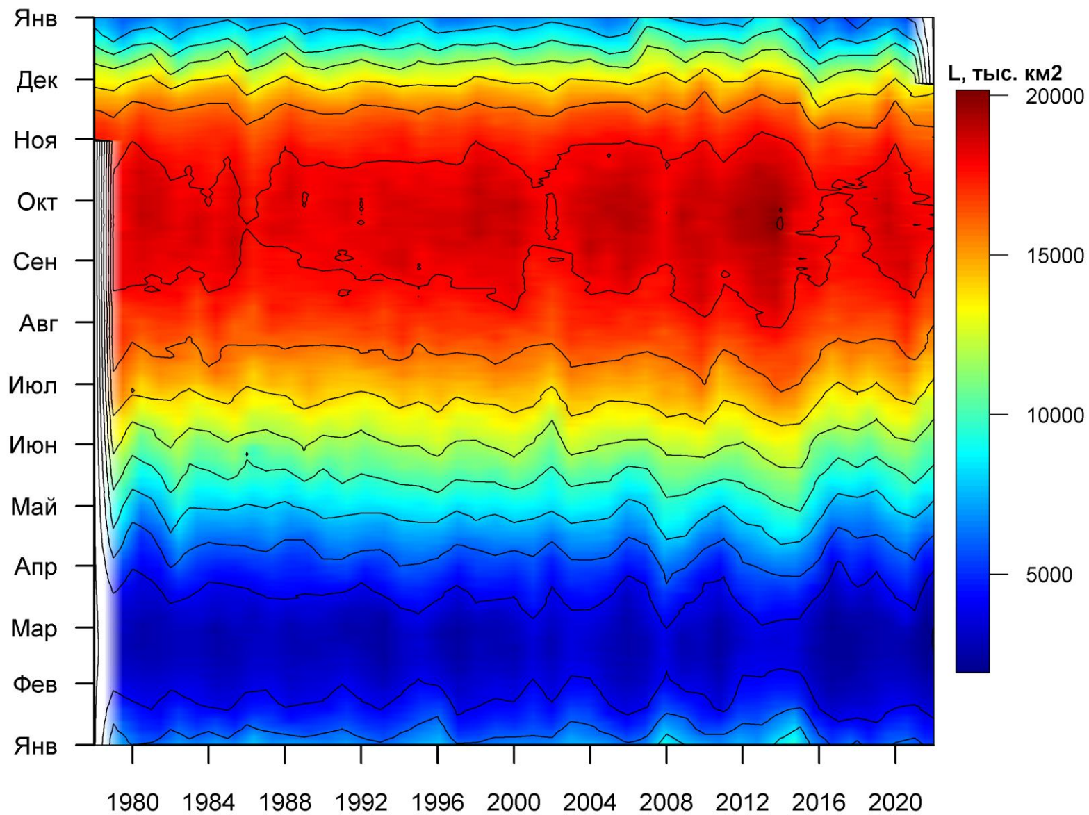
Рисунок 76 – Ежедневные оценки сезонных изменений ледовитости для Южного океана за период 26.10.1978 – 28.11.2022 на основе расчетов по данным SSMR-SSM/I-SSMIS, алгоритм NASATEAM.
