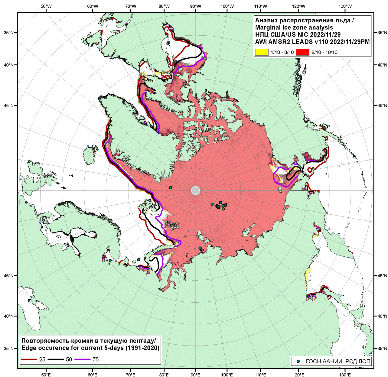
Рисунок 1в – Положение кромки льда и зон разреженных ( <8/10 ) и сплоченных ( \geq 8/10 ) льдов СЛО за 29.11.2022 г. на основе ледового анализа Национального Ледового Центра США и повторяемость кромки за 26-30.11 за период 1991-2020 гг. по наблюдениям SSMR-SSM/I-SSMIS (алгоритм NASATEAM).
