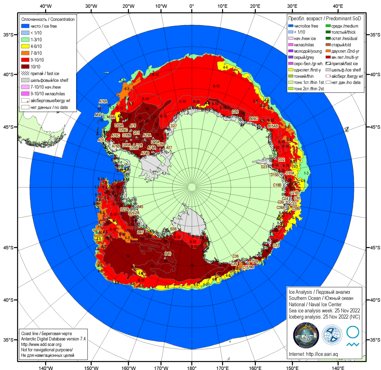
Рисунок 5а – Ледовая карта Южного океана (цветовая окраска по общей сплоченности) и расположение крупных айсбергов на основе ледового анализа за 25.11.2022 в рамках проекта совместного ледового картирования Южного океана ААНИИ, НЛЦ США и НМИ.
