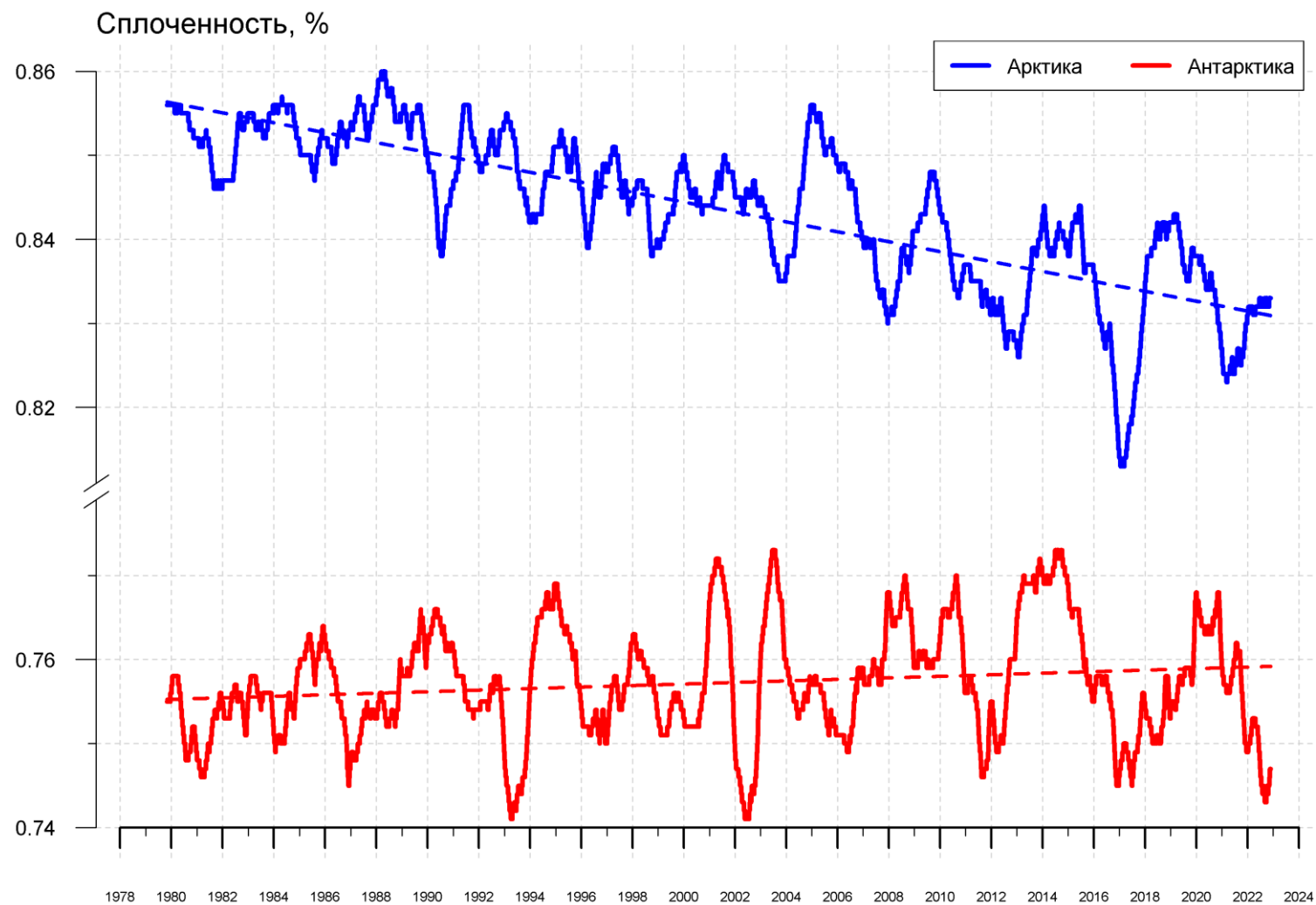
Рисунок 11 – Ежедневные сглаженные окном 365 суток значения средней общей сплоченности Арктики и Антарктики с 07.11.1978 по 28.11.2022 на основе SSMR-SSM/I-SSMIS
