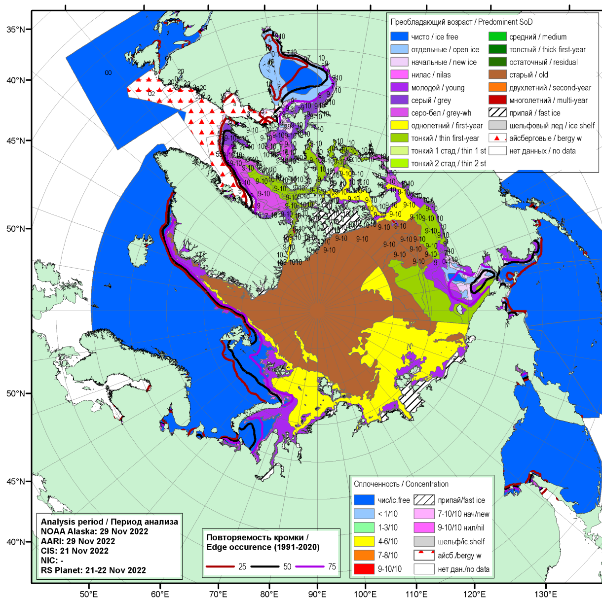
Рисунок 16 – Обзорная ледовая карта СЛО за 21.11-29.11.2022 г. (цветовая раскраска по преобладающему возрасту) на основе ледового анализа ААНИИ (29.11), NOAA Аляска (29.11), Канадской ледовой службы (21.11), НИЦ Планета (21-22.11) и Национального ледового центра США (-) и повторяемость кромки за 26-30.11 за период 1991-2020гг. по наблюдениям SSMR-SSM/I-SSMIS (алгоритм NASATEAM).
