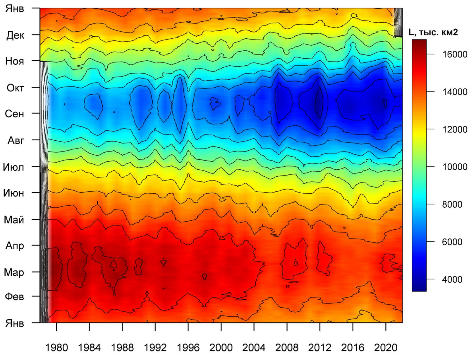
Рисунок 36 – Ежедневные оценки сезонных изменений ледовитости для Северной Полярной Области за период 26.10.1978 – 28.11.2022 на основе расчетов по данным SSMR-SSM/I-SSMIS, алгоритм NASATEAM.
