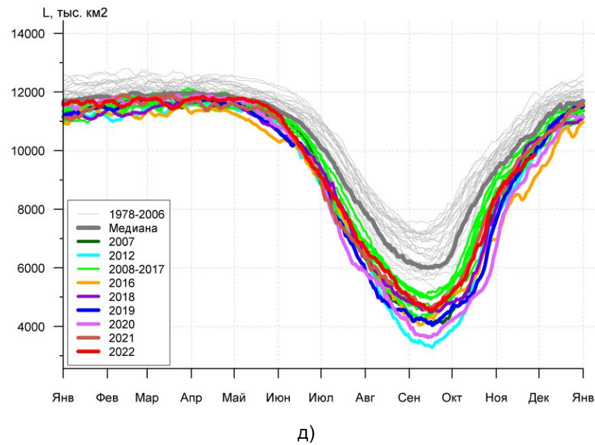
Рисунок 3а – Ежедневные оценки сезонного хода ледовитости для Северной Полярной Области и трех меридиональных секторов за период 26.10.1978 - 28.11.2022 по годам на основе расчетов по данным SSMR-SSM/I-SSMIS, алгоритмы NASATEAM: а) Северная полярная область, б) сектор 45°W-95°E (Гренландское – Карское моря), в) сектор 95°E-170°W (моря Лаптевых – Чукотское и Берингово, Охотское), г) сектор 170°W-45°W (море Бофорта и Канадская Арктика), д) Северный Ледовитый океан, е) Северный морской путь (Карское - Чукотское моря).
