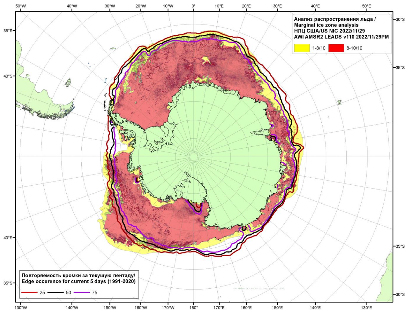
Рисунок 5в – Положение кромки льда и зон разреженных ( <8/10 ) и сплошных ( \geq 8/10 ) льдов Южного океана за 29.11.2022 г. на основе ледового анализа Национального Ледового Центра США и повторяемость кромки за 26-30.11 за период 1991-2020 гг. по наблюдениям SSMR-SSM/I-SSMIS (алгоритм NASATEAM), совмещенное с положением разрежений на основе данных ИСЗ AMSR2 за 29.11.2022 (AWI, v110).
