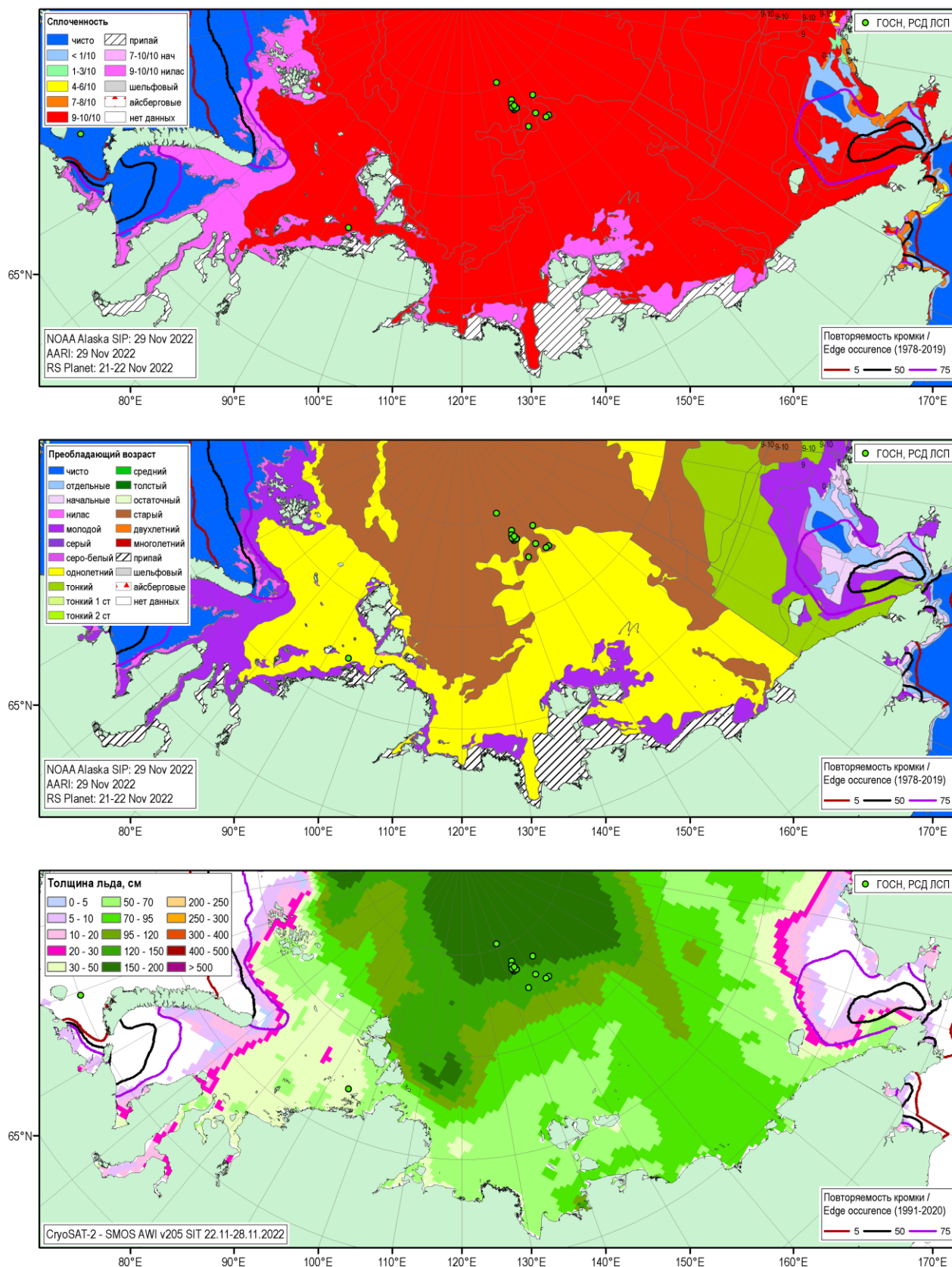
Рисунок 1г – Обзорная ледовая карта СМП за 21.11-29.11.2022 г. (цветовая раскраска по общей сплоченности – верх, по преобладающему возрасту - центр) на основе ледового анализа ААНИИ (29.11), NOAA Аляска (29.11), НИЦ Планета (21-22.11), Канадской ледовой службы (-.-) и Национального ледового центра США (-), оценка толщин льда по данным CryoSAT-2-SMOS AWI v205 за 22-28.11.2022 г. и повторяемость кромки за 26-20.11 за период 1991-2020гг. по наблюдениям SSMR-SSM/I-SSMIS (алгоритм NASATEAM). Положение РСД ЛСП представлено за 30.11.2022 1700МСК
