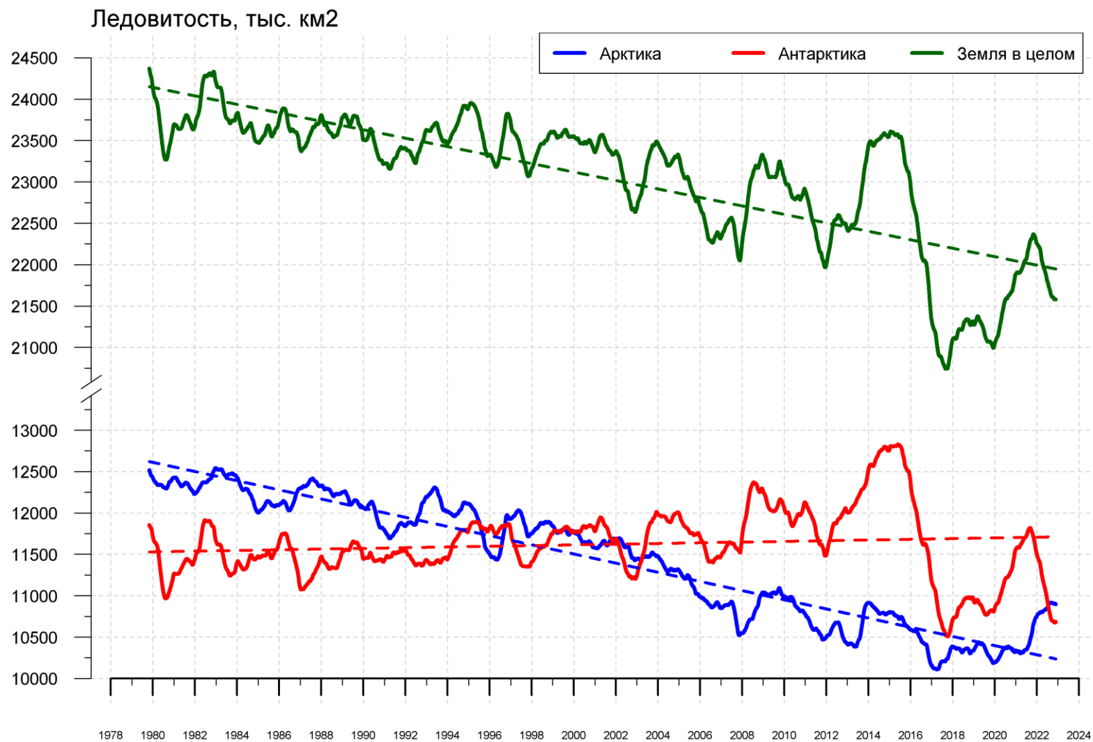
Рисунок 9 – Ежедневные сглаженные окном 365 суток значения ледовитости (площади распространения морского льда) Арктики, Антарктики и Земли в целом с 26.10.1978 по 28.11.2022 на основе SSMR-SSM/I-SSMIS
