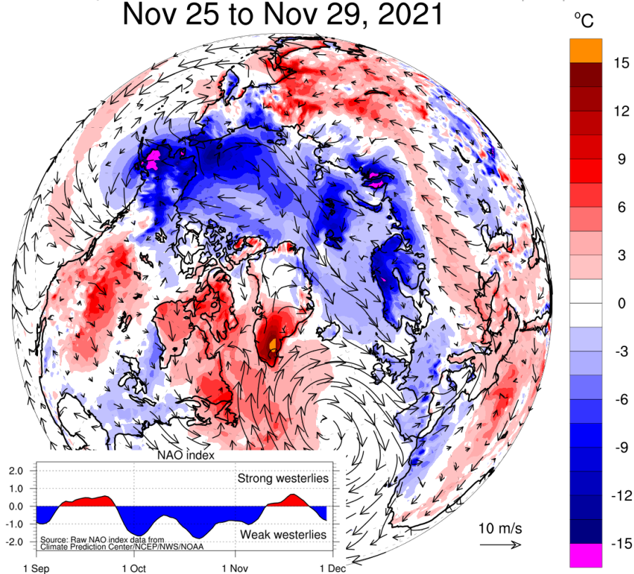
Рисунок 2е – Аномалии приземной температуры воздуха (2м) и осредненные вектора скорости ветра (10 м) за 25.11 - 29.11 в 2021-2022 гг. относительно периода 2004-2013 гг. ( http://polarportal.dk )
