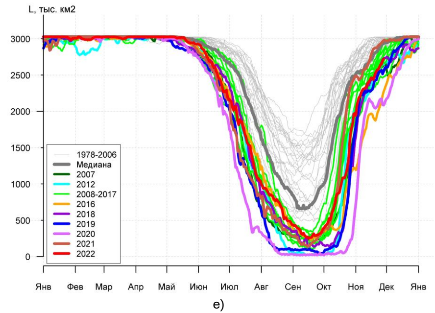
Рисунок 3а – Ежедневные оценки сезонного хода ледовитости для Северной Полярной Области и трех меридиональных секторов за период 26.10.1978 - 28.11.2022 по годам на основе расчетов по данным SSMR-SSM/I-SSMIS, алгоритмы NASATEAM: а) Северная полярная область, б) сектор 45°W-95°E (Гренландское – Карское моря), в) сектор 95°E-170°W (моря Лаптевых – Чукотское и Берингово, Охотское), г) сектор 170°W-45°W (море Бофорта и Канадская Арктика), д) Северный Ледовитый океан, е) Северный морской путь (Карское - Чукотское моря).
