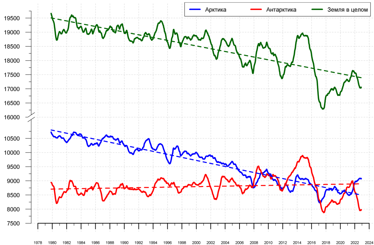
Рисунок 10 – Ежедневные сглаженные окном 365 суток значения приведенной ледовитости (площади морского льда) Арктики, Антарктики и Земли в целом с 26.10.1978 по 28.11.2022 на основе SSMR-SSM/I-SSMIS
