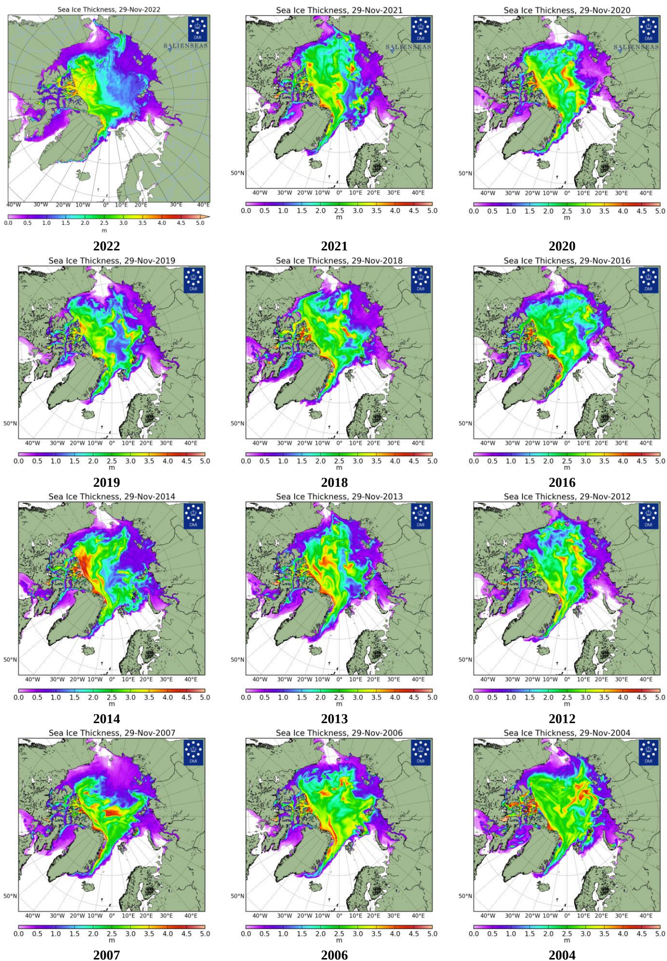
Рисунок 26 – Поля распределения средневзвешенной толщины льда совместной модели морского льда – океана HYCOM/CICE Датского метеорологического института 29.11 за 2004-2022 гг.
