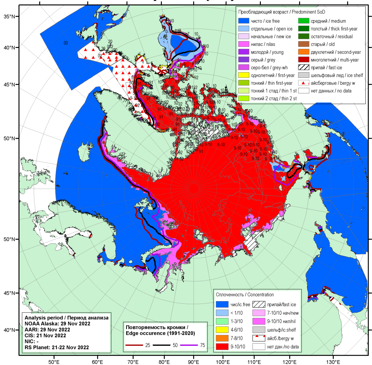
Рисунок 1а – Обзорная ледовая карта СЛО за 21.11-29.11.2022 г. (цветовая раскраска по общей сплоченности) на основе ледового анализа ААНИИ (29.11), НОАА Аляска (29.11), Канадской ледовой службы (21.11), НИЦ Планета (21-22.11) и Национального ледового центра США (-) и повторяемость кромки за 26-30.11 за период 1991-2020гг. по наблюдениям SSMR-SSM/I-SSMIS (алгоритм NASATEAM).
