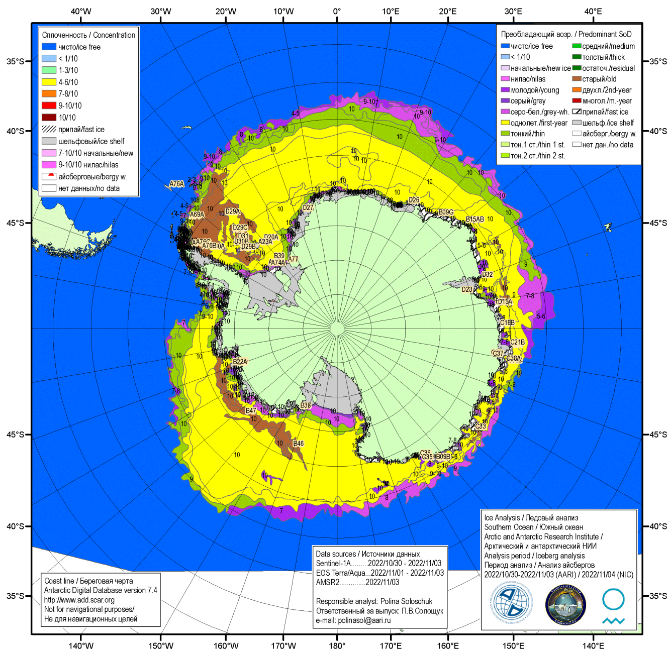
Рисунок 5в – Ледовая карта Южного океана (цветовая окраска по возрасту) и расположение крупных айсбергов на основе ледового анализа за 04.11.2022 в рамках проекта совместного ледового картирования Южного океана ААНИИ, НЛЦ США и НМИ.
