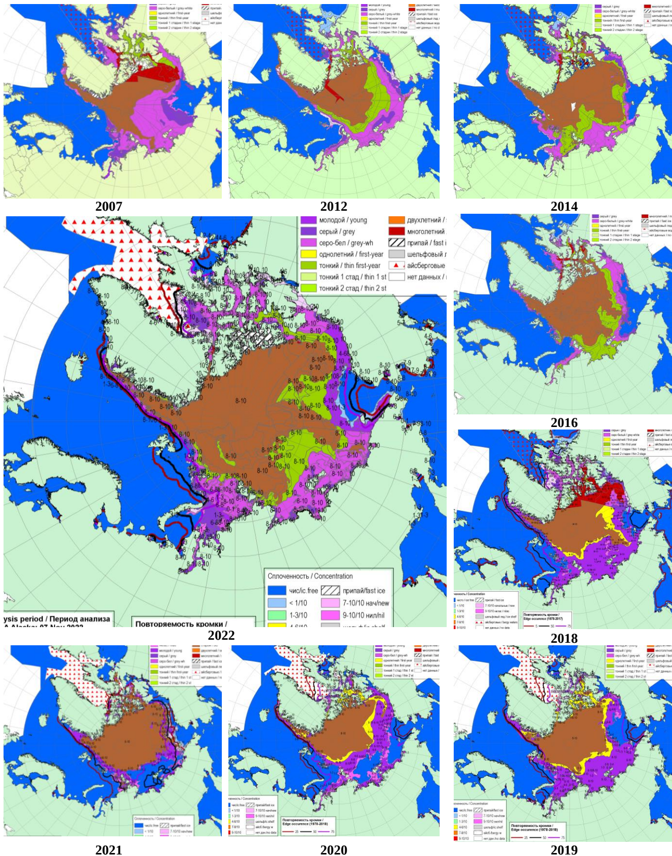
Рисунок 2а – Оценка сплоченности морского льда за 04.11-08.11.2022г. и аналогичные периоды 2007-2021гг. на основе ледового анализа ААНИИ, НИЦ Планета, Канадской ледовой службы и Национального ледового центра США.
