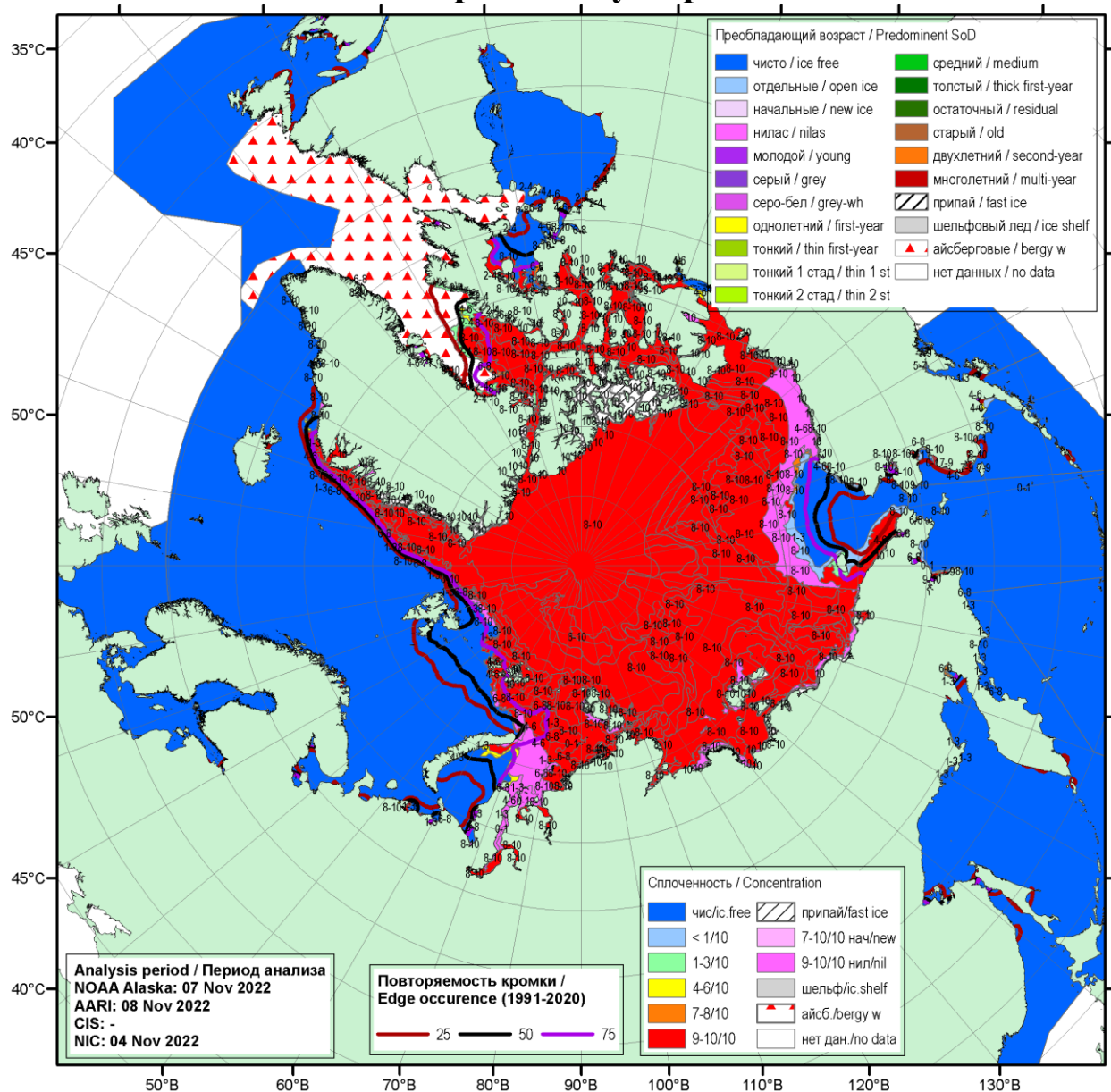
Рисунок 1а – Обзорная ледовая карта СЛО за 03.11-08.11.2022 г. (цветовая раскраска по общей сплоченности) на основе ледового анализа ААНИИ (08.11), NOAA Аляска (07.11), Канадской ледовой службы (-.-) и Национального ледового центра США (04.11) и повторяемость кромки за 06-10.11 за период 1991-2020гг. по наблюдениям SSMR-SSM/I-SSMIS (алгоритм NASATEAM).
