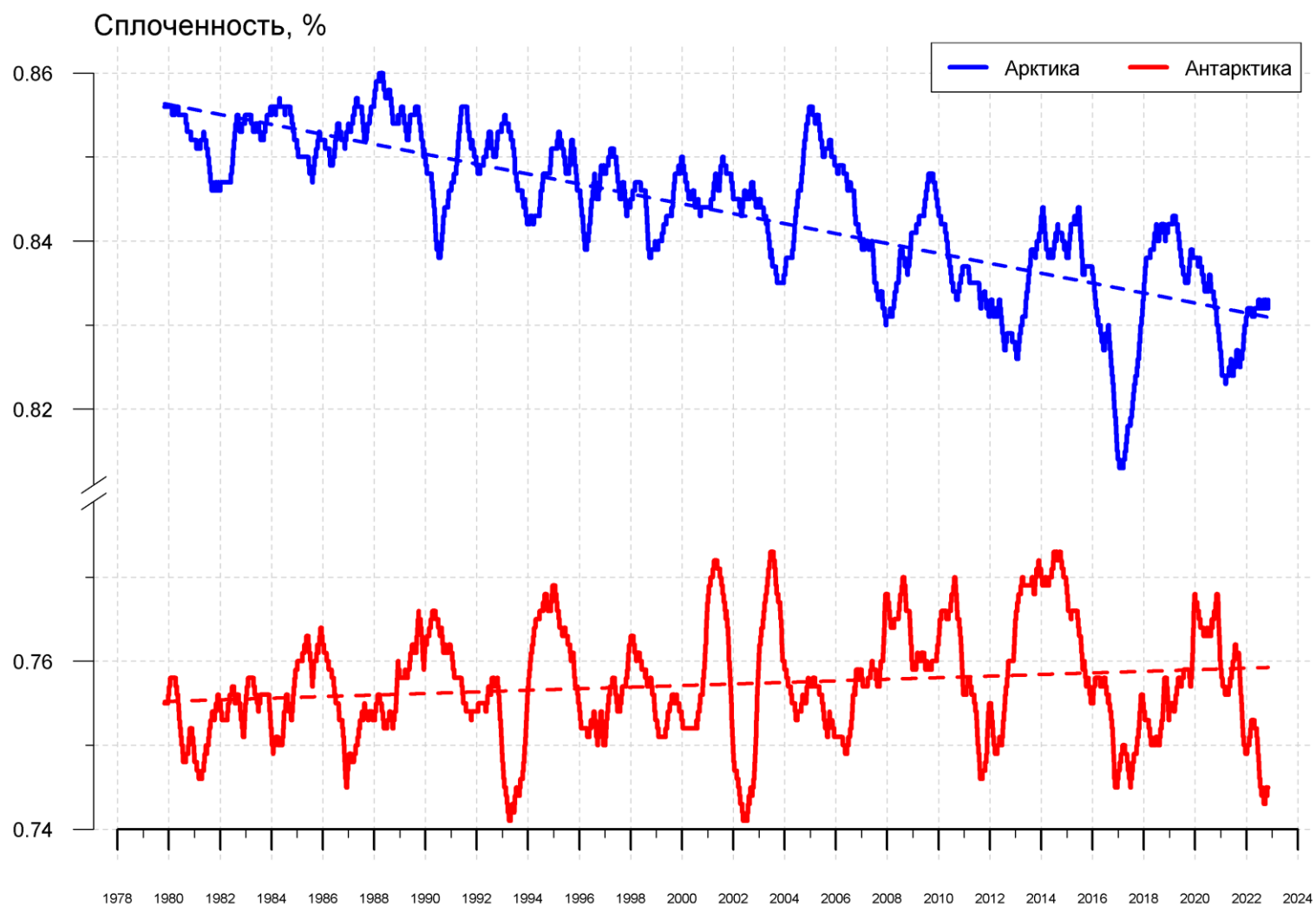
Рисунок 11 – Ежедневные сглаженные окном 365 суток значения средней общей сплоченности Арктики и Антарктики с 06.11.1978 по 30.10.2022 на основе SSMR-SSM/I-SSMIS
