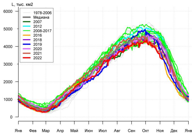
Рисунок 7а – Ежедневные оценки сезонного хода ледовитости Южного Океана и меридиональных секторов за период 26.10.1978 – 06.11.2022 по годам на основе расчетов по данным SSMR-SSM/I-SSMIS, алгоритм NASATEAM: а) Южный Океан, б) Атлантический сектор (60°W-30°E, море Уэдделла), в) Индоокеанский сектор (30°E-150°E, моря Космонавтов, Содружества, Моусона), г) Тихоокеанский сектор (150°E-60°W, моря Росса, Беллинсгаузена)
