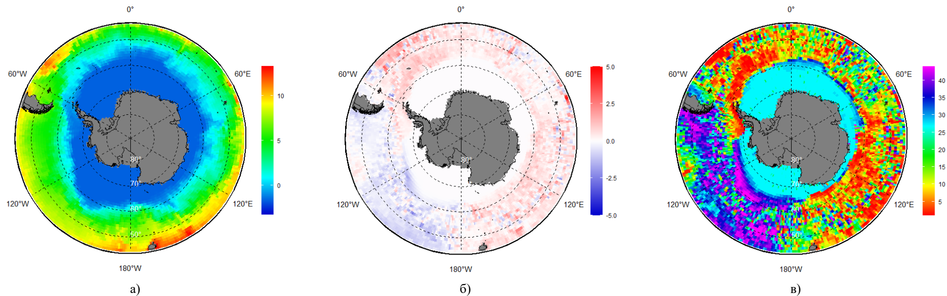
Рисунок 66 – Реанализ ERA5 температуры поверхности воды ( ^{\circ}\text{C} ) за период 26.10 – 01.11.2022 г.: (а) – осредненные значения, (б) – аномалия относительно периода 1991-2020 гг. и (в) – ранг за период 1979-2022 гг.
