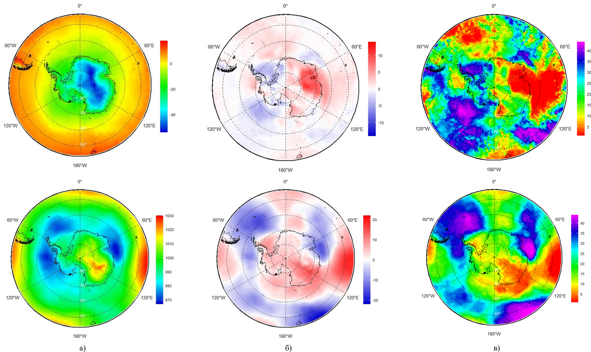
Рисунок 6а – Реанализ ERA5 температуры воздуха на уровне 2м (C°) и атмосферного давления на уровне моря (гПа) за период 26.10 – 01.11.2022 г.: (а) -средненные значения, (б) – аномалия относительно периода 1991-2020 гг. и (в) – ранг за период 1979-2022 гг.
