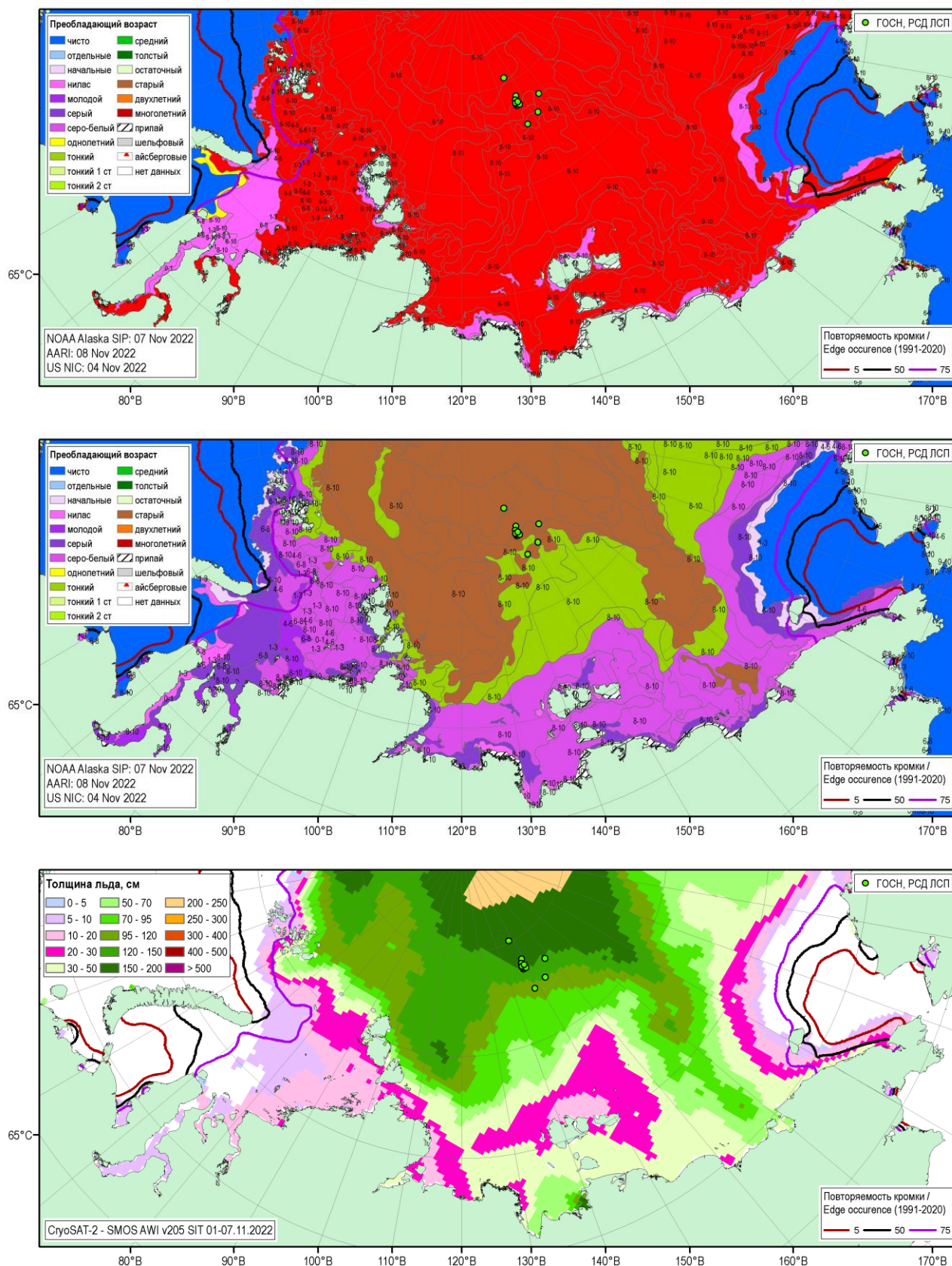
Рисунок 1г – Обзорная ледовая карта СМП за 04.11-08.11.2022 г. (цветовая раскраска по общей сплоченности – верх, по преобладающему возрасту - центр) на основе ледового анализа ААНИИ (08.11), NOAA Аляска (07.11), Канадской ледовой службы (-) и Национального ледового центра США (04.11), оценка толщин льда по данным CryoSAT-2-SMOS AWI v205 за 01-07.11.2022 г. и повторяемость кромки за 06-10.11 за период 1991-2020гг. по наблюдениям SSMR-SSM/I-SSMIS (алгоритм NASATEAM). Положение РСД ЛСП представлено за 08.11.2022 1300МСК
