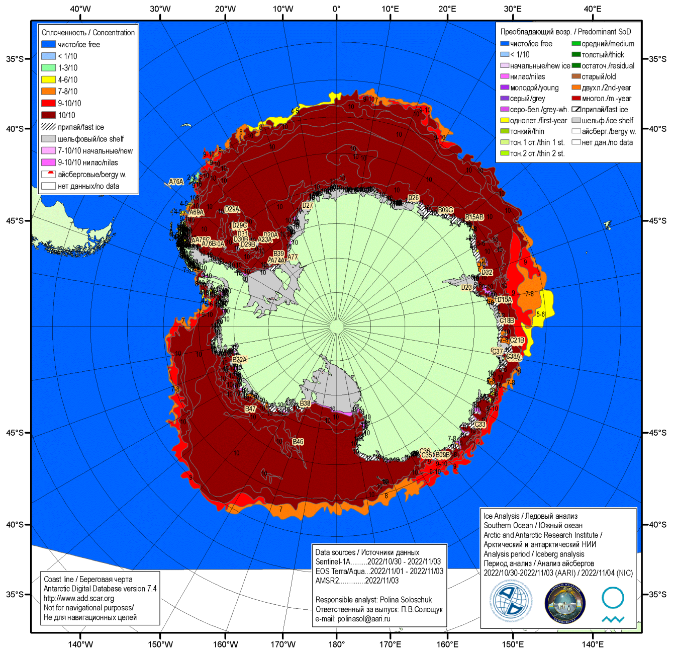
Рисунок 5а – Ледовая карта Южного океана (цветовая окраска по общей сплоченности) и расположение крупных айсбергов на основе ледового анализа за 04.11.2022 в рамках проекта совместного ледового картирования Южного океана ААНИИ, НЛЦ США и НМИ.
