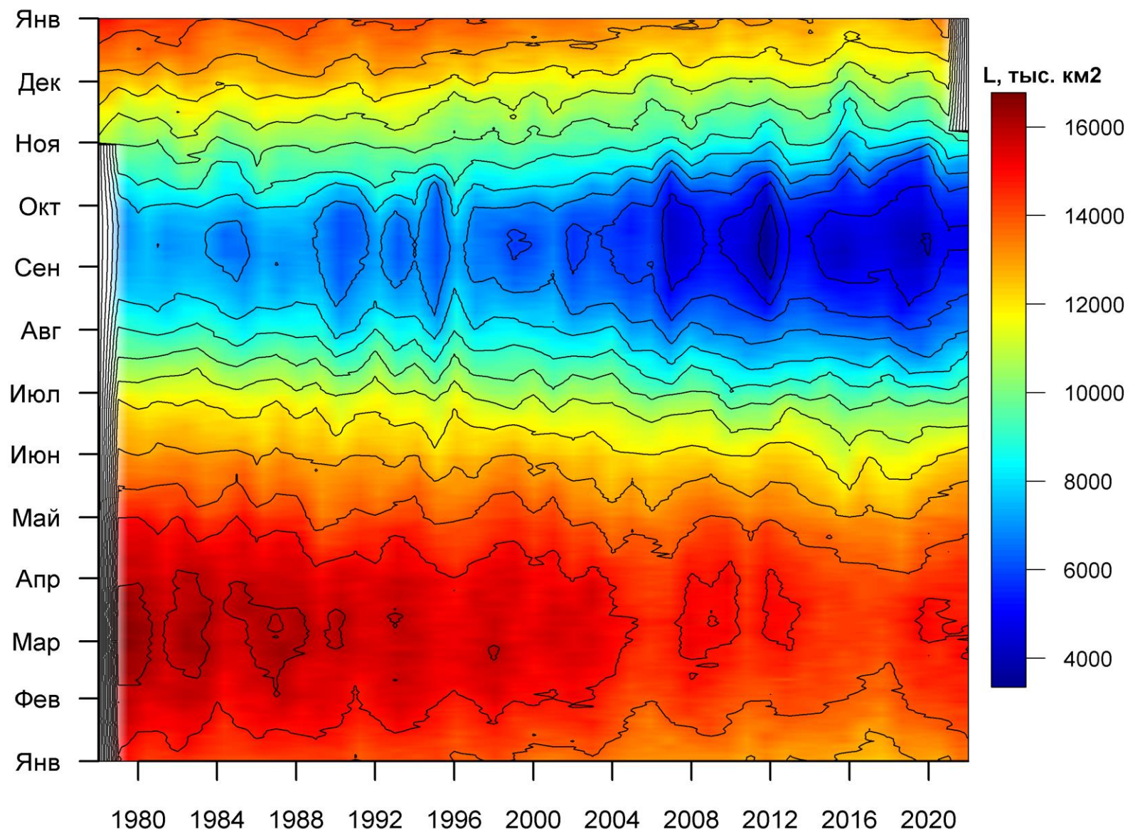
Рисунок 36 – Ежедневные оценки сезонных изменений ледовитости для Северной Полярной Области за период 26.10.1978 – 06.11.2022 на основе расчетов по данным SSMR-SSM/I-SSMIS, алгоритм NASATEAM.
