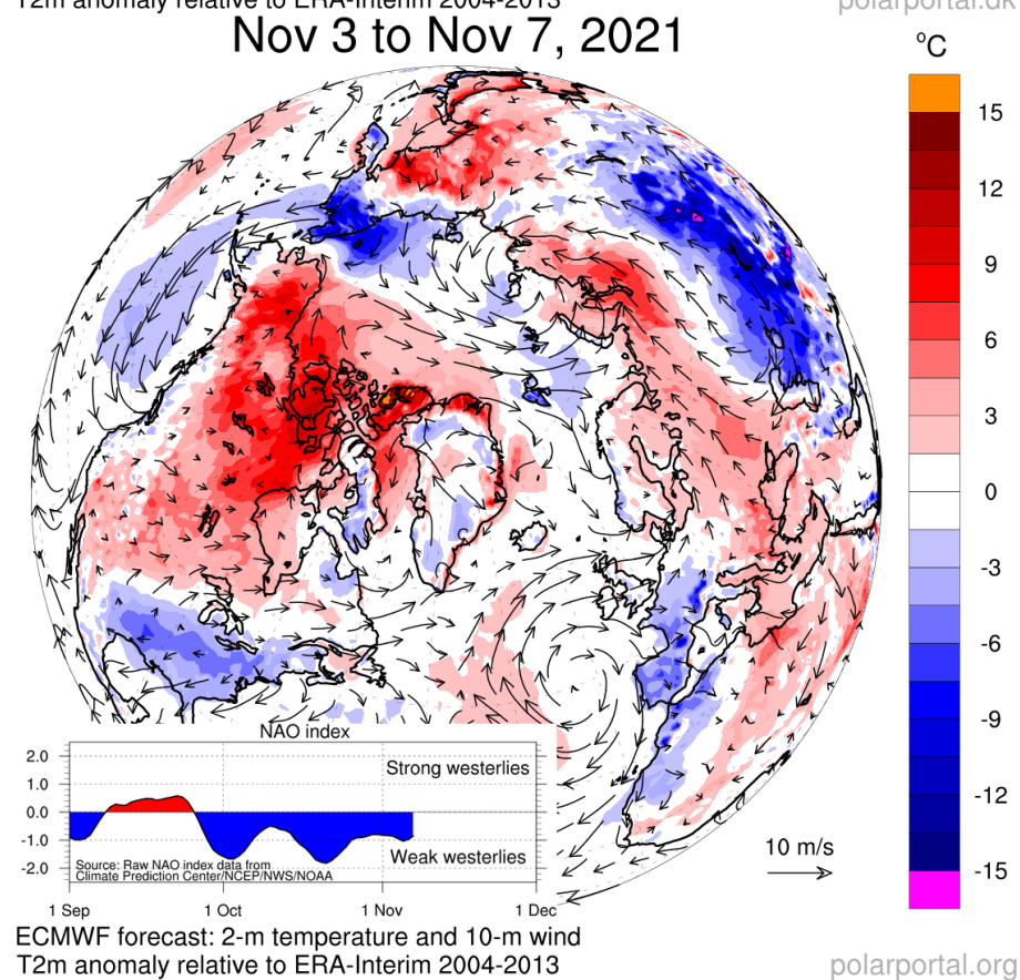
Рисунок 2е – Аномалии приземной температуры воздуха (2м) и осредненные вектора скорости ветра (10 м) за 03.11 - 07.11 в 2021-2022 гг. относительно периода 2004-2013 гг. ( http://polarportal.dk )
