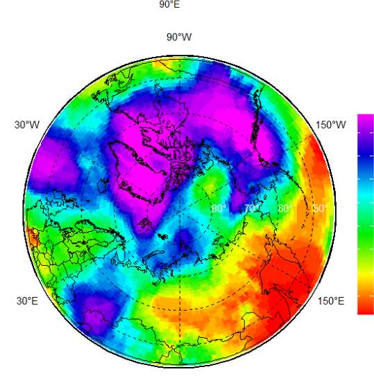
Рисунок 3а – Реанализ ERA5 температуры воздуха на уровне 2м (C°) и атмосферного давления на уровне моря (гПа) за период 26.10 – 01.11.2022 г.: (а) – осредненные значения, (б) – аномалия относительно периода 1991-2020 гг. и (в) – ранг за период 1979-2022 гг.
