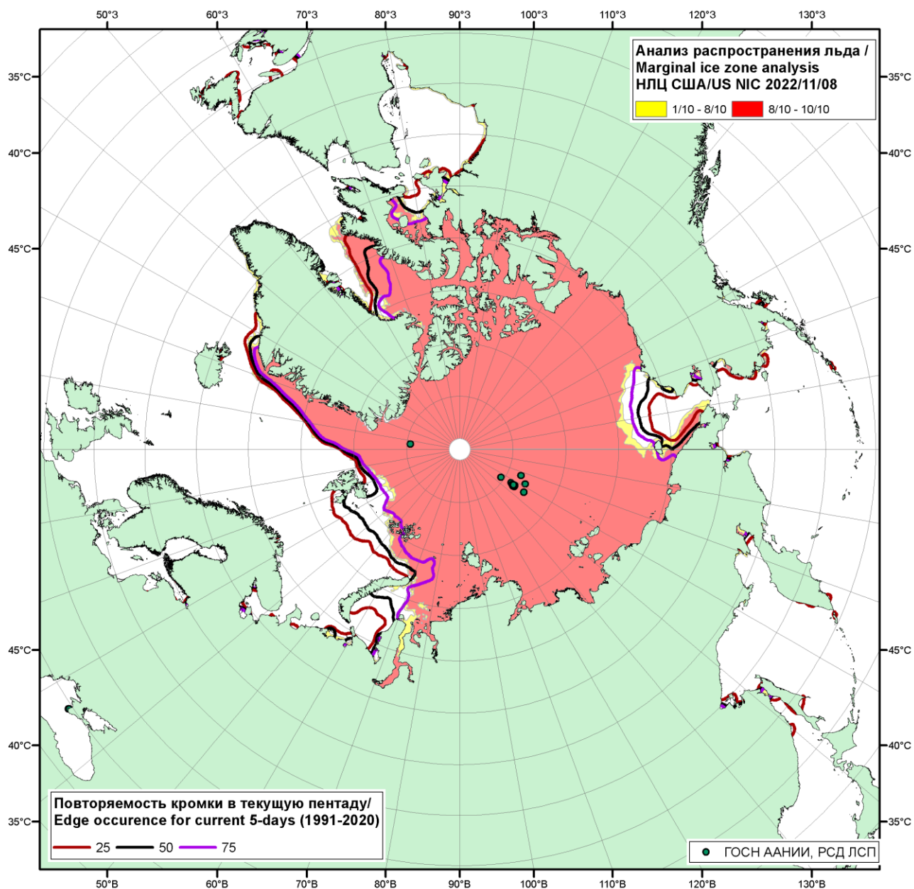
Рисунок 1в – Положение кромки льда и зон разреженных ( <8/10 ) и сплоченных ( \geq 8/10 ) льдов СЛО за 08.11.2022 г. на основе ледового анализа Национального Ледового Центра США и повторяемость кромки за 06-10.11 за период 1991-2020 гг. по наблюдениям SSMR-SSM/I-SSMIS (алгоритм NASATEAM).
