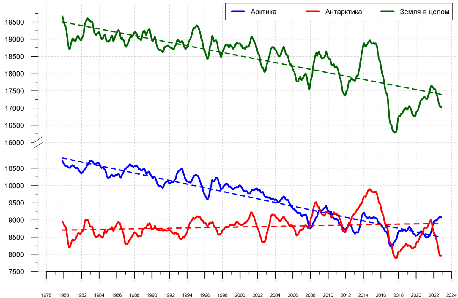
Рисунок 10 – Ежедневные сглаженные окном 365 суток значения приведенной ледовитости (площади морского льда) Арктики, Антарктики и Земли в целом с 26.10.1978 по 06.11.2022 на основе SSMR-SSM/I-SSMIS
