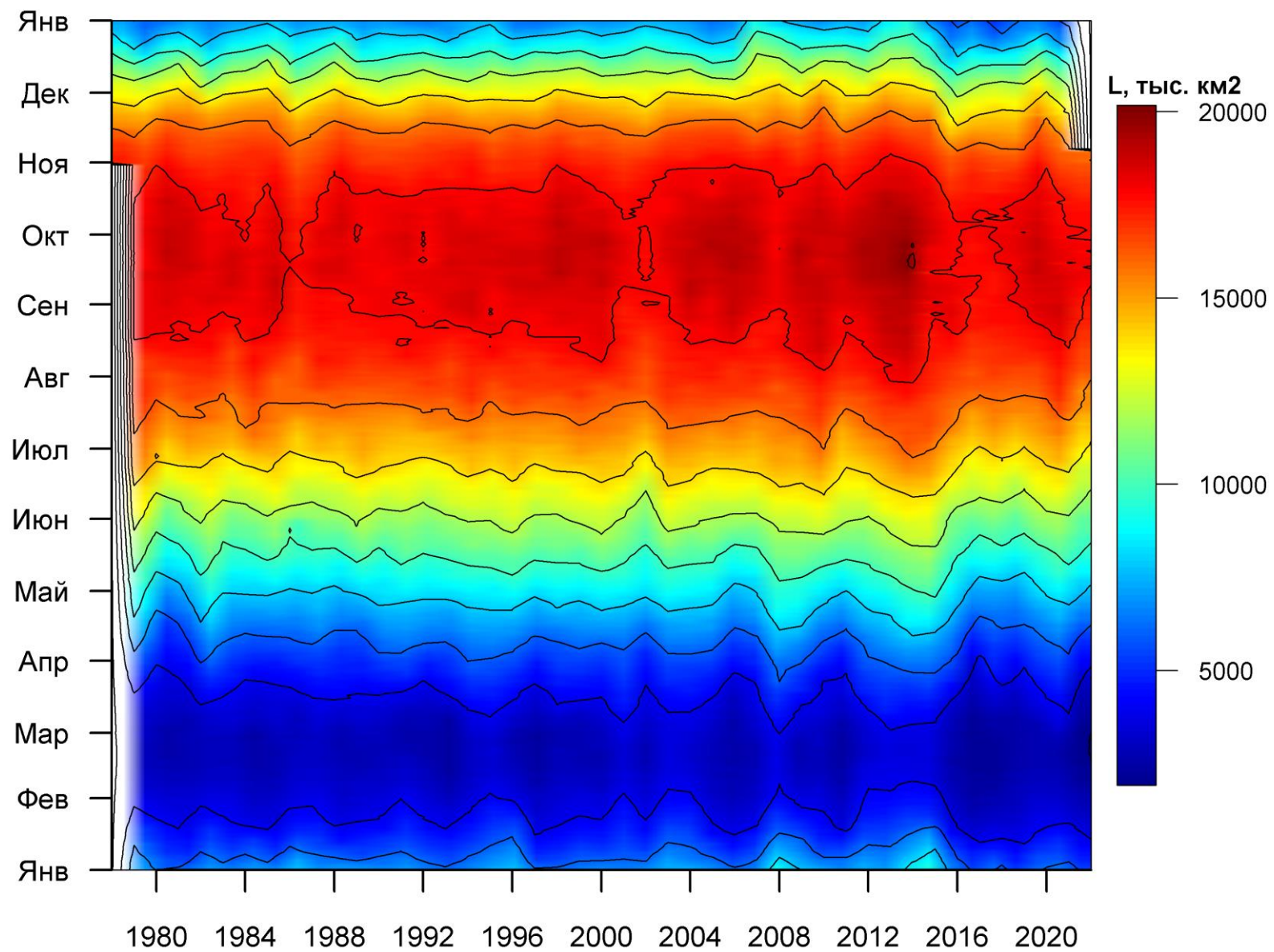
Рисунок 76 – Ежедневные оценки сезонных изменений ледовитости для Южного океана за период 26.10.1978 – 06.11.2022 на основе расчетов по данным SSMR-SSM/I-SSMIS, алгоритм NASATEAM.
