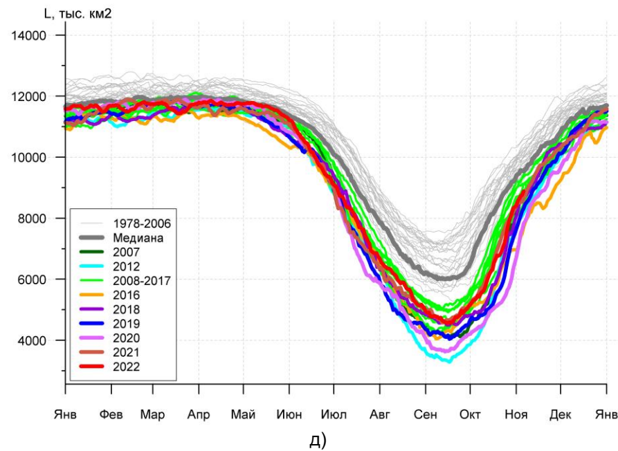
Рисунок 3а – Ежедневные оценки сезонного хода ледовитости для Северной Полярной Области и трех меридиональных секторов за период 26.10.1978 - 06.11.2022 по годам на основе расчетов по данным SSMR-SSM/I-SSMIS, алгоритмы NASATEAM: а) Северная полярная область, б) сектор 45°W-95°E (Гренландское – Карское моря), в) сектор 95°E-170°W (моря Лаптевых – Чукотское и Берингово, Охотское), г) сектор 170°W-45°W (море Бофорта и Канадская Арктика), д) Северный Ледовитый океан, е) Северный морской путь (Карское - Чукотское моря).
