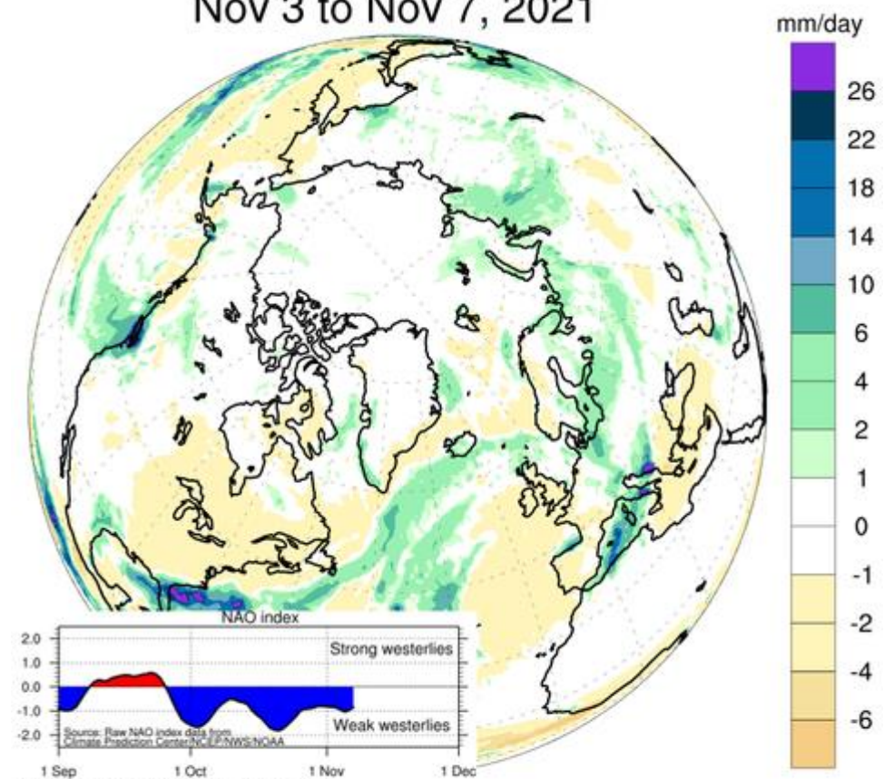
Рисунок 2ж – Аномалии приземной суммы осадков за 03.11-07.11 в 2021-2022 гг. относительно периода 2004-2013 гг. ( http://polarportal.dk )
