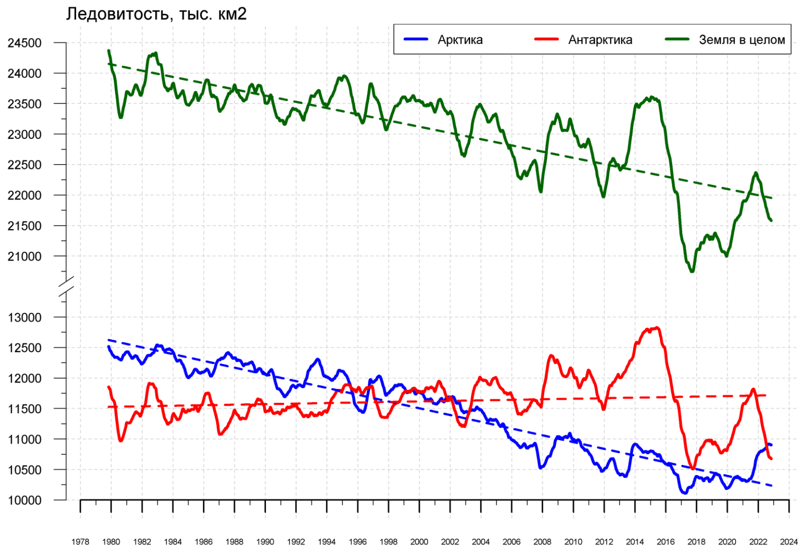
Рисунок 9 – Ежедневные сглаженные окном 365 суток значения ледовитости (площади распространения морского льда) Арктики, Антарктики и Земли в целом с 26.10.1978 по 06.11.2022 на основе SSMR-SSM/I-SSMIS
