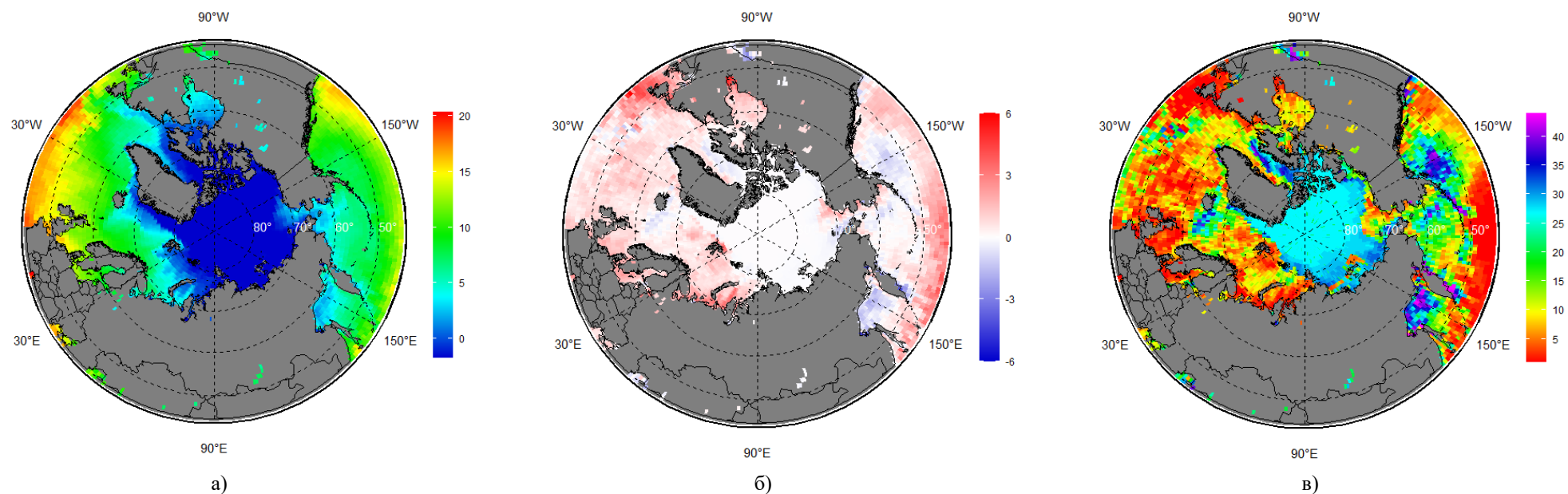
Рисунок 3б – Реанализ ERA5 температуры поверхности воды (C°) за период 26.10 – 01.11.2022 г.: (а) – осредненные значения, (б) – аномалия относительно периода 1991-2020 гг. и (в) – ранг за период 1979-2022 гг.
