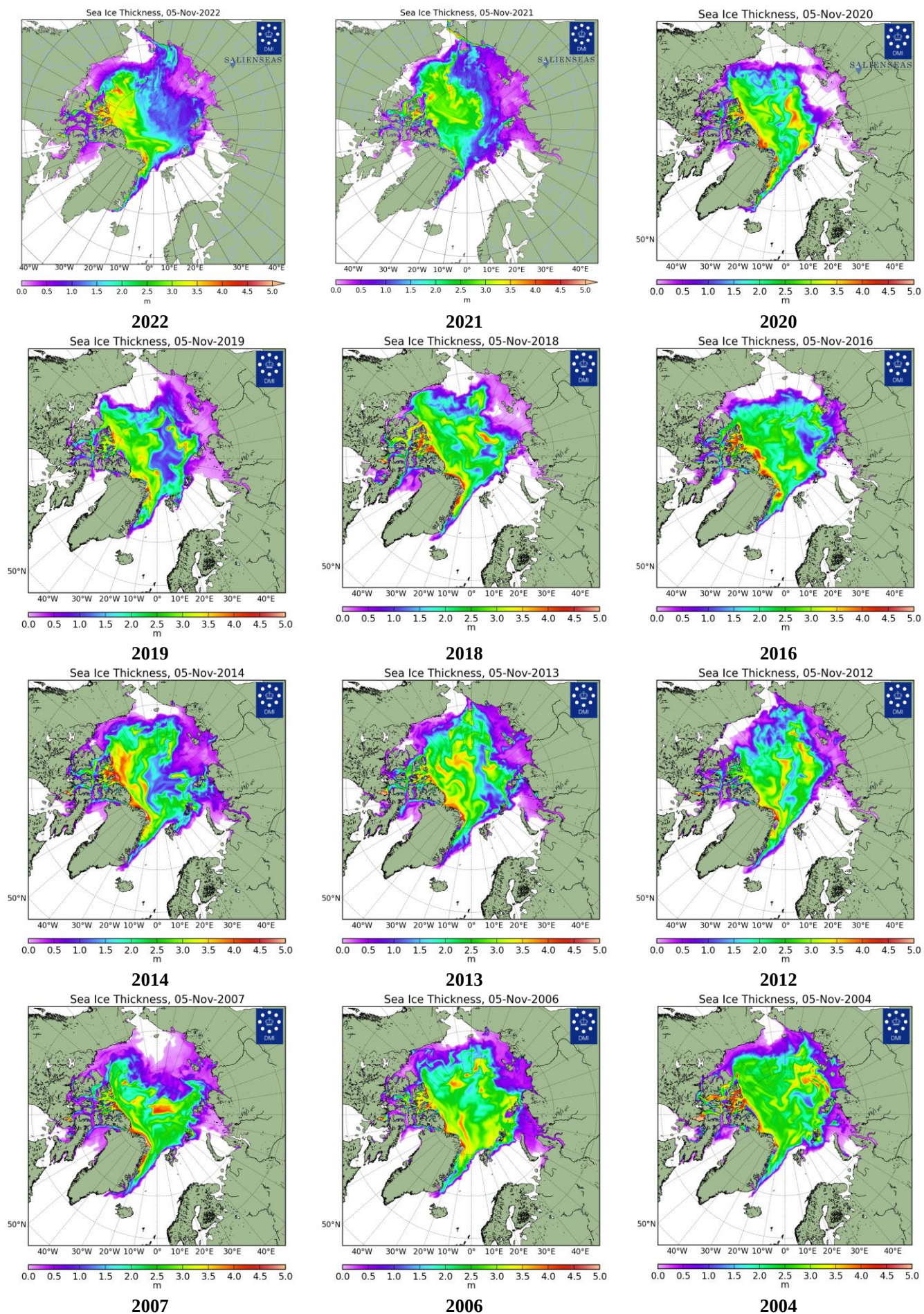
Рисунок 26 – Поля распределения средневзвешенной толщины льда совместной модели морского льда – океана NUCOM/CICE Датского метеорологического института 05.11 за 2004-2022 гг.
