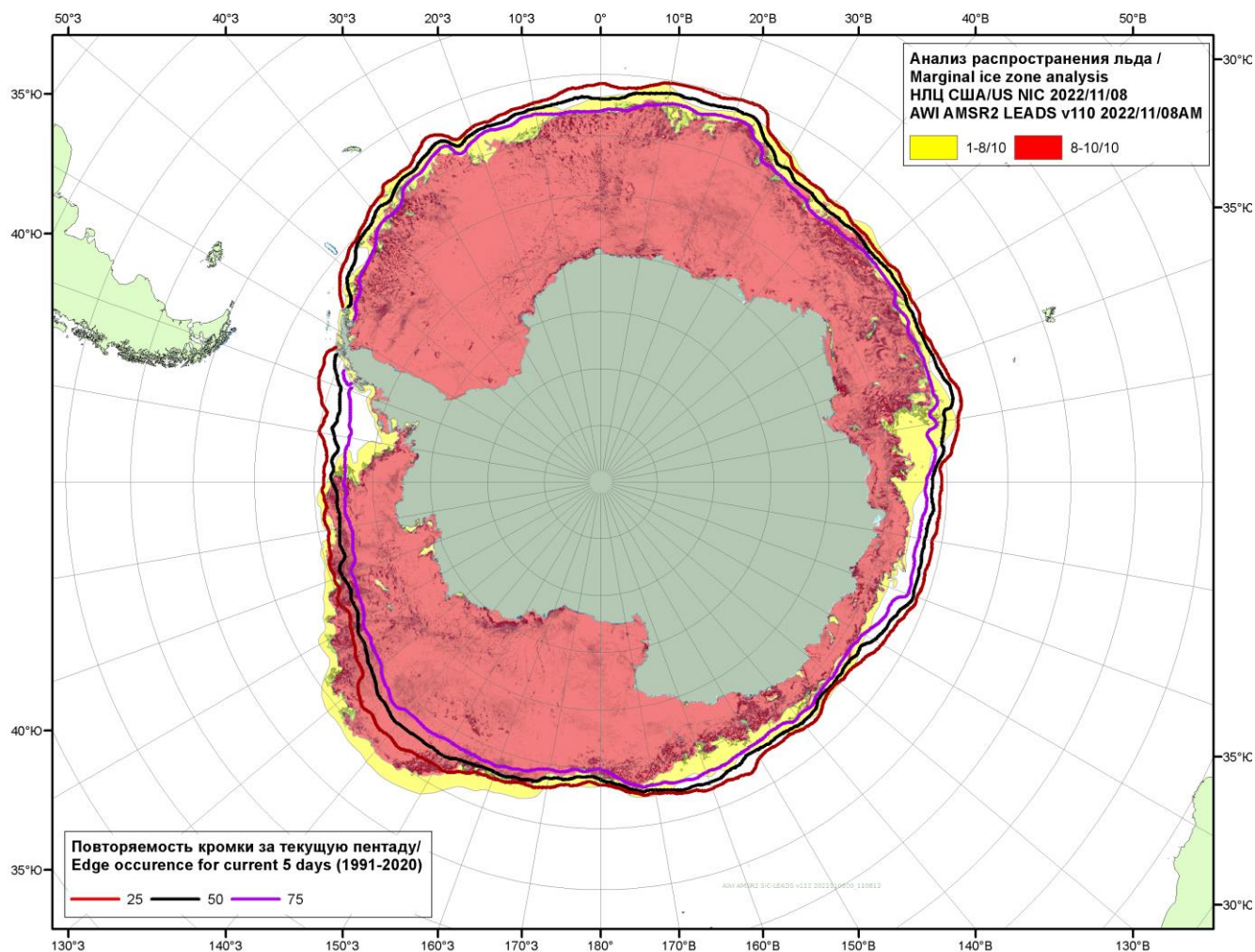
Рисунок 5в – Положение кромки льда и зон разреженных ( <8/10 ) и сплошных ( \geq 8/10 ) льдов Южного океана за 08.11.2022 г. на основе ледового анализа Национального Ледового Центра США и повторяемость кромки за 06-11.11 за период 1991-2020 гг. по наблюдениям SSMR-SSM/I-SSMIS (алгоритм NASATEAM), совмещенное с положением разрежений на основе данных ИСЗ AMSR2 за 08.11.2022 (AWI, v110).
