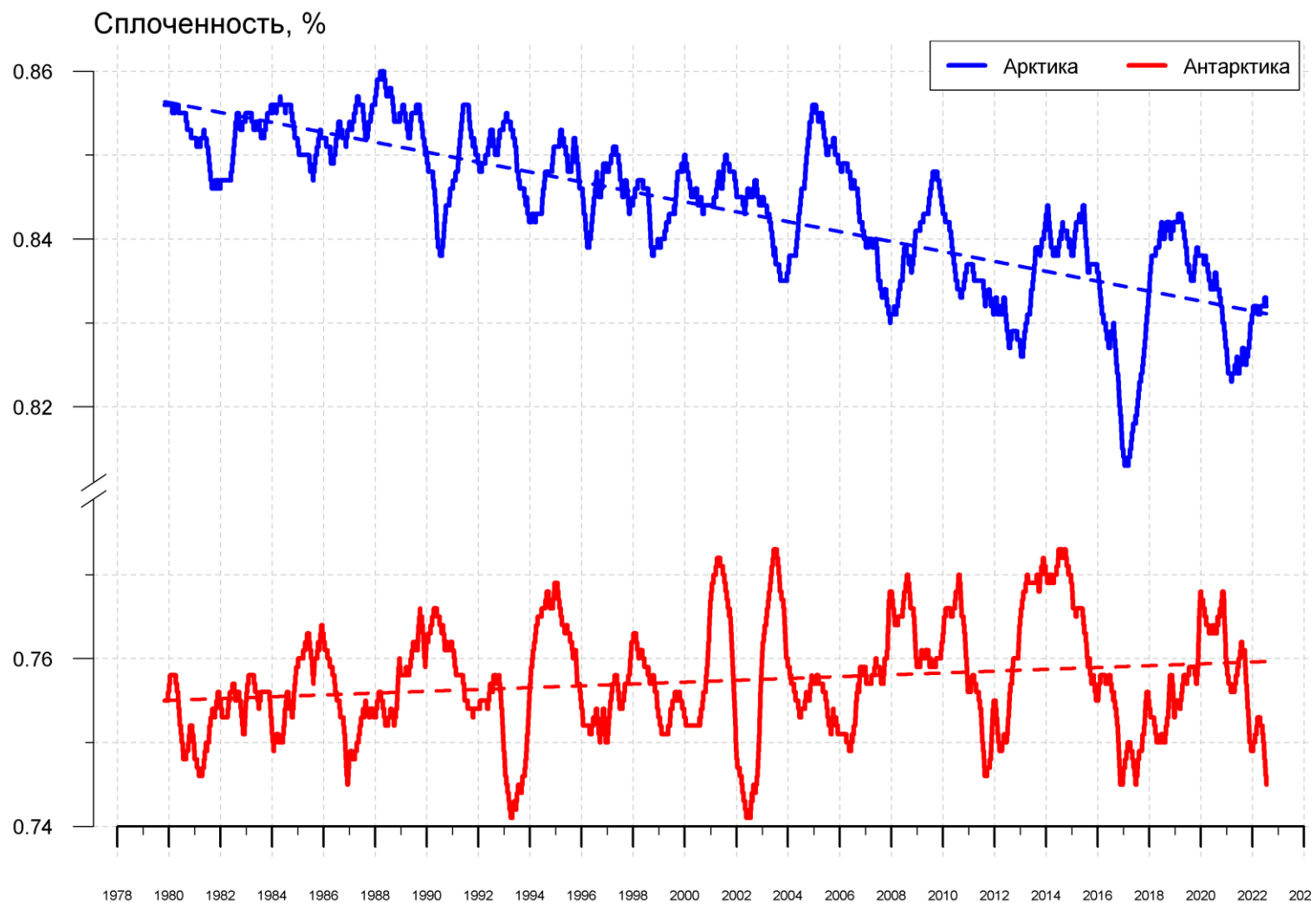
Рисунок 11 – Ежедневные сглаженные окном 365 суток значения средней общей сплоченности Арктики и Антарктики с 07.11.1978 по 19.07.2022 на основе SSMR-SSM/I-SSMIS
