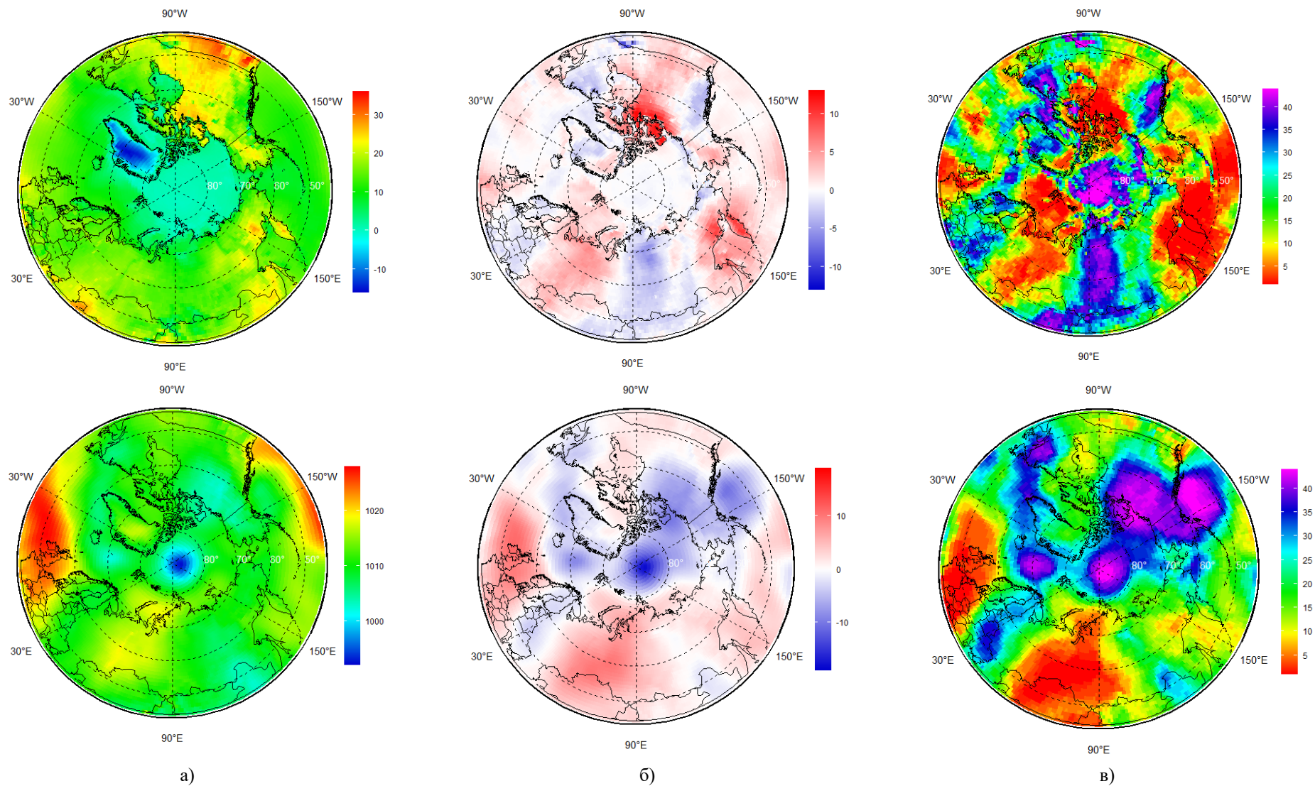
Рисунок 3а – Реанализ ERA5 температуры воздуха на уровне 2м (C°) и атмосферного давления на уровне моря (гПа) за период 08.07 – 14.07.2022 г.: (а) – осредненные значения, (б) – аномалия относительно периода 1991-2020 гг. и (в) – ранг за период 1979-2022 гг.
