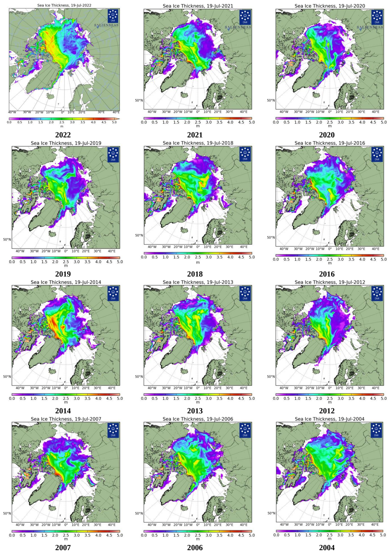
Рисунок 26 – Поля распределения средневзвешенной толщины льда совместной модели морского льда – океана NUCOM/CICE Датского метеорологического института 19.07 за 2004-2022 гг.
