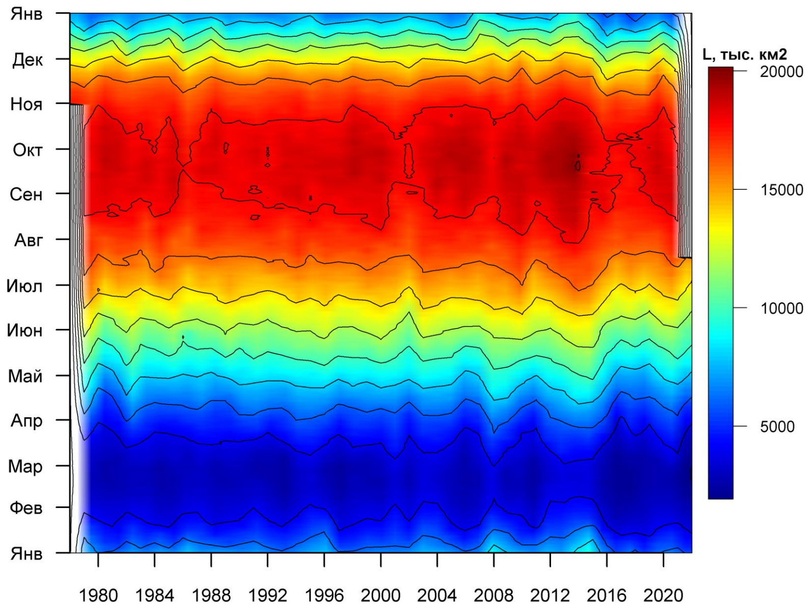
Рисунок 76 – Ежедневные оценки сезонных изменений ледовитости для Южного океана за период 26.10.1978 – 19.07.2022 на основе расчетов по данным SSMR-SSM/I-SSMIS, алгоритм NASATEAM.
