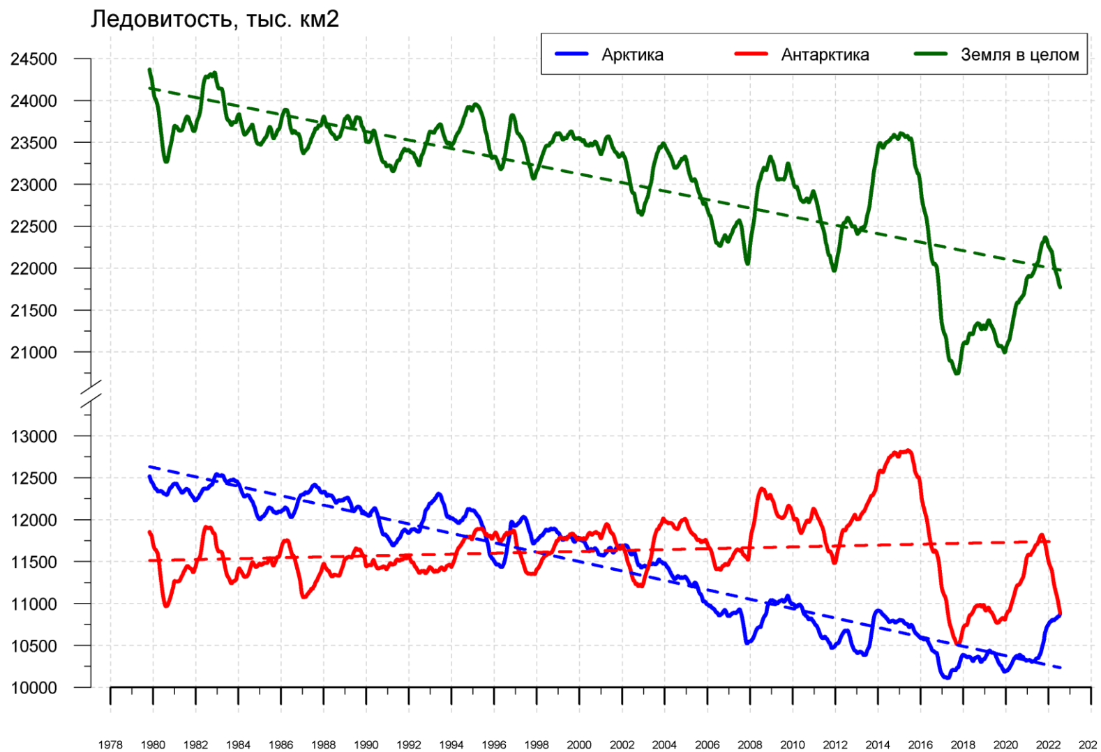
Рисунок 9 – Ежедневные сглаженные окном 365 суток значения ледовитости (площади распространения морского льда) Арктики, Антарктики и Земли в целом с 26.10.1978 по 19.07.2022 на основе SSMR-SSM/I-SSMIS
