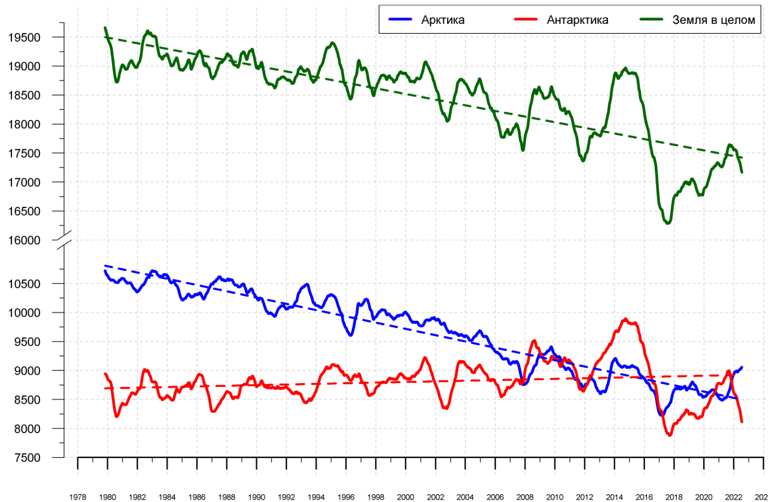
Рисунок 10 – Ежедневные сглаженные окном 365 суток значения приведенной ледовитости (площади морского льда) Арктики, Антарктики и Земли в целом с 26.10.1978 по 19.07.2022 на основе SSMR-SSM/I-SSMIS
