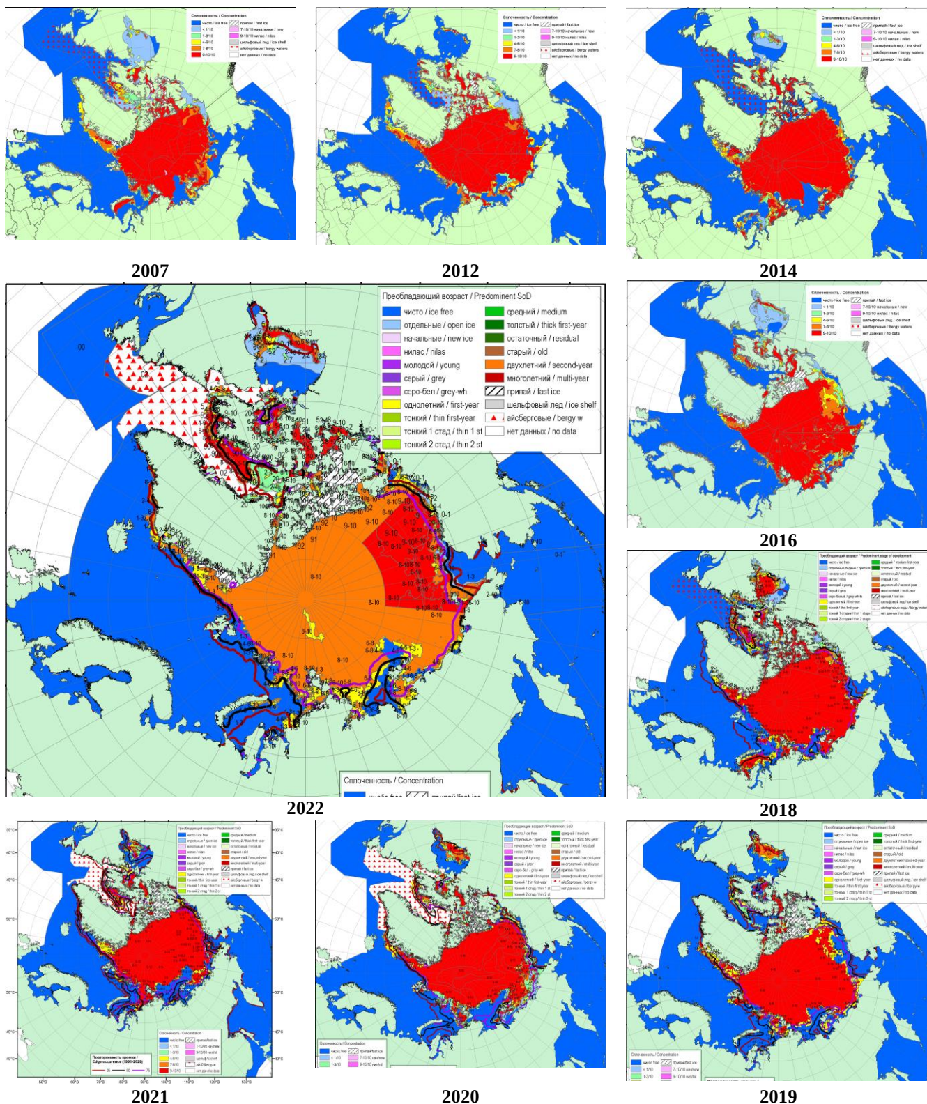
Рисунок 2а – Оценка сплоченности морского льда за 15.07-20.07.2022г. и аналогичные периоды 2007-2021гг. на основе ледового анализа ААНИИ, НИЦ Планета, Канадской ледовой службы и Национального ледового центра США.
