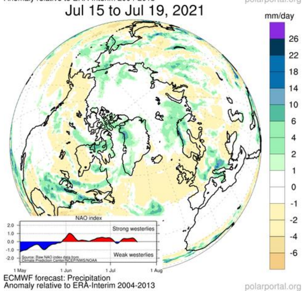
Рисунок 2ж – Аномалии приземной суммы осадков за 15.07 - 19.07 в 2021-2022 гг. относительно периода 2004-2013 гг. ( http://polarportal.dk )
