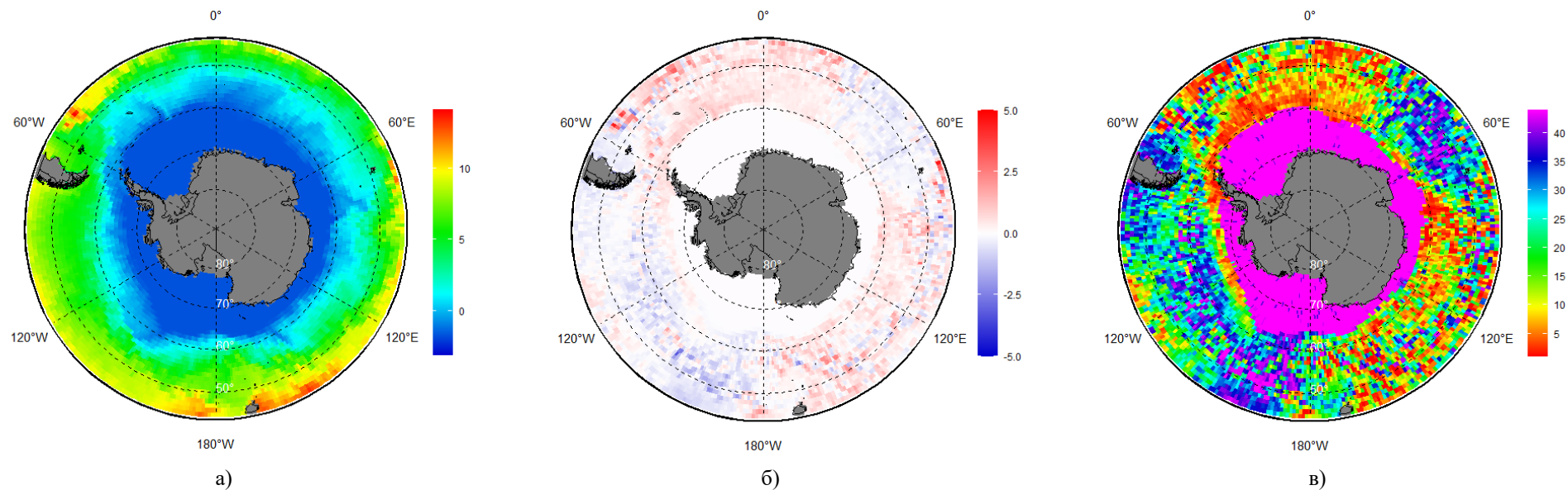
Рисунок 66 – Реанализ ERA5 температуры поверхности воды ( ^{\circ}\text{C} ) за период 08.07 – 14.07.2022 г.г.: (а) – осредненные значения, (б) – аномалия относительно периода 1991-2020 гг. и (в) – ранг за период 1979-2022 гг.
