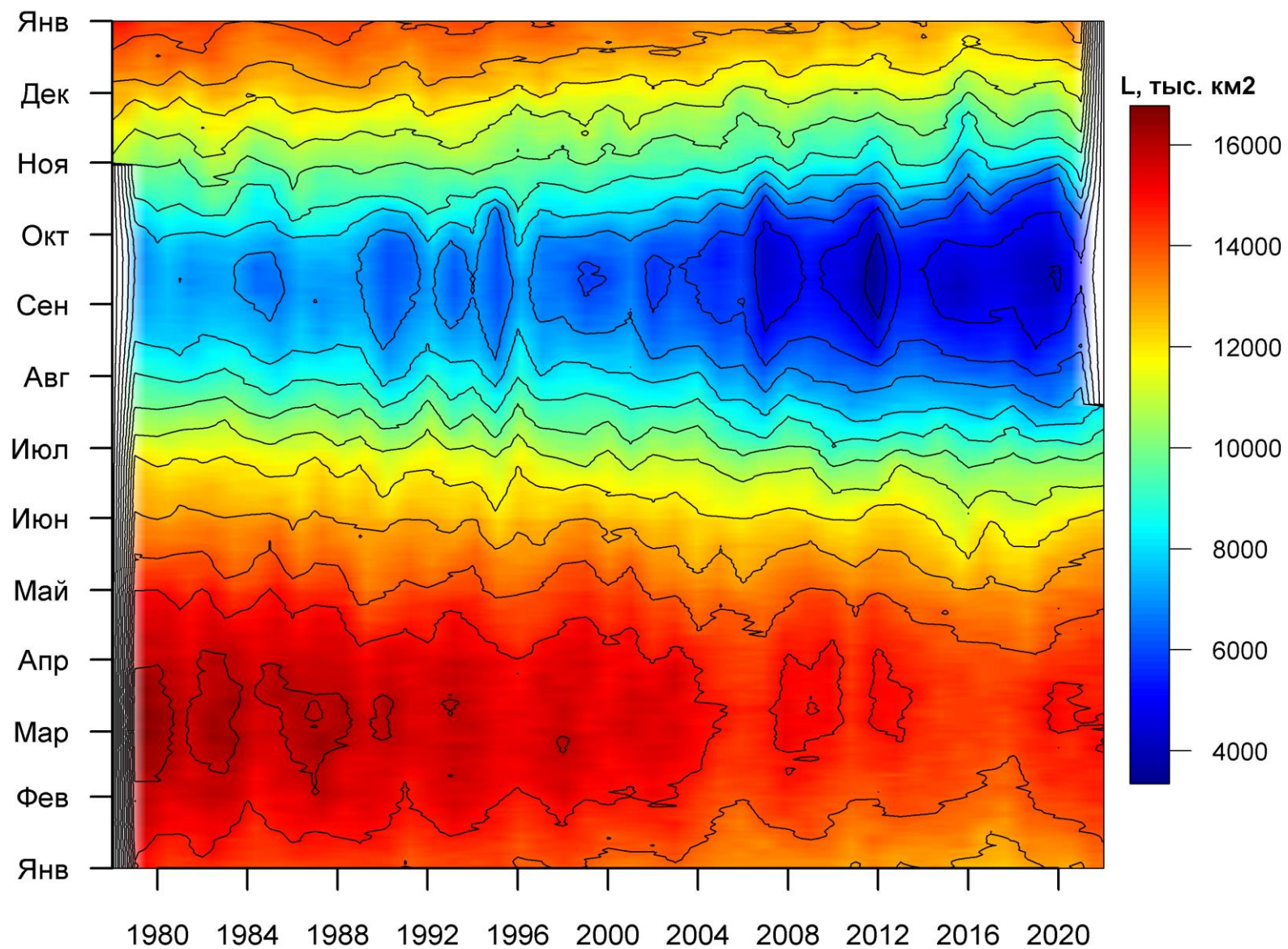
Рисунок 36 – Ежедневные оценки сезонных изменений ледовитости для Северной Полярной Области за период 26.10.1978 – 19.07.2022 на основе расчетов по данным SSMR-SSM/I-SSMIS, алгоритм NASATEAM.
