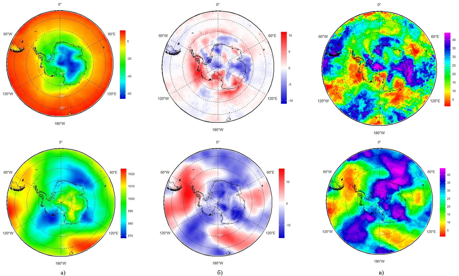
Рисунок 6а – Реанализ ERA5 температуры воздуха на уровне 2м (C°) и атмосферного давления на уровне моря (гПа) за период 08.07 –14.07.2022 г.: (а) -средненные значения, (б) – аномалия относительно периода 1991-2020 гг. и (в) – ранг за период 1979-2022 гг.
