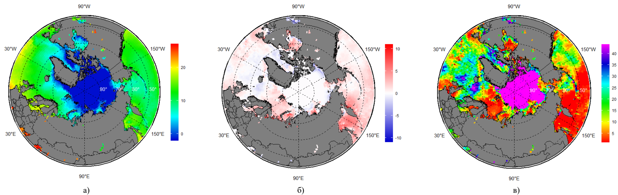
Рисунок 3б – Реанализ ERA5 температуры поверхности воды (C°) за период 08.07 –14.07.2022 г.: (а) – осредненные значения, (б) – аномалия относительно периода 1991-2020 гг. и (в) – ранг за период 1979-2022 гг.
