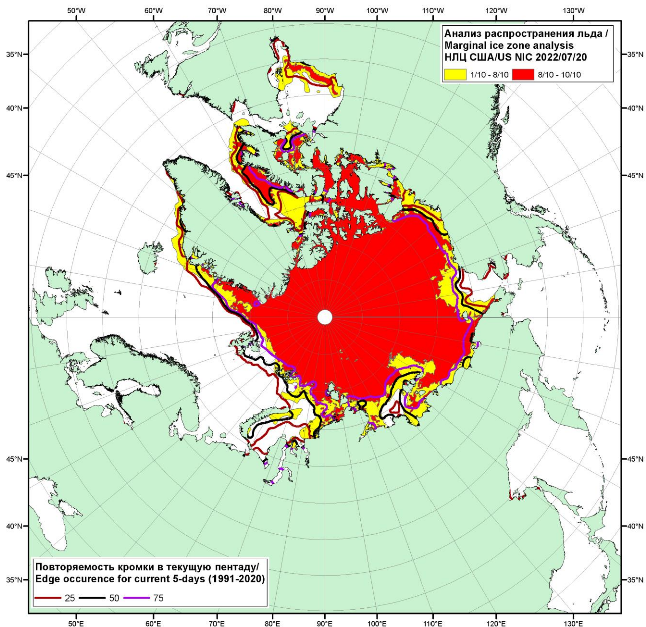
Рисунок 1г – Положение кромки льда и зон разреженных ( <8/10 ) и сплоченных ( \geq 8/10 ) льдов СЛО за 20.07.2022 г. на основе ледового анализа Национального Ледового Центра США и повторяемость кромки за 16-20.07 за период 1991-2020 гг. по наблюдениям SSMR-SSM/I-SSMIS (алгоритм NASATEAM)
