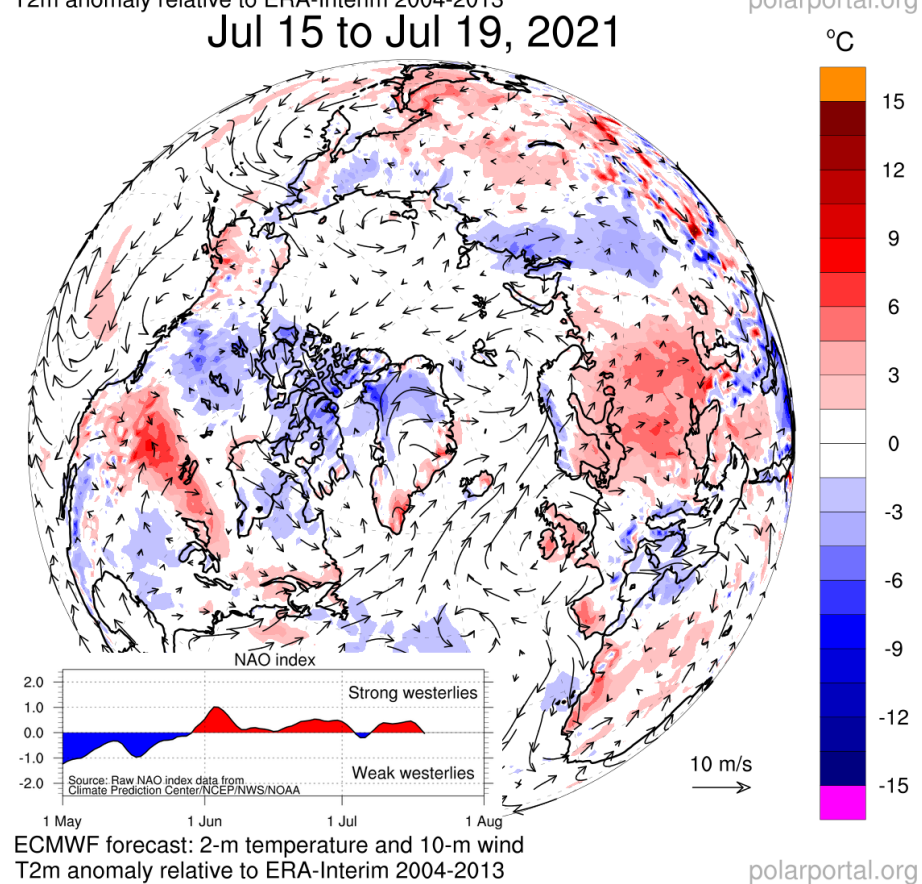
Рисунок 2е – Аномалии приземной температуры воздуха (2м) и осредненные вектора скорости ветра (10 м) за 15.07 - 19.07 в 2021-2022 гг. относительно периода 2004-2013 гг. ( http://polarportal.dk )
