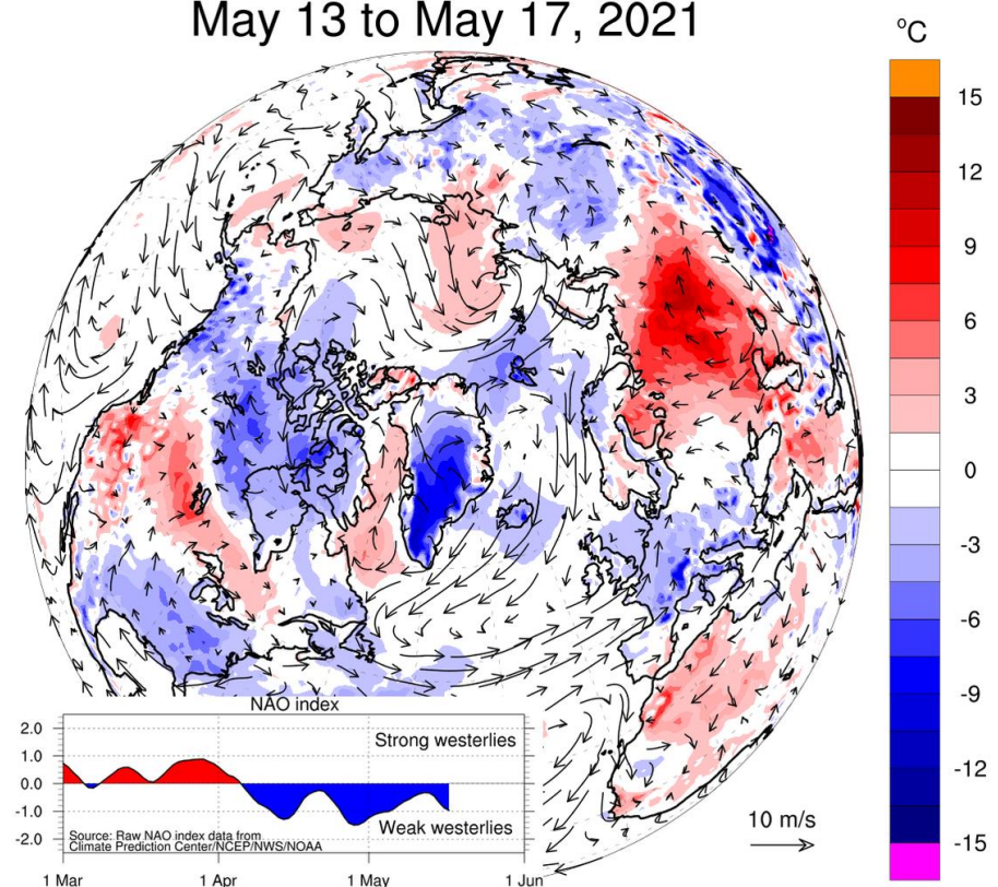
Рисунок 2е – Аномалии приземной температуры воздуха (2м) и осредненные вектора скорости ветра (10 м) за 13.05 - 17.05 в 2021-2022 гг. относительно периода 2004-2013 гг. ( http://polarportal.dk )
