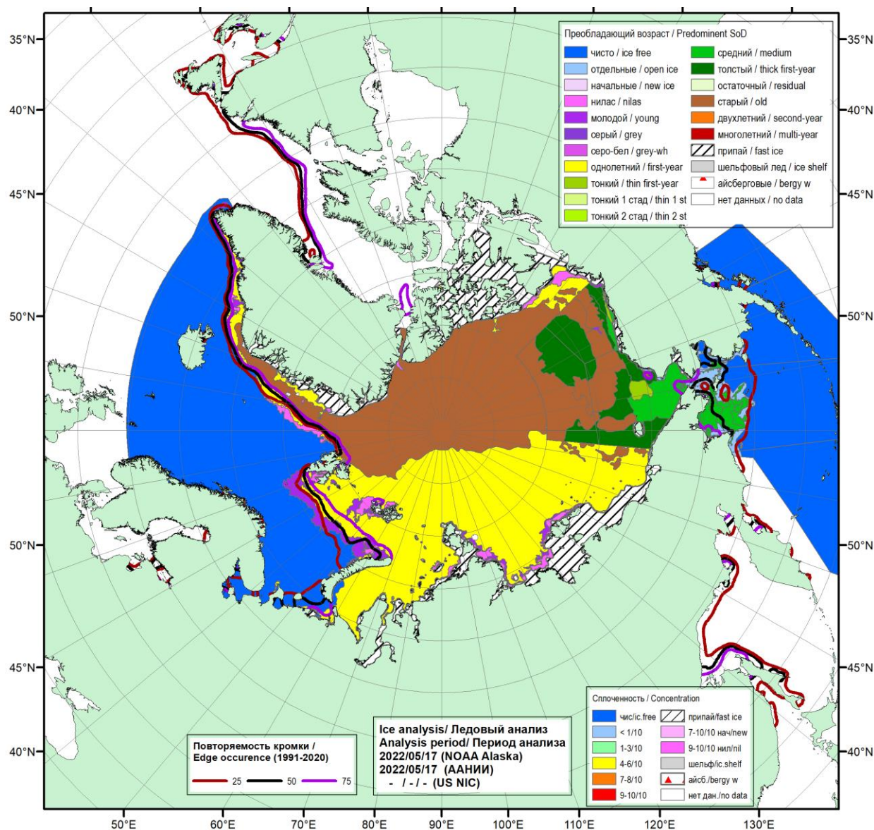
Рисунок 16 – Обзорная ледовая карта САО за 17.05.2022 г. (цветовая раскраска по преобладающему возрасту) на основе ледового анализа ААНИИ (17.05), NOAA Аляска (17.05) и Национального ледового центра США (-.-) и повторяемость кромки за 16-20.05 за период 1991-2020гг. по наблюдениям SSMR-SSM/I-SSMIS (алгоритм NASATEA).
