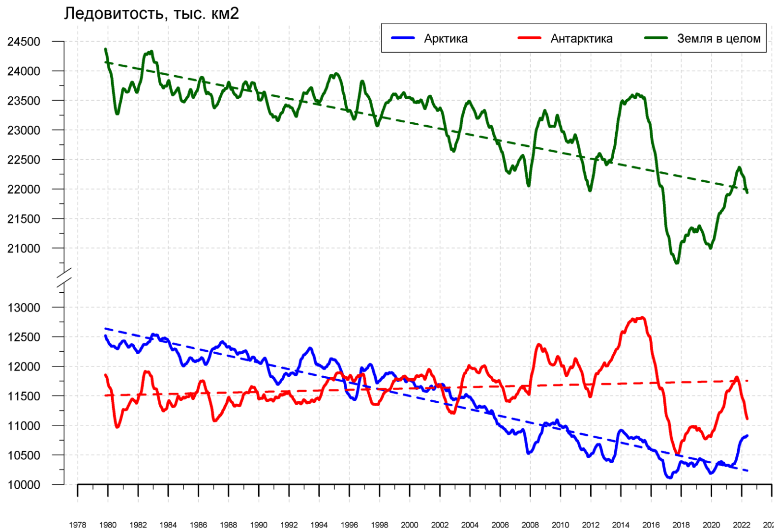
Рисунок 9 – Ежедневные сглаженные окном 365 суток значения ледовитости (площади распространения морского льда) Арктики, Антарктики и Земли в целом с 26.10.1978 по 15.05.2022 на основе SSMR-SSM/I-SSMIS
