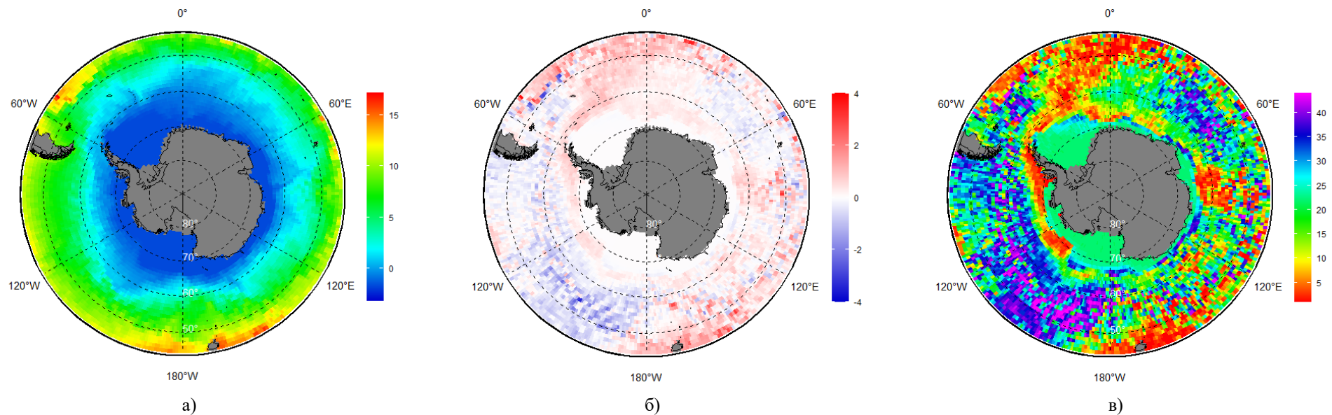
Рисунок 66 – Реанализ ERA5 температуры поверхности воды ( ^{\circ}\text{C} ) за период 05.05 – 11.05.2022 г.: (а) – осредненные значения, (б) – аномалия относительно периода 1991-2020 гг. и (в) – ранг за период 1979-2022 гг.
