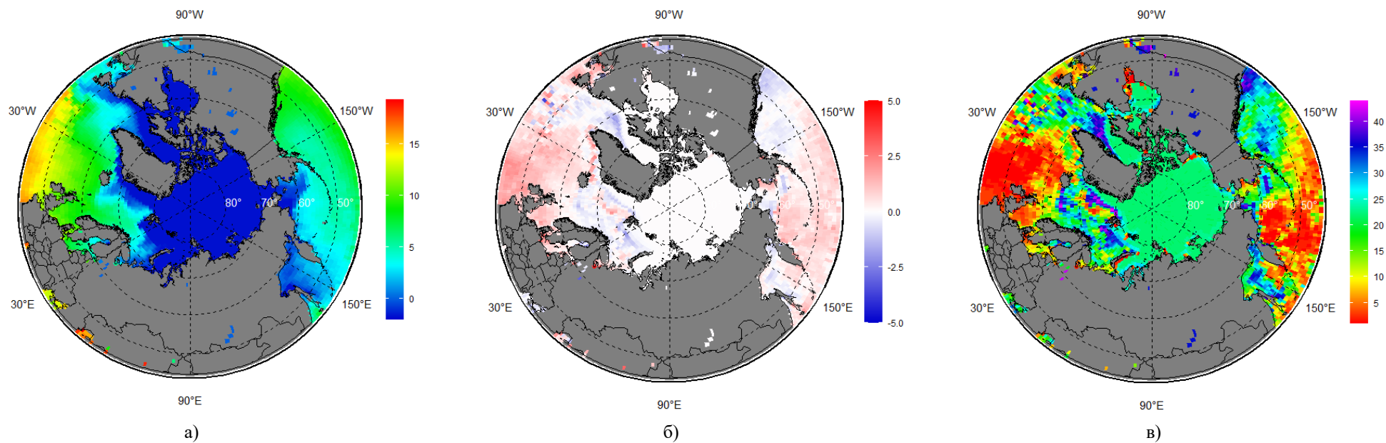
Рисунок 36 – Реанализ ERA5 температуры поверхности воды ( ^{\circ}\text{C} ) за период 05.05 – 11.05.2022 г.: (а) – осредненные значения, (б) – аномалия относительно периода 1991-2020 гг. и (в) – ранг за период 1979-2022 гг.
