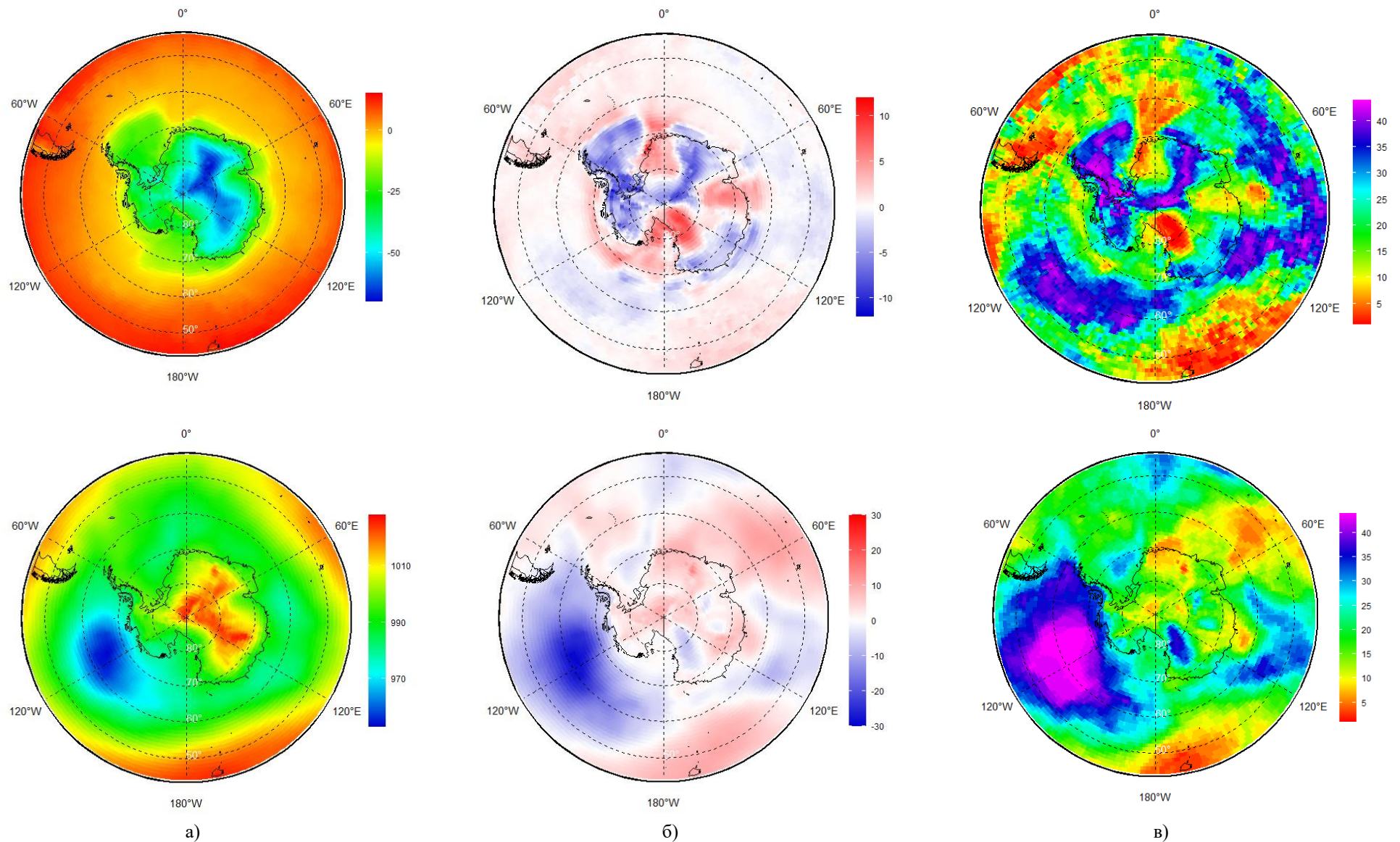
Рисунок 6а – Реанализ ERA5 температуры воздуха на уровне 2м (C°) и атмосферного давления на уровне моря (гПа) за период 05.05 – 11.05.2022 г.: (а) -средненные значения, (б) – аномалия относительно периода 1991-2020 гг. и (в) – ранг за период 1979-2022 гг.
