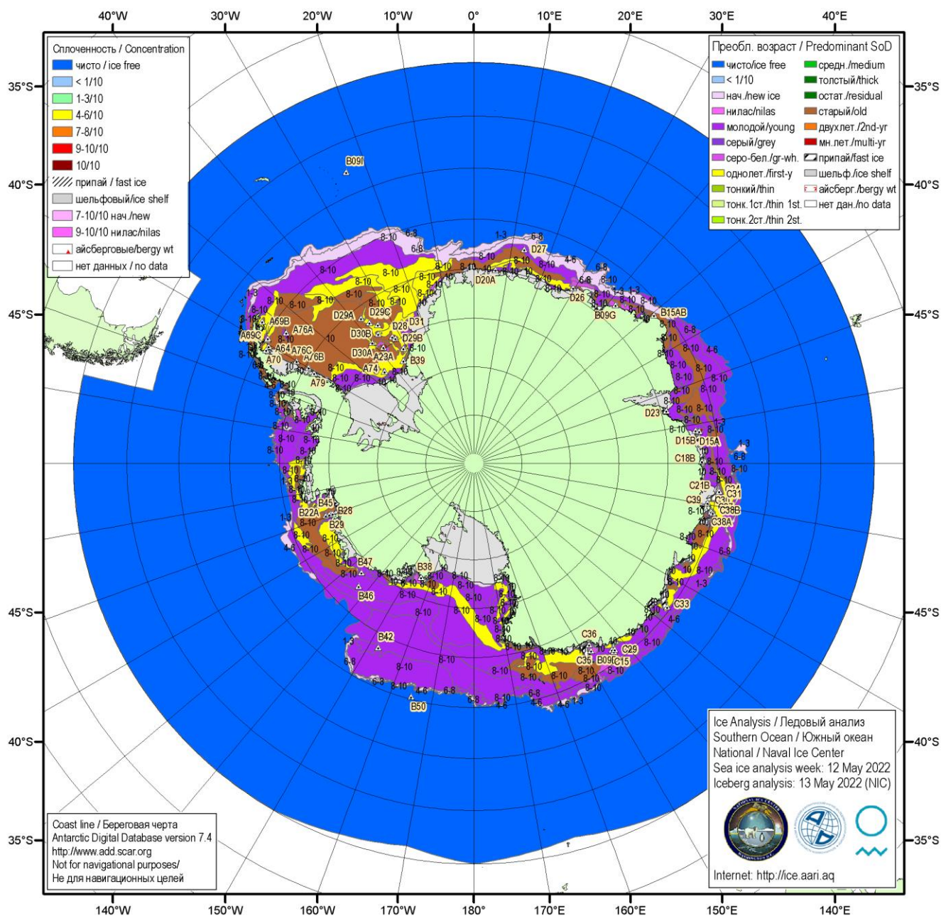
Рисунок 5в – Ледовая карта Южного океана (цветовая окраска по возрасту) и расположение крупных айсбергов на основе ледового анализа ААНИИ за 12.05.2022 в рамках проекта совместного ледового картоирования Южного океана ААНИИ, НЛЦ США и НМИ.
