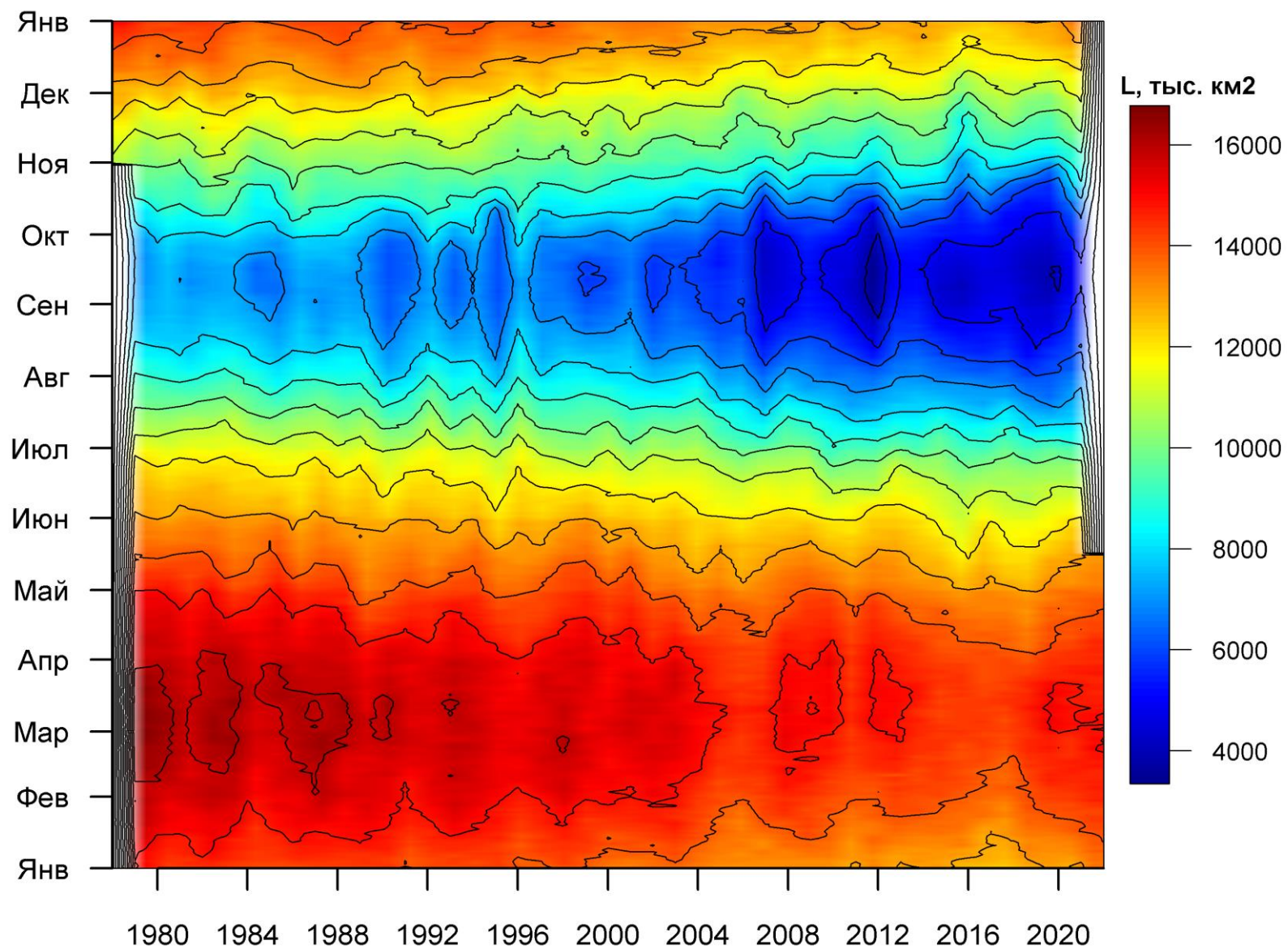
Рисунок 36 – Ежедневные оценки сезонных изменений ледовитости для Северной Полярной Области за период 26.10.1978 – 15.05.2022 на основе расчетов по данным SSMR-SSM/I-SSMIS, алгоритм NASATEAM.
