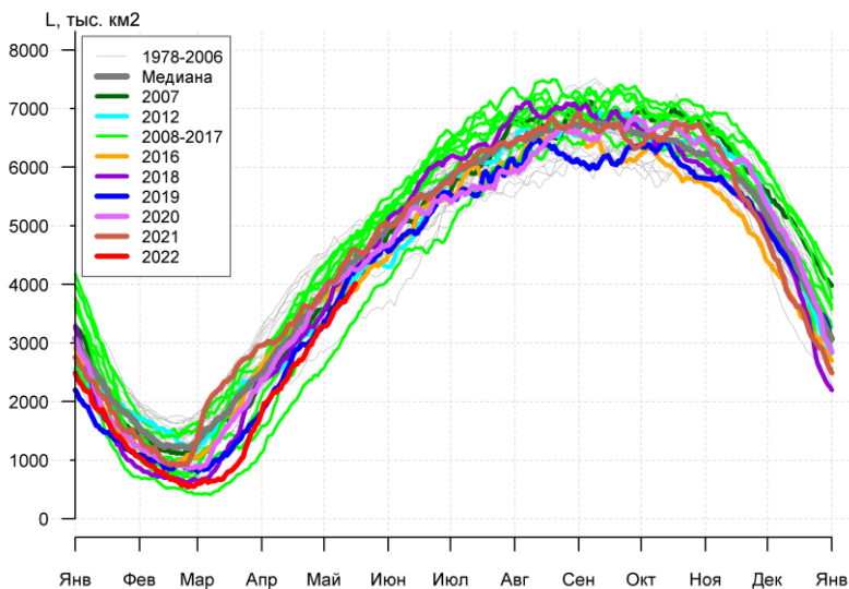
Рисунок 7а – Ежедневные оценки сезонного хода ледовитости Южного Океана и меридиональных секторов за период 26.10.1978 – 15.05.2022 по годам на основе расчетов по данным SSMR-SSM/I-SSMIS, алгоритм NASATEAM: а) Южный Океан, б) Атлантический сектор (60°W-30°E, море Уэдделла), в) Индоокеанский сектор (30°E-150°E, моря Космонавтов, Содружества, Моусона), г) Тихоокеанский сектор (150°E-60°W, моря Росса, Беллинсгаузена)
