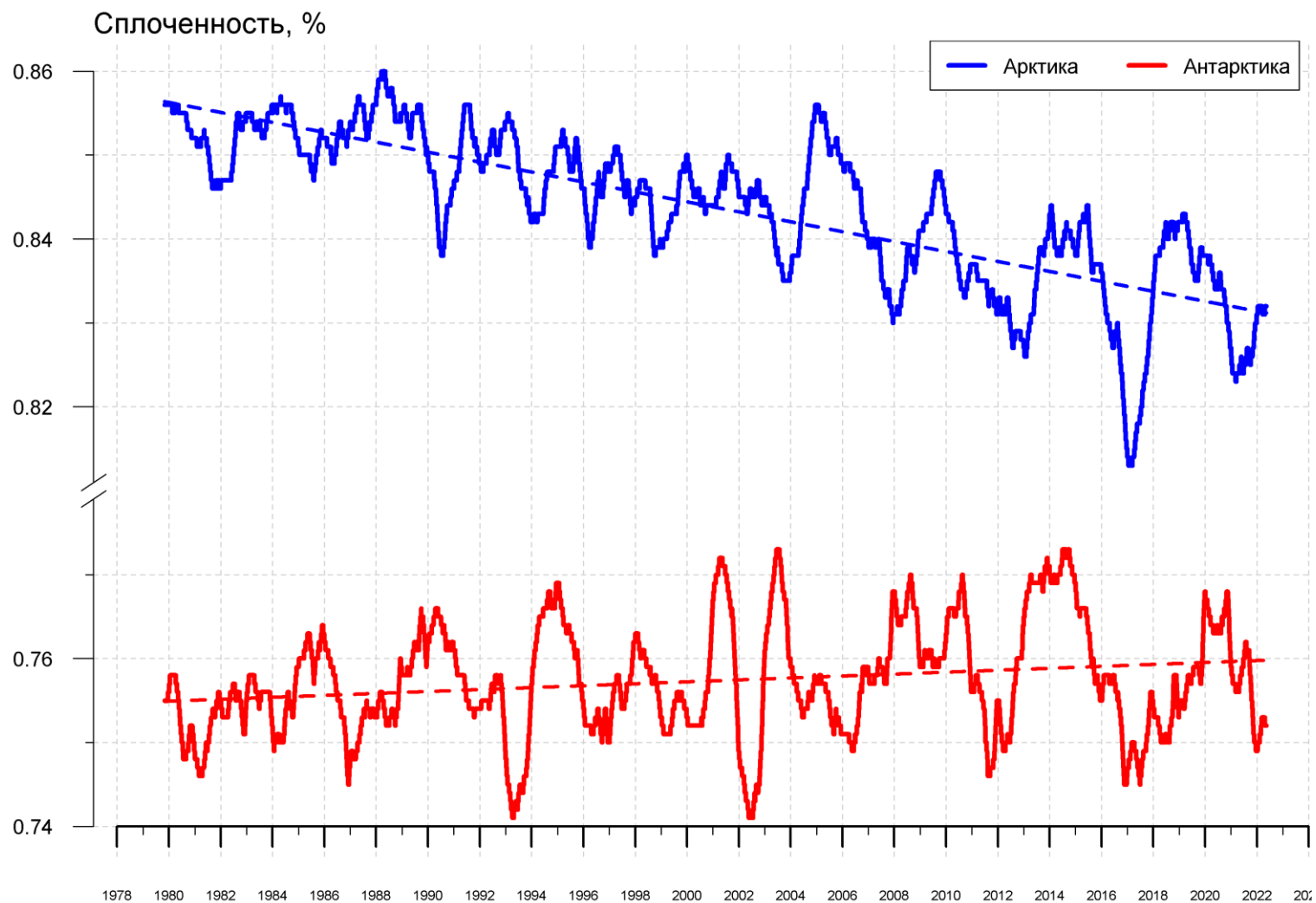
Рисунок 11 – Ежедневные сглаженные окном 365 суток значения средней общей сплоченности Арктики и Антарктики с 07.11.1978 по 15.05.2022 на основе SSMR-SSM/I-SSMIS
