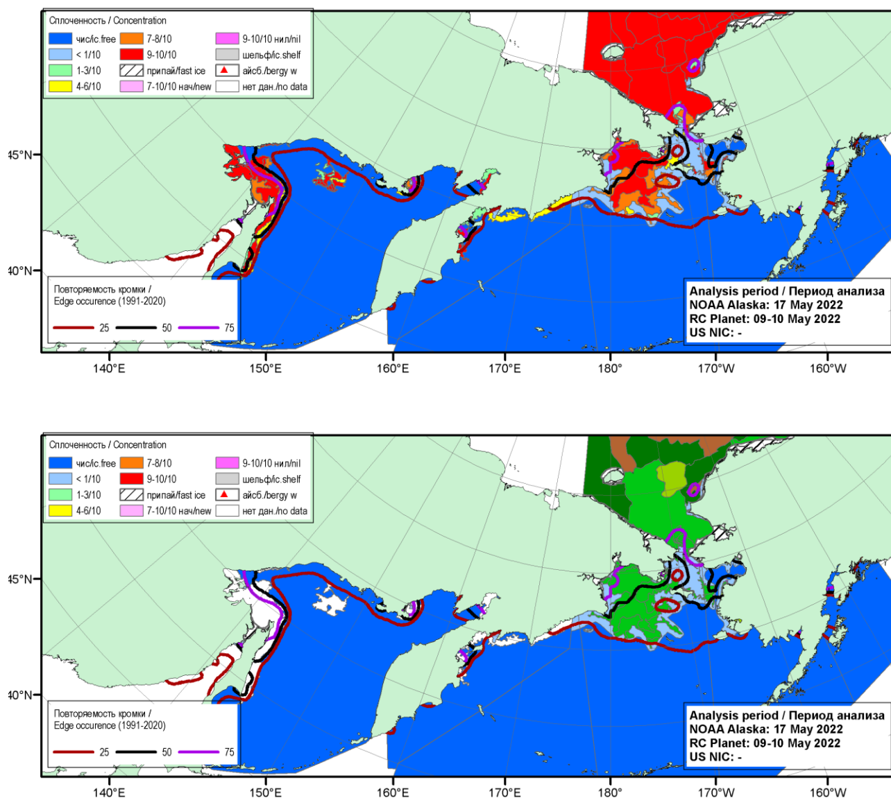
Рисунок 16 – Ледовая карта Японского – Берингово и Чукотского морей (цветовая окраска по общей сплоченности – верх и преобладающему возрасту - низ) на основе информации НОАА Аляска (17.05), НИЦ Планета (09-10.05), и повторяемость кромки за 11-15.05 за период 1991-2020 гг. по наблюдениям SSMR-SSM/I-SSMIS (алгоритм NASATEAM).
