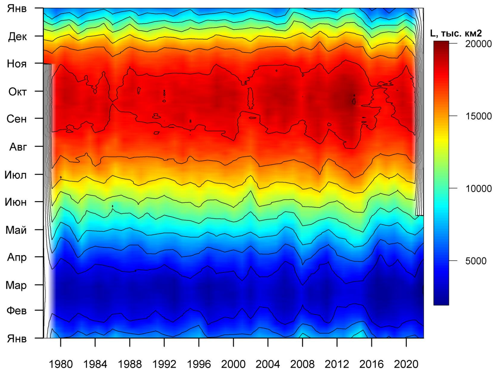
Рисунок 76 – Ежедневные оценки сезонных изменений ледовитости для Южного океана за период 26.10.1978 – 15.05.2022 на основе расчетов по данным SSMR-SSM/I-SSMIS, алгоритм NASATEAM.
