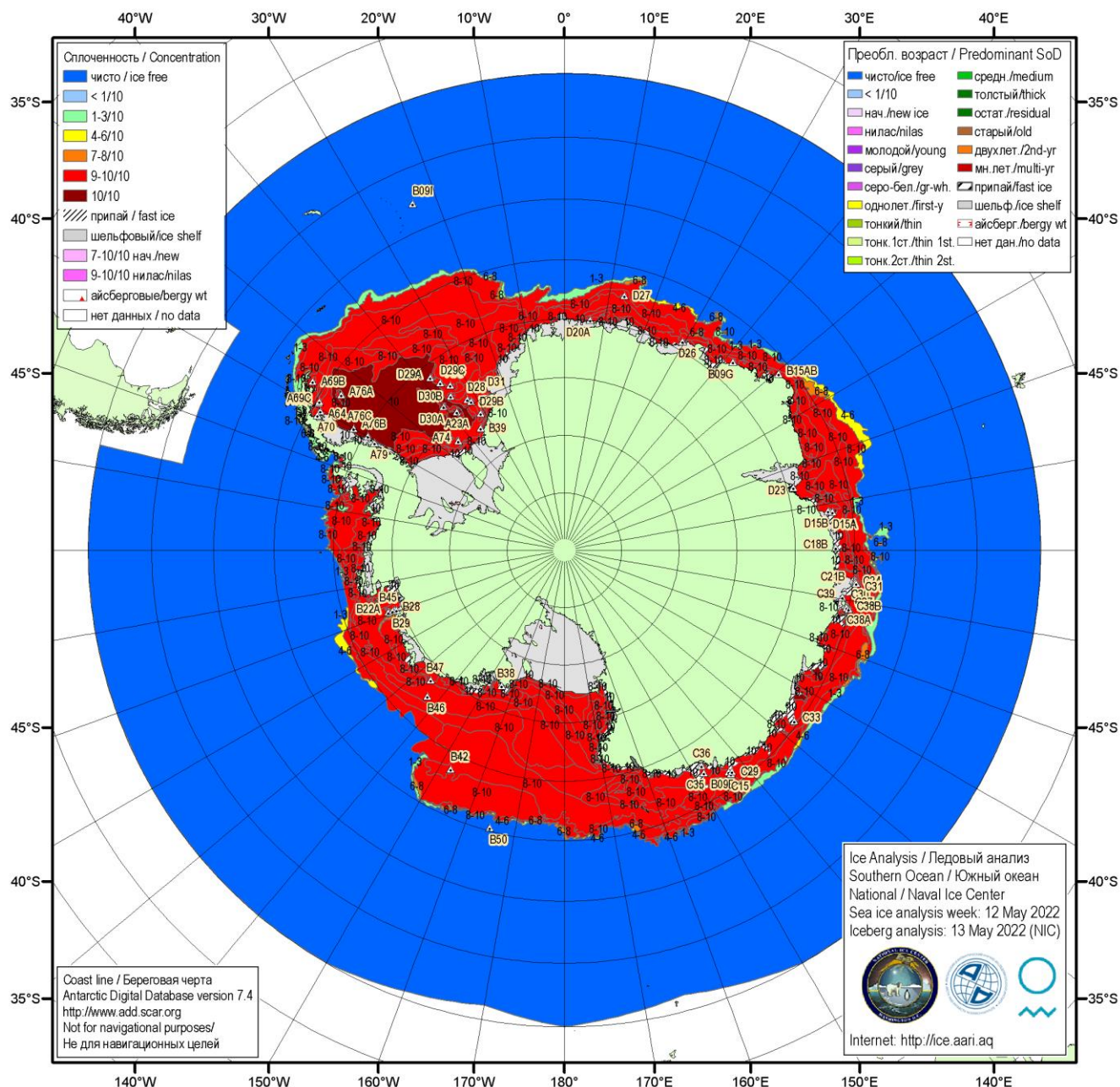
Рисунок 5а – Ледовая карта Южного океана (цветовая окраска по общей сплоченности) и расположение крупных айсбергов на основе ледового анализа ААНИИ за 12.05.2022 в рамках проекта совместного ледового картирования Южного океана ААНИИ, НЛЦ США и НМИ.
