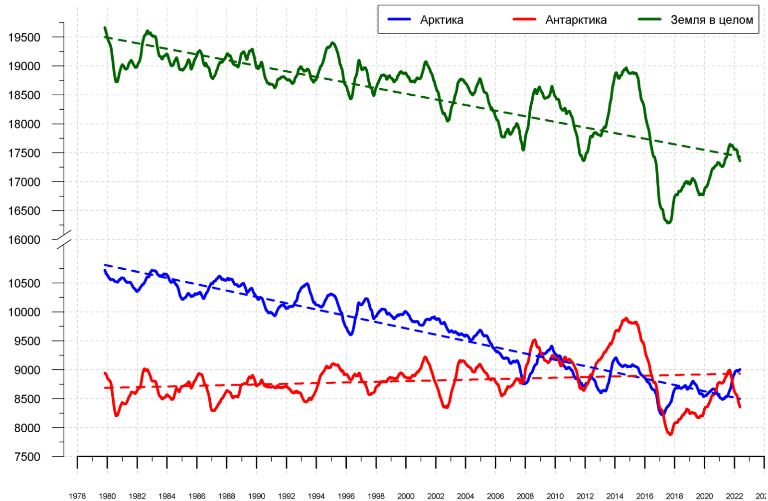
Рисунок 10 – Ежедневные сглаженные окном 365 суток значения приведенной ледовитости (площади морского льда) Арктики, Антарктики и Земли в целом с 26.10.1978 по 15.05.2022 на основе SSMR-SSM/I-SSMIS
