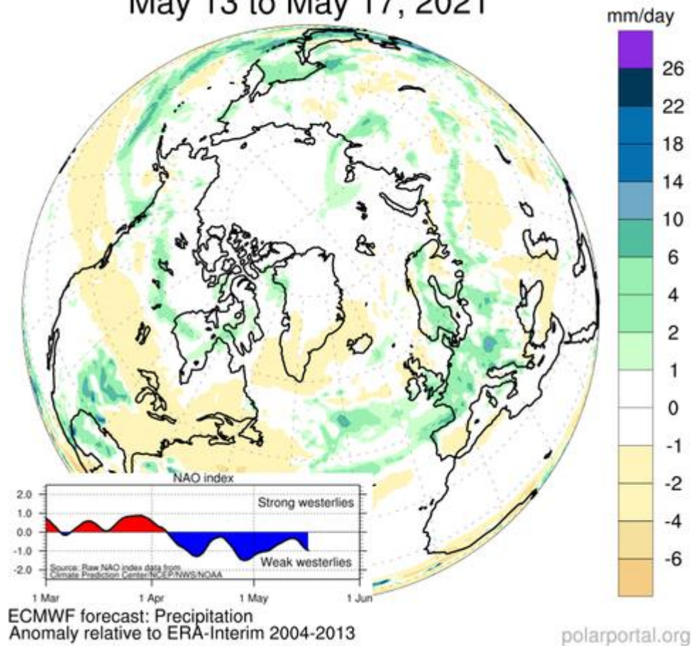
Рисунок 2ж – Аномалии приземной суммы осадков за 13.05 - 17.05 в 2021-2022 гг. относительно периода 2004-2013 гг. ( http://polarportal.dk )
