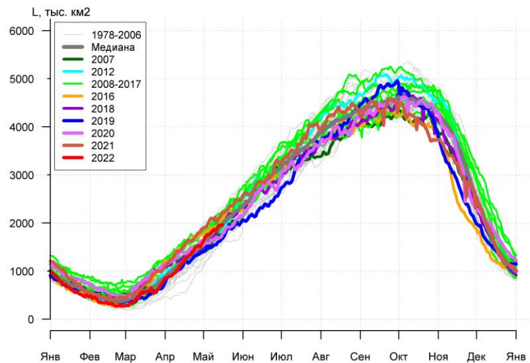
Рисунок 7а – Ежедневные оценки сезонного хода ледовитости Южного Океана и меридиональных секторов за период 26.10.1978 – 15.05.2022 по годам на основе расчетов по данным SSMR-SSM/I-SSMIS, алгоритм NASATEAM: а) Южный Океан, б) Атлантический сектор (60°W-30°E, море Уэдделла), в) Индоокеанский сектор (30°E-150°E, моря Космонавтов, Содружества, Моусона), г) Тихоокеанский сектор (150°E-60°W, моря Росса, Беллинсгаузена)
