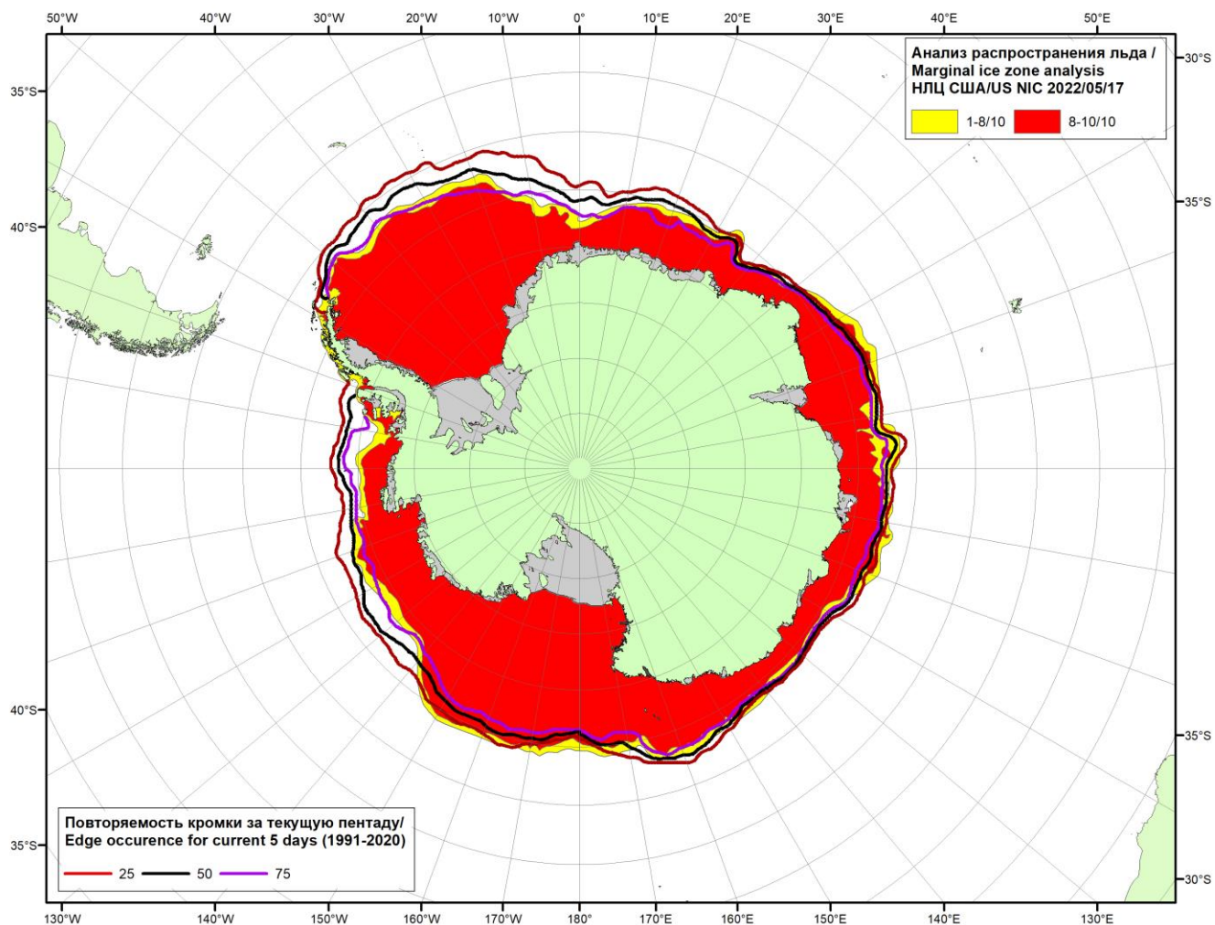
Рисунок 5в – Положение кромки льда и зон разреженных ( <8/10 ) и сплоченных ( \geq 8/10 ) льдов Южного океана за 17.05.2022 г. на основе ледового анализа Национального Ледового Центра США и повторяемость кромки за 16-20.05 за период 1991-2020 гг. по наблюдениям SSMR-SSM/I-SSMIS (алгоритм NASATEAM).
