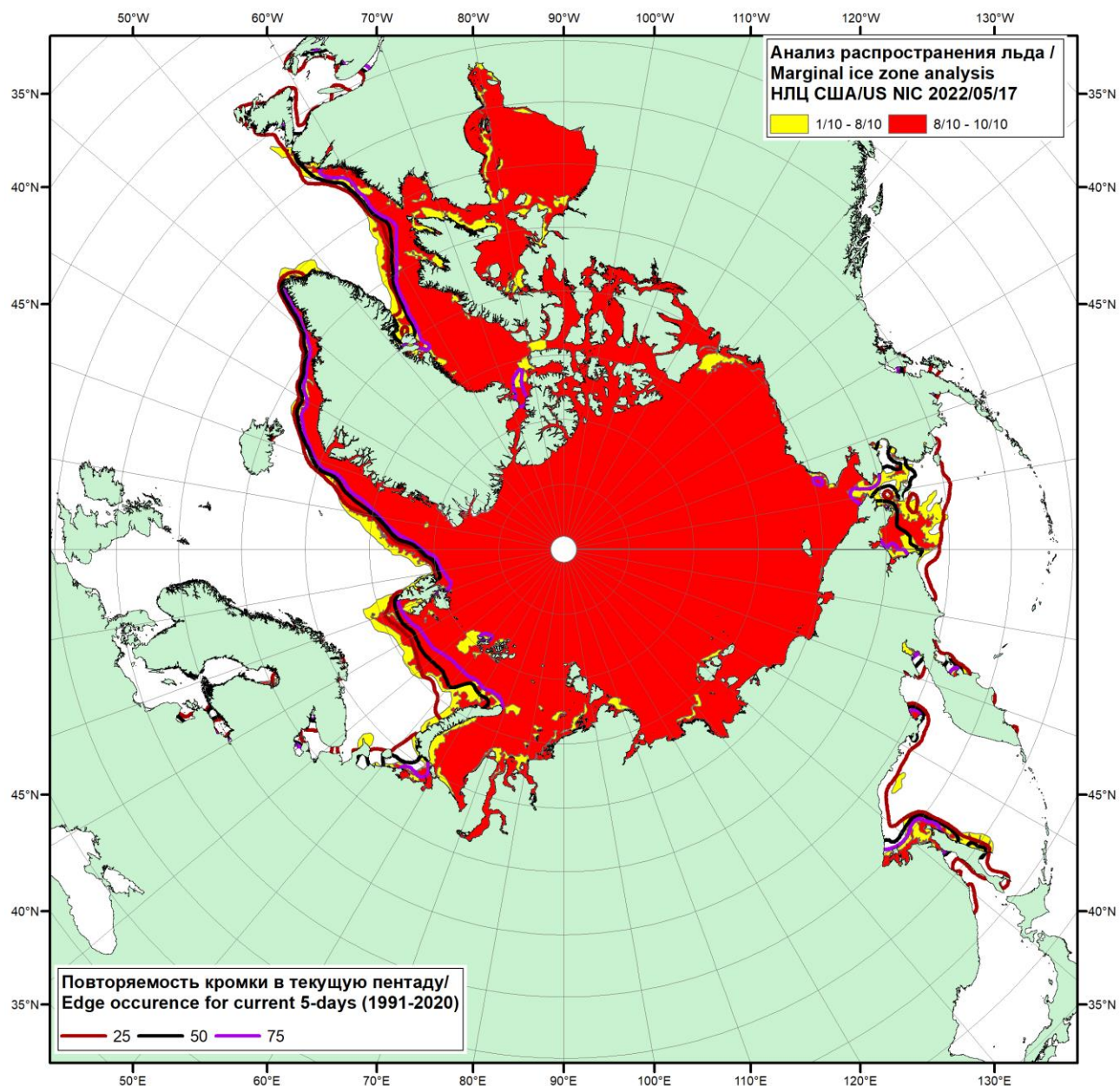
Рисунок 1в – Положение кромки льда и зон разреженных ( <8/10 ) и сплоченных ( \geq 8/10 ) льдов СЛО за 17.05.2022 г. на основе ледового анализа Национального Ледового Центра США и повторяемость кромки за 16.05-20.05 за период 1991-2020 гг. по наблюдениям SSMR-SSM/I-SSMIS (алгоритм NASATEAM)
