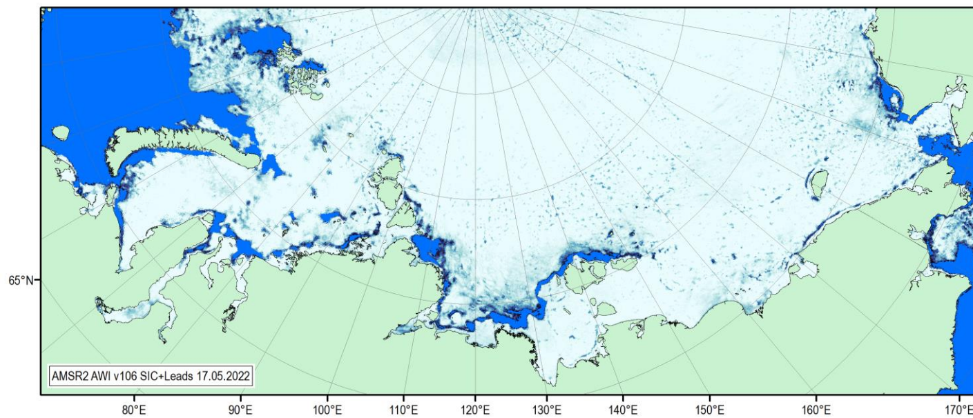
Рисунок 1г – Оценка сплоченности льда и расположения полыней по данным ИСЗ AMSR2 за 17.05.2022.
