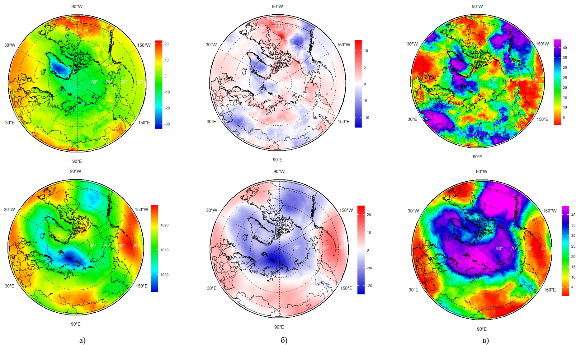
Рисунок 3а – Реанализ ERA5 температуры воздуха на уровне 2м (C°) и атмосферного давления на уровне моря (гПа) за период 05.05 – 11.05.2022 г.г.: (а) – осредненные значения, (б) – аномалия относительно периода 1991-2020 гг. и (в) – ранг за период 1979-2022 гг.
