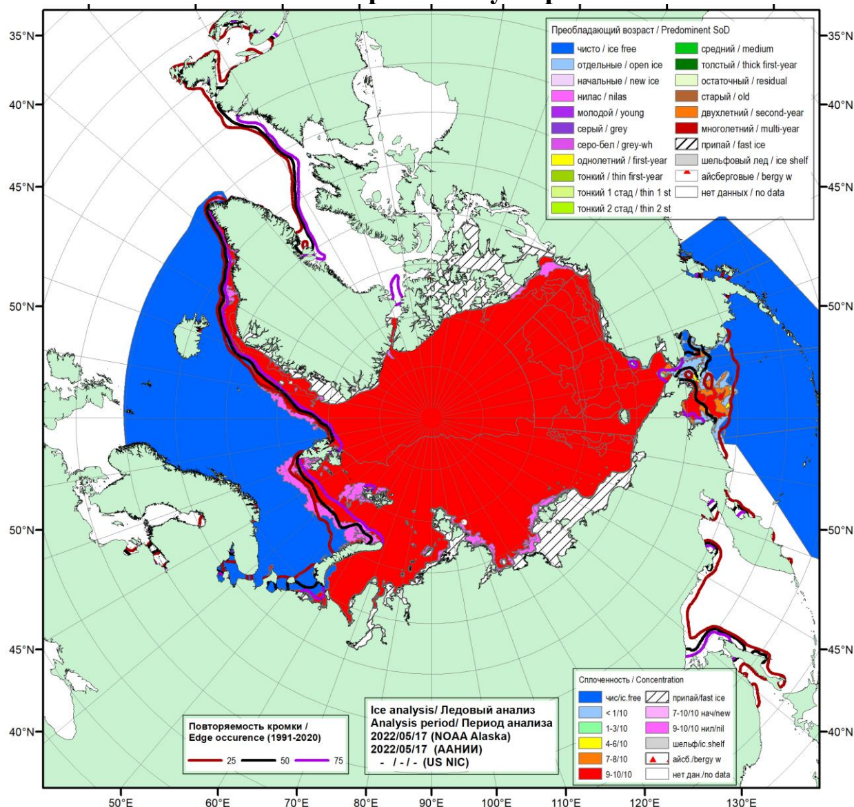
Рисунок 1а – Обзорная ледовая карта СЛО за 17.05.2022 г. (цветовая раскраска по общей сплоченности) на основе ледового анализа ААНИИ (17.05), NOAA Аляска (17.05) и Национального ледового центра США (-,-) и повторяемость кромки за 16-20.05 за период 1991-2020гг. по наблюдениям SSMR-SSM/I-SSMIS (алгоритм NASATEAM).
