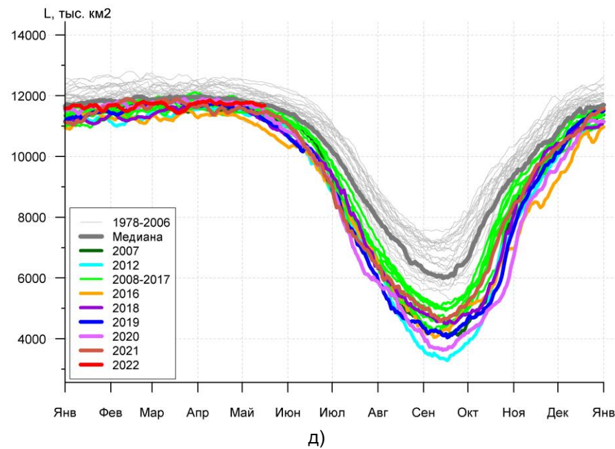
Рисунок 3а – Ежедневные оценки сезонного хода ледовитости для Северной Полярной Области и трех меридиональных секторов за период 26.10.1978 - 15.05.2022 по годам на основе расчетов по данным SSMR-SSM/I-SSMIS, алгоритмы NASATEAM: а) Северная полярная область, б) сектор 45°W-95°E (Гренландское – Карское моря), в) сектор 95°E-170°W (моря Лаптевых – Чукотское и Берингово, Охотское), г) сектор 170°W-45°W (море Бофорта и Канадская Арктика), д) Северный Ледовитый океан, е) Северный морской путь (Карское - Чукотское моря).
