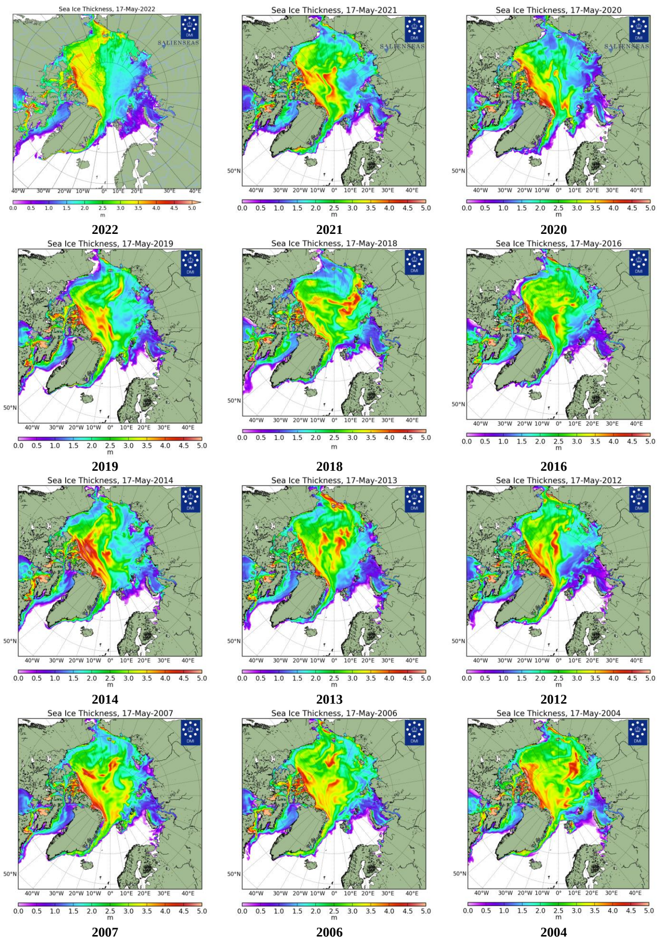
Рисунок 26 – Поля распределения средневзвешенной толщины льда совместной модели морского льда – океана NUCOM/CICE Датского метеорологического института 17.05 за 2004-2022 гг.
