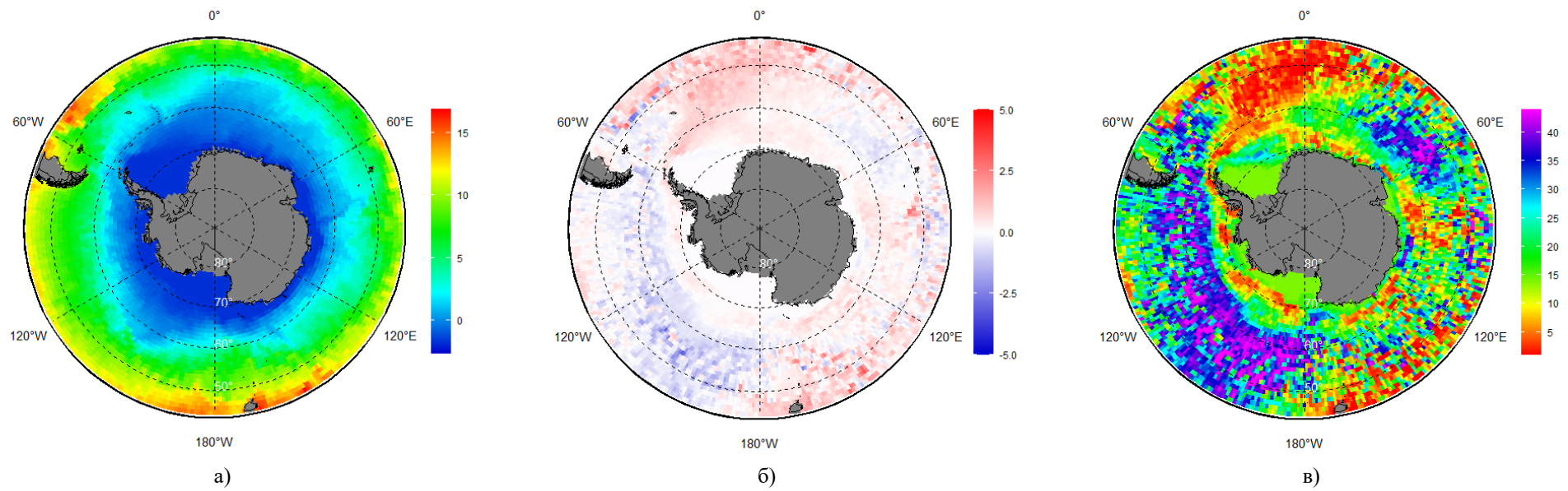
Рисунок 66 – Реанализ ERA5 температуры поверхности воды (C°) за период 14.04 – 20.04.2022г.: (а) – осредненные значения, (б) – аномалия относительно периода 1991-2020 гг. и (в) – ранг за период 1979-2022 гг.
