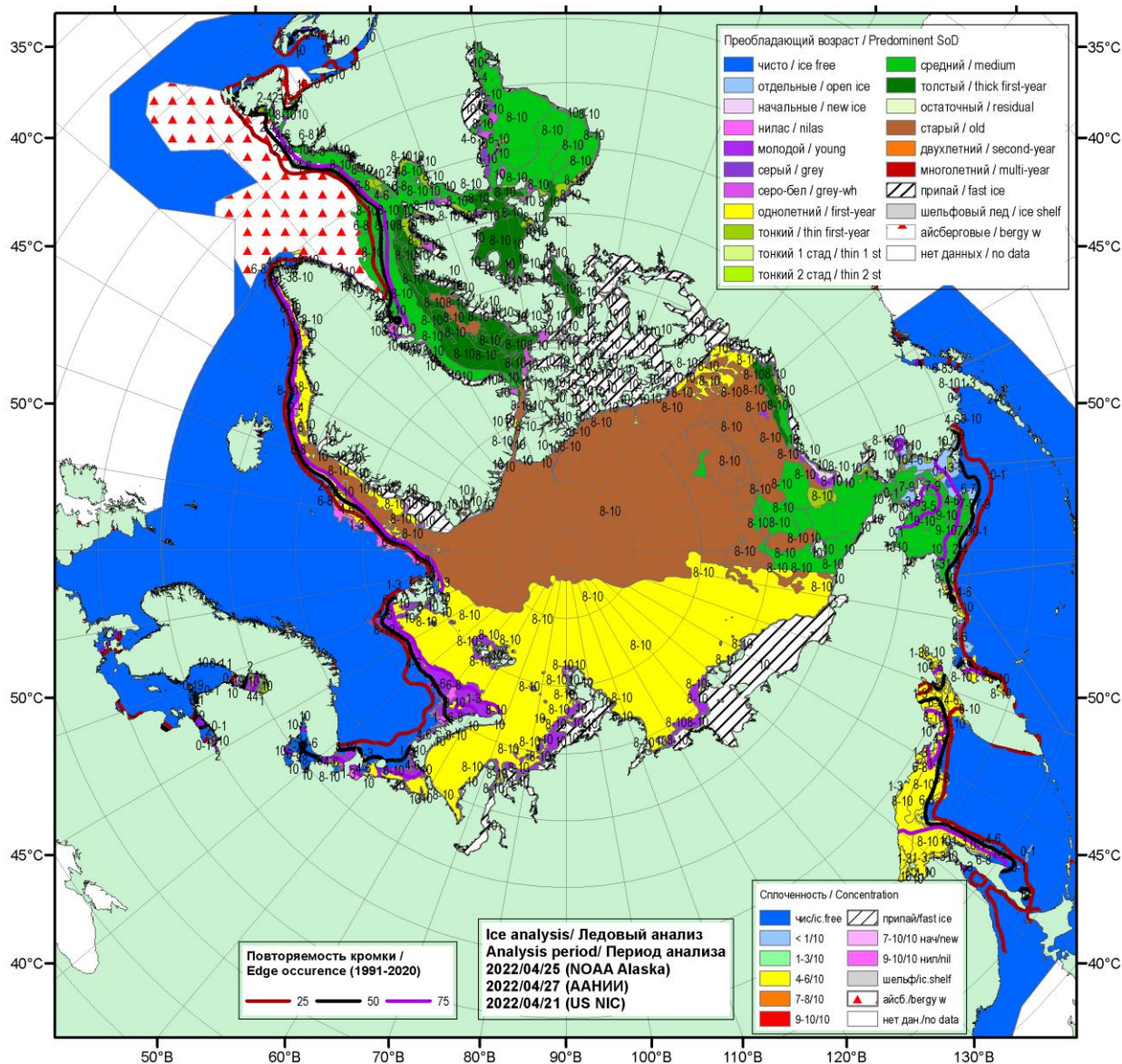
Рисунок 16 – Обзорная ледовая карта СЮ за 21.04-27.04.2022 г. (цветовая раскраска по преобладающему возрасту) на основе ледового анализа ААНИИ (26.04), NOAA Аляска (25.04) и Национального ледового центра США (21.04) и повторяемость кромки за 26-30.04 за период 1991-2020гг. по наблюдениям SSMR-SSM/I-SSMIS (алгоритм NASATEAM).
