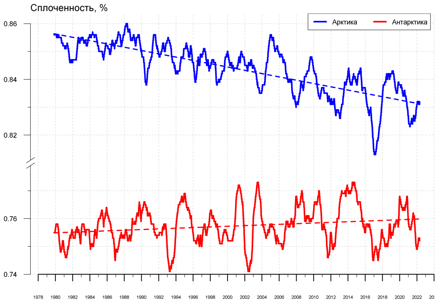
Рисунок 11 – Ежедневные сглаженные окном 365 суток значения средней общей сплоченности Арктики и Антарктики с 07.11.1978 по 24.04.2022 на основе SSMR-SSM/I-SSMIS
