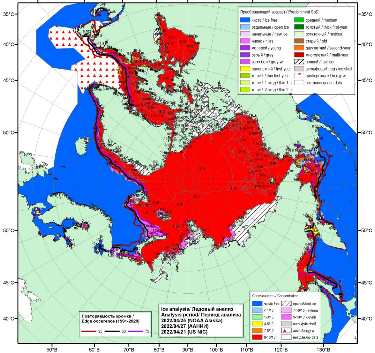
Рисунок 1а – Обзорная ледовая карта СЛЮ за 21.04-26.04.2022 г. (цветовая раскраска по общей сплоченности) на основе ледового анализа ААНИИ (27.04), NOAA Аляска (25.04) и Национального ледового центра США (21.04) и повторяемость кромки за 26-30.04 за период 1991-2020гг. по наблюдениям SSMR-SSM/I-SSMIS (алгоритм NASATEAM).
