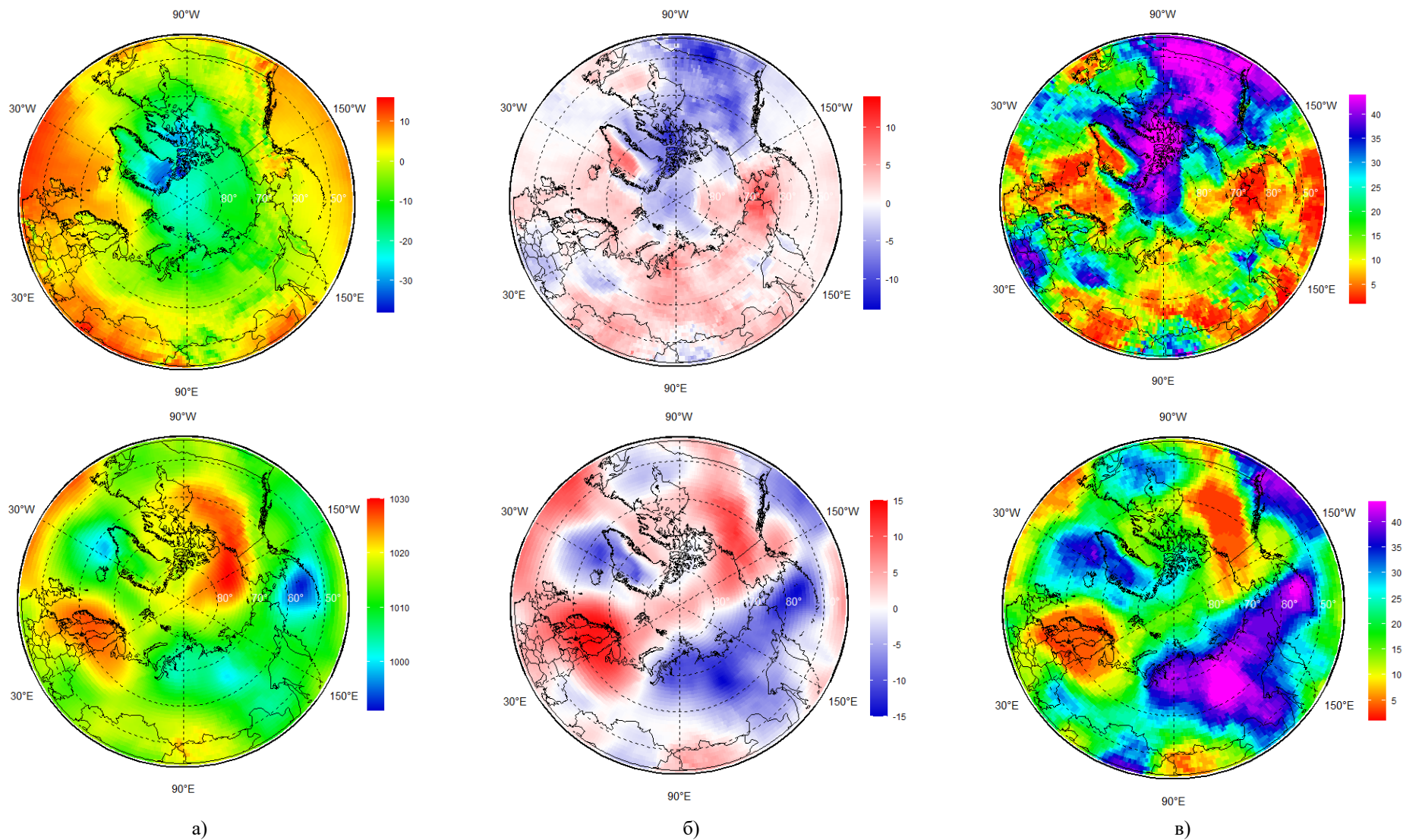
Рисунок 3а – Реанализ ERA5 температуры воздуха на уровне 2м (C°) и атмосферного давления на уровне моря (гПа) за период 14.04 – 20.04.2022 г.: (а) – осредненные значения, (б) – аномалия относительно периода 1991-2020 гг. и (в) – ранг за период 1979-2022 гг.
