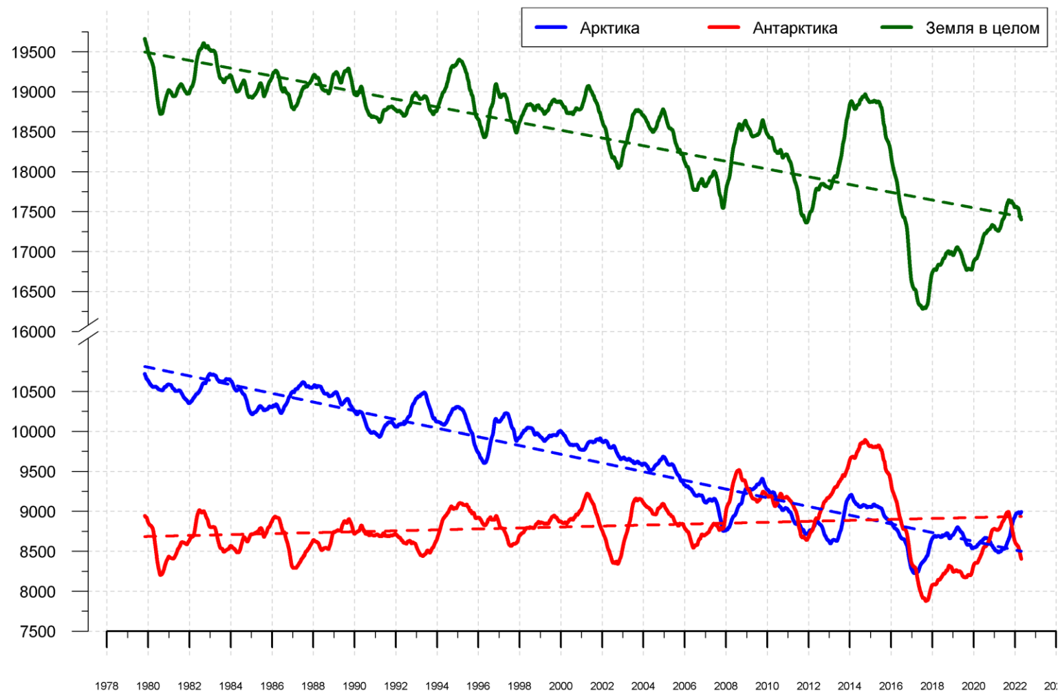
Рисунок 10 – Ежедневные сглаженные окном 365 суток значения приведенной ледовитости (площади морского льда) Арктики, Антарктики и Земли в целом с 26.10.1978 по 24.04.2022 на основе SSMR-SSM/I-SSMIS
