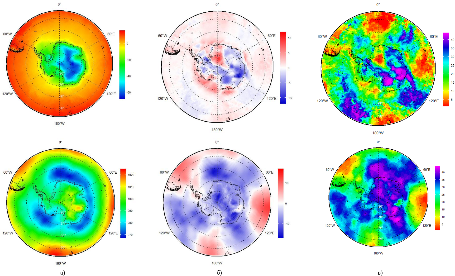
Рисунок ба – Реанализ ERA5 температуры воздуха на уровне 2м (C°) и атмосферного давления на уровне моря (гПа) за период 14.04 – 20.04.2022 г.: (а) -средненные значения, (б) – аномалия относительно периода 1991-2020 гг. и (в) – ранг за период 1979-2022 гг.
