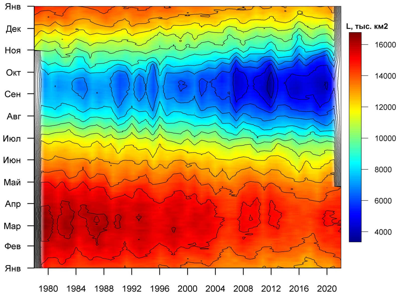
Рисунок 3б – Ежедневные оценки сезонных изменений ледовитости для Северной Полярной Области за период 26.10.1978 – 24.04.2022 на основе расчетов по данным SSMR-SSM/I-SSMIS, алгоритм NASATEAM.
