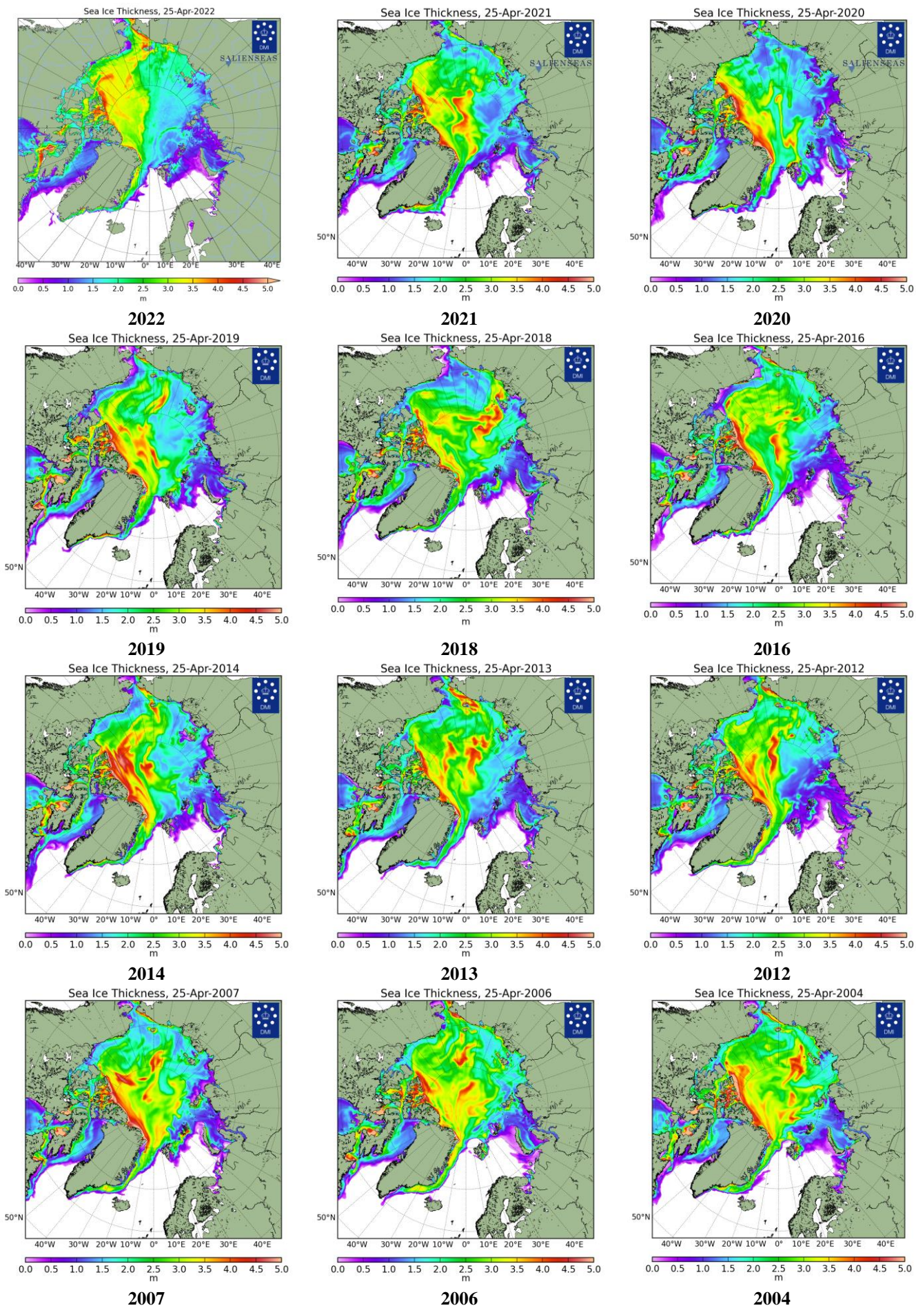
Рисунок 26 – Поля распределения средневзвешенной толщины льда совместной модели морского льда – океана НУСOM/СICE Датского метеорологического института 25.04 за 2004-2022 гг.
