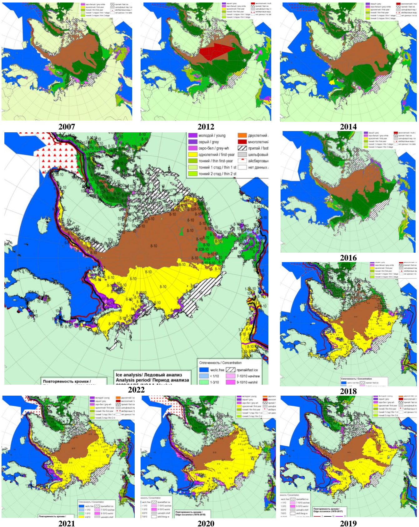
Рисунок 2а – Оценка сплоченности морского льда за 21.04-27.04.2022г. и аналогичные периоды 2007-2020гг. на основе ледового анализа ААНИИ, НИЦ Планета, Канадской ледовой службы и Национального ледового центра США.
