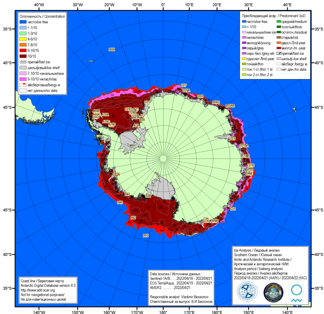
Рисунок 5а – Ледовая карта Южного океана (цветовая окраска по общей сплоченности) и расположение крупных айсбергов на основе ледового анализа ААНИИ за 21.04.2022 в рамках проекта совместного ледового картирования Южного океана ААНИИ, НЛЦ США и НМИ.
