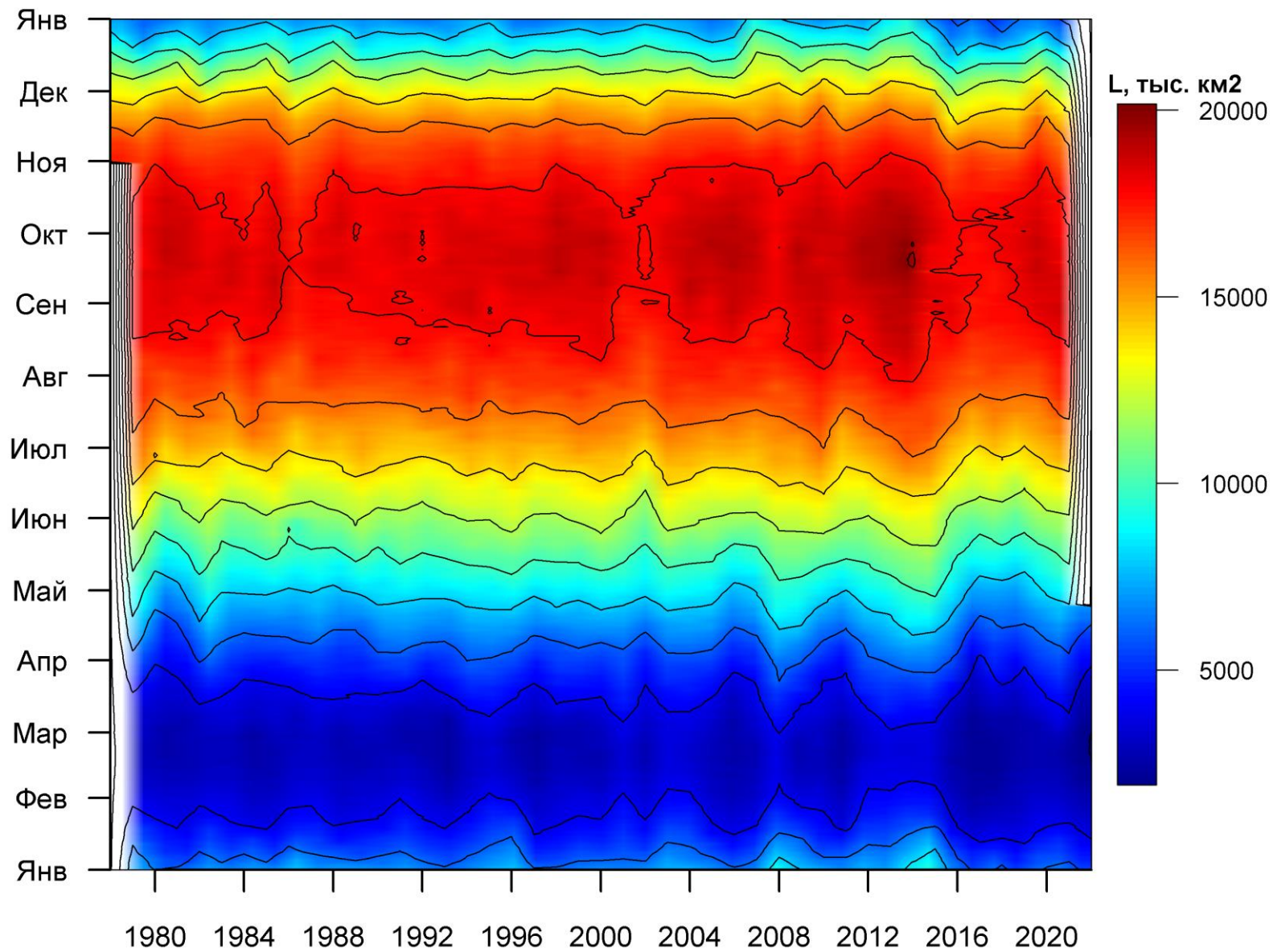
Рисунок 76 – Ежедневные оценки сезонных изменений ледовитости для Южного океана за период 26.10.1978 – 24.04.2022 на основе расчетов по данным SSMR-SSM/I-SSMIS, алгоритм NASATEAM.
