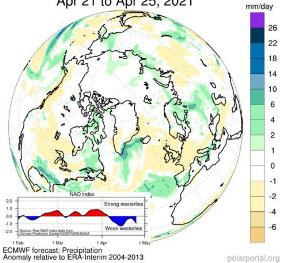
Рисунок 2ж – Аномалии приземной суммы осадков за 21.04 - 25.04 в 2021-2022 гг. относительно периода 2004-2013 гг. ( http://polarportal.dk )
