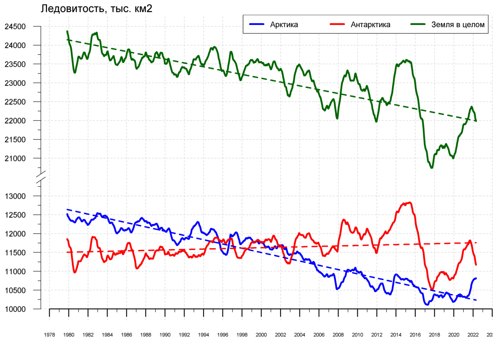
Рисунок 9 – Ежедневные сглаженные окном 365 суток значения ледовитости (площади распространения морского льда) Арктики, Антарктики и Земли в целом с 26.10.1978 по 24.04.2022 на основе SSMR-SSM/I-SSMIS
