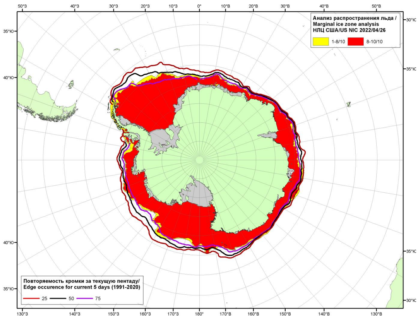
Рисунок 5в – Положение кромки льда и зон разреженных ( <8/10 ) и сплоченных ( \geq 8/10 ) льдов Южного океана за 26.04.2022 г. на основе ледового анализа Национального Ледового Центра США и повторяемость кромки за 26-30.04 за период 1991-2020 гг. по наблюдениям SSMR-SSM/I-SSMIS (алгоритм NASATEAM).
