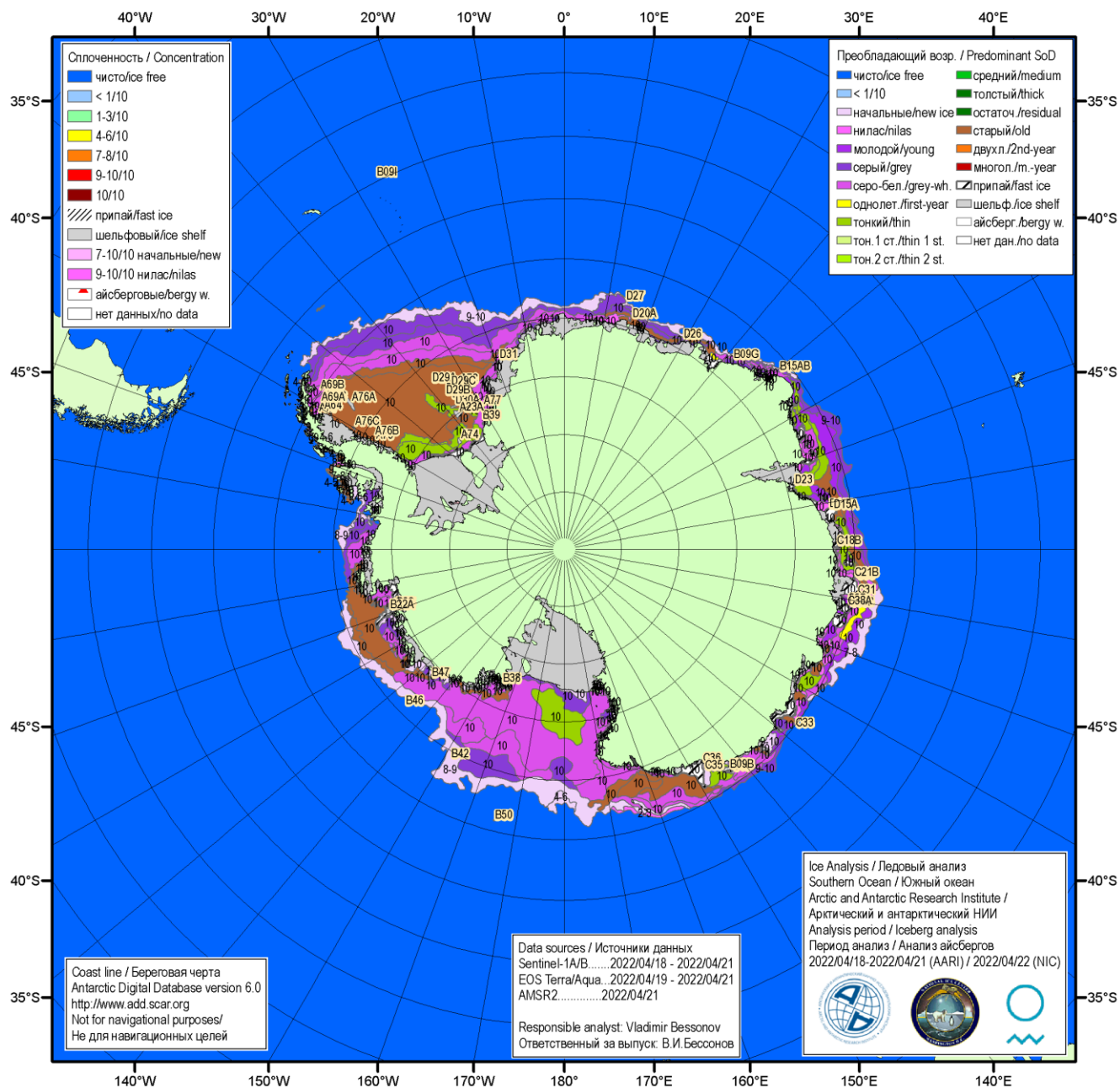
Рисунок 5в – Ледовая карта Южного океана (цветовая окраска по возрасту) и расположение крупных айсбергов на основе ледового анализа ААНИИ за 21.04.2022 в рамках проекта совместного ледового картирования Южного океана ААНИИ, НЛЦ США и НМИ.
