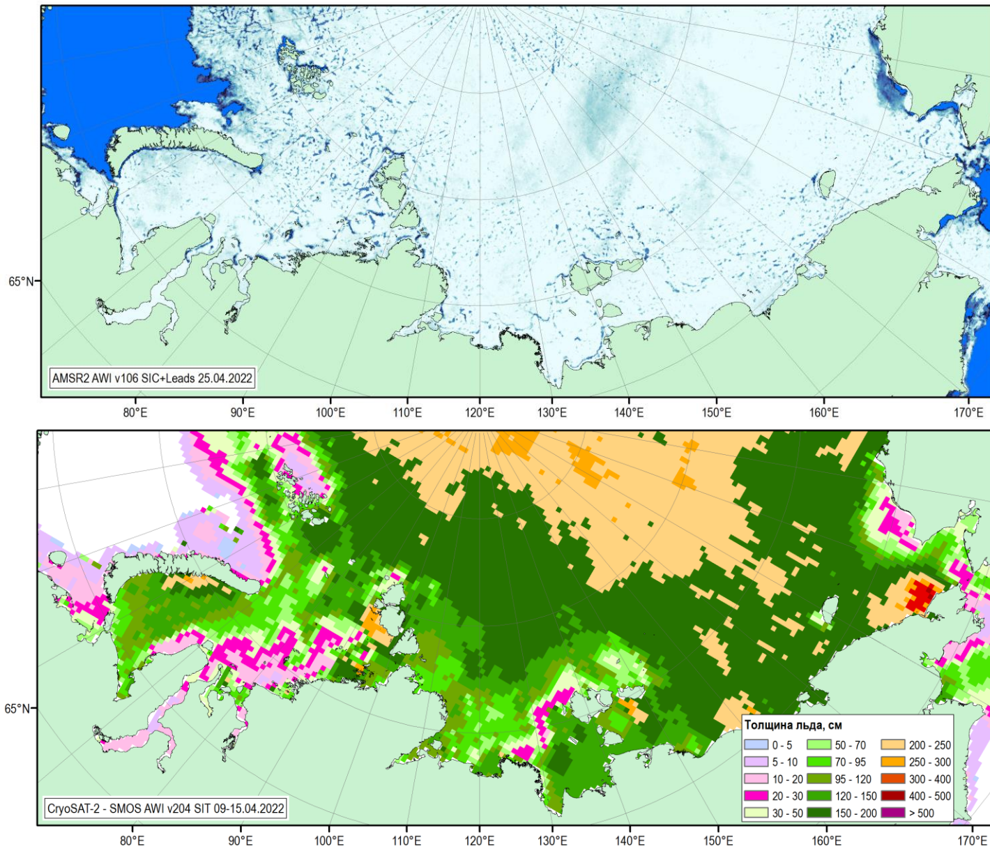
Рисунок 1г – Оценка сплоченности льда и расположения полыней по данным ИСЗ AMSR2 за 25.04.2022 (верх) и оценка толщин льда по данным ИСЗ CryoSAT-2 – SMOS за 09.04-15.04.2022 (AWI SIRAL).
