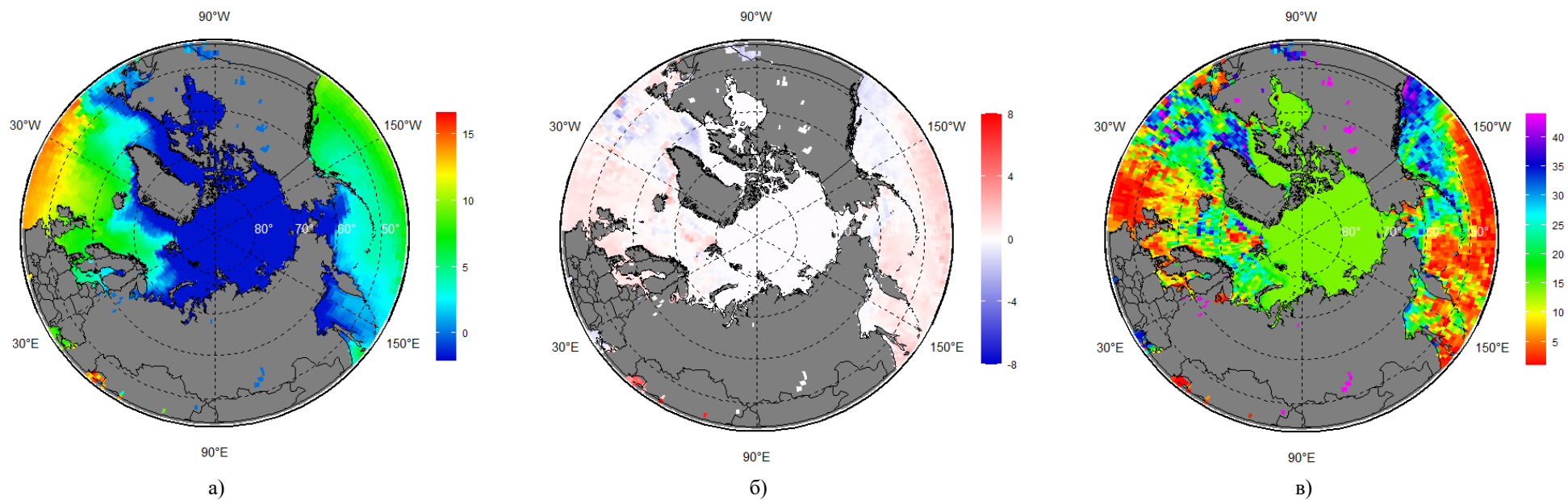
Рисунок 36 – Реанализ ERA5 температуры поверхности воды ( C^{\circ} ) за период 14.04 – 20.04.2022 г.: (а) – осредненные значения, (б) – аномалия относительно периода 1991-2020 гг. и (в) – ранг за период 1979-2022 гг.
