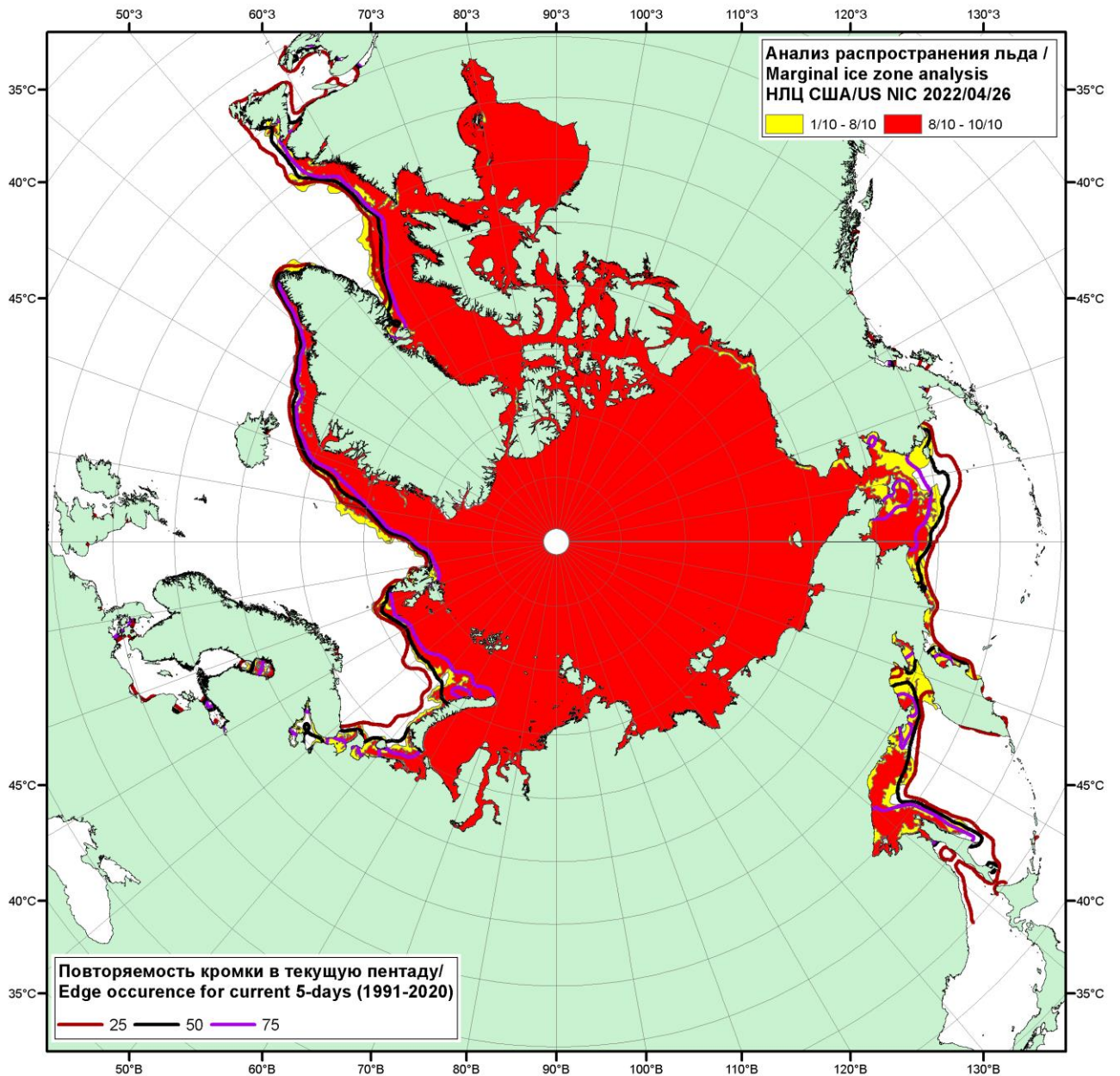
Рисунок 1в – Положение кромки льда и зон разреженных (<8/10) и сплоченных (≥8/10) льдов СЛО за 26.04.2022 г. на основе ледового анализа Национального Ледового Центра США и повторяемость кромки за 26.04-30.04 за период 1991-2020 гг. по наблюдениям SSMR-SSM/I-SSMIS (алгоритм NASATEAM)
