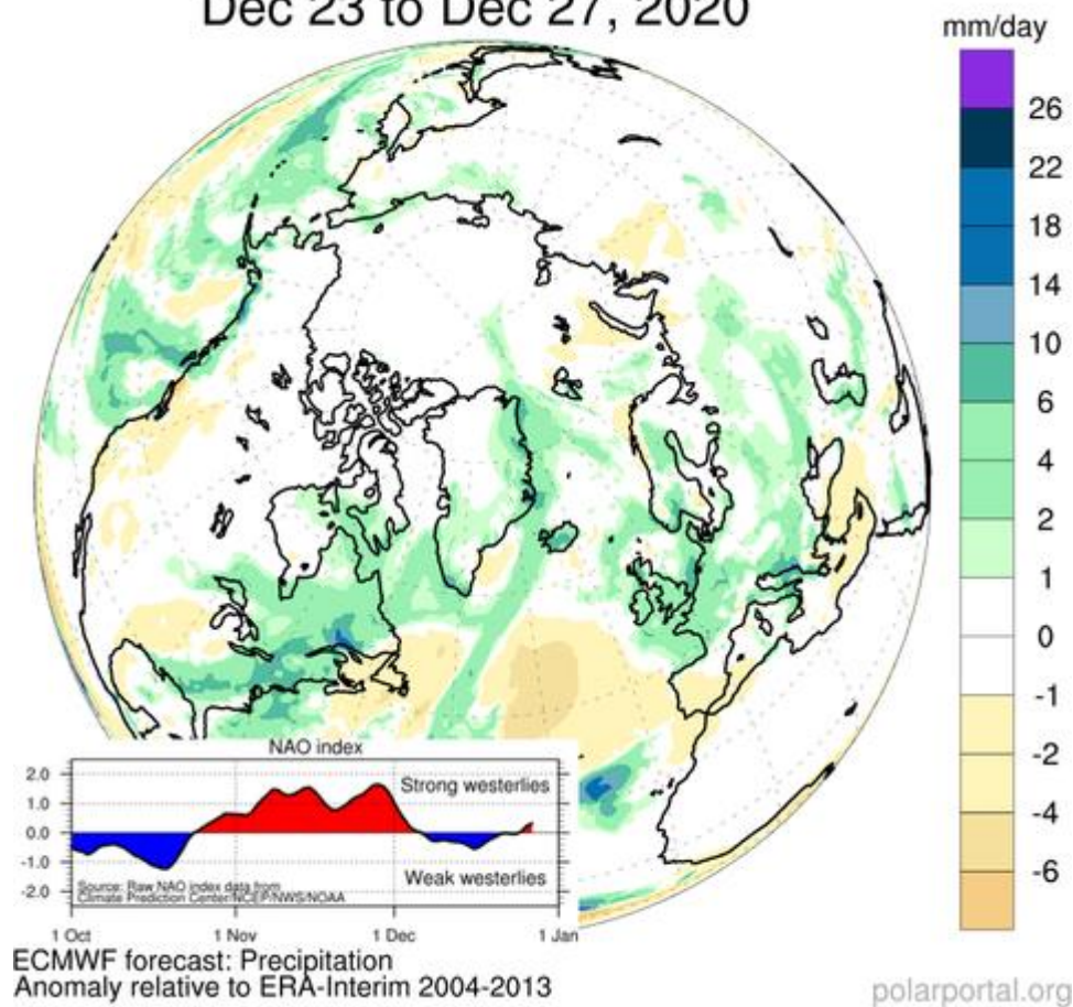
Рисунок 2ж – Аномалии приземной суммы осадков за 23.12 - 27.12 в 2020-2021 гг. относительно периода 2004-2013 гг. ( http://polarportal.dk )
