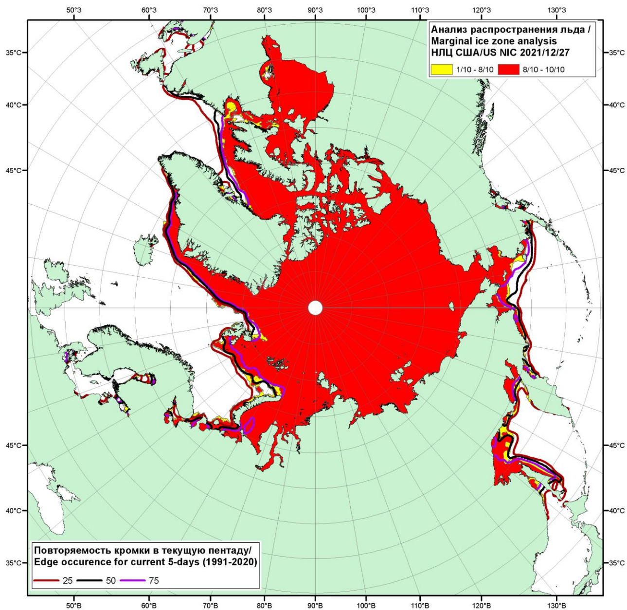
Рисунок 1в – Положение кромки льда и зон разреженных ( <8/10 ) и сплоченных ( \geq 8/10 ) льдов СЛО за 27.12.2021 г. на основе ледового анализа Национального Ледового Центра США и повторяемость кромки за 26-31.12 за период 1991-2020 гг. по наблюдениям SSMR-SSM/I-SSMIS (алгоритм NASATEAM)
