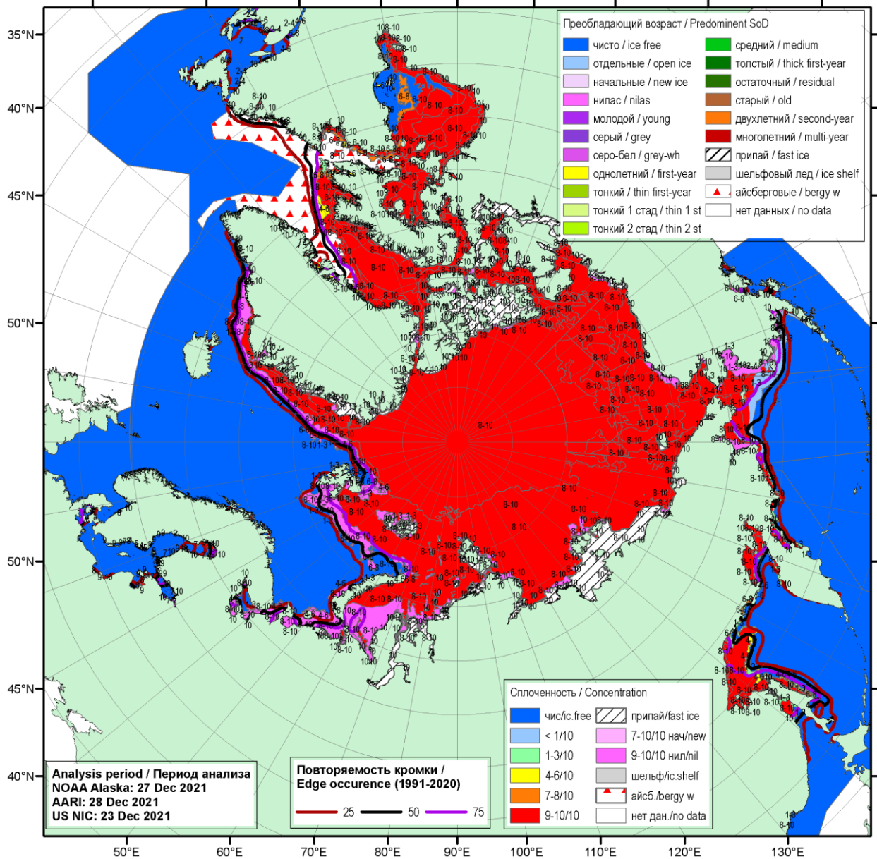
Рисунок 1а – Обзорная ледовая карта СЛО за 23.12-28.12.2021 г. (цветовая раскраска по общей сплоченности) на основе ледового анализа ААНИИ (28.12), NOAA Аляска (27.12) и Национального ледового центра США (23.12), и повторяемость кромки за 26.12-31.12 за период 1991-2020гг. по наблюдениям SSMR-SSM/I-SSMIS (алгоритм NASATEAM).
