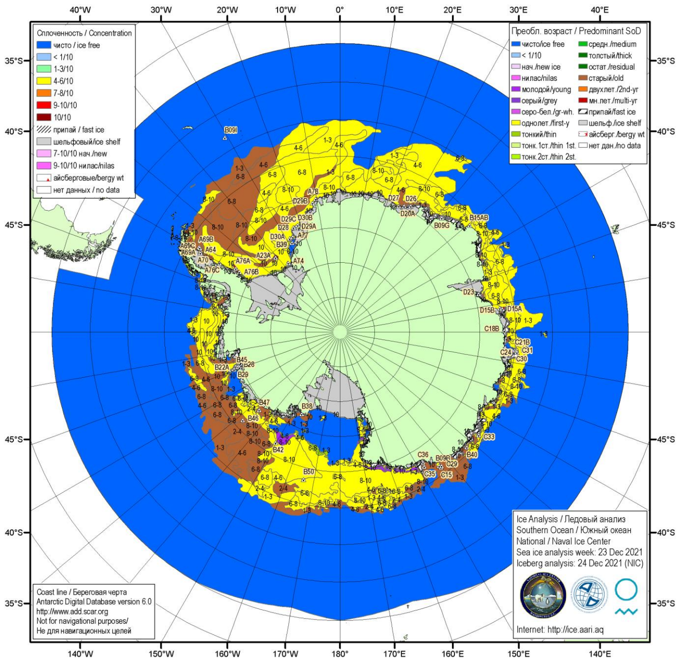
Рисунок 5б – Ледовая карта Южного океана (цветовая окраска по возрасту) и расположение крупных айсбергов на основе информации совместного ледового анализа НЛЦ США, ААНИИ и НМИ (Норвегия) за 23.12.2021.
