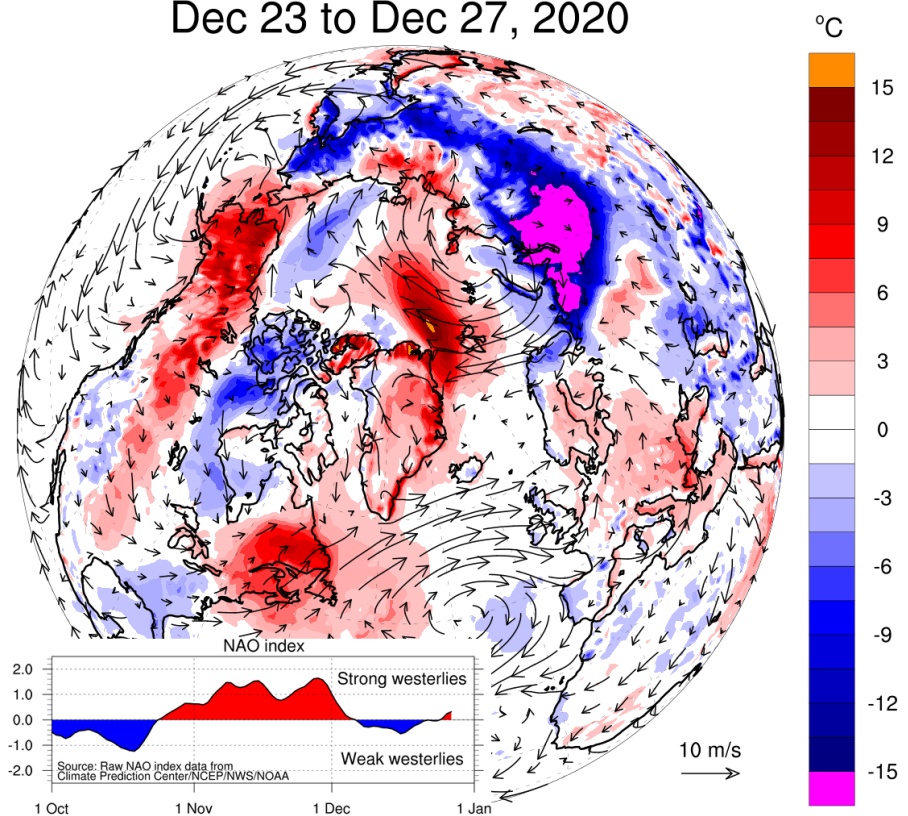
Рисунок 2е – Аномалии приземной температуры воздуха (2м) и осредненные вектора скорости ветра (10 м) за 23.12 - 27.12 в 2020-2021 гг. относительно периода 2004-2013 гг. ( http://polarportal.dk )
