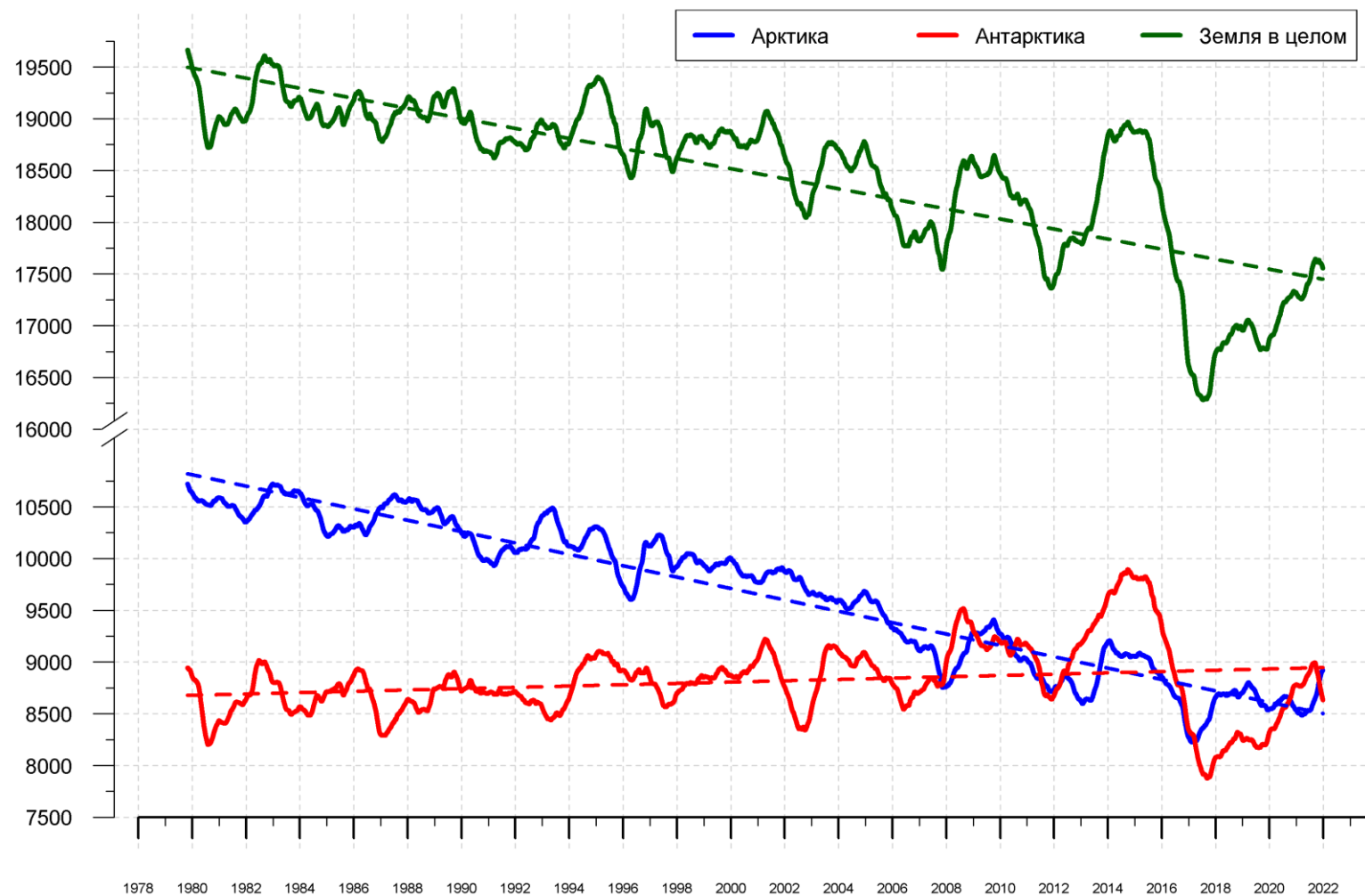
Рисунок 10 – Ежедневные сглаженные окном 365 суток значения приведенной ледовитости (площади морского льда) Арктики, Антарктики и Земли в целом с 26.10.1978 по 26.12.2021 на основе SSMR-SSM/I-SSMIS
