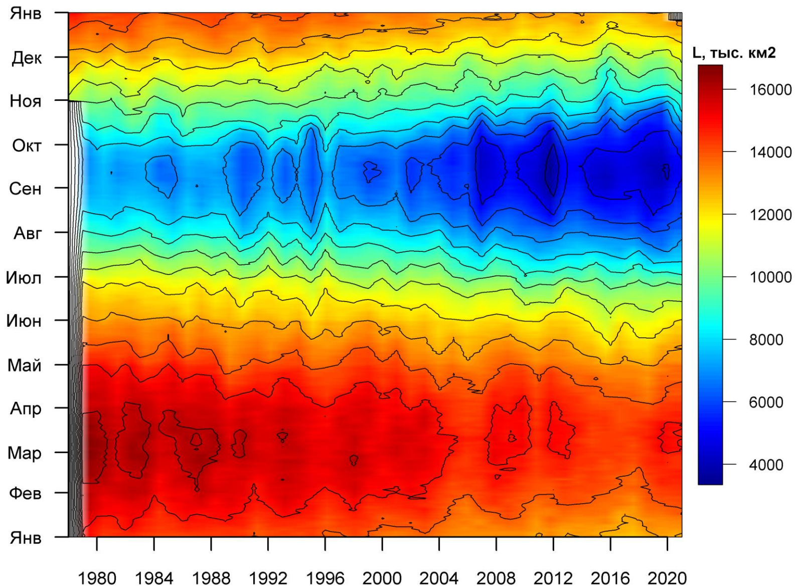
Рисунок 36 – Ежедневные оценки сезонных изменений ледовитости для Северной Полярной Области за период 26.10.1978 – 26.12.2021 на основе расчетов по данным SSMR-SSM/I-SSMIS, алгоритм NASATEAM.
