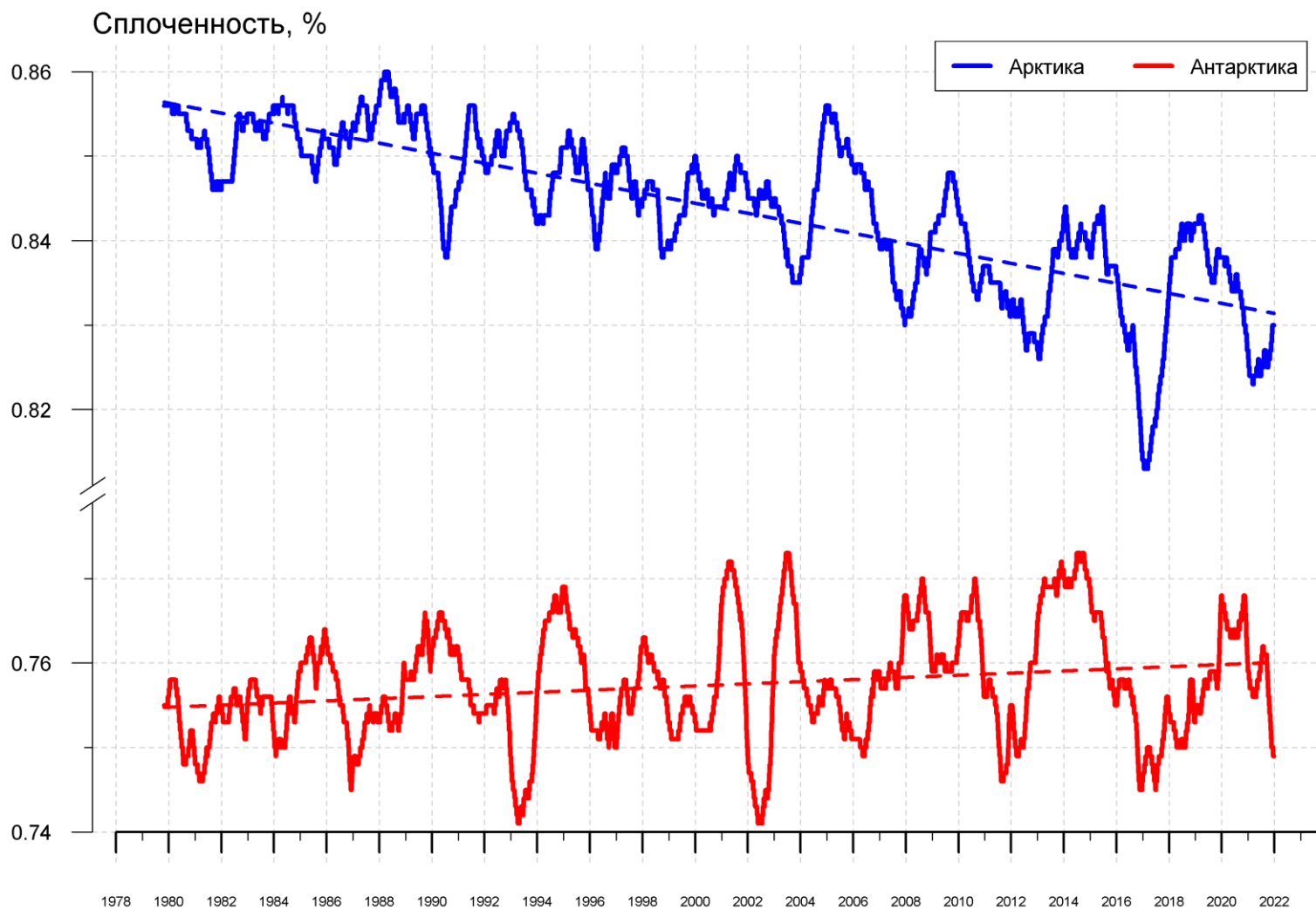
Рисунок 11 – Ежедневные сглаженные окном 365 суток значения средней общей сплоченности Арктики и Антарктики с 07.11.1978 по 26.12.2021 на основе SSMR-SSM/I-SSMIS
