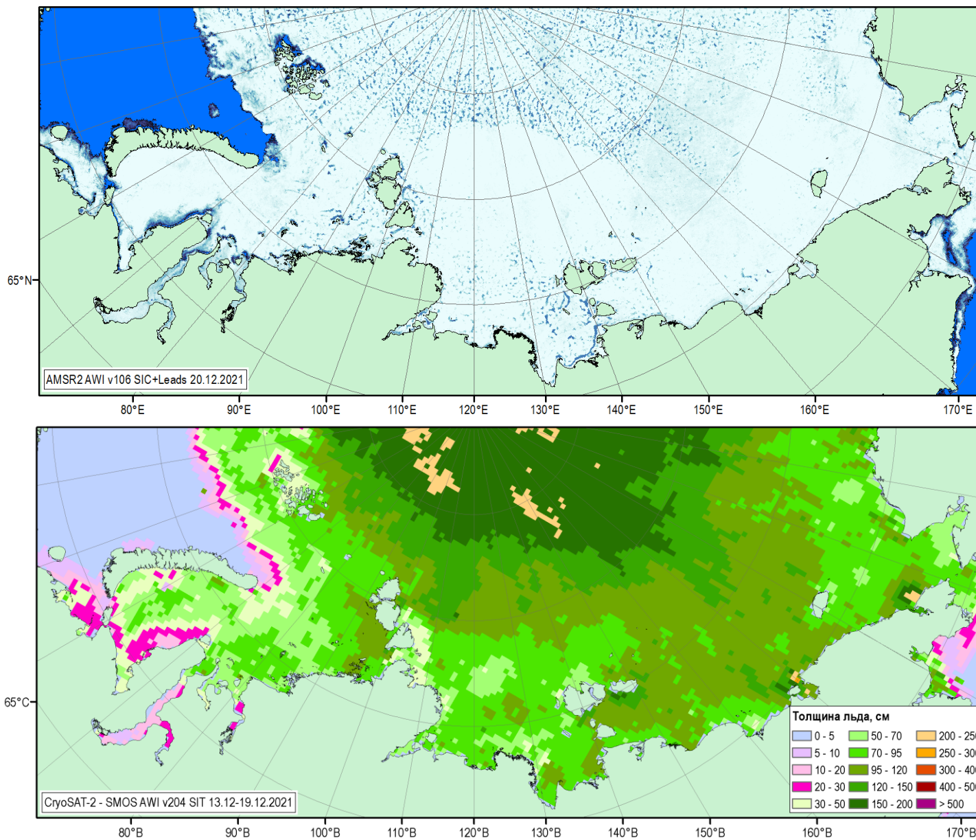
Рисунок 1г – Оценка сплоченности льда и расположения полыней по данным ИСЗ AMSR2 за 27.12.2021 (верх) и оценка толщин льда по данным ИСЗ CryoSAT-2 – SMOS за 20.12-26.12.2021 (AWI SIRAL).
