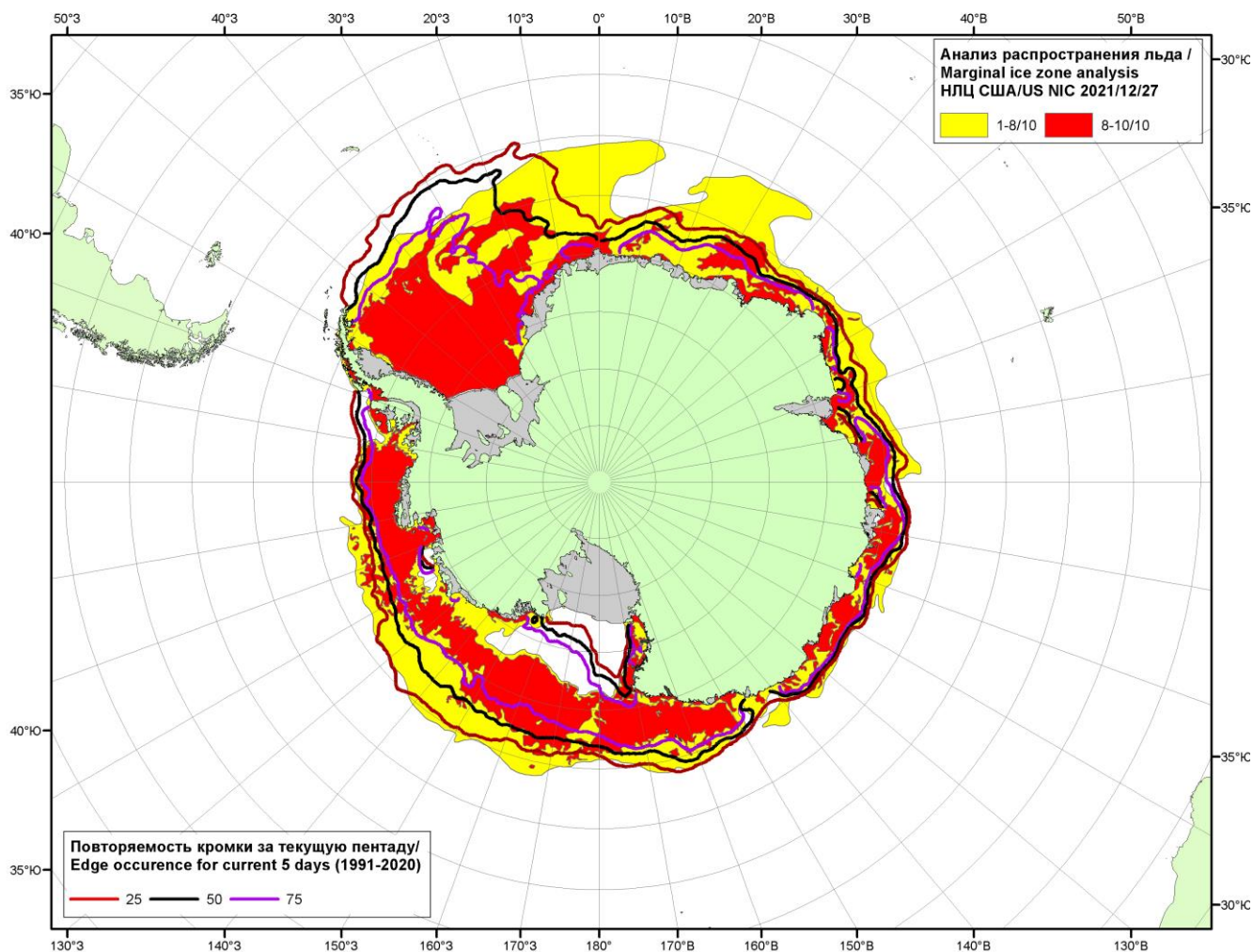
Рисунок 5в – Положение кромки льда и зон разреженных ( <8/10 ) и сплоченных ( \geq 8/10 ) льдов Южного океана за 27.12.2021 г. на основе ледового анализа Национального Ледового Центра США и повторяемость кромки за 26-31.12 за период 1991-2020 гг. по наблюдениям SSMR-SSM/I-SSMIS (алгоритм NASATEAM).
