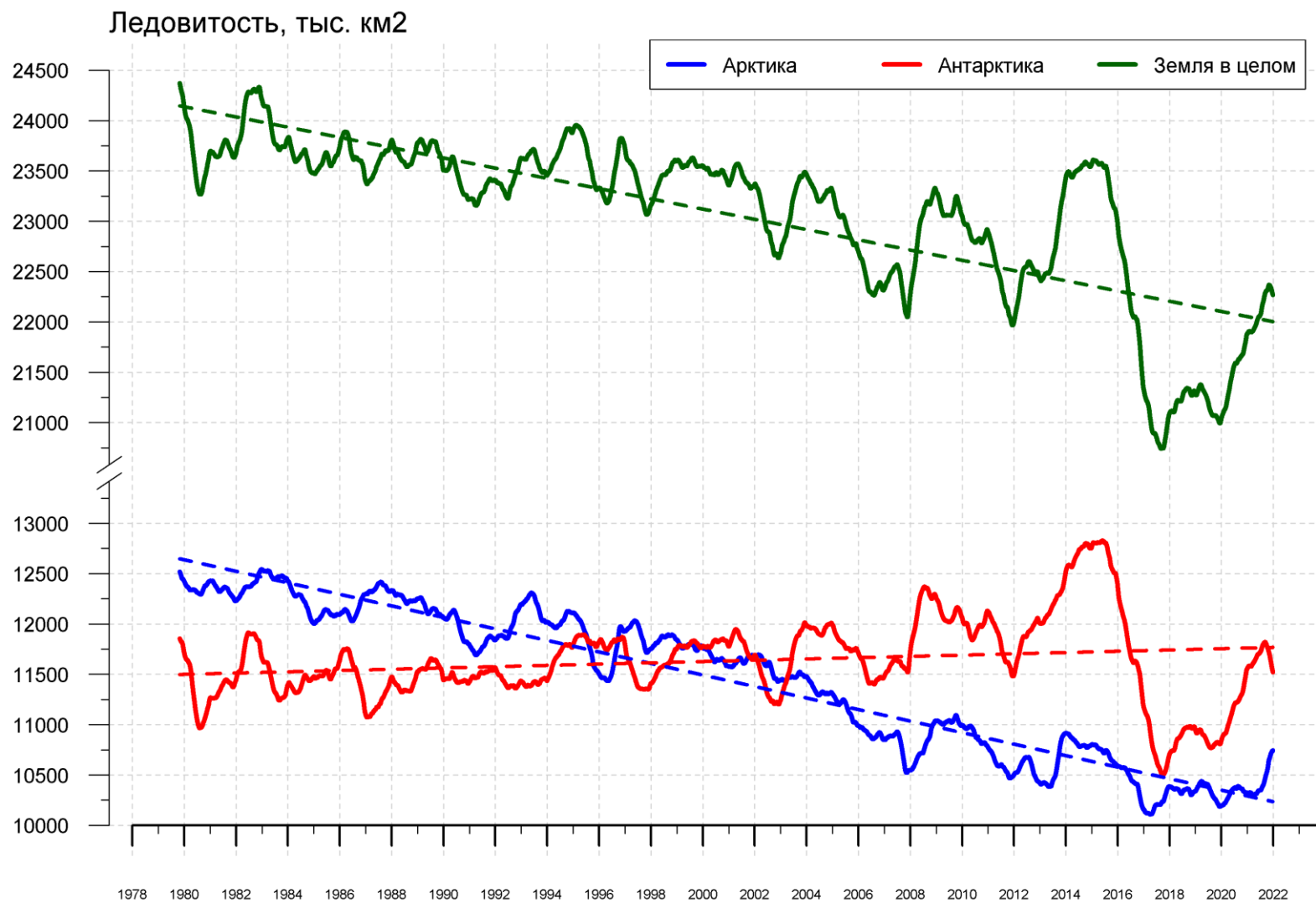
Рисунок 9 – Ежедневные сглаженные окном 365 суток значения ледовитости (площади распространения морского льда) Арктики, Антарктики и Земли в целом с 26.10.1978 по 26.12.2021 на основе SSMR-SSM/I-SSMIS
