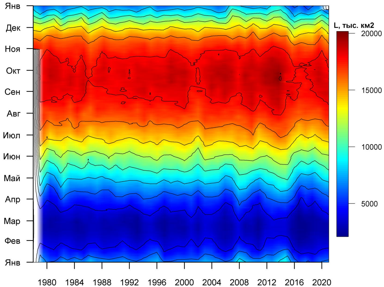
Рисунок 76 – Ежедневные оценки сезонных изменений ледовитости для Южного океана за период 26.10.1978 – 26.12.2021 на основе расчетов по данным SSMR-SSM/I-SSMIS, алгоритм NASATEAM.
