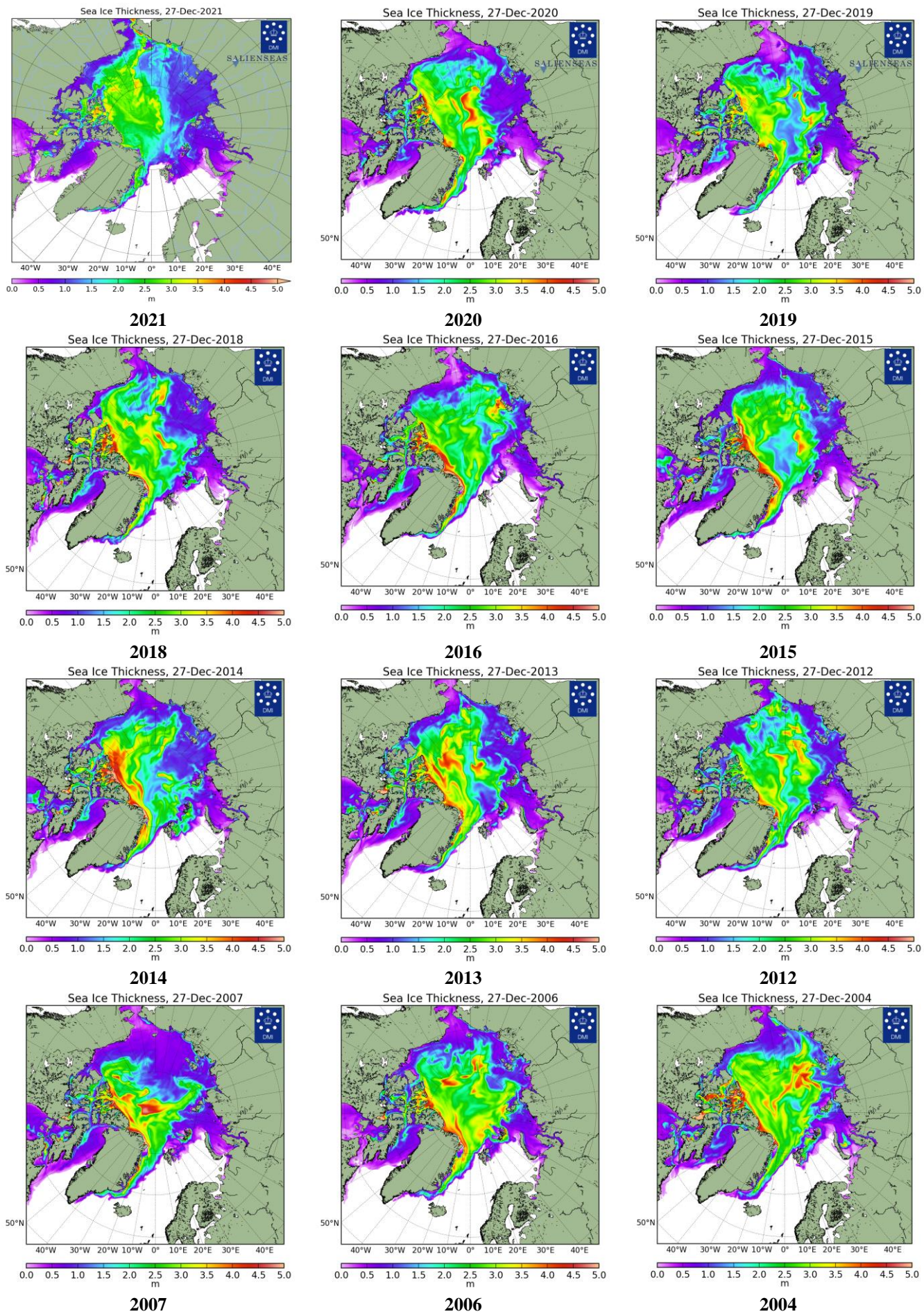
Рисунок 26 – Поля распределения средневзвешенной толщины льда совместной модели морского льда – океана NUCOM/CICE Датского метеорологического института 27.12 за 2004-2021 гг.
