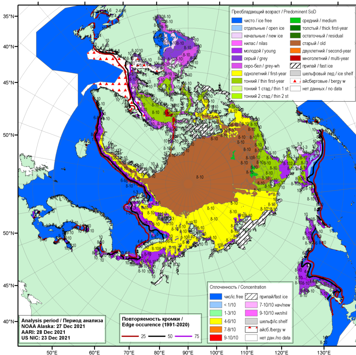
Рисунок 16 – Обзорная ледовая карта СЛО за 23.12-28.12.2021 г. (цветовая раскраска по преобладающему возрасту) на основе ледового анализа ААНИИ (28.12), NOAA Аляска (27.12) и Национального ледового центра США (23.12), и повторяемость кромки за 26.12-31.12 за период 1991-2020гг. по наблюдениям SSMR-SSM/I-SSMIS (алгоритм NASATEAM).
