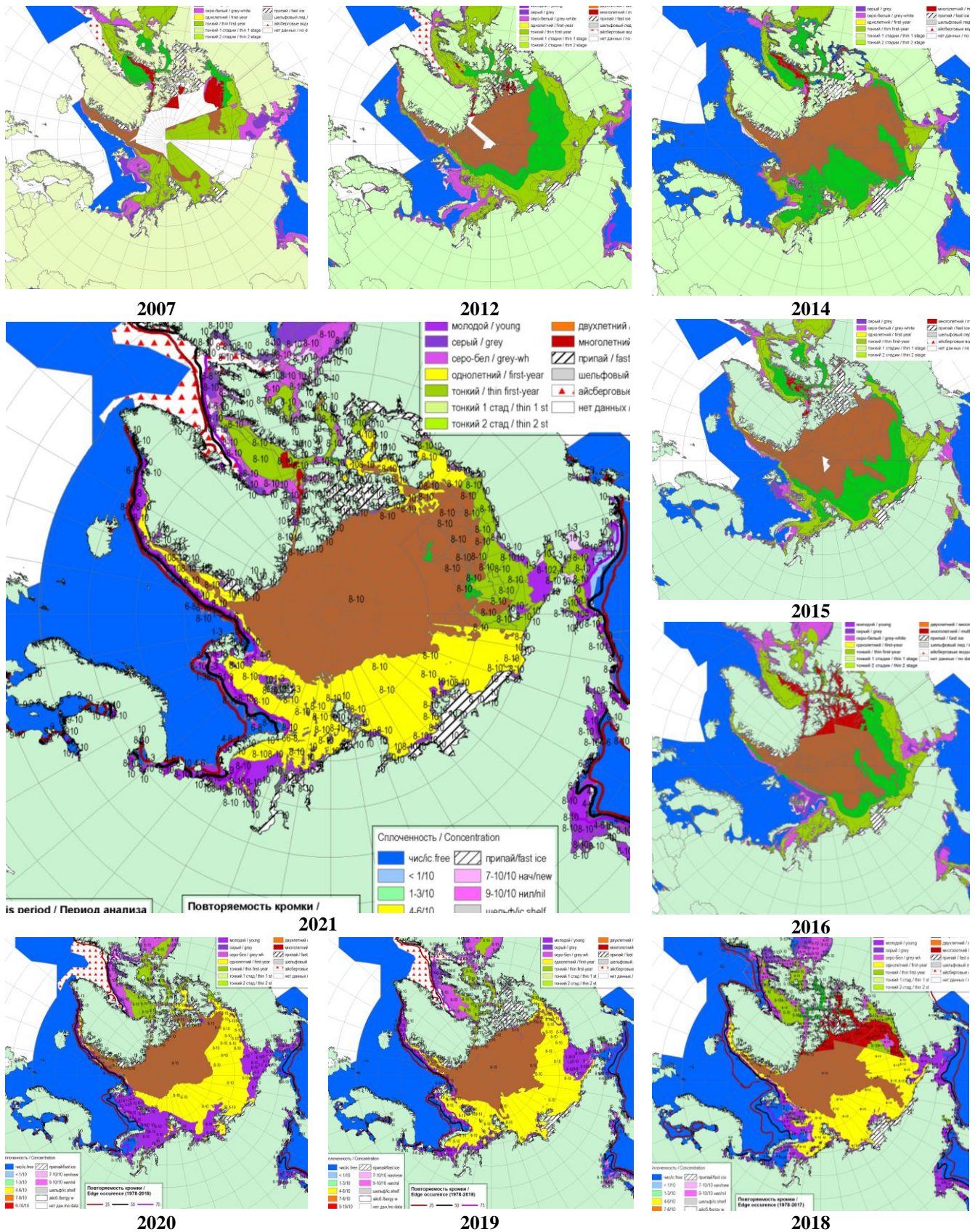
Рисунок 2а – Обзорная ледовая карта СЮ за 23.12-28.12.2021 г. и аналогичные периоды 2007-2020гг. на основе ледового анализа ААНИИ, НИЦ Планета, Канадской ледовой службы и Национального ледового центра США.
