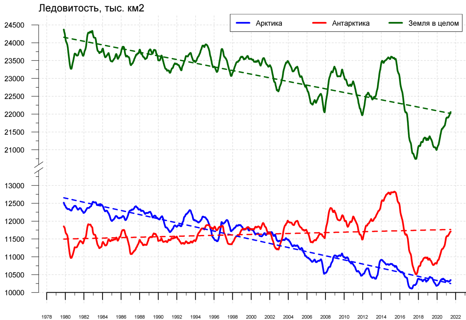
Рисунок 9 – Ежедневные сглаженные окном 365 суток значения ледовитости (площади распространения морского льда) Арктики, Антарктики и Земли в целом с 26.10.1978 по 20.06.2021 на основе SSMR-SSM/I-SSMIS
