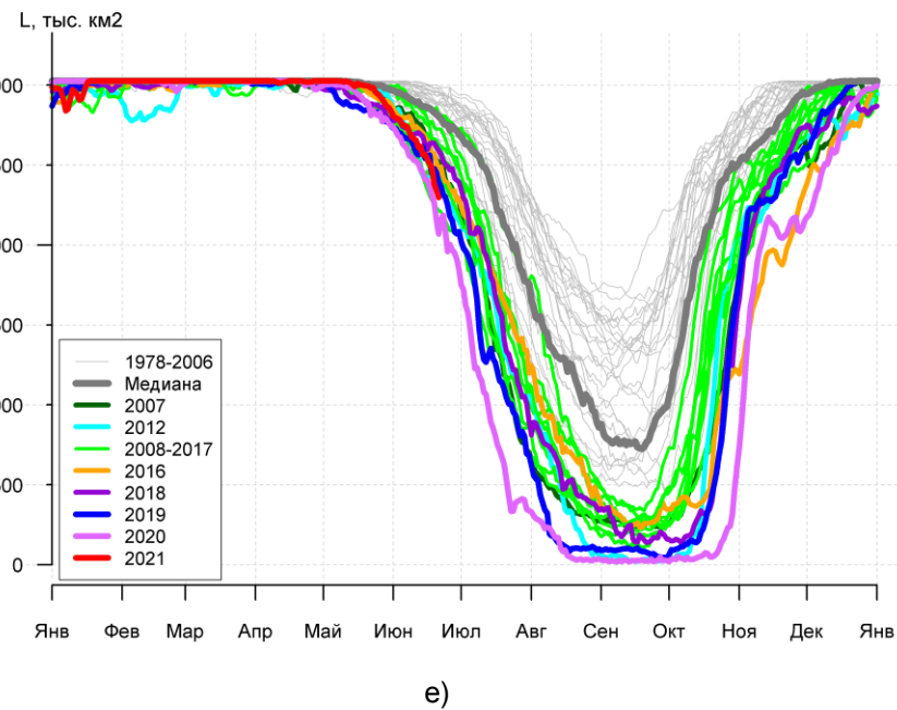
Рисунок 3а – Ежедневные оценки сезонного хода ледовитости для Северной Полярной Области и трех меридиональных секторов за период 26.10.1978 - 20.06.2021 по годам на основе расчетов по данным SSMR-SSM/I-SSMIS, алгоритмы NASATEAM: а) Северная полярная область, б) сектор 45°W-95°E (Гренландское – Карское моря), в) сектор 95°E-170°W (моря Лаптевых – Чукотское и Берингово, Охотское), г) сектор 170°W-45°W (море Бофорта и Канадская Арктика), д) Северный Ледовитый океан, е) Северный морской путь (Карское - Чукотское моря).
