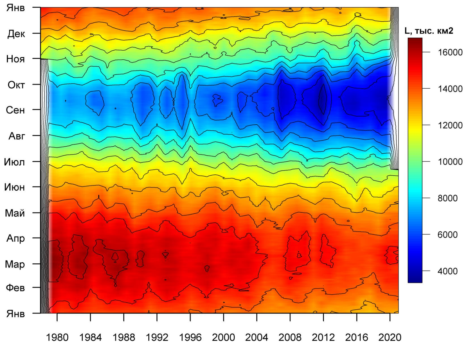
Рисунок 3б – Ежедневные оценки сезонных изменений ледовитости для Северной Полярной Области за период 26.10.1978 – 20.06.2021 на основе расчетов по данным SSMR-SSM/I-SSMIS, алгоритм NASATEAM.
