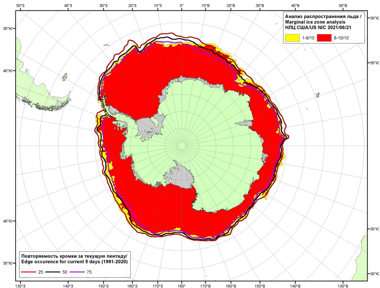
Рисунок 5в – Положение кромки льда и зон разреженных ( <8/10 ) и сплоченных ( \geq 8/10 ) льдов Южного океана за 21.06.2021 г. на основе ледового анализа Национального Ледового Центра США и повторяемость кромки за 21-25.06 за период 1991-2020 гг. по наблюдениям SSMR-SSM/I-SSMIS (алгоритм NASATEAM).
