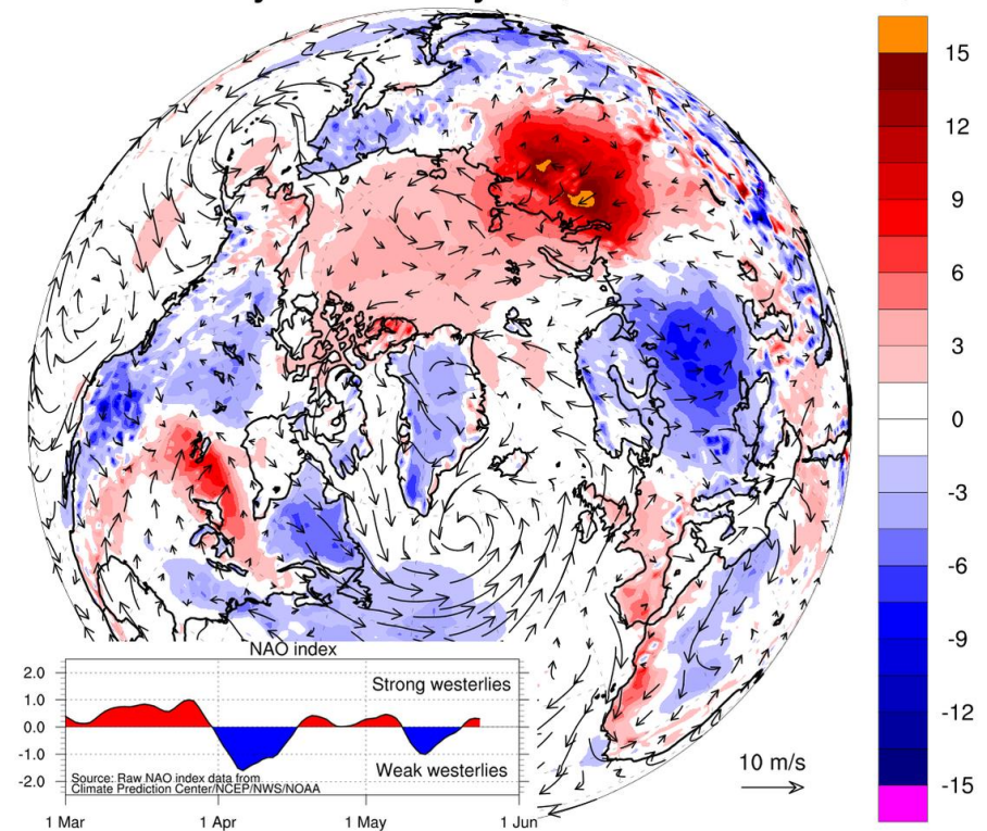
Рисунок 2е – Аномалии приземной температуры воздуха (2м) и осредненные вектора скорости ветра (10 м) за 20.05 - 24.05.2021 гг. относительно периода 2004-2013 гг. ( http://polarportal.dk )
