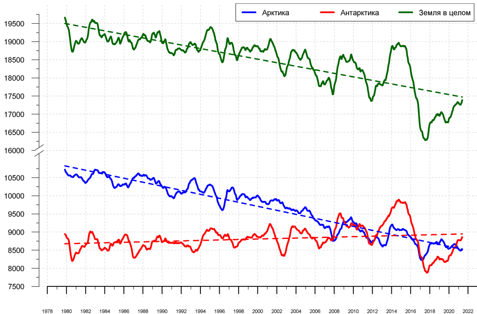
Рисунок 10 – Ежедневные сглаженные окном 365 суток значения приведенной ледовитости (площади морского льда) Арктики, Антарктики и Земли в целом с 26.10.1978 по 23.05.2021 на основе SSMR-SSM/I-SSMIS
