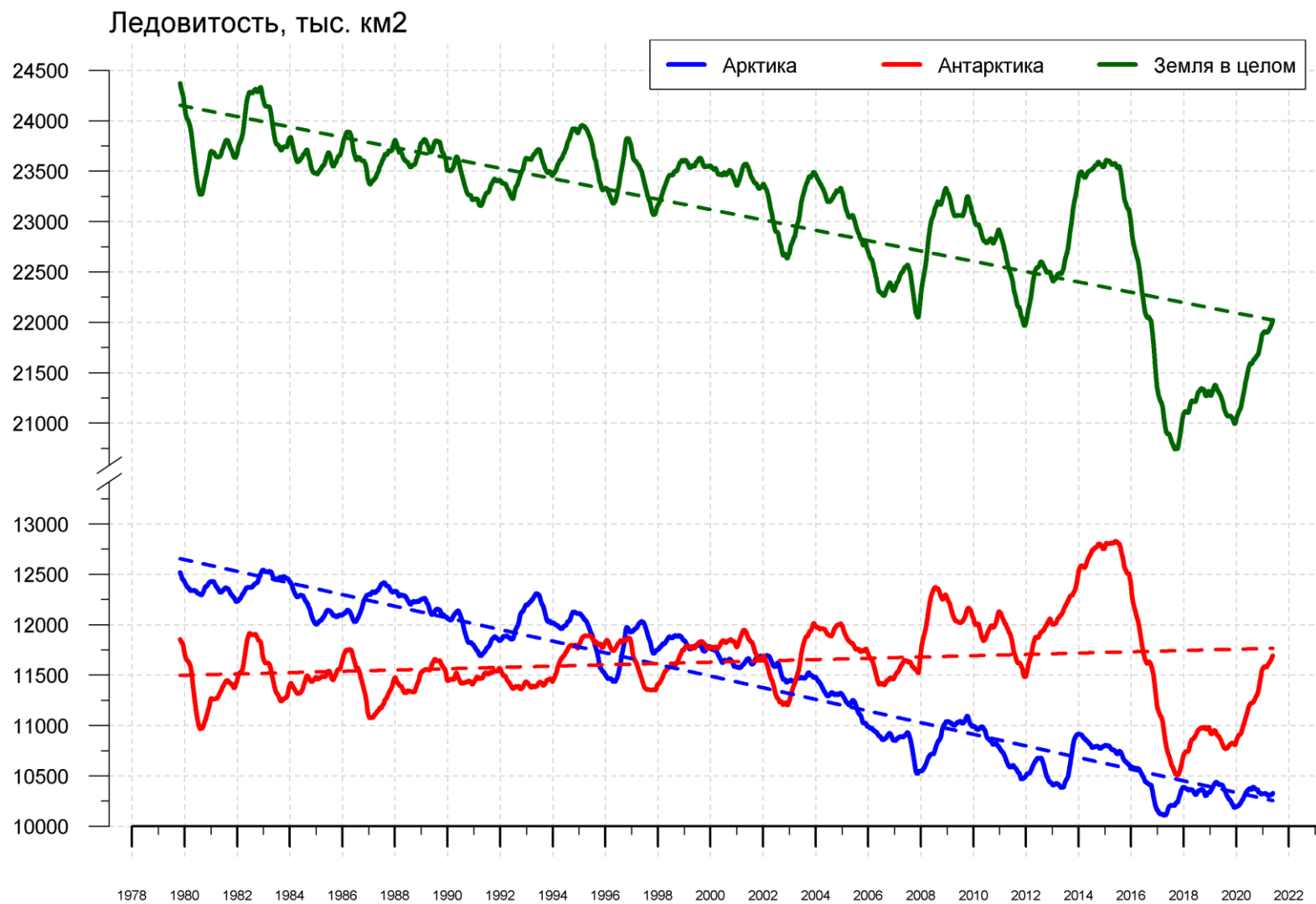
Рисунок 9 – Ежедневные сглаженные окном 365 суток значения ледовитости (площади распространения морского льда) Арктики, Антарктики и Земли в целом с 26.10.1978 по 23.05.2021 на основе SSMR-SSM/I-SSMIS
