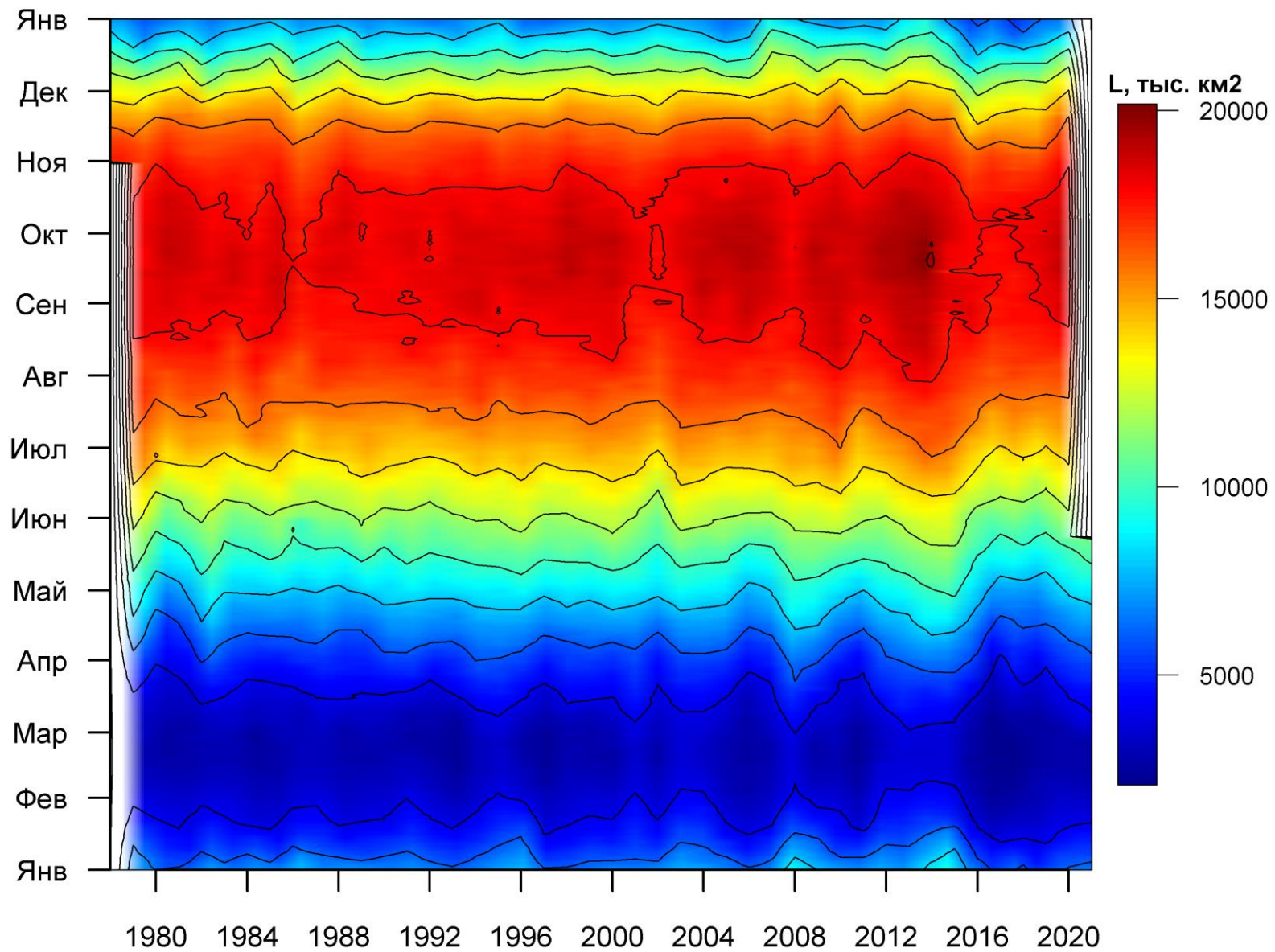
Рисунок 76 – Ежедневные оценки сезонных изменений ледовитости для Южного океана за период 26.10.1978 – 23.05.2021 на основе расчетов по данным SSMR-SSM/I-SSMIS, алгоритм NASATEAM.
