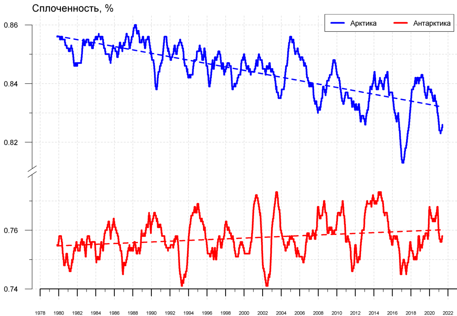
Рисунок 11 – Ежедневные сглаженные окном 365 суток значения средней общей сплоченности Арктики и Антарктики с 26.10.1978 по 23.05.2021 на основе SSMR-SSM/I-SSMIS
