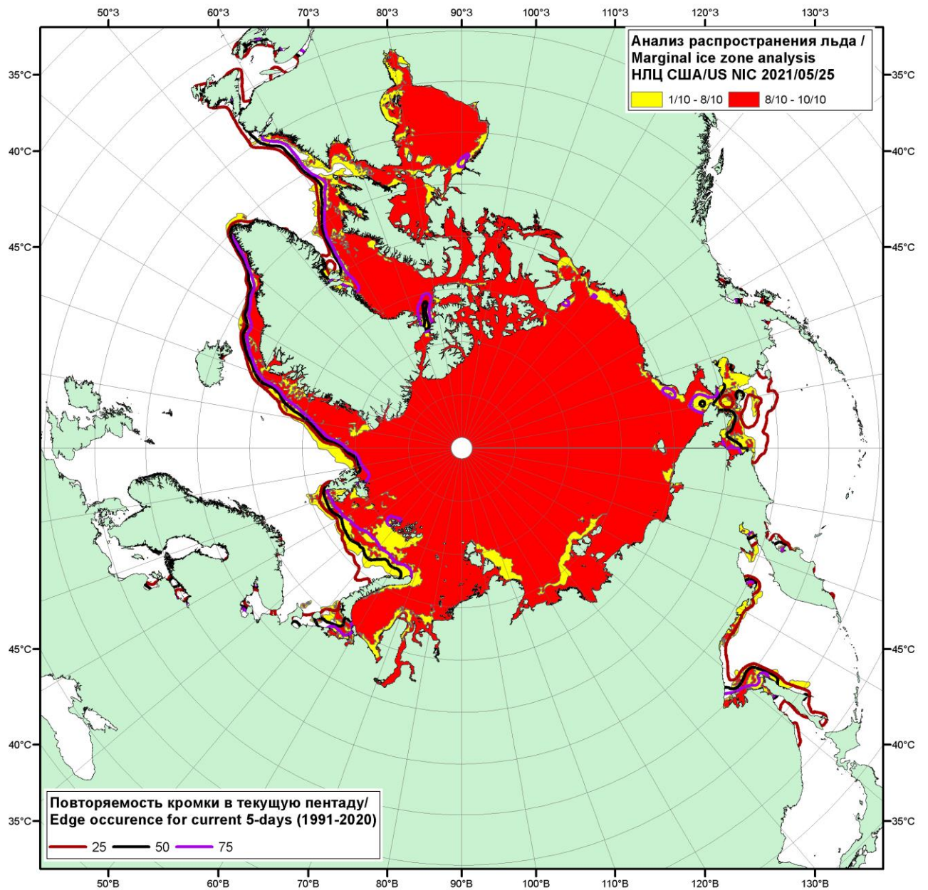
Рисунок 1в – Положение кромки льда и зон разреженных (<8/10) и сплоченных ( \geq 8/10 ) льдов СЛО за 25.05.2021 г. на основе ледового анализа Национального Ледового Центра США и повторяемость кромки за 21-25.05 за период 1991-2020 гг. по наблюдениям SSMR-SSM/I-SSMIS (алгоритм NASATEAM)
