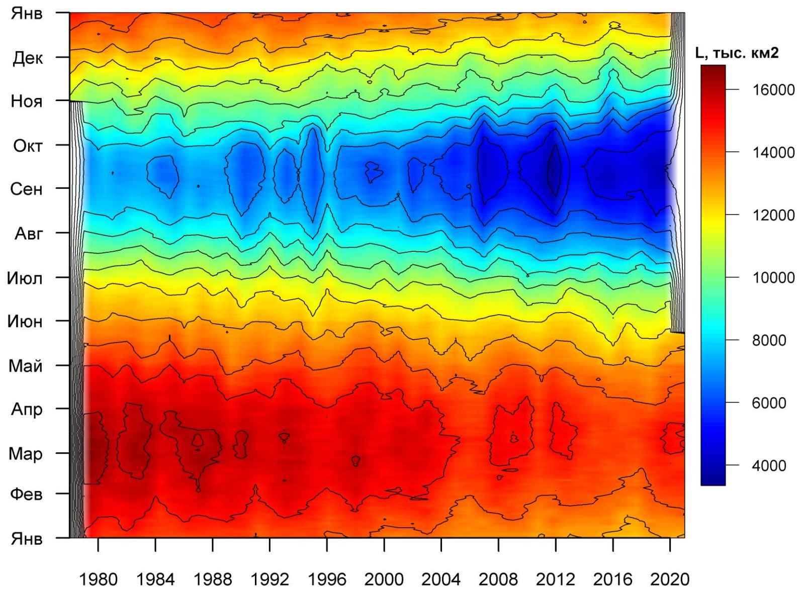
Рисунок 3б – Ежедневные оценки сезонных изменений ледовитости для Северной Полярной Области за период 26.10.1978 – 23.05.2021 на основе расчетов по данным SSMR-SSM/I-SSMIS, алгоритм NASATEAM.
