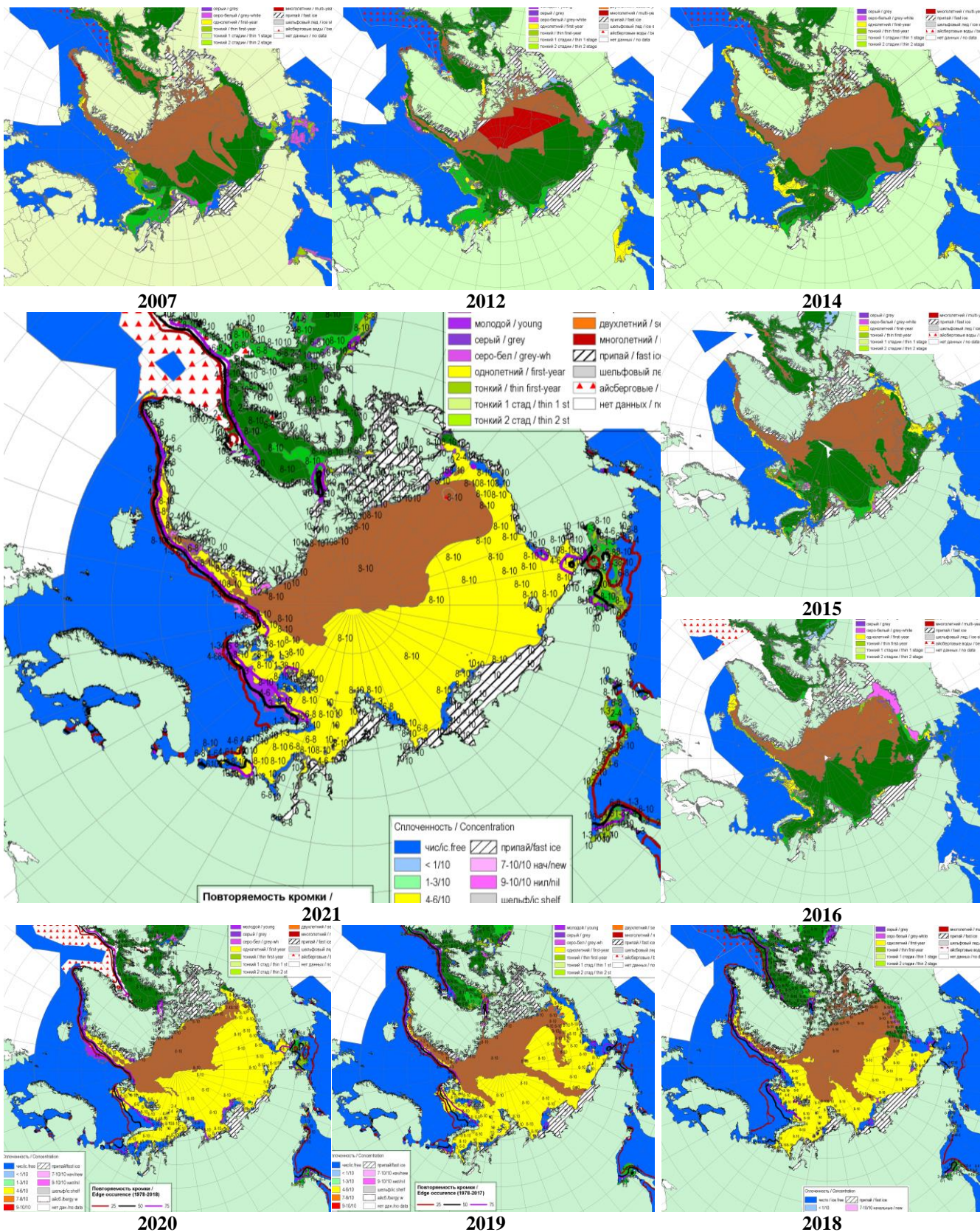
Рисунок 2а – Обзорная ледовая карта СЛО за 20.05-25.05.2021 г и аналогичные периоды 2007-2020гг. на основе ледового анализа ААНИИ, НИЦ Планета, Канадской ледовой службы и Национального ледового центра США.
