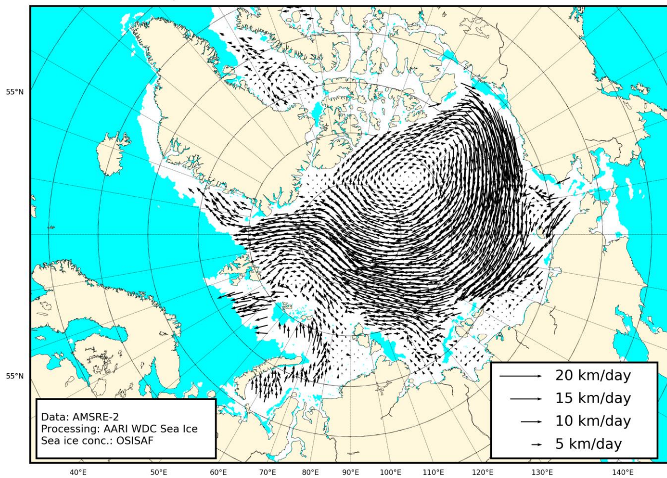
Рисунок 2г – Поле дрейфа морского льда Арктики за 17.05-24.05.2021 г., источник данных EUMETSAT OSISAF.
