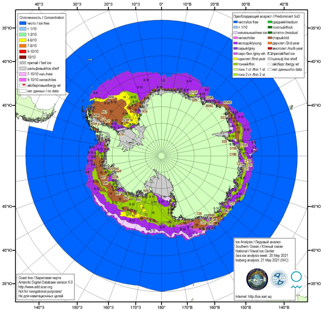
Рисунок 5б – Ледовая карта Южного океана (цветовая окраска по возрасту) и расположение крупных айсбергов на основе информации совместного ледового анализа НЛЦ США, ААНИИ и НМИ (Норвегия) за 20.05.2021.
