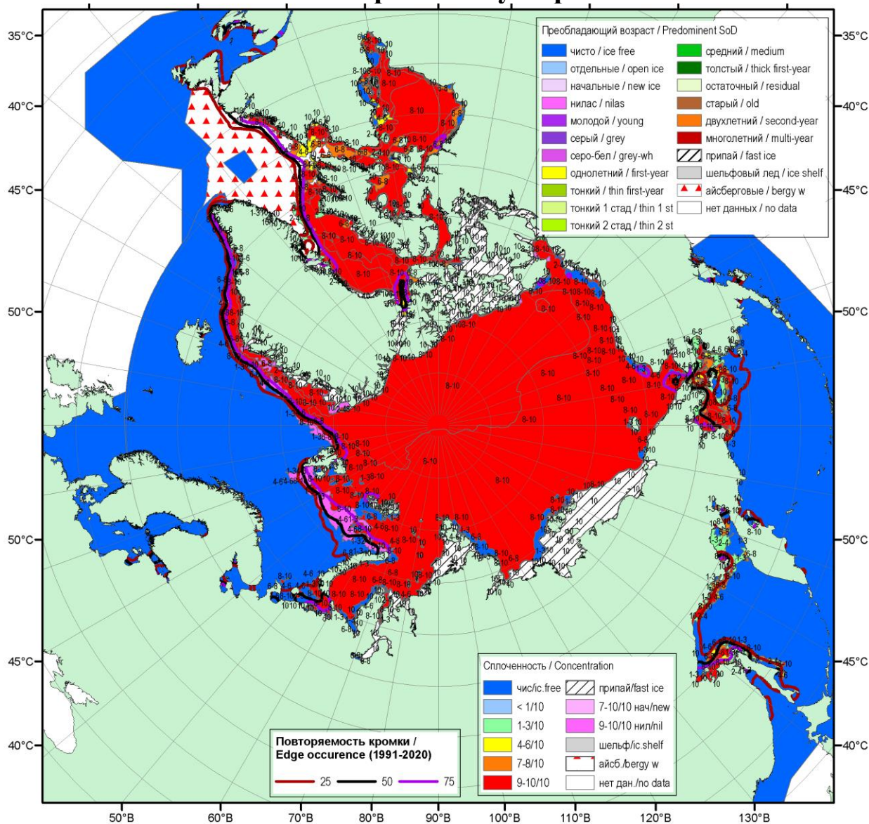
Рисунок 1а – Обзорная ледовая карта СЛЮ за 20.05-25.05.2021 г. (цветовая раскраска по общей сплоченности) на основе ледового анализа ААНИИ (25.05), Национального ледового центра США (20.05) и повторяемость кромки за 21-25.05 за период 1991-2020 гг. по наблюдениям SSMR-SSM/I-SSMIS (алгоритм NASATEAM).
