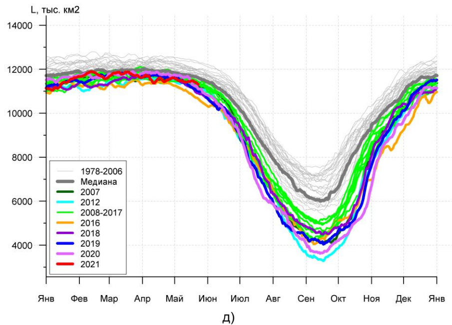
Рисунок 3а – Ежедневные оценки сезонного хода ледовитости для Северной Полярной Области и трех меридиональных секторов за период 26.10.1978 - 23.05.2021 по годам на основе расчетов по данным SSMR-SSM/I-SSMIS, алгоритмы NASATEAM: а) Северная полярная область, б) сектор 45°W-95°E (Гренландское – Карское моря), в) сектор 95°E-170°W (моря Лаптевых – Чукотское и Берингово, Охотское), г) сектор 170°W-45°W (море Бофорта и Канадская Арктика), д) Северный Ледовитый океан, е) Северный морской путь (Карское - Чукотское моря).
