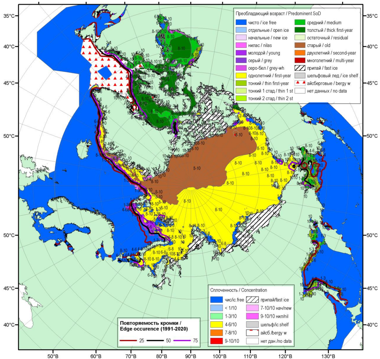
Рисунок 16 – Обзорная ледовая карта СЮ за 20.05-25.05.2021 г. (цветовая раскраска по преобладающему возрасту) на основе ледового анализа ААНИИ (25.05), Национального ледового центра США (20.05) и повторяемость кромки за 21-25.05 за период 1991-2020 гг. по наблюдениям SSMR-SSM/I-SSMIS (алгоритм NASATEAM).
