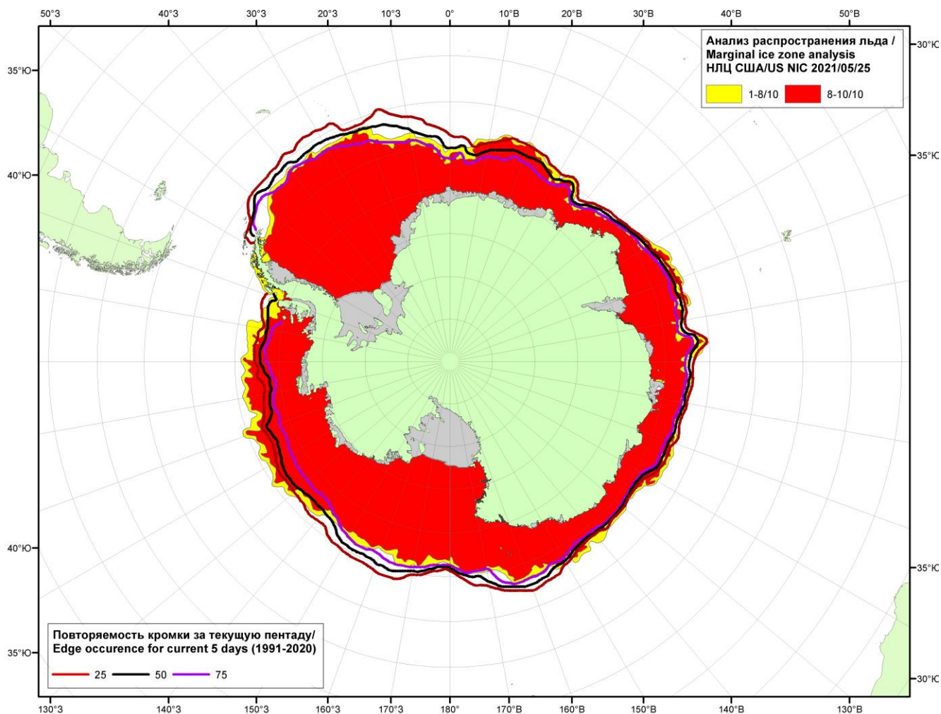
Рисунок 5в – Положение кромки льда и зон разреженных ( <8/10 ) и сплоченных ( \geq 8/10 ) льдов Южного океана за 25.05.2021 г. на основе ледового анализа Национального Ледового Центра США и повторяемость кромки за 21-25.05 за период 1991-2020 гг. по наблюдениям SSMR-SSM/I-SSMIS (алгоритм NASATEAM)..
