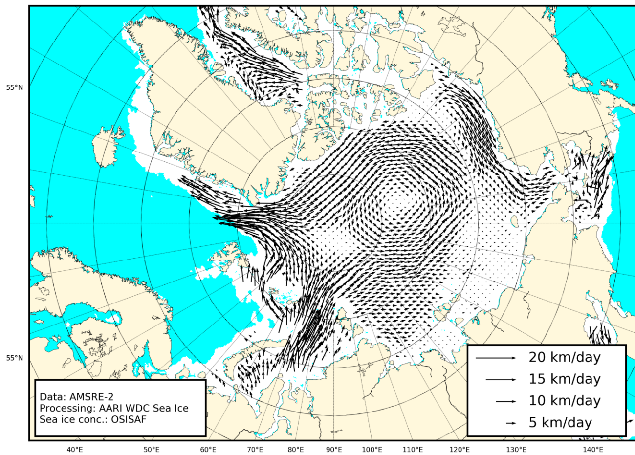
Рисунок 2г – Поле дрейфа морского льда Арктики за 29.03-05.04.2021 г., источник данных EUMETSAT OSISAF.
