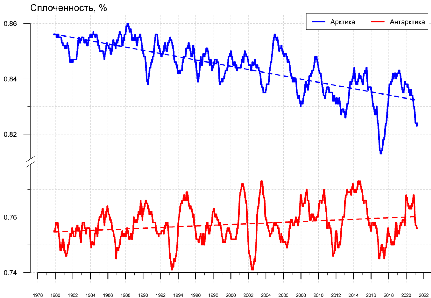
Рисунок 11 – Ежедневные сглаженные окном 365 суток значения средней общей сплоченности Арктики и Антарктики с 26.10.1978 по 04.04.2021 на основе SSMR-SSM/I-SSMIS
