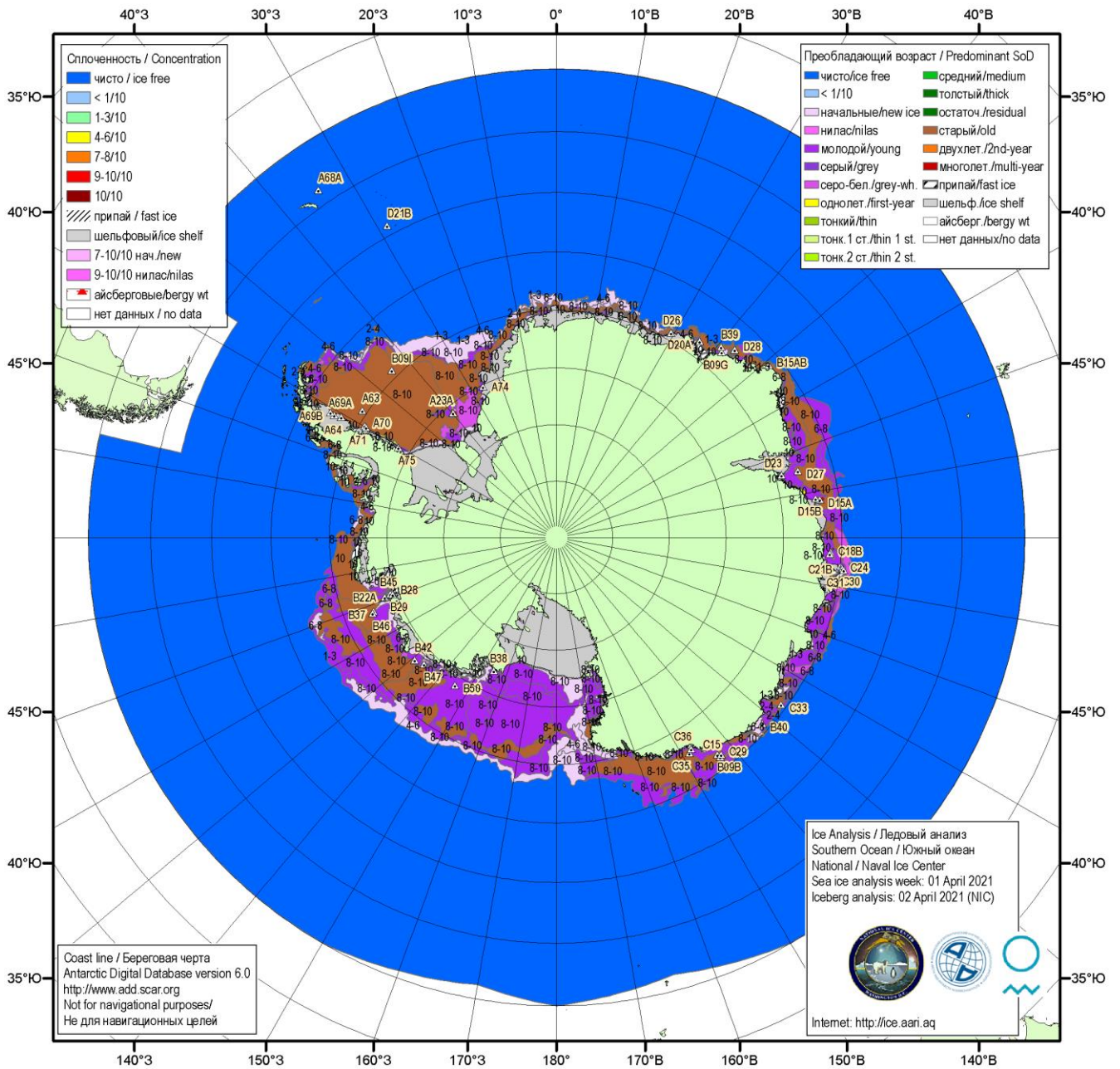
Рисунок 5б – Ледовая карта Южного океана (цветовая окраска по возрасту) и расположение крупных айсбергов на основе информации совместного ледового анализа НЛЦ США, ААНИИ и НМИ (Норвегия) за 01.04.2021.
