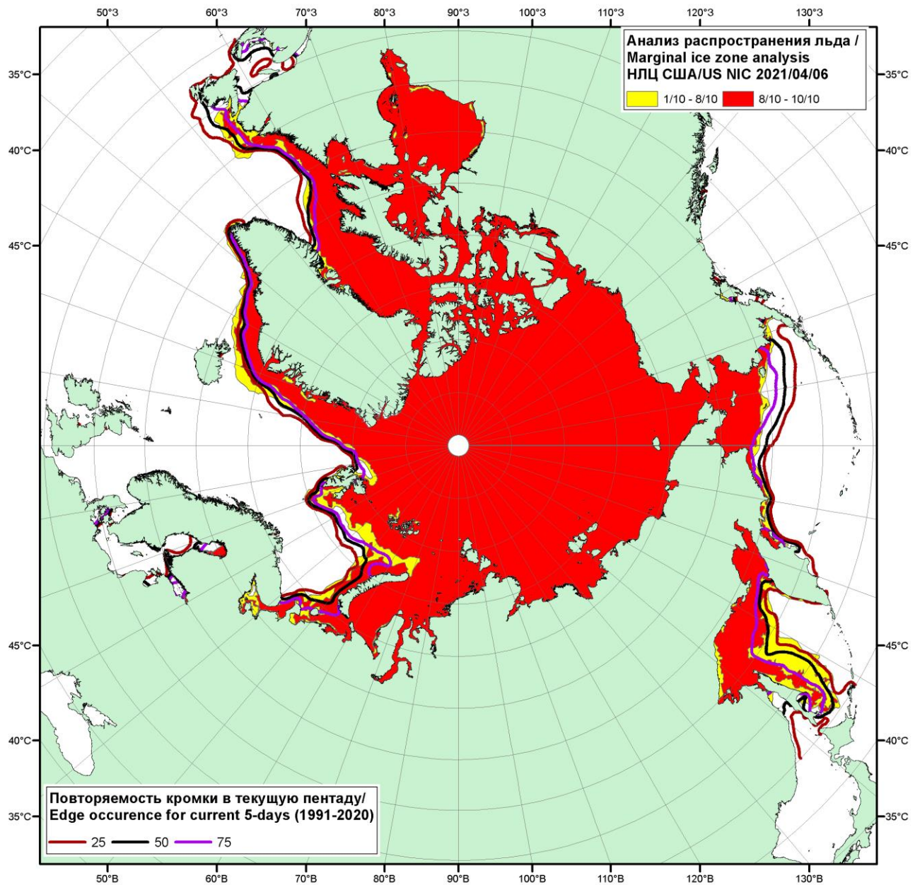
Рисунок 1в – Положение кромки льда и зон разреженных ( <8/10 ) и сплоченных ( \geq 8/10 ) льдов СЛО за 06.04.2021 г. на основе ледового анализа Национального Ледового Центра США и повторяемость кромки за 01-05.04 за период 1991-2020 гг. по наблюдениям SSMR-SSM/I-SSMIS (алгоритм NASATEAM)
