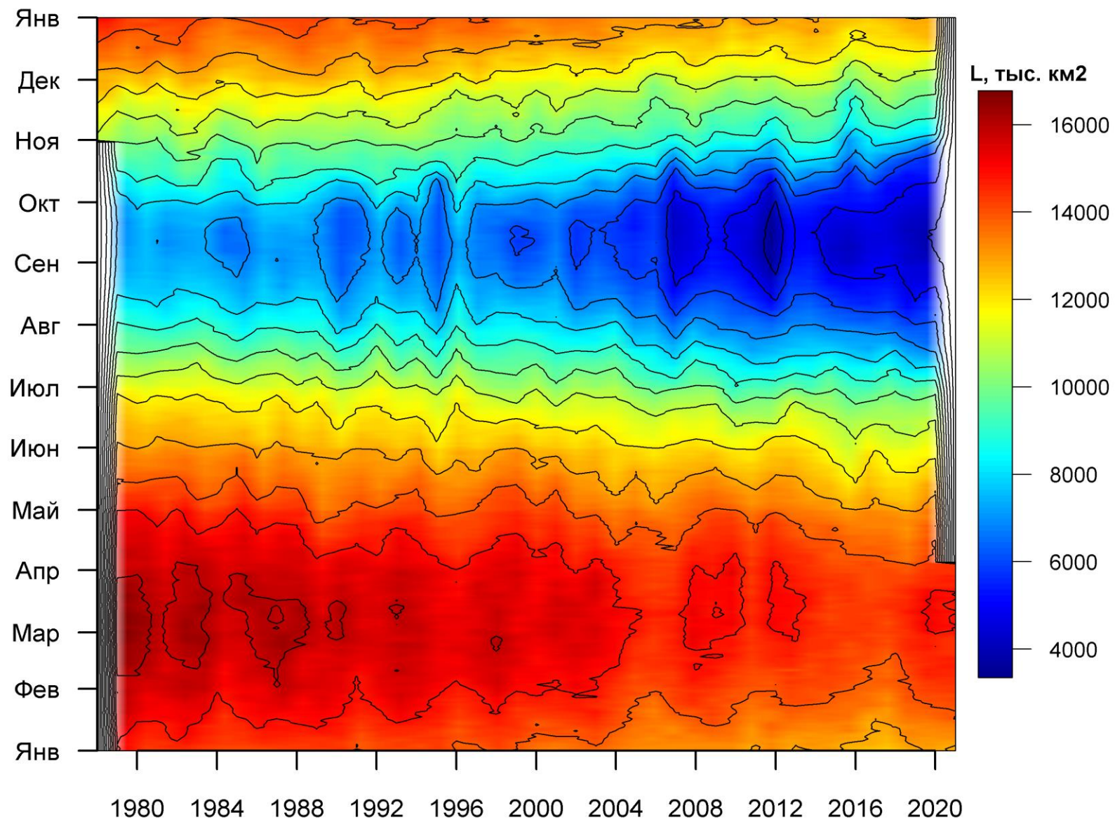
Рисунок 3б – Ежедневные оценки сезонных изменений ледовитости для Северной Полярной Области за период 26.10.1978 – 04.04.2021 на основе расчетов по данным SSMR-SSM/I-SSMIS, алгоритм NASATEAM.
