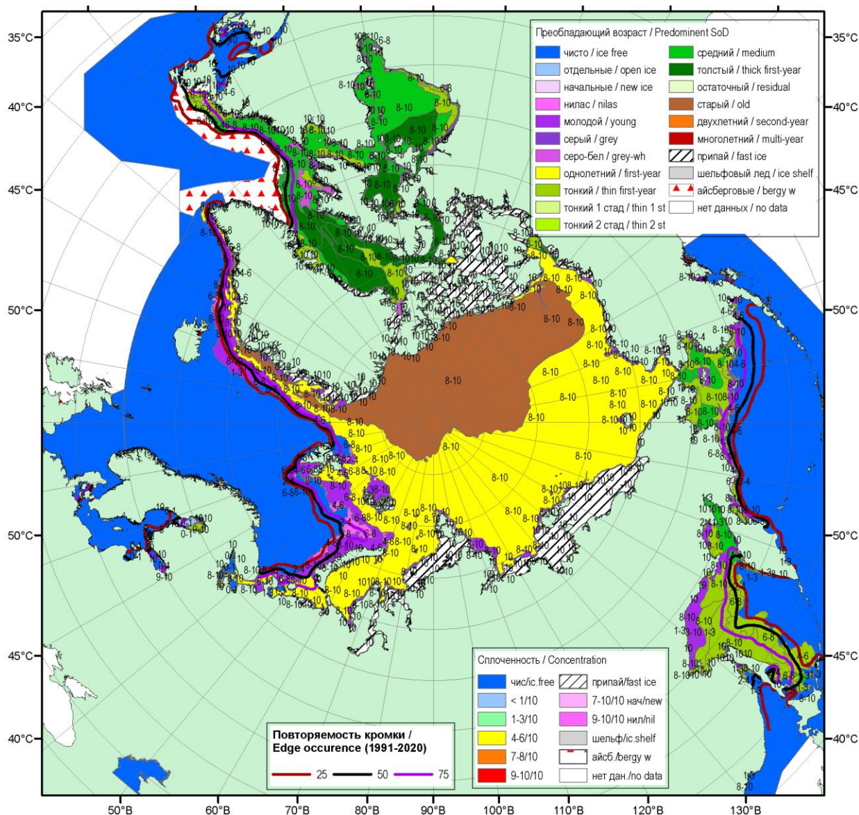
Рисунок 16 – Обзорная ледовая карта СЮ за 01.04-06.04.2021 г. (цветовая раскраска по преобладающему возрасту) на основе ледового анализа ААНИИ (06.04), Национального ледового центра США (01.04) и НИЦ Планета (30.03 Каспийское море) и повторяемость кромки за 01-05.03 за период 1991-2020 гг. по наблюдениям SSMR-SSM/I-SSMIS (алгоритм NASATEAM).
