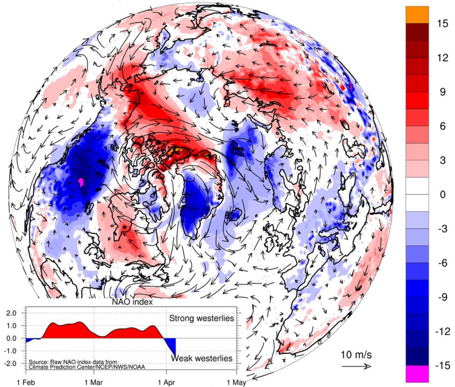
Рисунок 2е – Аномалии приземной температуры воздуха (2м) и осредненные вектора скорости ветра (10 м) за 01.04 - 05.04.2021 гг. относительно периода 2004-2013 гг. ( http://polarportal.dk )
