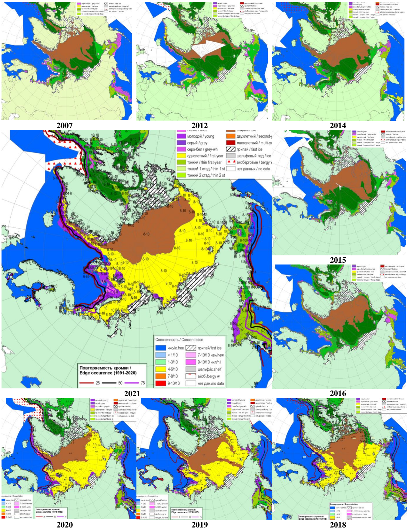
Рисунок 2а – Обзорная ледовая карта САО за 01.04-06.04.2021 г и аналогичные периоды 2007-2020гг. на основе ледового анализа ААНИИ, НИЦ Планета, Канадской ледовой службы и Национального ледового центра США.
