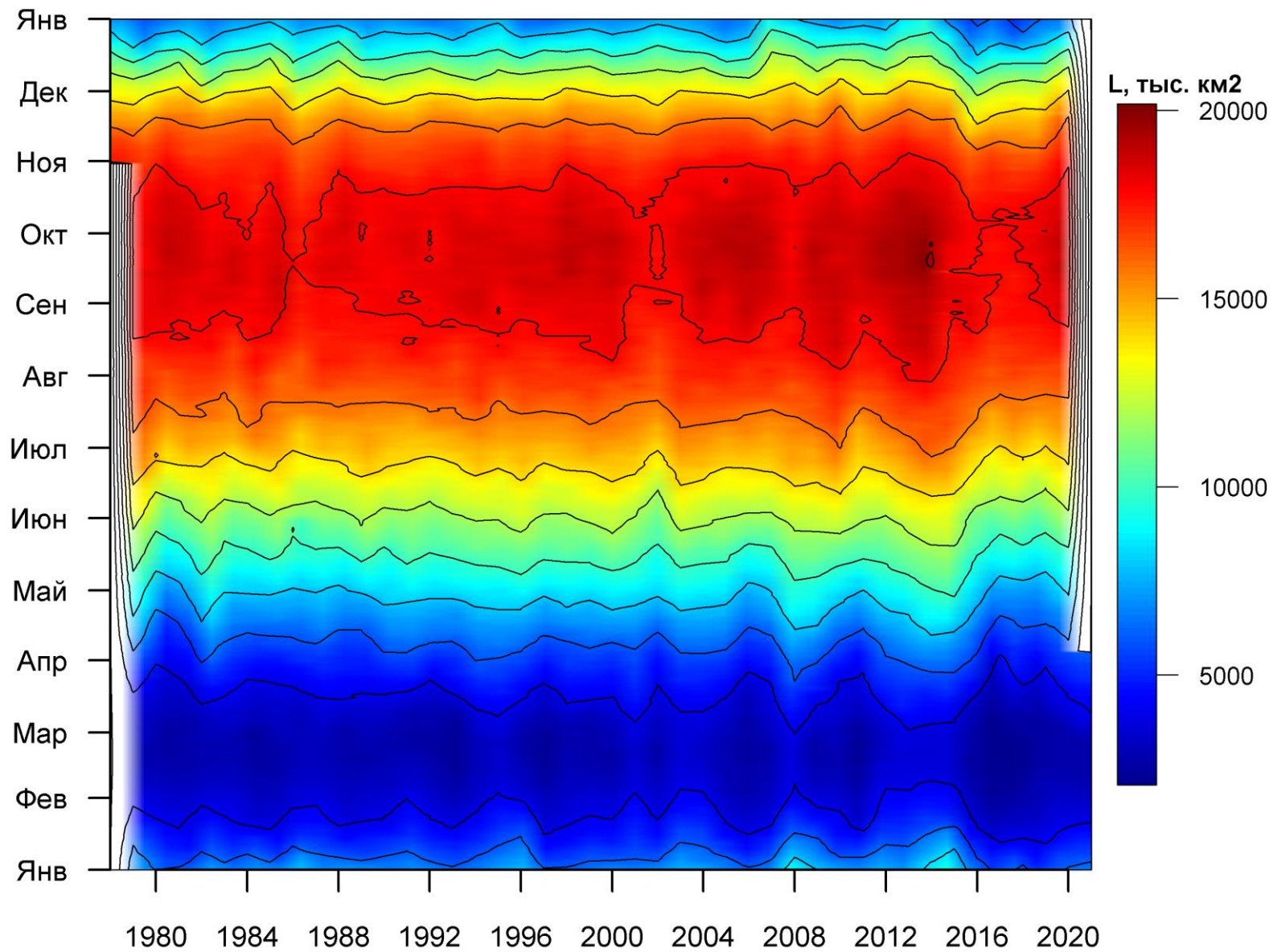
Рисунок 76 – Ежедневные оценки сезонных изменений ледовитости для Южного океана за период 26.10.1978 – 04.04.2021 на основе расчетов по данным SSMR-SSM/I-SSMIS, алгоритм NASATEAM.
