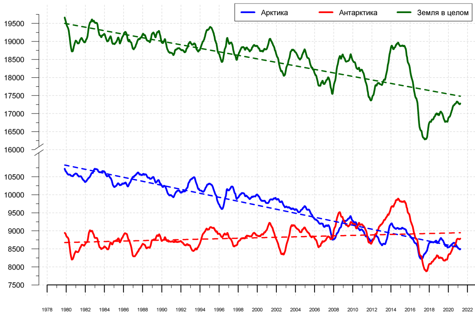
Рисунок 10 – Ежедневные сглаженные окном 365 суток значения приведенной ледовитости (площади морского льда) Арктики, Антарктики и Земли в целом с 26.10.1978 по 04.04.2021 на основе SSMR-SSM/I-SSMIS
