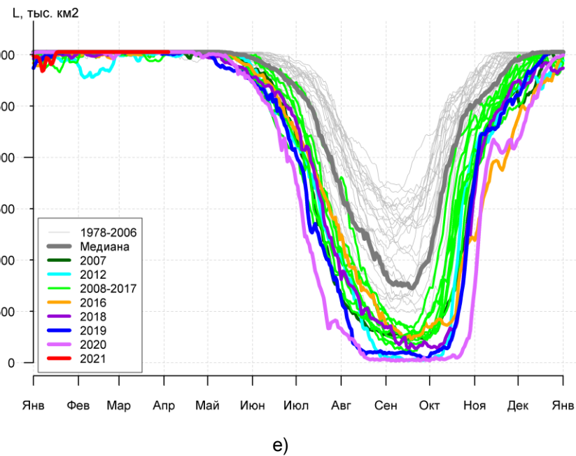
Рисунок 3а – Ежедневные оценки сезонного хода ледовитости для Северной Полярной Области и трех меридиональных секторов за период 26.10.1978 - 04.04.2021 по годам на основе расчетов по данным SSMR-SSM/I-SSMIS, алгоритмы NASATEAM: а) Северная полярная область, б) сектор 45°W-95°E (Гренландское – Карское моря), в) сектор 95°E-170°W (моря Лаптевых – Чукотское и Берингово, Охотское), г) сектор 170°W-45°W (море Бофорта и Канадская Арктика), д) Северный Ледовитый океан, е) Северный морской путь (Карское - Чукотское моря).
