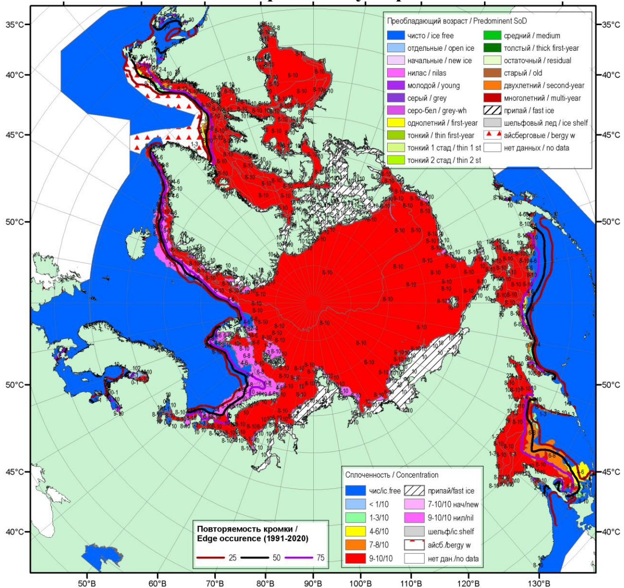
Рисунок 1а – Обзорная ледовая карта СЛО за 01.04-06.04.2021 г. (цветовая раскраска по общей сплоченности) на основе ледового анализа ААНИИ (06.04), Национального ледового центра США (01.04) и НИЦ Планета (30.03 Каспийское море) и повторяемость кромки за 01-05.03 за период 1991-2020 гг. по наблюдениям SSMR-SSM/I-SSMIS (алгоритм NASATEAM).
