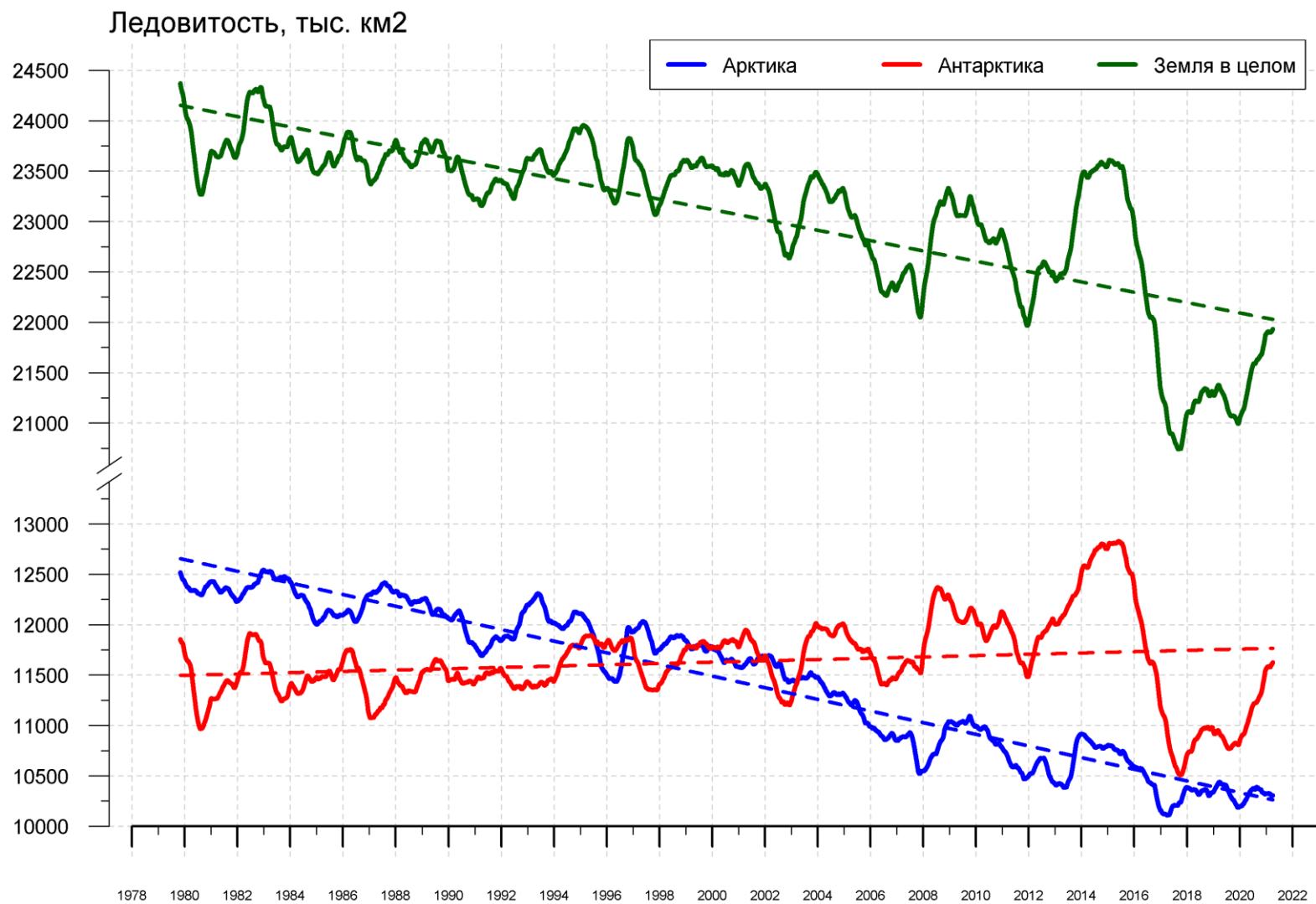
Рисунок 9 – Ежедневные сглаженные окном 365 суток значения ледовитости (площади распространения морского льда) Арктики, Антарктики и Земли в целом с 26.10.1978 по 04.04.2021 на основе SSMR-SSM/I-SSMIS
