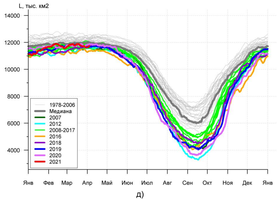
Рисунок 3а – Ежедневные оценки сезонного хода ледовитости для Северной Полярной Области и трех меридиональных секторов за период 26.10.1978 - 04.04.2021 по годам на основе расчетов по данным SSMR-SSM/I-SSMIS, алгоритмы NASATEAM: а) Северная полярная область, б) сектор 45°W-95°E (Гренландское – Карское моря), в) сектор 95°E-170°W (моря Лаптевых – Чукотское и Берингово, Охотское), г) сектор 170°W-45°W (море Бофорта и Канадская Арктика), д) Северный Ледовитый океан, е) Северный морской путь (Карское - Чукотское моря).
