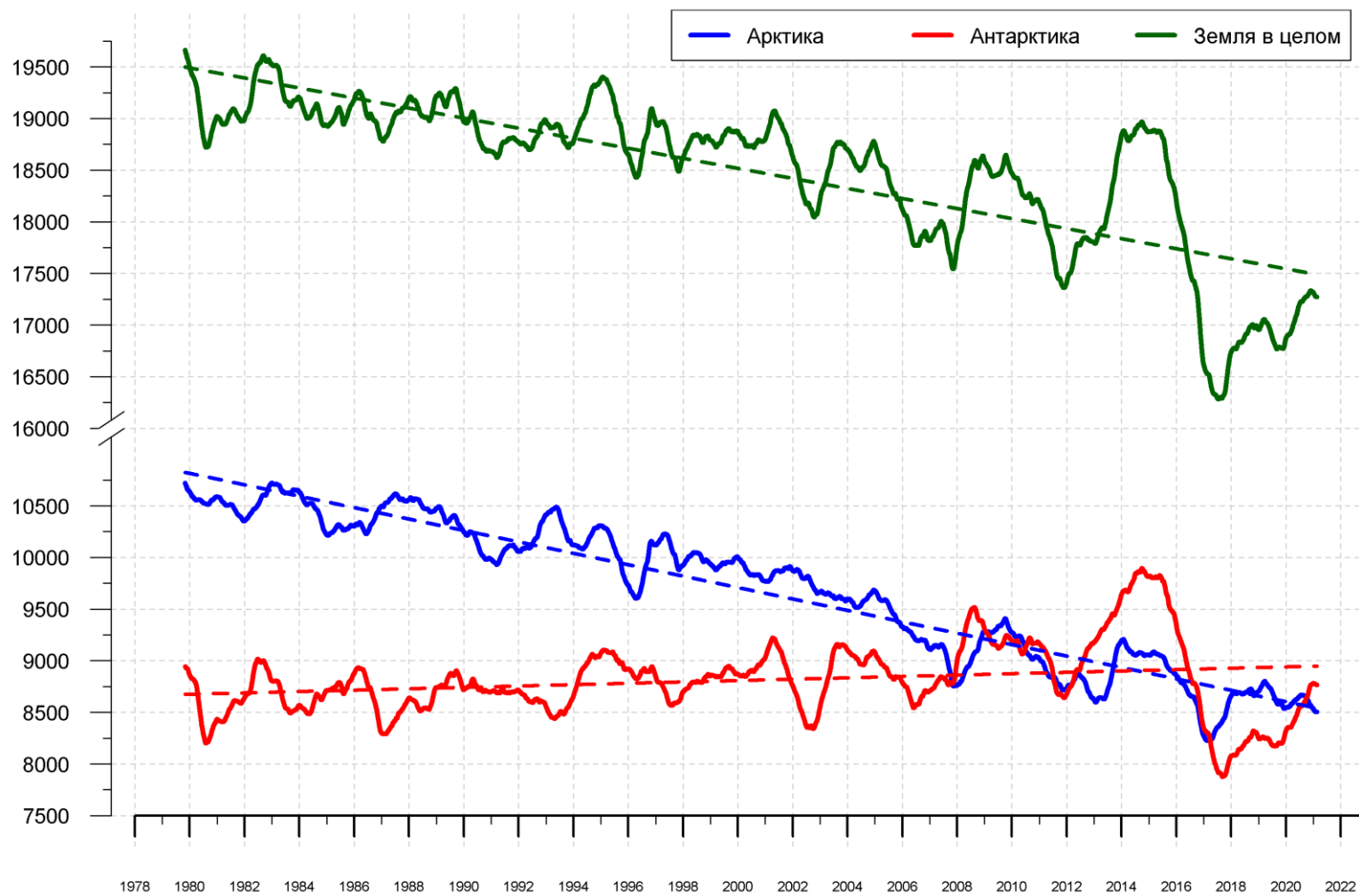
Рисунок 10 – Ежедневные сглаженные окном 365 суток значения приведенной ледовитости (площади морского льда) Арктики, Антарктики и Земли в целом с 26.10.1978 по 18.02.2021 на основе SSMR-SSM/I-SSMIS
