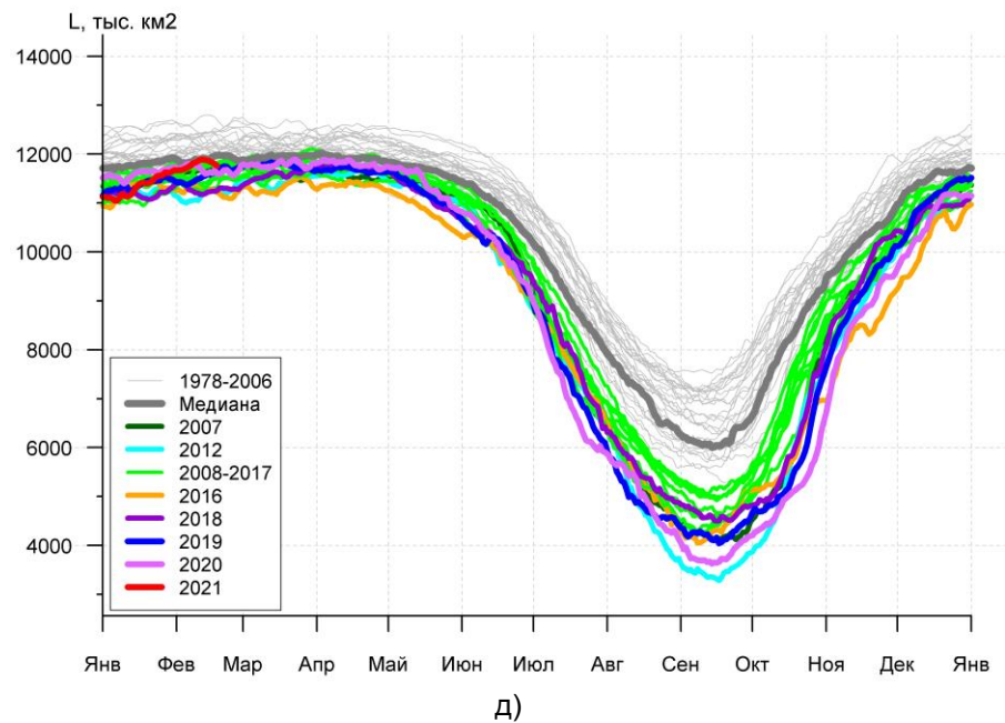
Рисунок 3а – Ежедневные оценки сезонного хода ледовитости для Северной Полярной Области и трех меридиональных секторов за период 26.10.1978 - 18.02.2021 по годам на основе расчетов по данным SSMR-SSM/I-SSMIS, алгоритмы NASATEAM: а) Северная полярная область, б) сектор 45°W-95°E (Гренландское – Карское моря), в) сектор 95°E-170°W (моря Лаптевых – Чукотское и Берингово, Охотское), г) сектор 170°W-45°W (море Бофорта и Канадская Арктика), д) Северный Ледовитый океан, е) Северный морской путь (Карское - Чукотское моря).
