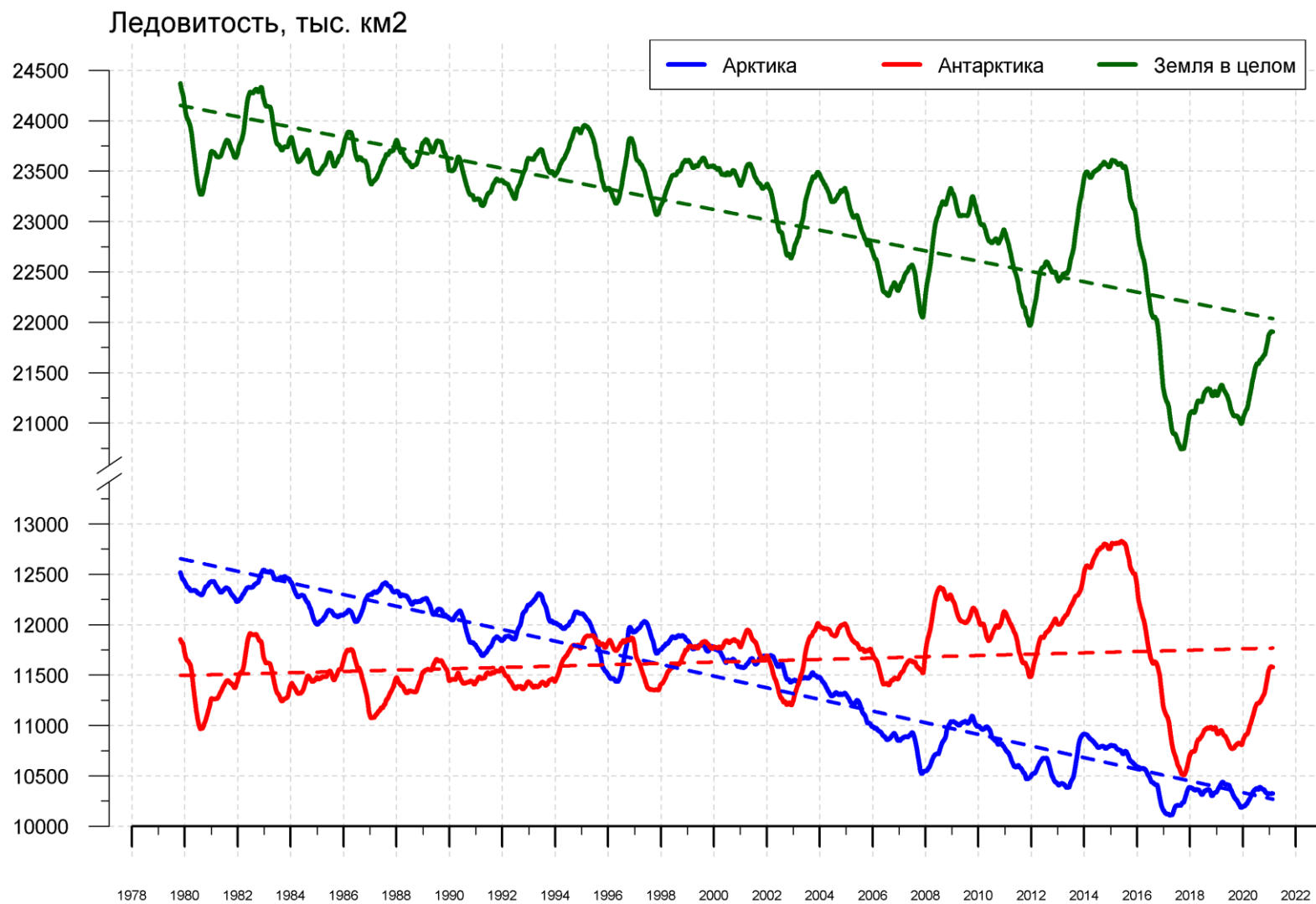
Рисунок 9 – Ежедневные сглаженные окном 365 суток значения ледовитости (площади распространения морского льда) Арктики, Антарктики и Земли в целом с 26.10.1978 по 18.02.2021 на основе SSMR-SSM/I-SSMIS
