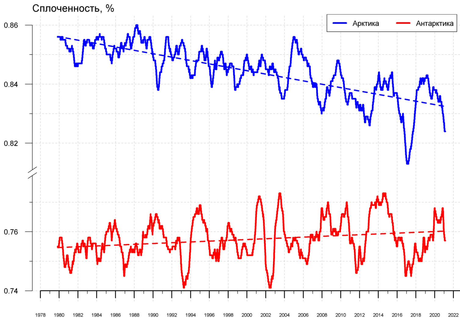
Рисунок 11 – Ежедневные сглаженные окном 365 суток значения средней общей сплоченности Арктики и Антарктики с 26.10.1978 по 18.02.2021 на основе SSMR-SSM/I-SSMIS
