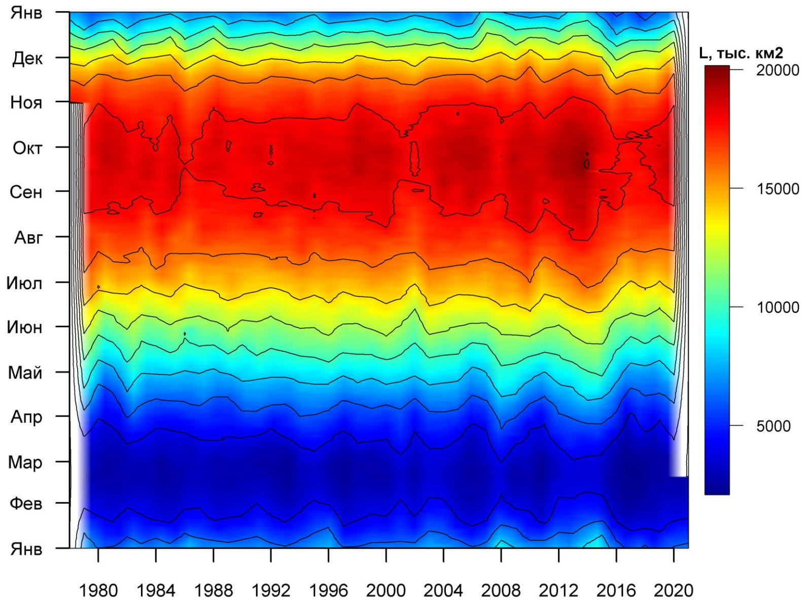
Рисунок 76 – Ежедневные оценки сезонных изменений ледовитости для Южного океана за период 26.10.1978 – 18.02.2021 на основе расчетов по данным SSMR-SSM/I-SSMIS, алгоритм NASATEAM.
