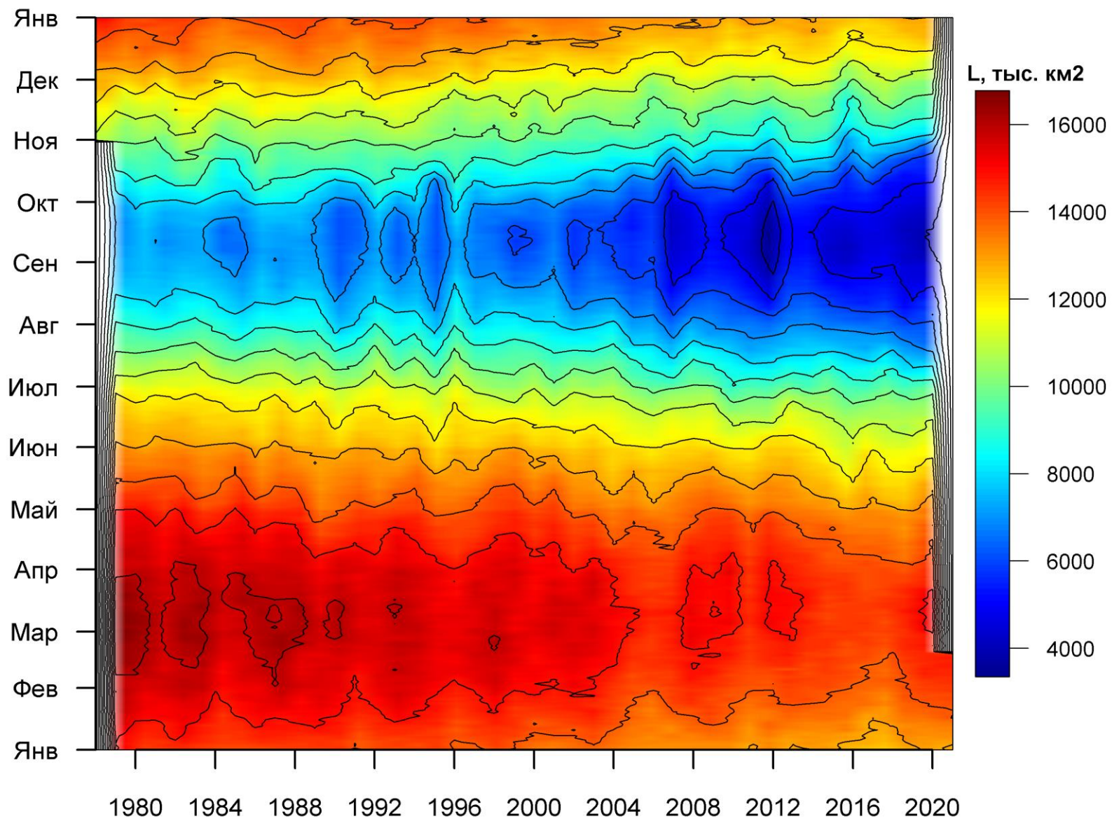
Рисунок 3б – Ежедневные оценки сезонных изменений ледовитости для Северной Полярной Области за период 26.10.1978 – 18.02.2021 на основе расчетов по данным SSMR-SSM/I-SSMIS, алгоритм NASATEAM.
