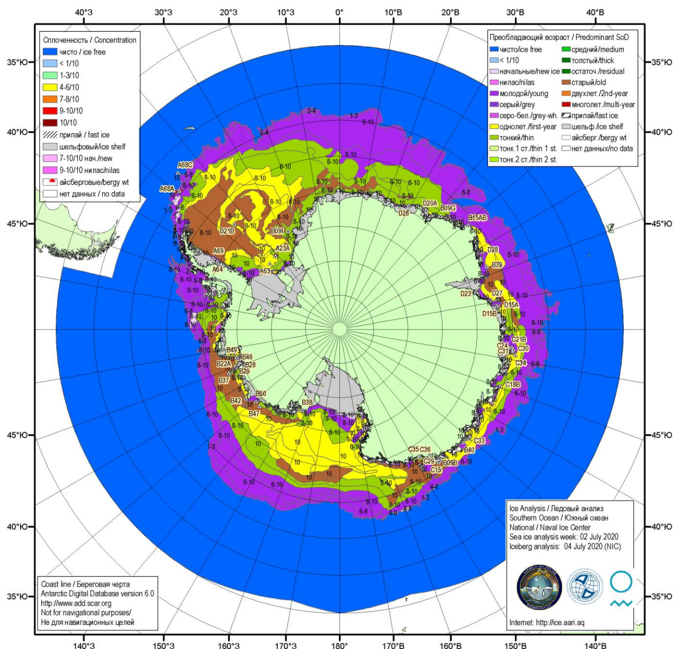
Рисунок 5б – Ледовая карта Южного океана (цветовая окраска по возрасту) и расположение крупных айсбергов на основе информации совместного ледового анализа НЛЦ США, ААНИИ и НМИ (Норвегия) за 02.07.2020.
