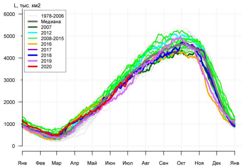
Рисунок 7а – Ежедневные оценки сезонного хода ледовитости Южного Океана и меридиональных секторов за период 26.10.1978 – 05.07.2020 по годам на основе расчетов по данным SSMR-SSM/I-SSMIS, алгоритм NASATEAM: а) Южный Океан, б) Атлантический сектор (60°W-30°E, море Уэдделла), в) Индоокеанский сектор (30°E-150°E, моря Космонавтов, Содружества, Моусона), г) Тихоокеанский сектор (150°E-60°W, моря Росса, Беллингаузена)
