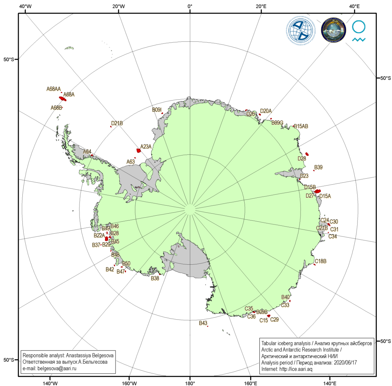
Рисунок 5д – Анализ ААНИИ крупных айсбергов Южного океана за 17.06.2020.
