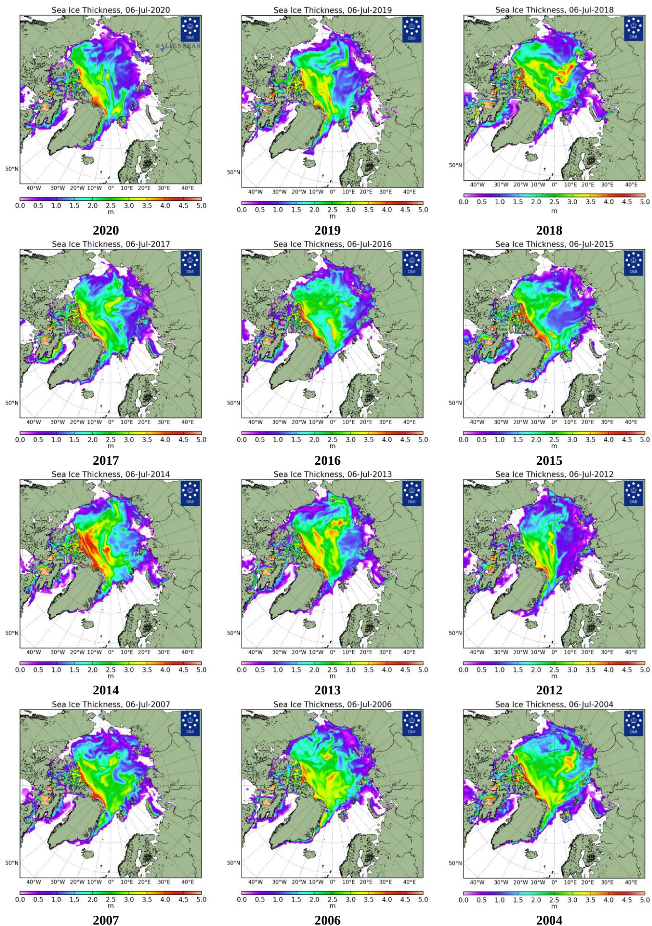
Рисунок 26 – Поля распределения средневзвешенной толщины льда совместной модели морского льда – океана NUCOM/CICE Датского метеорологического института 17.02.2004-06.07.2020 гг.
