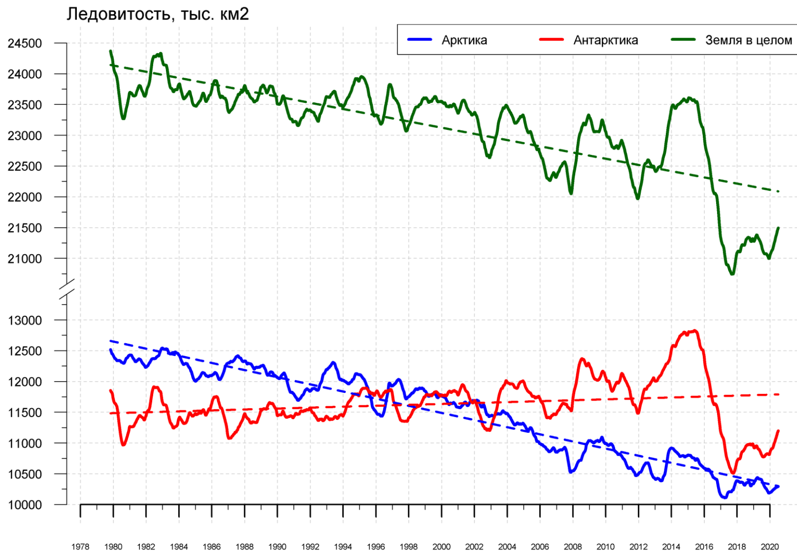
Рисунок 9 – Ежедневные сглаженные окном 365 суток значения приведенной ледовитости (площади морского льда) Арктики, Антарктики и Земли в целом с 26.10.1978 по 05.07.2020 на основе SSMR-SSM/I-SSMIS
