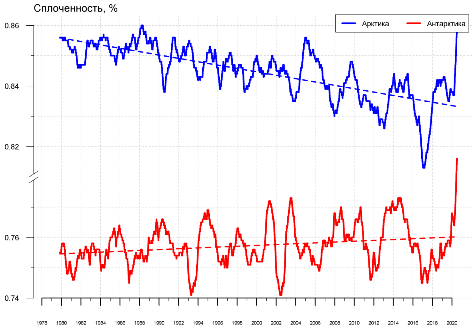
Рисунок 11 – Ежедневные сглаженные окном 365 суток значения средней общей сплоченности Арктики и Антарктики с 26.10.1978 по 05.07.2020 на основе SSMR-SSM/I-SSMIS
