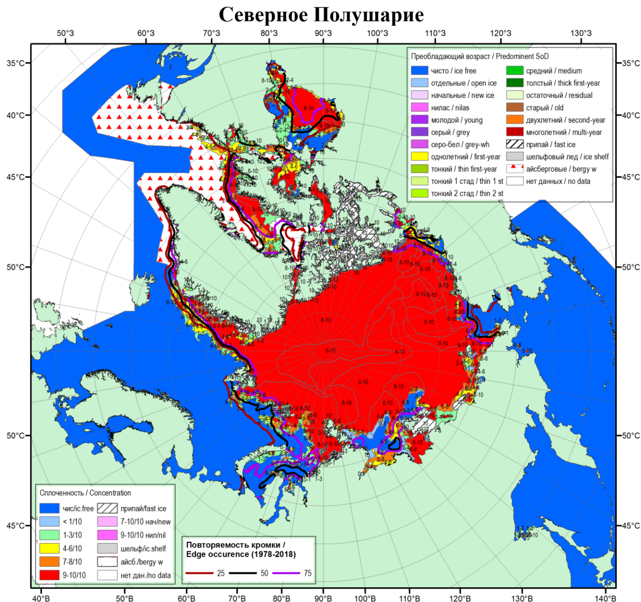
Рисунок 1а – Обзорная ледовая карта СЛО за 02.07.2020-07.07.2020 г. (цветовая раскраска по общей сплоченности) на основе ледового анализа ААНИИ (07.07), Национального ледового центра США (02.07) и повторяемость кромки за 01-05.07 за период 1979-2018 гг. по наблюдениям SSMR-SSM/I-SSMIS (алгоритм NASATEAM).
