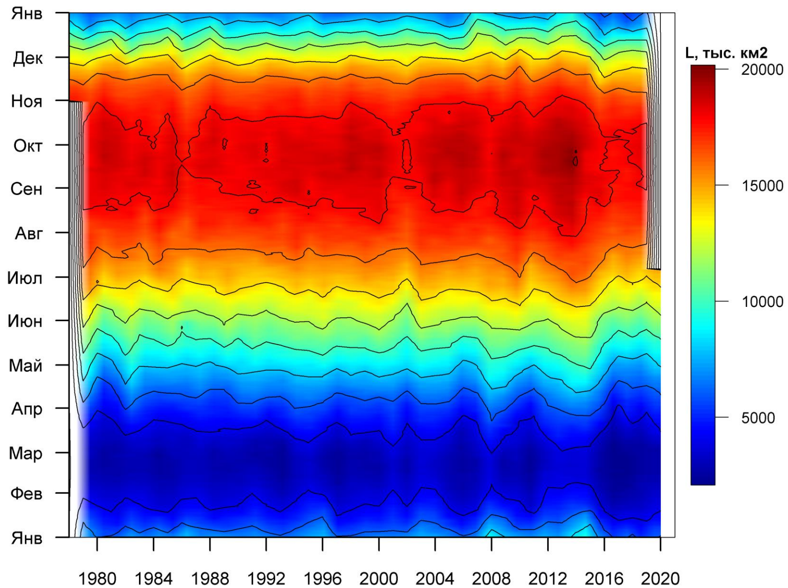
Рисунок 76 – Ежедневные оценки сезонных изменений ледовитости для Южного океана за период 26.10.1978 - 05.07.2020 на основе расчетов по данным SSMR-SSM/I-SSMIS, алгоритм NASATEAM.
