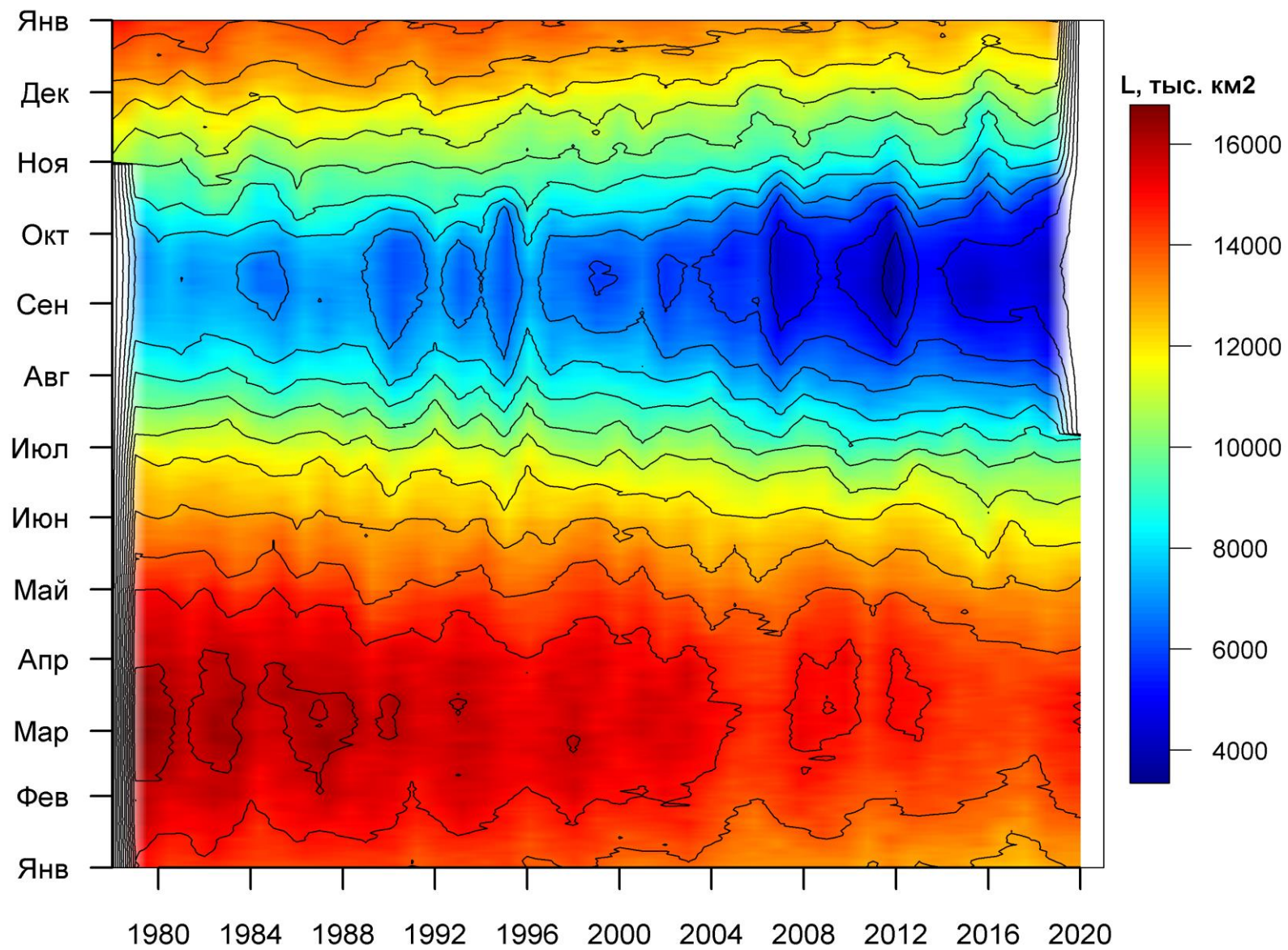
Рисунок 3б – Ежедневные оценки сезонных изменений ледовитости для Северной Полярной Области за период 26.10.1978 – 05.07.2020 на основе расчетов по данным SSMR-SSM/I-SSMIS, алгоритм NASATEAM.
