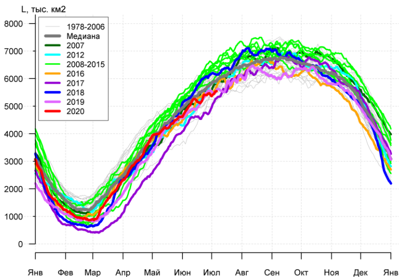
Рисунок 7а – Ежедневные оценки сезонного хода ледовитости Южного Океана и меридиональных секторов за период 26.10.1978 – 05.07.2020 по годам на основе расчетов по данным SSMR-SSM/I-SSMIS, алгоритм NASATEAM: а) Южный Океан, б) Атлантический сектор (60°W-30°E, море Уэдделла), в) Индоокеанский сектор (30°E-150°E, моря Космонавтов, Содружества, Моусона), г) Тихоокеанский сектор (150°E-60°W, моря Росса, Беллингаузена)
