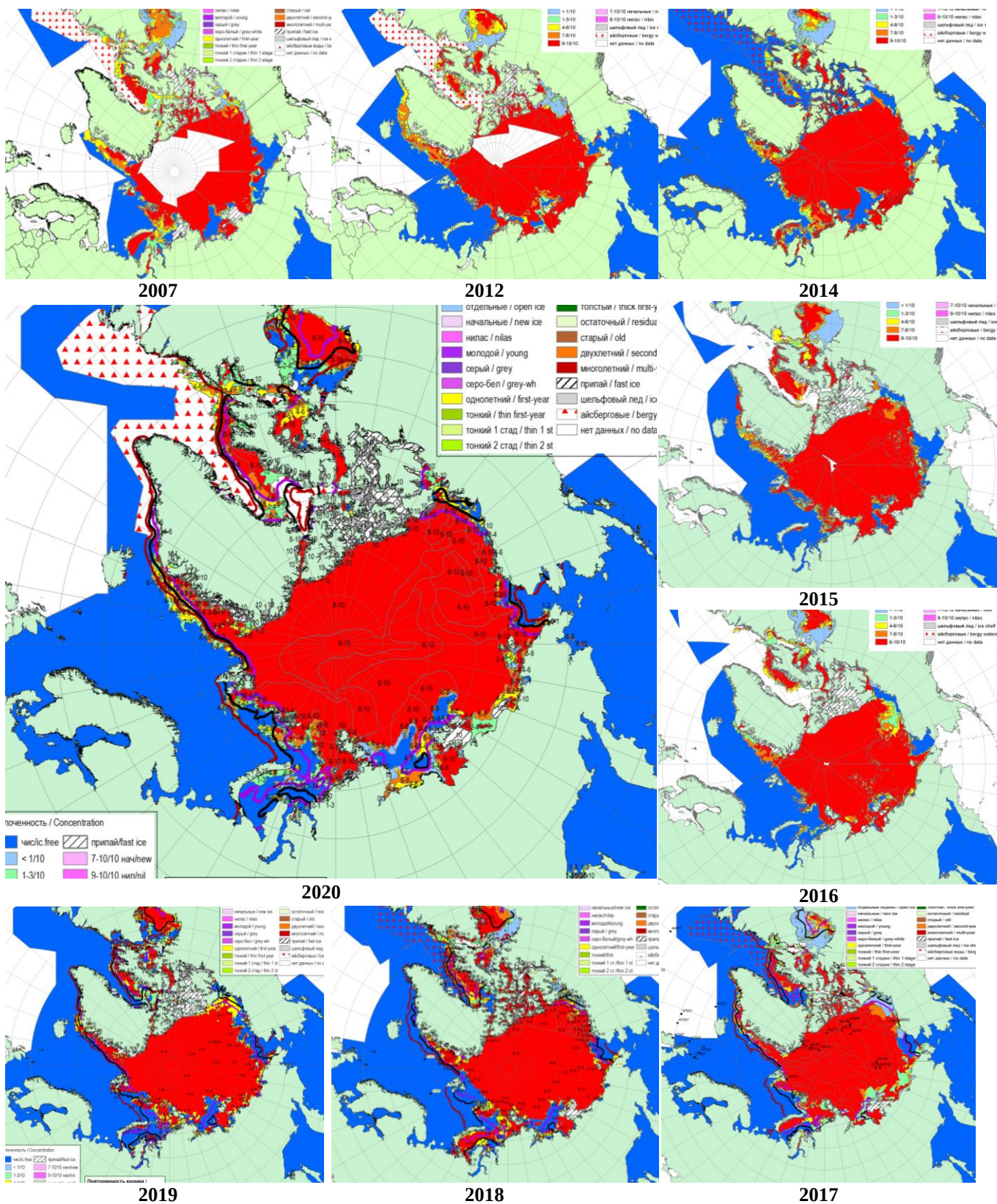
Рисунок 2а – Обзорная ледовая карта СЛО за 02.07 –07.07.2020 г. и аналогичные периоды 2007-2019гг. на основе ледового анализа ААНИИ, НИЦ Планета, Канадской ледовой службы и Национального ледового центра США.
