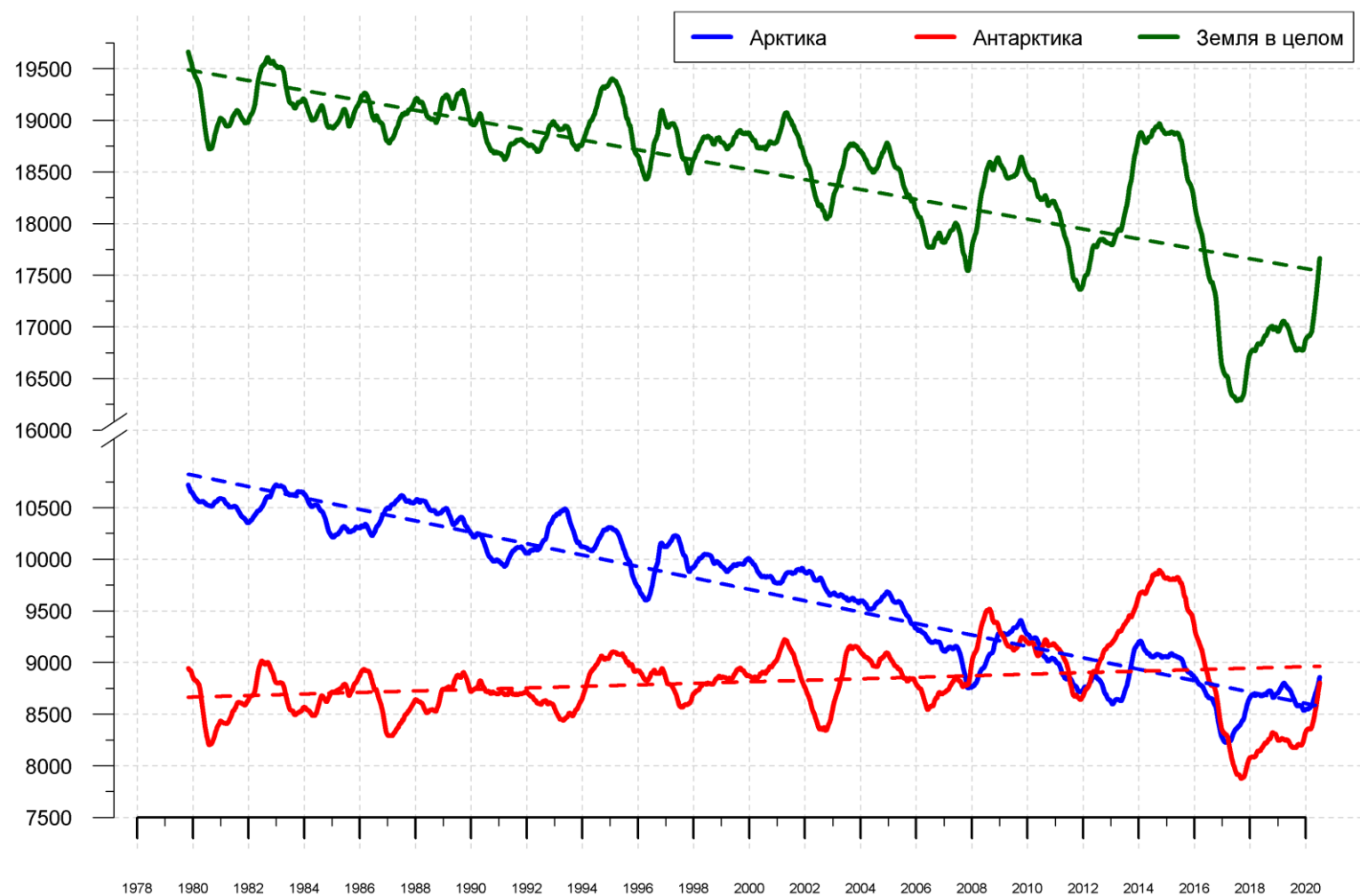
Рисунок 10 – Ежедневные сглаженные окном 365 суток значения ледовитости (площади распространения морского льда) Арктики, Антарктики и Земли в целом с 26.10.1978 по 05.07.2020 на основе SSMR-SSM/I-SSMIS
