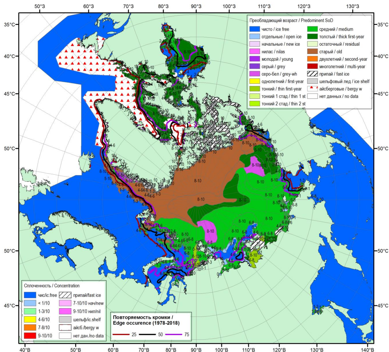
Рисунок 16 – Обзорная ледовая карта СЛО за 02.07.2020-07.07.2020 г. (цветовая раскраска по преобладающему возрасту) на основе ледового анализа ААНИИ (07.07), Национального ледового центра США (02.07) и повторяемость кромки за 01-05.07 за период 1979-2018 гг. по наблюдениям SSMR-SSM/I-SSMIS (алгоритм NASATEAM).
