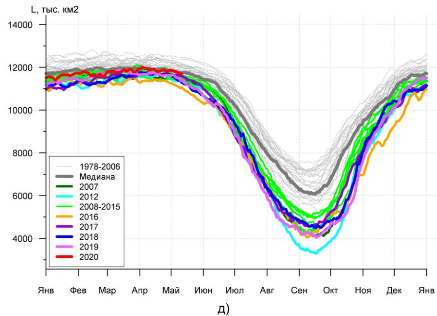
Рисунок 3а – Ежедневные оценки сезонного хода ледовитости для Северной Полярной Области и трех меридиональных секторов за период 26.10.1978 – 10.05.2020 по годам на основе расчетов по данным SSMR-SSM/I-SSMIS, алгоритмы NASATEAM: а) Северная полярная область, б) сектор 45°W-95°E (Гренландское – Карское моря), в) сектор 95°E-170°W (моря Лаптевых – Чукотское и Берингово, Охотское), г) сектор 170°W-45°W (море Бофорта и Канадская Арктика), д) Северный Ледовитый океан, е) Северный морской путь (Карское - Чукотское моря).
