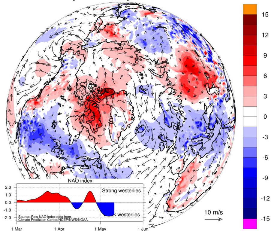
Рисунок 2е – Аномалии приземной температуры воздуха (2м) и осредненные вектора скорости ветра (10 м) за 07.05.-11.05.2020 гг. относительно периода 2004-2013 гг. ( http://polarportal.dk )
