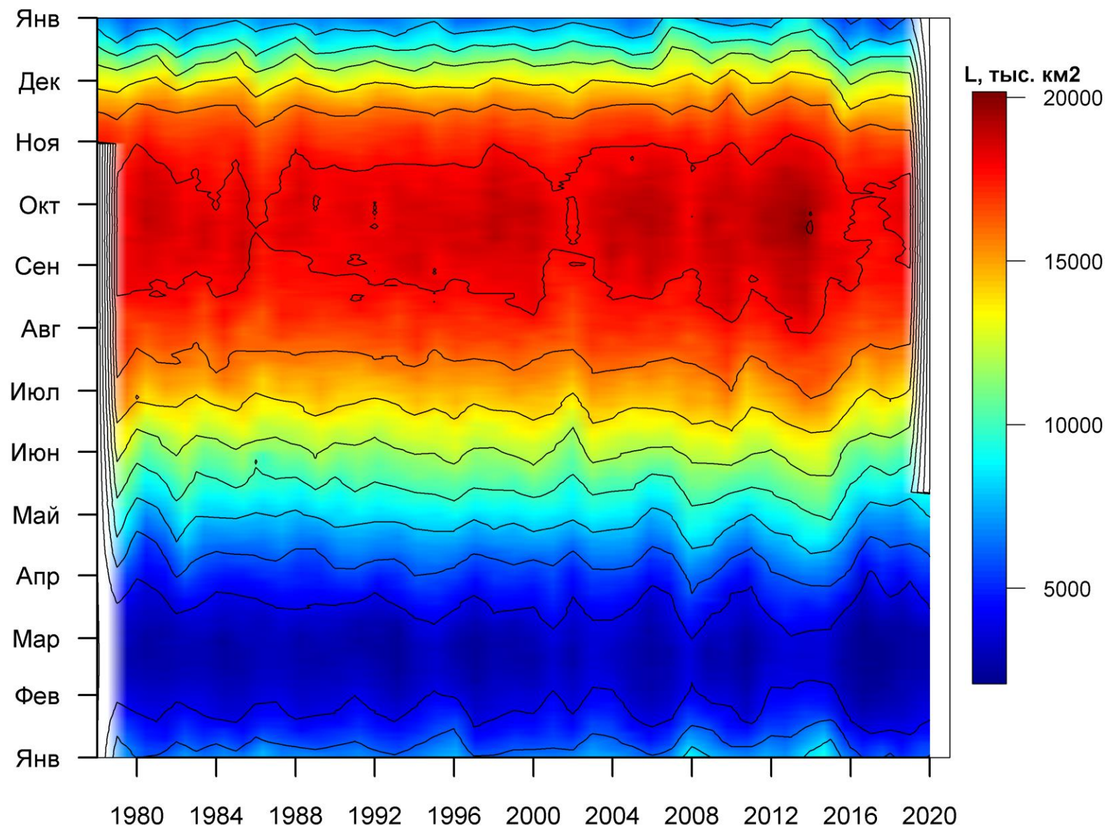
Рисунок 76 – Ежедневные оценки сезонных изменений ледовитости для Южного океана за период 26.10.1978 - 10.05.2020 на основе расчетов по данным SSMR-SSM/I-SSMIS, алгоритм NASATEAM.
