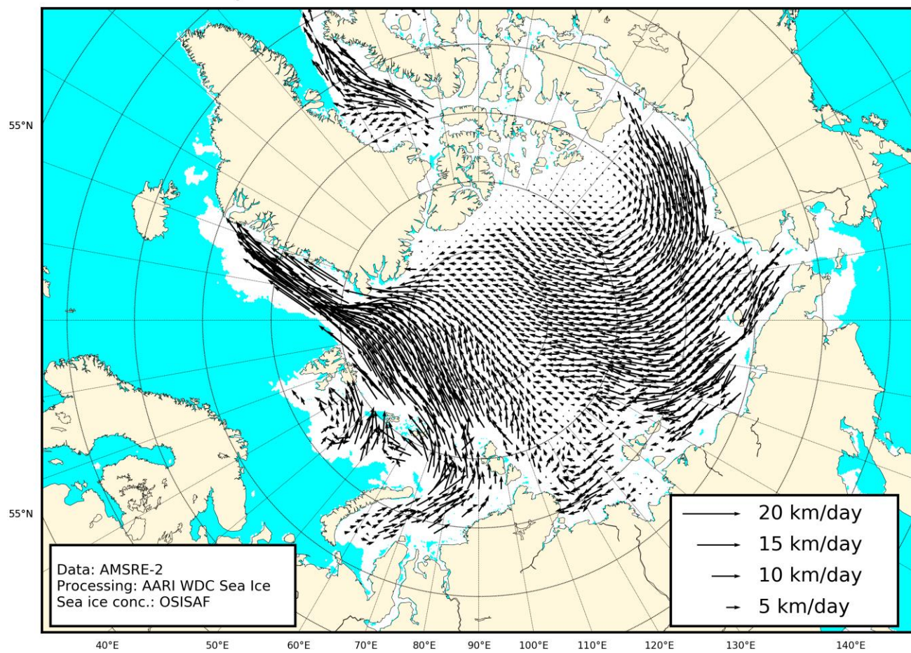
Рисунок 2г – Поле дрейфа морского льда Арктики за 04.05-11.05.2020 г., источник данных EUMETSAT OSISAF.
