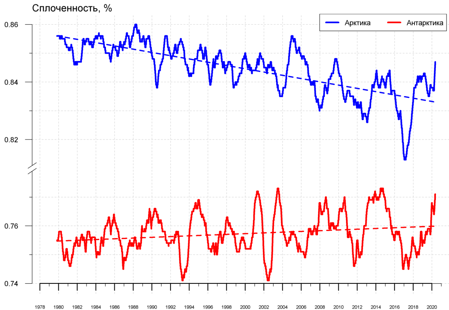
Рисунок 11 – Ежедневные сглаженные окном 365 суток значения средней общей сплоченности Арктики и Антарктики с 26.10.1978 по 10.05.2020 на основе SSMR-SSM/I-SSMIS
