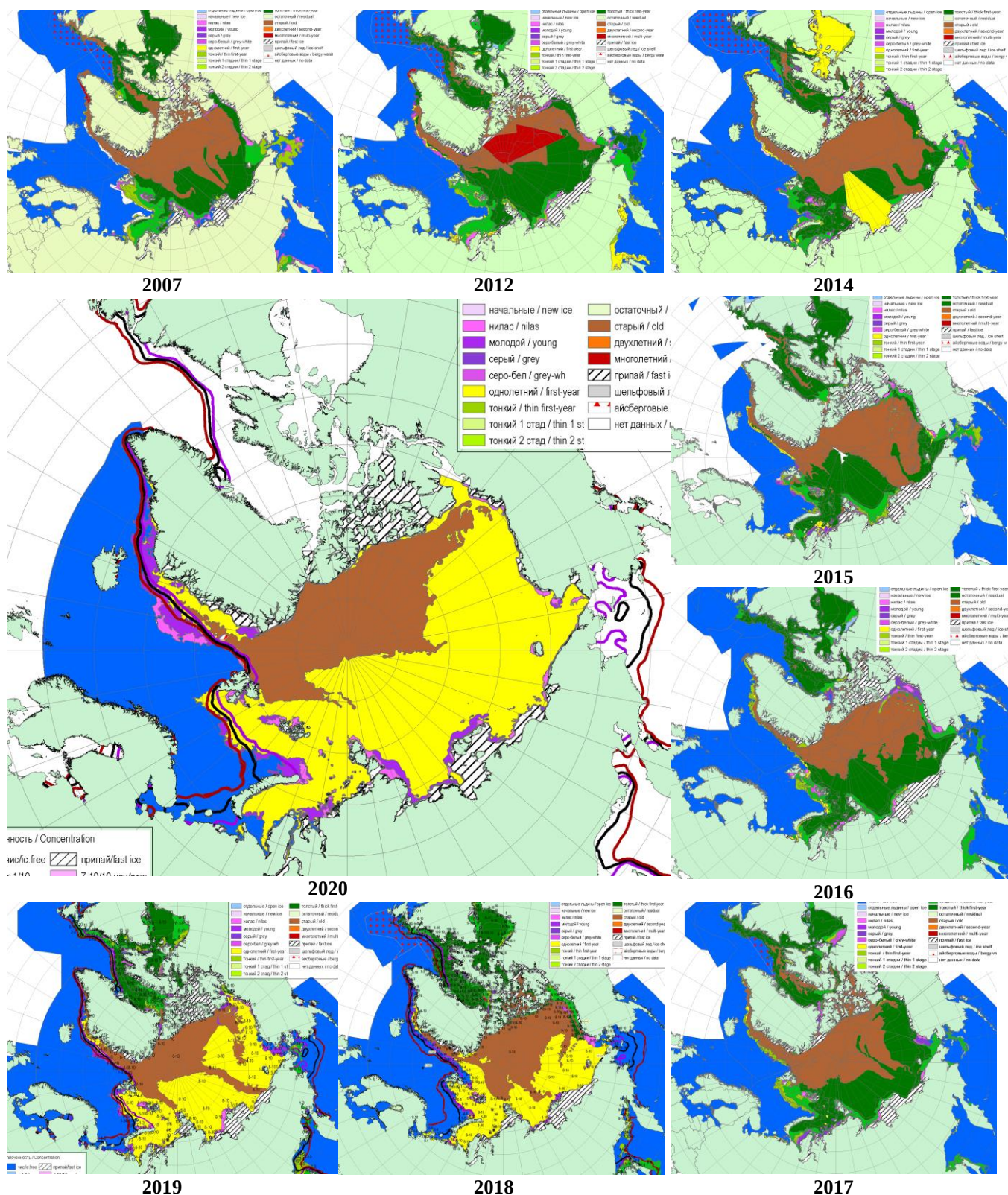
Рисунок 2а – Обзорная ледовая карта САО за 07.05 – 12.05.2020 г. и аналогичные периоды 2007-2019гг. на основе ледового анализа ААНИИ, НИЦ Планета, Канадской ледовой службы и Национального ледового центра США.
