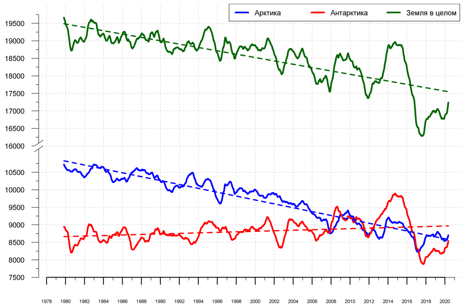
Рисунок 10 – Ежедневные сглаженные окном 365 суток значения ледовитости (площади распространения морского льда) Арктики, Антарктики и Земли в целом с 26.10.1978 по 10.05.2020 на основе SSMR-SSM/I-SSMIS
