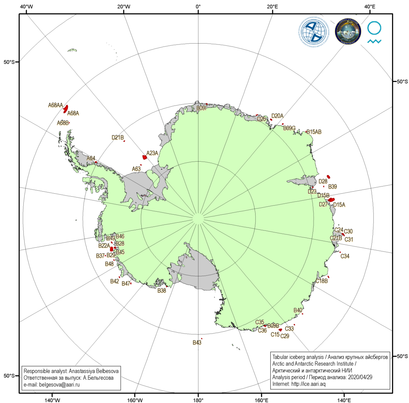
Рисунок 5д – Анализ ААНИИ крупных айсбергов Южного океана за 29.04.2020.
