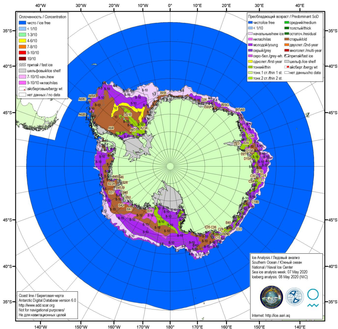
Рисунок 5б – Ледовая карта Южного океана (цветовая окраска по возрасту) и расположение крупных айсбергов на основе информации совместного ледового анализа НЛЦ США, ААНИИ и НМИ (Норвегия) за 07.05.2020.
