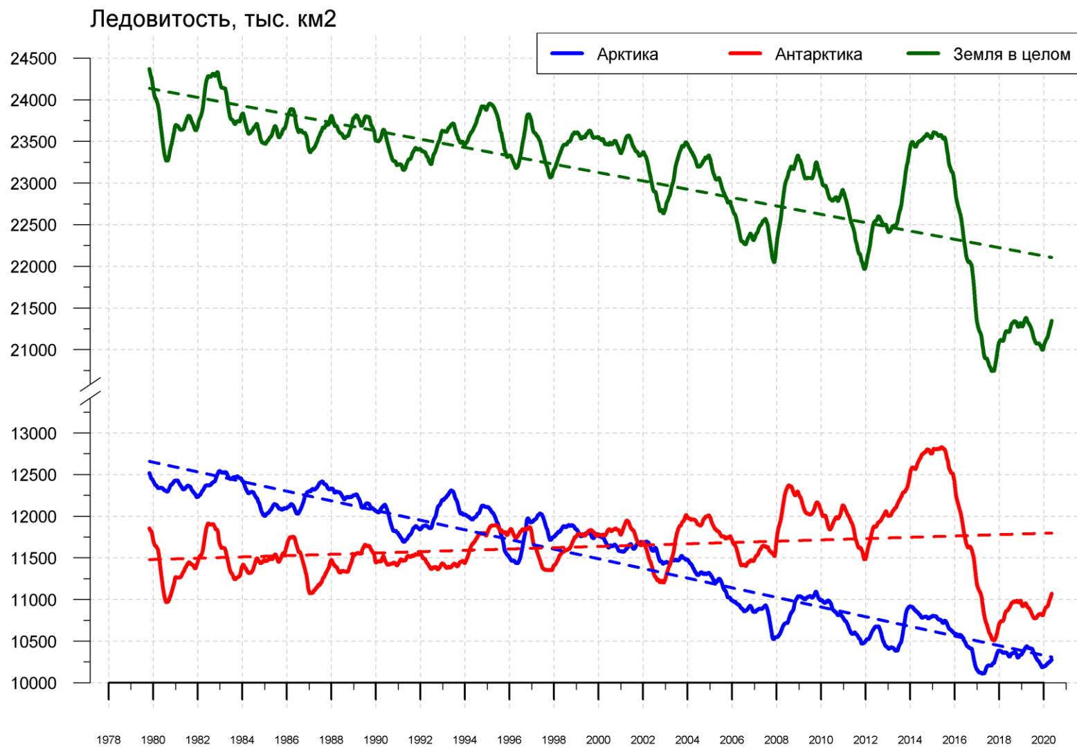
Рисунок 9 – Ежедневные сглаженные окном 365 суток значения приведенной ледовитости (площади морского льда) Арктики, Антарктики и Земли в целом с 26.10.1978 по 10.05.2020 на основе SSMR-SSM/I-SSMIS
