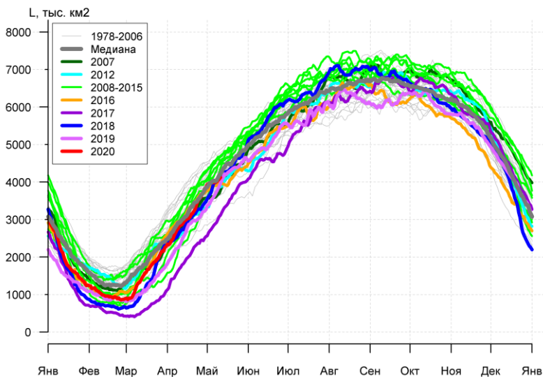
Рисунок 7а – Ежедневные оценки сезонного хода ледовитости Южного Океана и меридиональных секторов за период 26.10.1978 – 10.05.2020 по годам на основе расчетов по данным SSMR-SSM/I-SSMIS, алгоритм NASATEAM: а) Южный Океан, б) Атлантический сектор (60°W-30°E, море Уэдделла), в) Индоокеанский сектор (30°E-150°E, моря Космонавтов, Содружества, Моусона), г) Тихоокеанский сектор (150°E-60°W, моря Росса, Беллингаузена)
