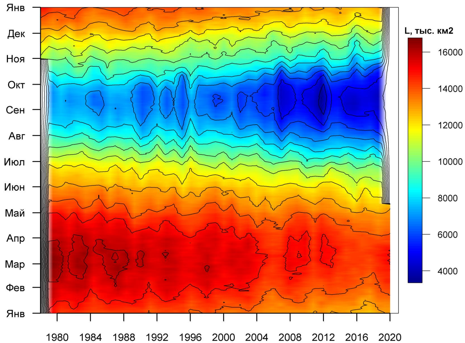
Рисунок 3б – Ежедневные оценки сезонных изменений ледовитости для Северной Полярной Области за период 26.10.1978 – 10.05.2020 на основе расчетов по данным SSMR-SSM/I-SSMIS, алгоритм NASATEAM.
