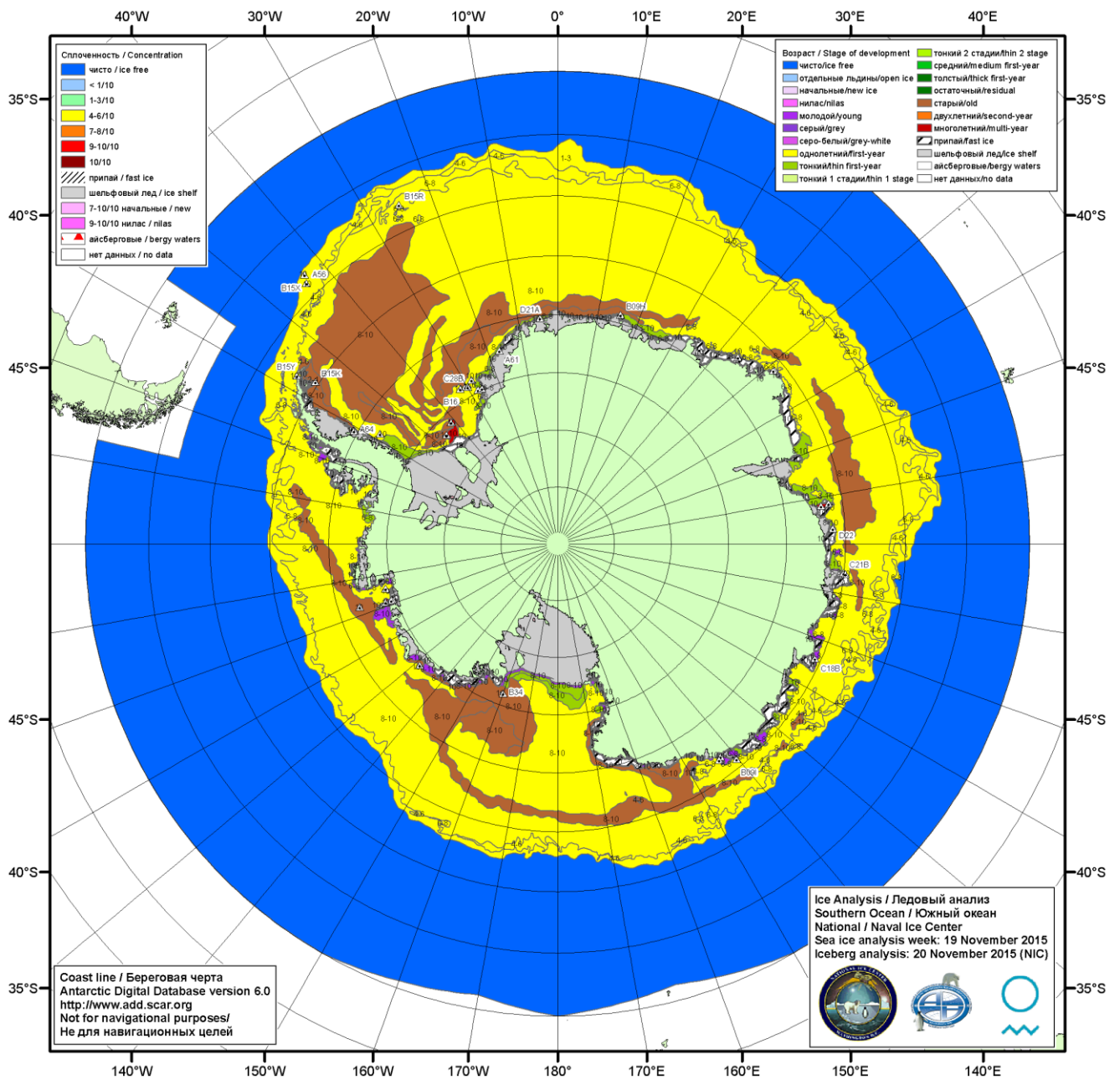
Рисунок 7б – Ледовая карта Южного океана (цветовая окраска по возрасту) и расположение крупных айсбергов на основе информации совместного ледового анализа НЛЦ США, ААНИИ и НМИ (Норвегия) за 19.11.2015.
