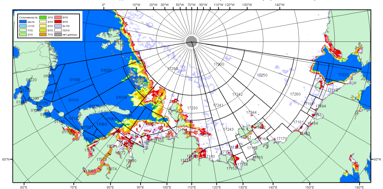
Рисунок 2б – Общая сплоченность морского льда морей СМП по данным AMSR2 на 24.11.2015 01:08 UTC и границы районов ГМССБ МЕТЗОН XX и XXI.
