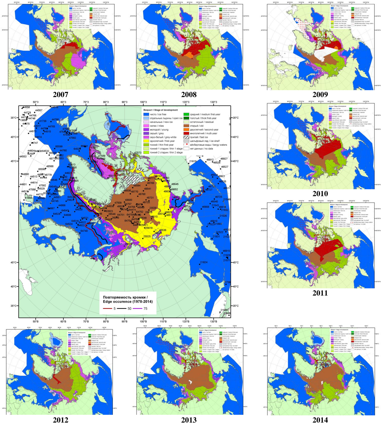
Рисунок 3 – Обзорная ледовая карта СЛО за 16.11 - 24.11.2015 г. и аналогичные периоды 2007-2014 гг. на основе ледового анализа ААНИИ, Канадской ледовой службы и Национального ледового центра США.
