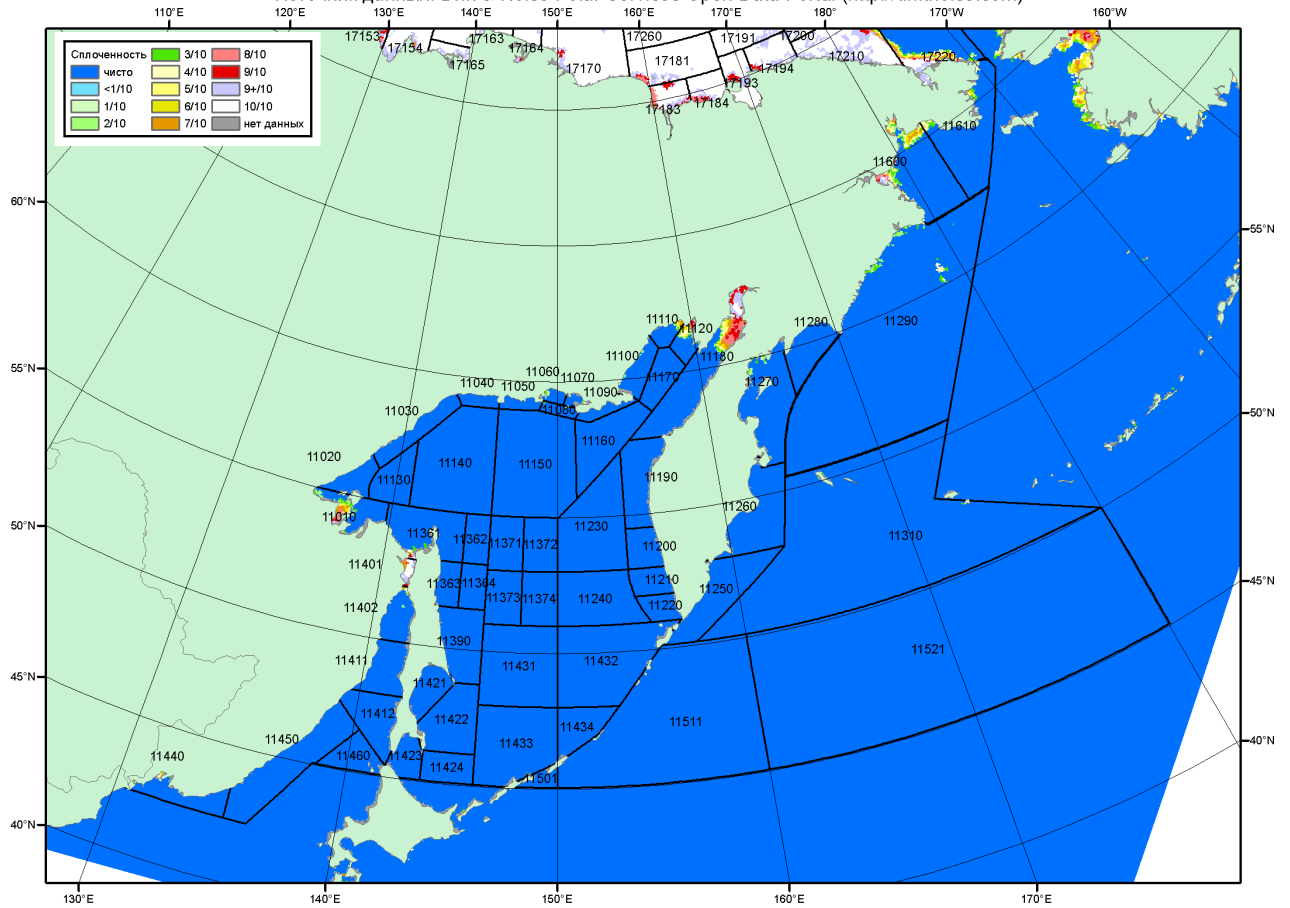
Рисунок 2в – Общая сплоченность морского льда дальневосточных морей по данным AMSR2 на 24.11.2015 01:08UTC и границы районов ГМССБ МЕТЗОНЫ XIII.
