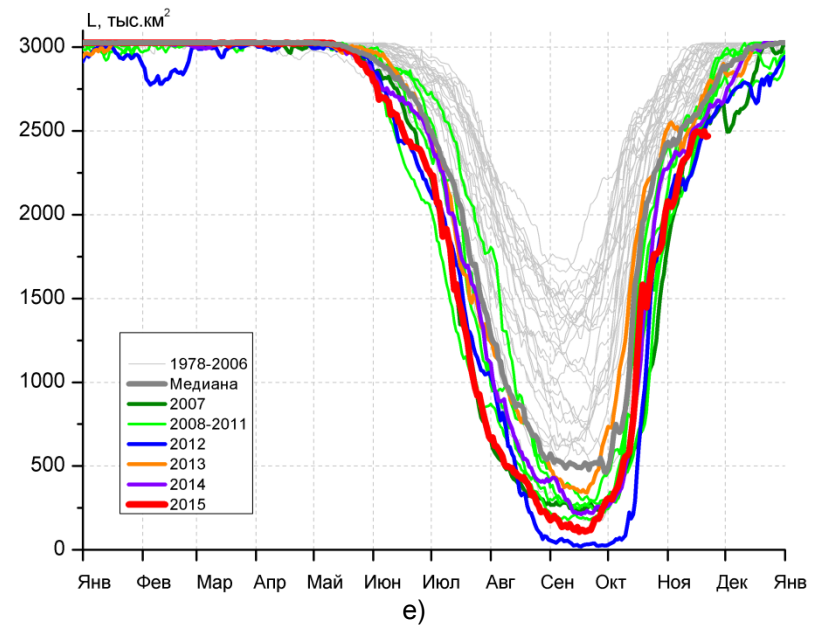
Рисунок 5 – Ежедневные оценки сезонного хода ледовитости для Северной Полярной Области и трех меридиональных секторов за период 26.10.1978 - 22.11.2015 по годам на основе расчетов по данным SSMR-SSM/I-SSMIS-AMSR2, алгоритмы NASATEAM/BOOTSTRAP: а) Северная полярная область, б) сектор 45°W-95°E (Гренландское – Карское моря), в) сектор 95°E-170°W (моря Лаптевых – Чукотское и Берингово, Охотское), г) сектор 170°W-45°W (море Бофорта и Канадская Арктика), д) Северный Ледовитый океан, е) Северный морской путь (Карское - Чукотское моря).
