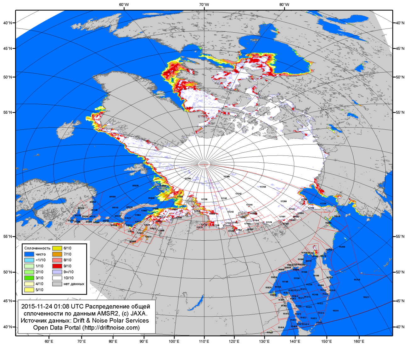
Рисунок 2а – Общая сплоченность морского льда СЛО и субарктических морей по данным AMSR2 на 24.11.2015 01:08 UTC и границы районов ГМССБ МЕТЗОН XIII, XX и XXI.
